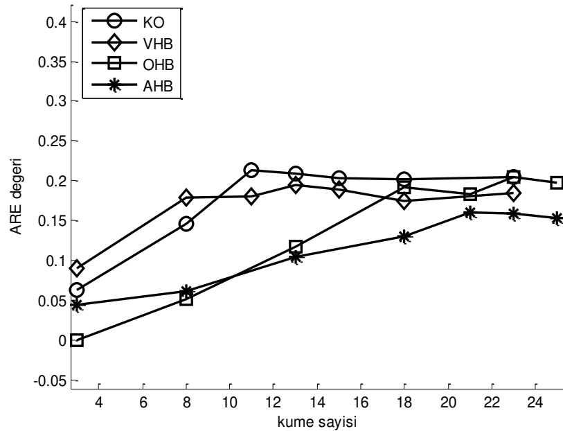
Şekil 4.21 Gruplama uygulanmış 40 adım aralıklı ATBA için kümeleme başarıları
