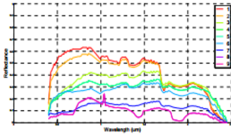
Şekil 7 Seçilen Noktaların Yansıma Değerleri
