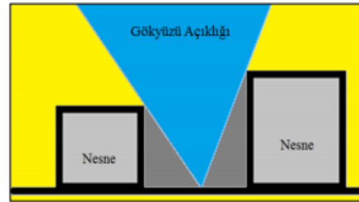
Şekil 3 Gökyüzü Açıklığı
