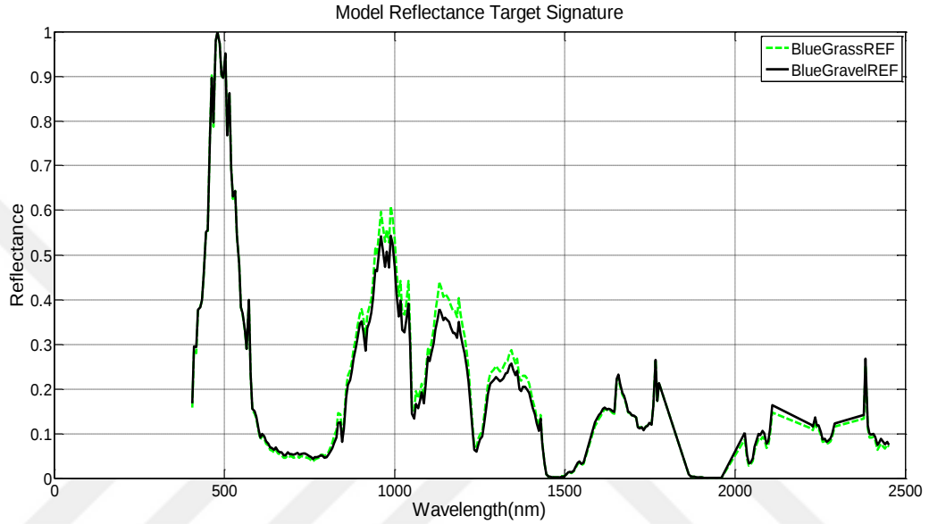
Şekil 40 Çim ve çakıl arkaplanında mavi keçe materyalinin gölge düzeltilmiş spektral yansımaları grafiği
