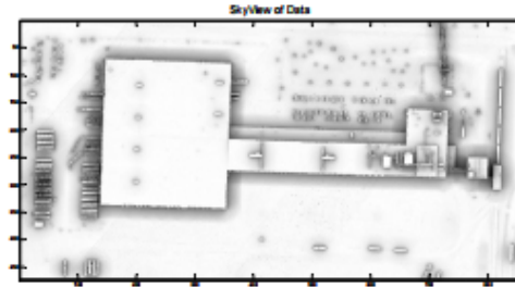
Şekil 5 Gökyüzü Açıklığı Haritası
