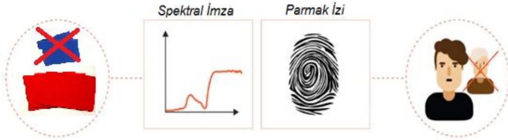
Şekil 2 Spektral imza [3]
