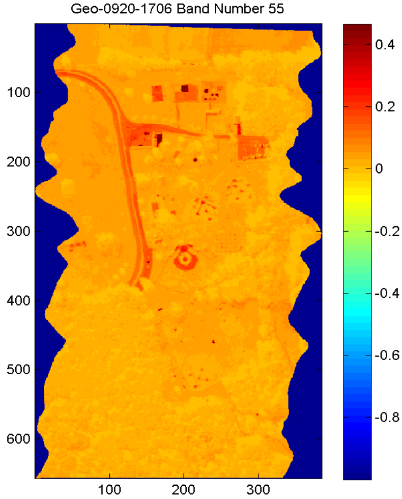
Şekil 24 UTC 17:06’ da alınan kırmızı dalga boylu yansıma verisi
