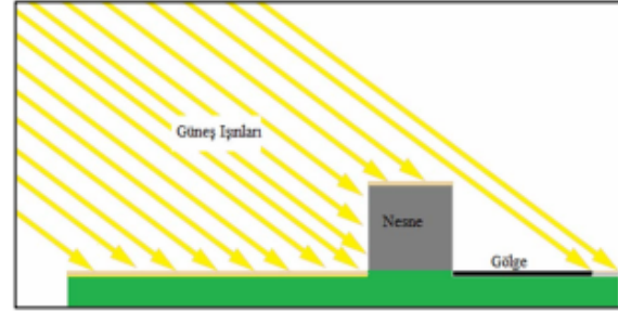
Şekil 2 Gölge Oluşumu
