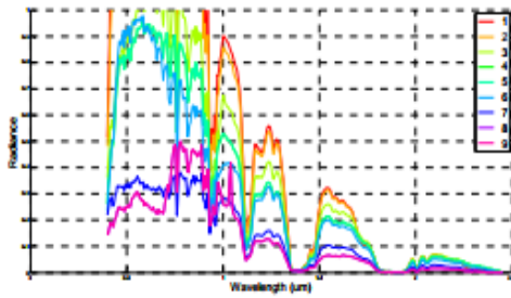
Şekil 6 Seçilen Noktaların Işıma Değerleri
