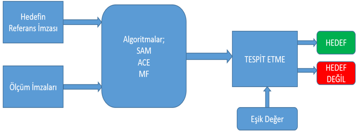
Şekil 45 Hedef Belirleme
