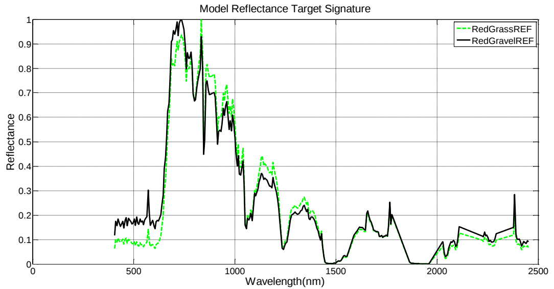
Şekil 41 Çim ve çakıl arkaplanında kırmızı keçe materyalinin gölge düzeltilmiş spektral yansımaları grafiği
