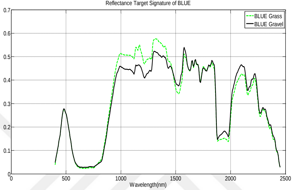
Şekil 38 Ölçüm içi çim ve çakıl arkaplanında mavi keçe materyalinin spektral yansımaya grafiği
