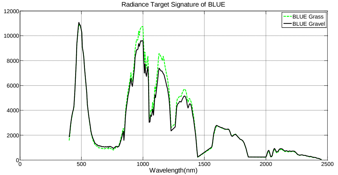
Şekil 37 Ölçüm içi çim ve çakıl arkaplanında mavi keçe materyalinin spektral ışma grafiği
