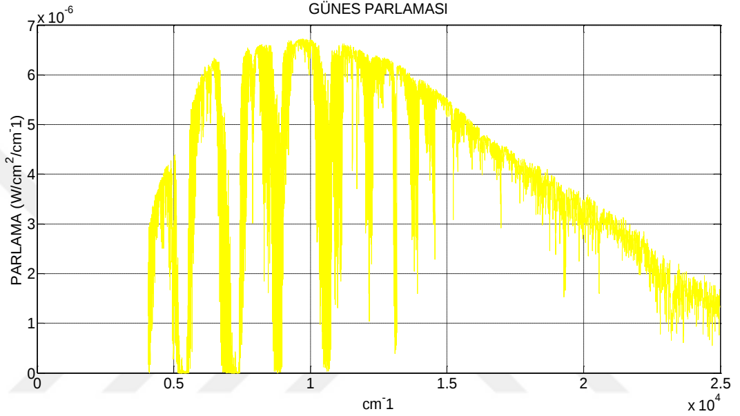
Şekil 32 Dalga numarasına göre güneş parlaması modtran koşum örneği
