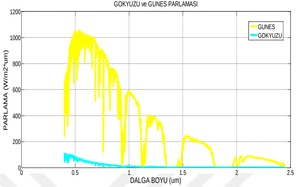
Şekil 34 Dalga boyuna göre gökyüzü ve güneş parlamaşı modtran koşum örneği
