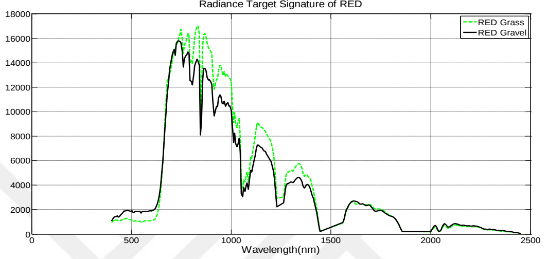
Şekil 36 Ölçüm içi çim ve çakıl arkaplanında kırmızı keçe materyalinin spektral ışma grafiği
