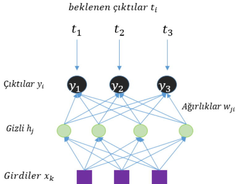
Şekil 2-11: Çapraz entropi maliyet fonsiyonu geri yayılımı
