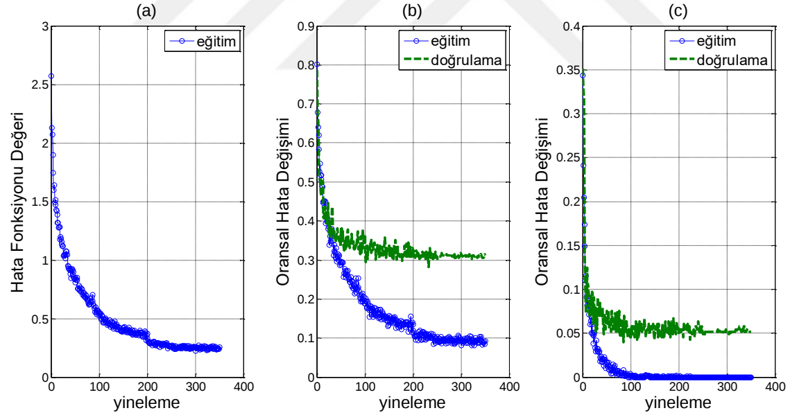
Şekil 6-6: Muufl EMAP_ LiDAR Haritalarına özel DESA Eğitim Grafikleri – a) Kayıp Fonksiyon Değişimi – b) Top-1 Hatalı Sınıflandırma Oranı Değişimini (Toplam Oransal Hata) – c) Top-5 Hatalı Sınıflandırma Oranı Değişimi (Olasılıksal olarak en yüksek 5 değerin doğru sınıfla eşleşmeme durumu) göstermektedir.
