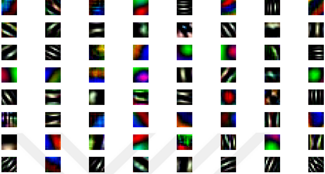
Şekil 4-3: MatConvNet_alexNet İlk Evrişim Katmanının Öğrendiği Filtreler (64 adet) ([37],[45])
