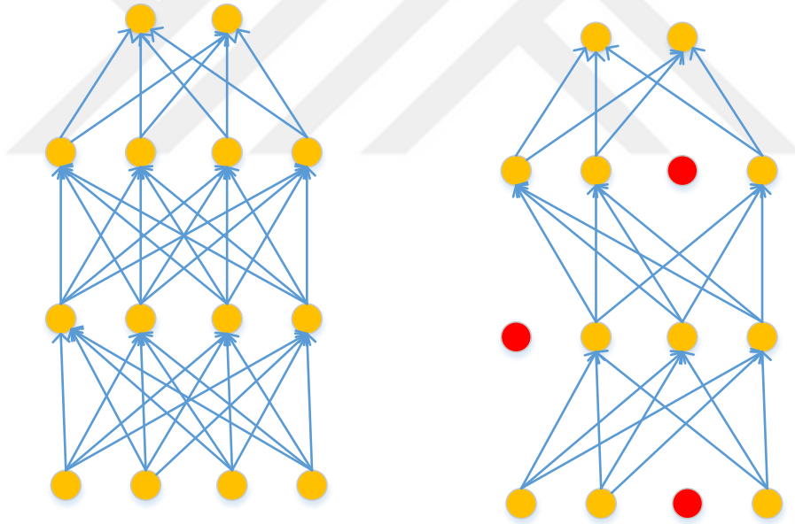
Şekil 2-8: Bırakma katmanı öncesi ve sonrası sinir ağı yapısı
