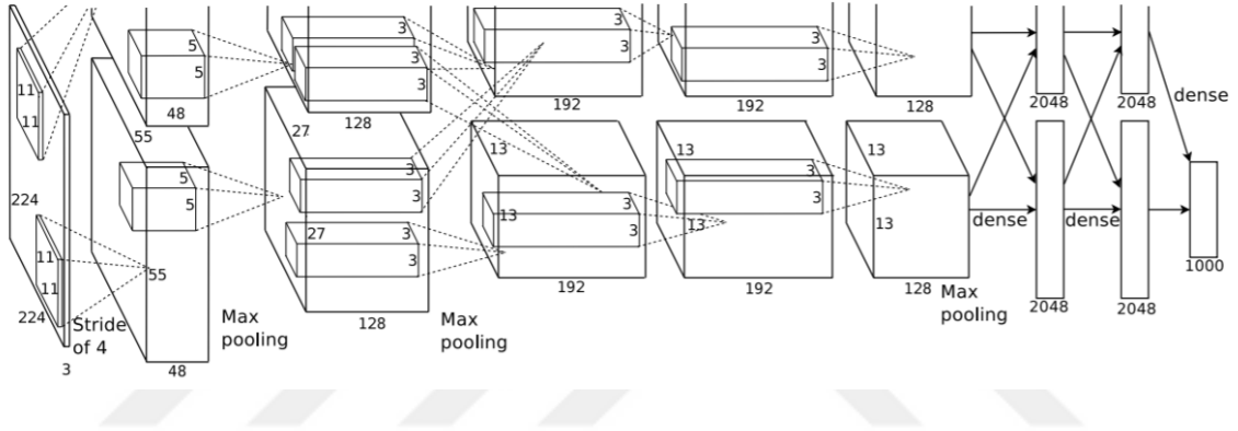
Şekil 2-3: AlexNet DESA Mimarisi [37]
