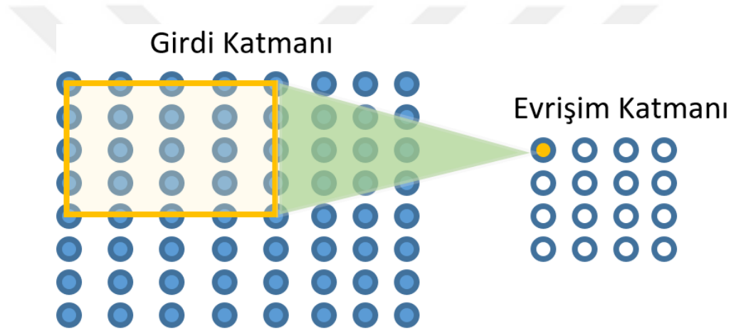
Şekil 2-4: Yerel Alıcı Alan Gösterimi
