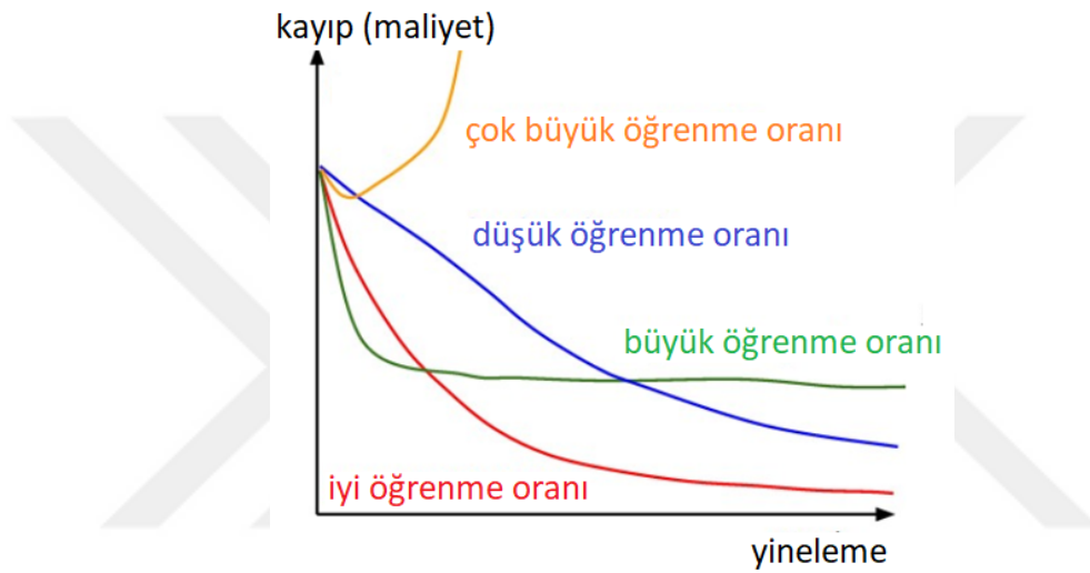
Şekil 2-12: Öğrenme Oranını Maliyet Fonksiyonuna Etkisi
