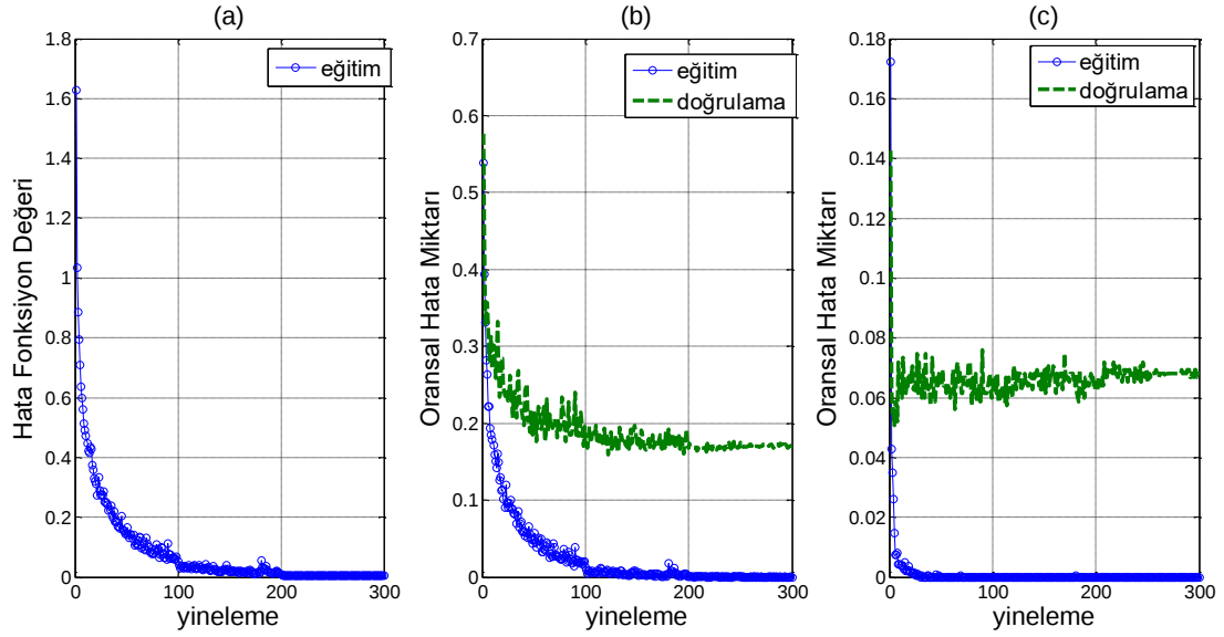
Şekil 6-1: Houston HSG spektral verilerine özel DESA Eğitim Grafikleri –a) Kayıp Fonksiyon Değişimini – b) Top-1 Hatalı Sınıflandırma Oranı Değişimini (Toplam Oransal Hata) – c) Top-5 Hatalı Sınıflandırma Oranı Değişimini (Olasılıksal olarak en yüksek 5 değerin doğru sınıfla eşleşme durumu ) göstermektedir.
