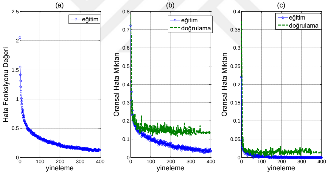
Şekil 6-2: Muufl HSG spektral verilerine özel DESA Eğitim Grafikleri – a) Kayıp Fonksiyon Değişimi –b) Top-1 Hatalı Sınıflandırma Oranı Değişimini (Toplam Oransal Hata) –c) Top-5 Hatalı Sınıflandırma Oranı Değişimini (Olasılıksal olarak en yüksek 5 değerin doğru sınıfla eşleşme durumu ) göstermektedir.
