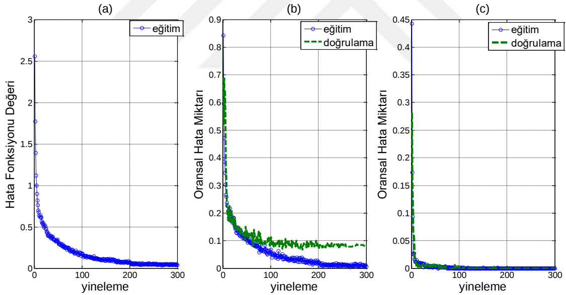
Şekil 6-11: Muufl EMAP_LiDAR ve EMAP_HSG piksel seviyesinde tümleştirilmiş veri kümesine özel DESA Eğitim Grafikleri – a) Hata Fonksiyonu Değişimini – b) Top-1 Hatalı Sınıflandırma Oranı Değişimini (Toplam Oransal Hata) – c) Top-5 Hatalı Sınıflandırma Oranı Değişimini (Olasılıksal olarak en yüksek 5 değerin doğru sınıfla eşleşmeme durumu) göstermektedir.
