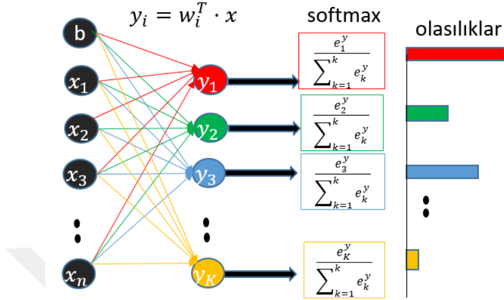
Şekil 2-9: YSA ve softmax fonksiyonu ile çok sınıflı sınıflandırma
