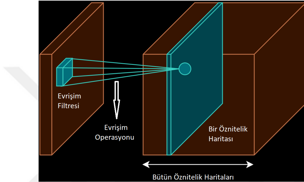
Şekil 2-5: Evrişim Katmanı Operasyonu ve Öznitelik Haritası Oluşumu
