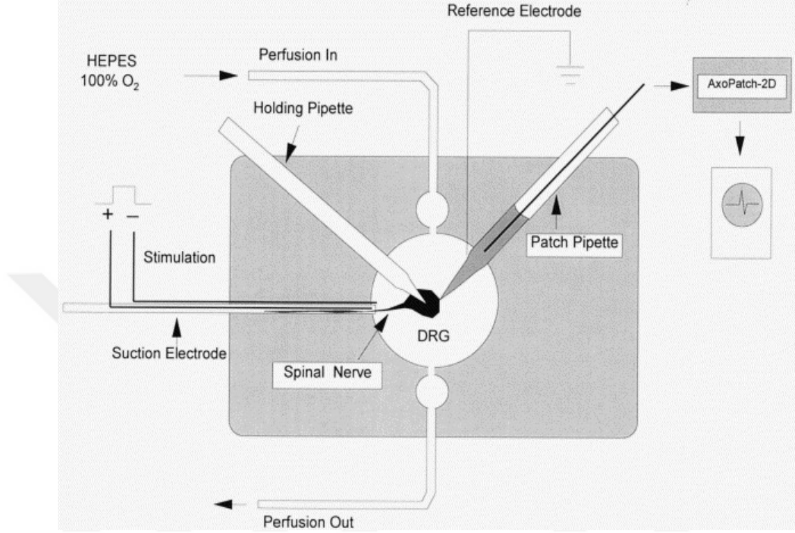
Şekil 1.6. Patch-Clamp deneysel düzeneğinin şematik diyagramı (Zhang, Donnelly, LaMotte, 1998)
