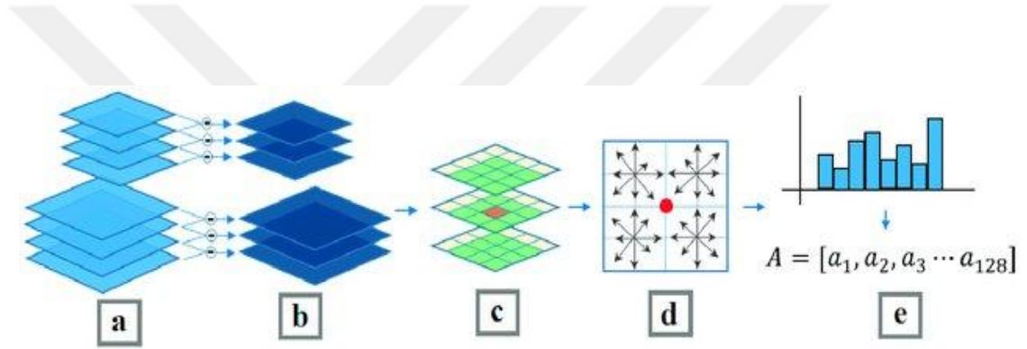
Şekil 4.3. ÖBÖD yönteminin adımları; (a) Ölçek alanı üretimi (b) DoG görüntü üretimi (c) Yerel maksimum ve minimum tespit (d) Gradyan hesaplama (e) Histogram hesabı ve 128 boyutlu vektörlerin üretimi [82]
