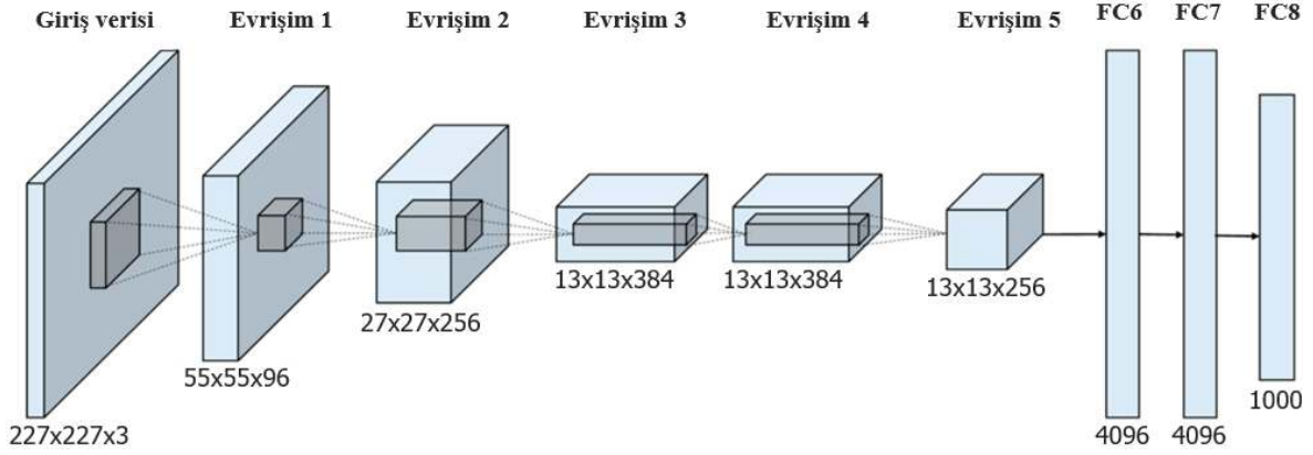
Şekil 3.8. AlexNet ağı [46]
