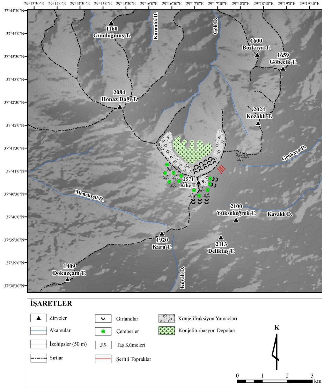
Şekil 23: Honaz Dağının Periglasyal Jeomorfoloji Haritası
