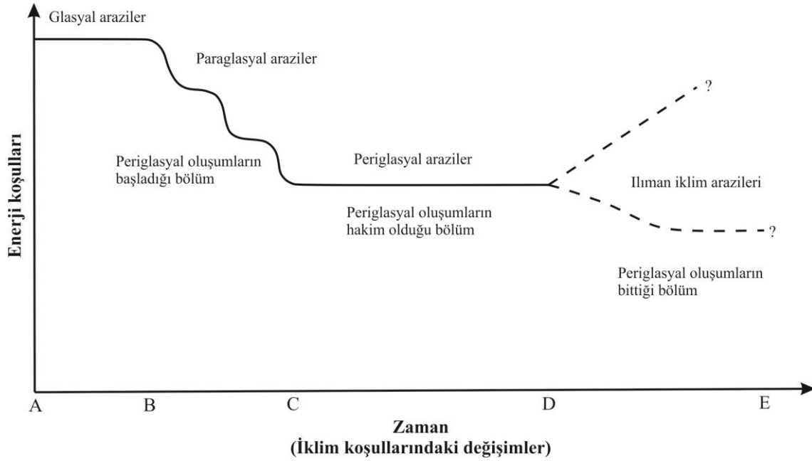
Şekil 3: Farklı Enerji Koşulları Altında Gelişen Glasyal, Periglasyal, Ilıman İklim Arasındaki Geçiş (A-B: Buzullaşma, B-C: Buzul gerilemesi, C-D: Periglasyal Kuşak, D-E: İklim Koşullarındaki Isınma veya Soğuma), (Thorn ve Loewenherz, 1987:59; French, 2007:17’den değiştirilmiştir)
