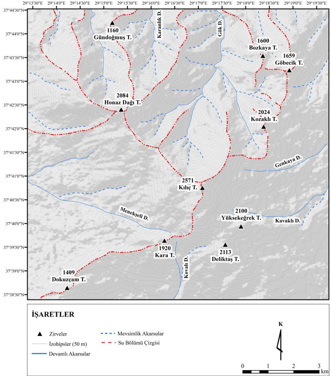
Şekil 12: Honaz Dağı Hidrografya Haritası
