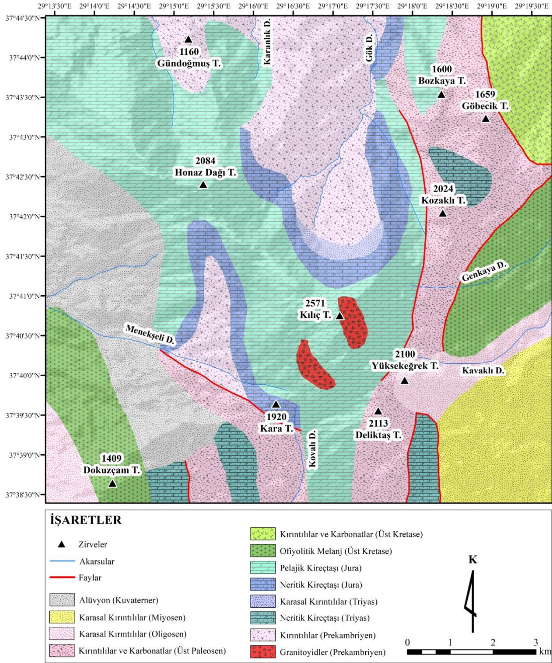
Şekil 10: Honaz Dağı Jeoloji Haritası
