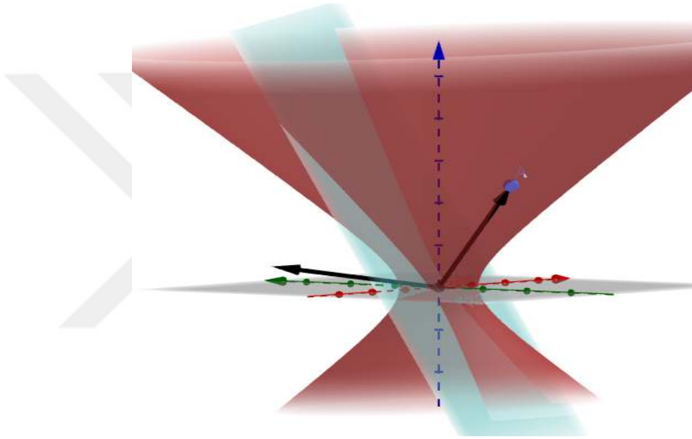
Şekil 2.6. Hiperboloid üzerindeki bir A noktasının orijinden geçen bir düzleme göre yansıması
