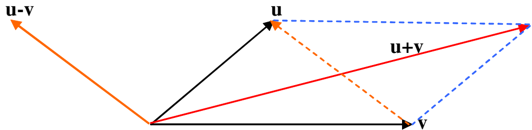
Şekil 2.4. Bir \mathbf{u} vektörünün, Householder dönüşümü ile eş normlu \mathbf{v} vektörüne yansıması
