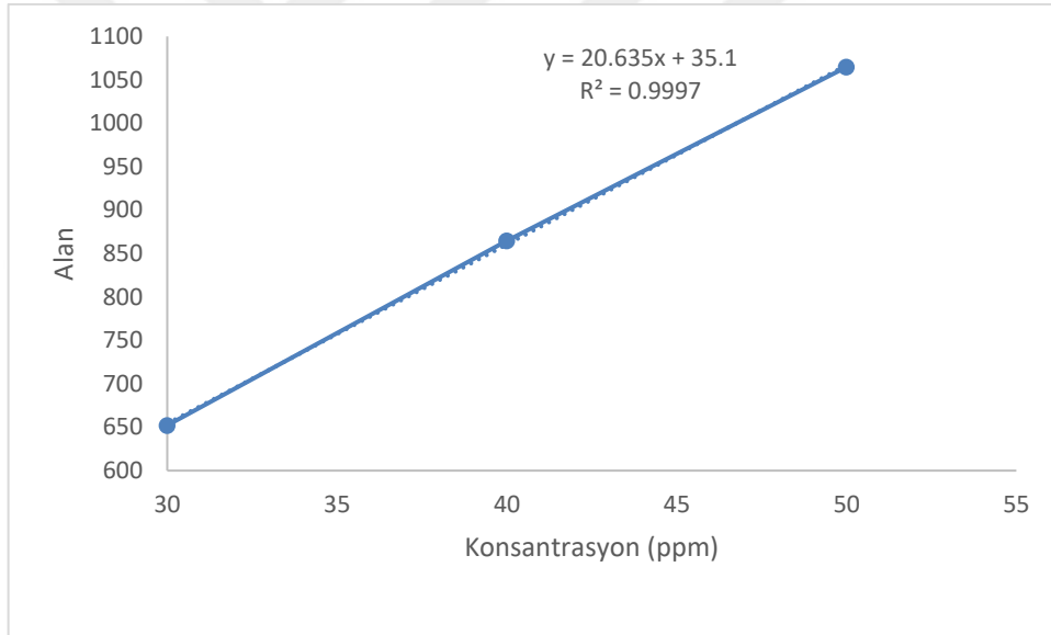
Şekil 4.10. Kersetin standartına ait kalibrasyon eğrisi.
