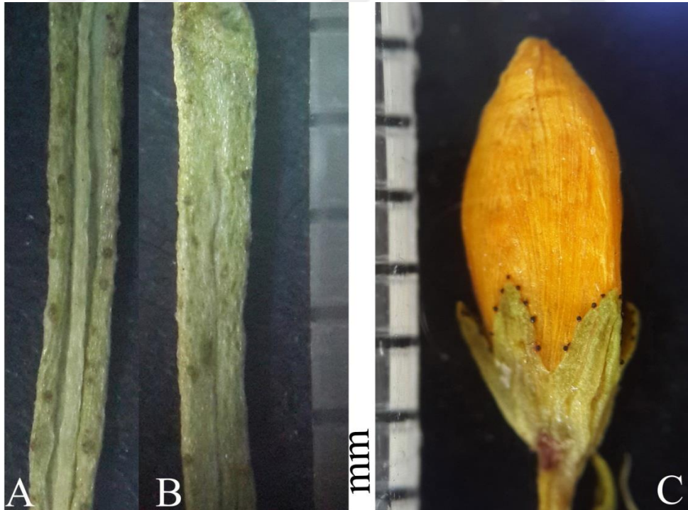
Şekil 4.3. TA 3004 nolu örneğin A: Yaprak alt yüzey, B: Yaprak üst yüzey C: Çiçek (Ölçü: 1 mm).
