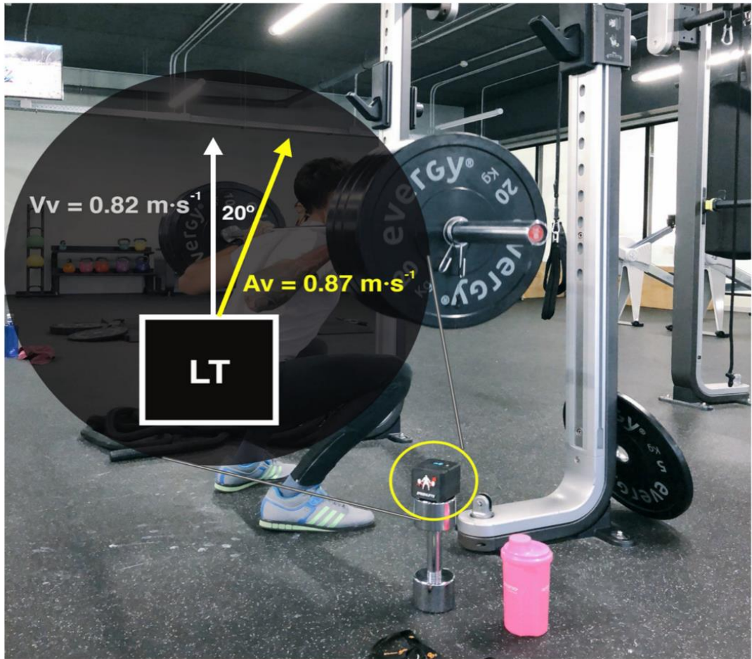
Şekil 2.1. 20° sapmayla yapılan vertikal skuat kaldırışı sırasında, sapmayı hesaba (dikey hız / kosinüs açısı) katmadan yapılan ölçümle 0.82 \text{ m·s}^{-1} hesaba katılarak elde edilen 0.87 \text{ m·s}^{-1} ortalama hız verisi arasında fark vardır.
