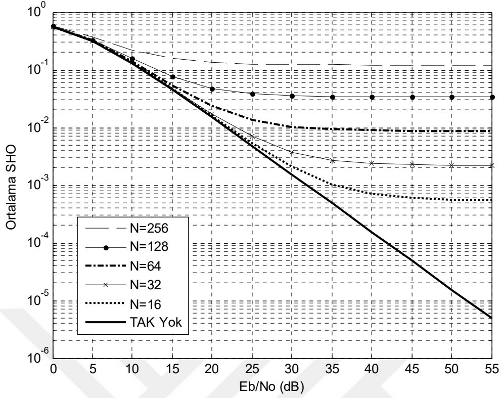
Şekil 3.6 16-DöGM’li klasik DFBC sisteminin varyans kullanılarak hesaplanan SHO başarımı. Gezin hızı 100 km/sa, f_d = 463 Hz.
