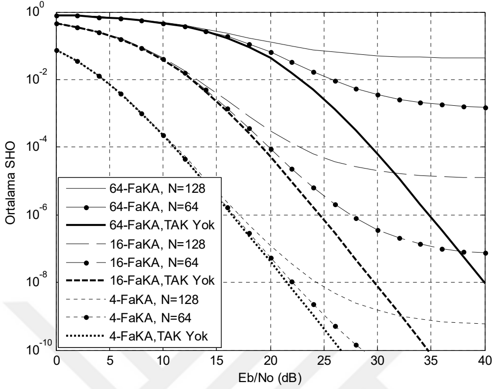
Şekil 4.14 2×2 Alamouti UZBK/DFBC sisteminin hızlı sönmlemeli Nakagami- m kanalda analitik sonuçlarının karşılaştırılması ( m=1, f_d=176 \times 2 Hz).
