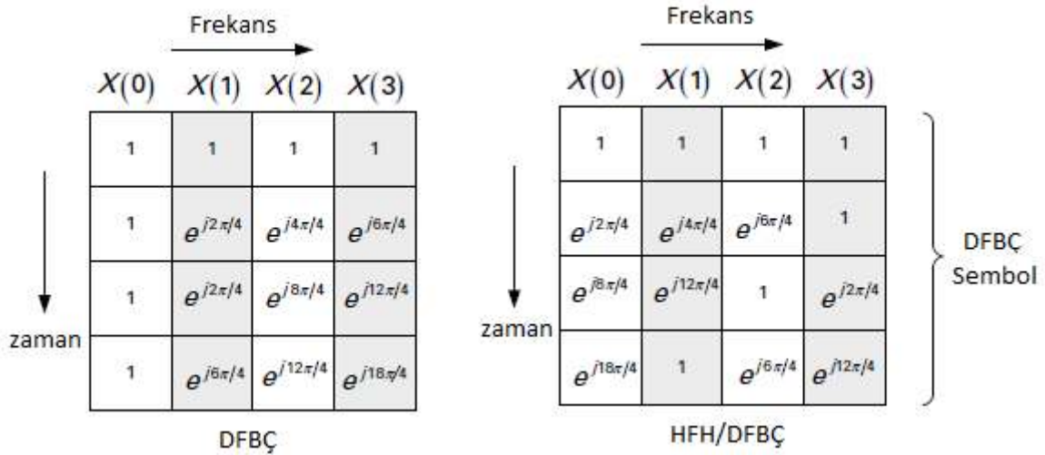
Şekil 5.4 DFBÇ ve HFH/DFBÇ semboller.
