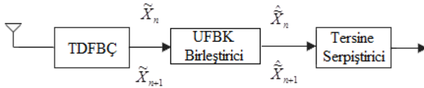
Şekil 4.25 TDFBC'li UFBK alıcı.
