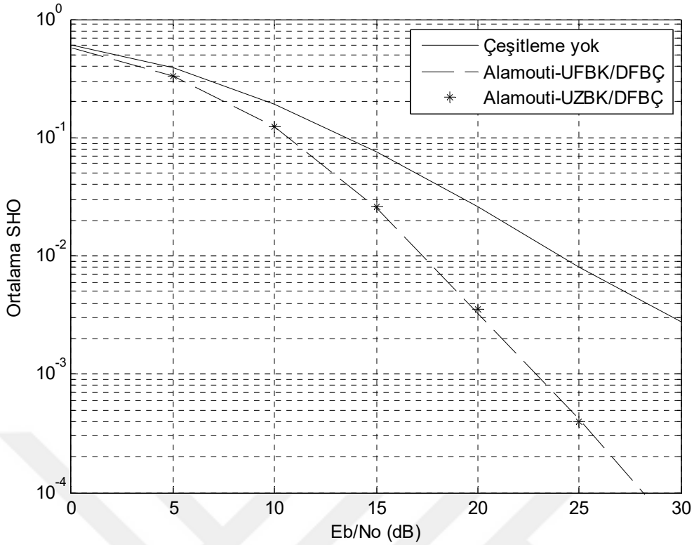
Şekil 4.27 2×1 Alamouti UFBK-UZBK/DFBC sistem için benzetim sonuçları.
