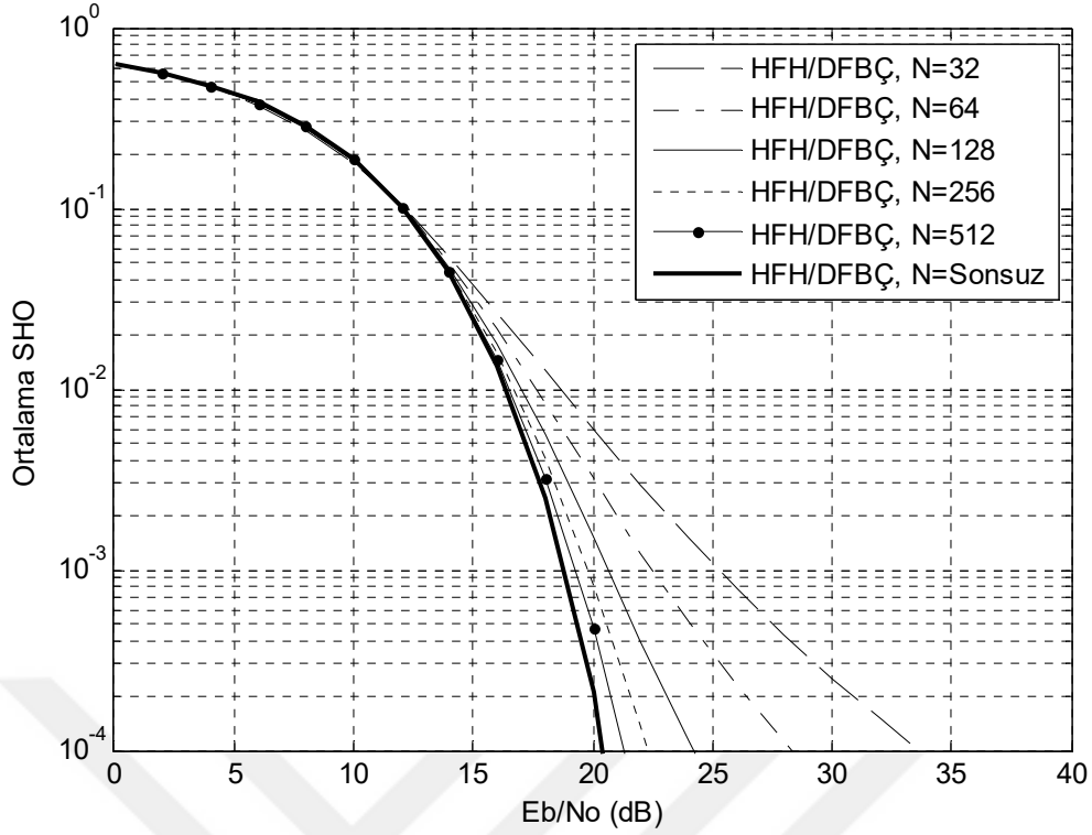
Şekil 6.7 16-DöGM’li HFH/DFBÇ işaretlerin frekans seçici yavaş sönmülemeli Nakagami- m kanalda SHO başarımları, EKOKH denkleştirme, m=1 .
