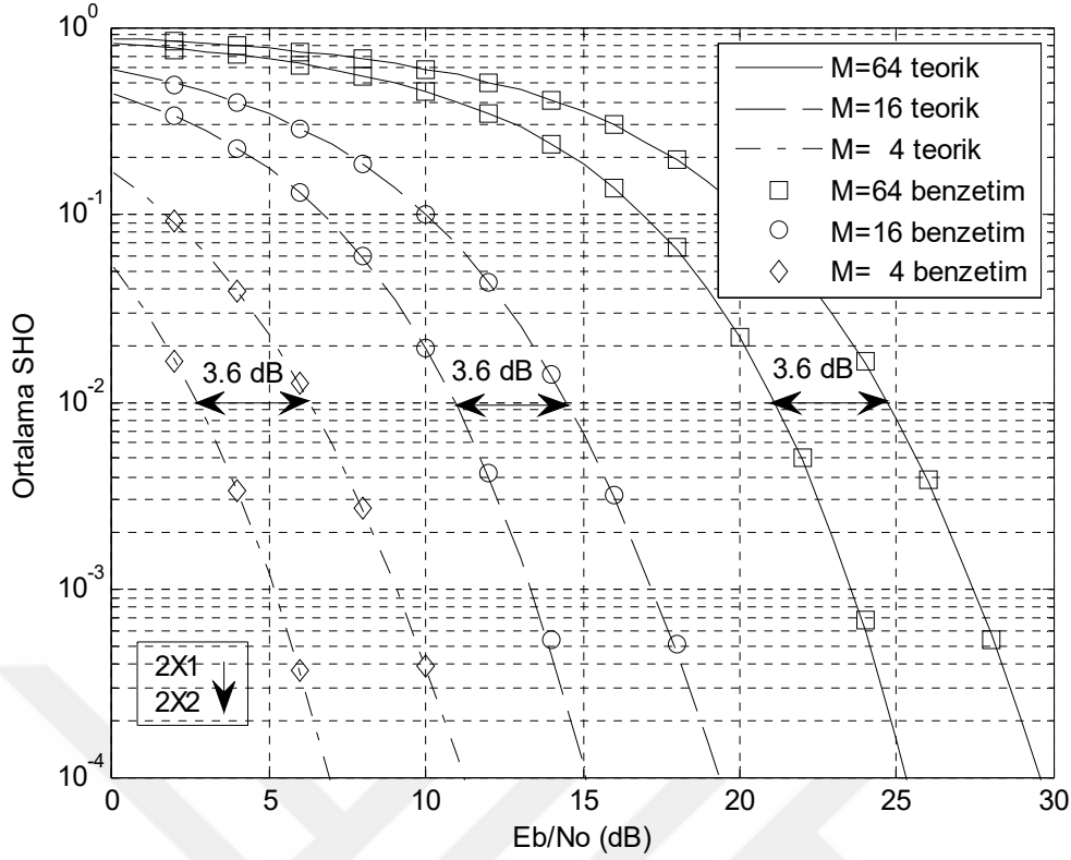
Şekil 4.10 2×1 ve 2×2 Alamouti UZBK/DFBÇ sisteminin yavaş sönmülemeli Nakagami- m kanalda başarımlarının karşılaştırılması ( m=4 , N=64 ).
