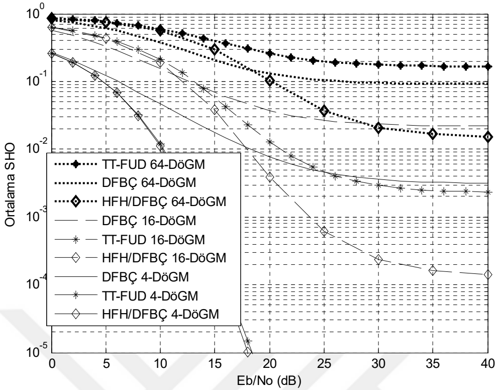
Şekil 7.7 Frekans seçici, hızlı sönmülemeli kanalda, işaretlerin SHO başarımlarının karşılaştırılması, N=128 , f_d=176 \times 2 Hz ( 76 \text{ km/sa} ), m=1 .
