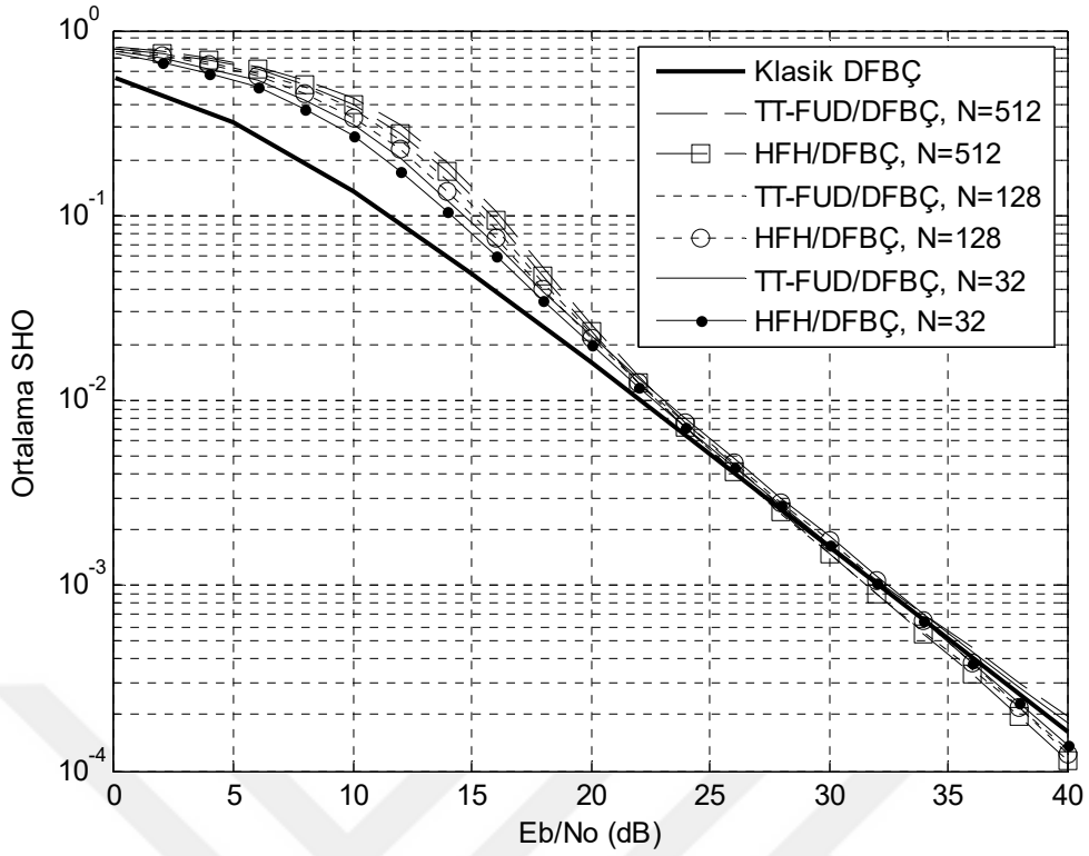
Şekil 6.11 16-DöGM’li işaretlerin frekans seçici yavaş sönmülemeli Nakagami- m kanalda SHO başarımlar karşılaştırması, SZ denkleştirme, m=1 .
