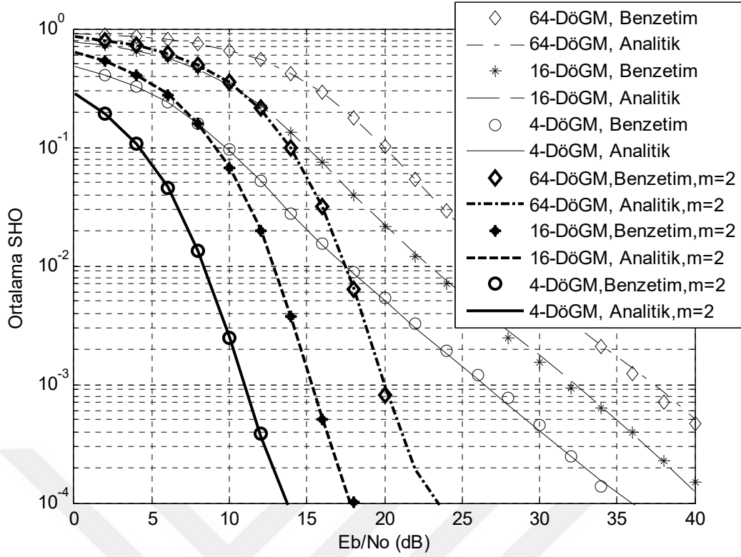
Şekil 6.5 HFH/DFBÇ işaretlerin frekans seçici yavaş sönmlemeli Nakagami- m kanalda SHO başarımları, N=128 , SZ denkleştirme, m=1 , m=2 .
