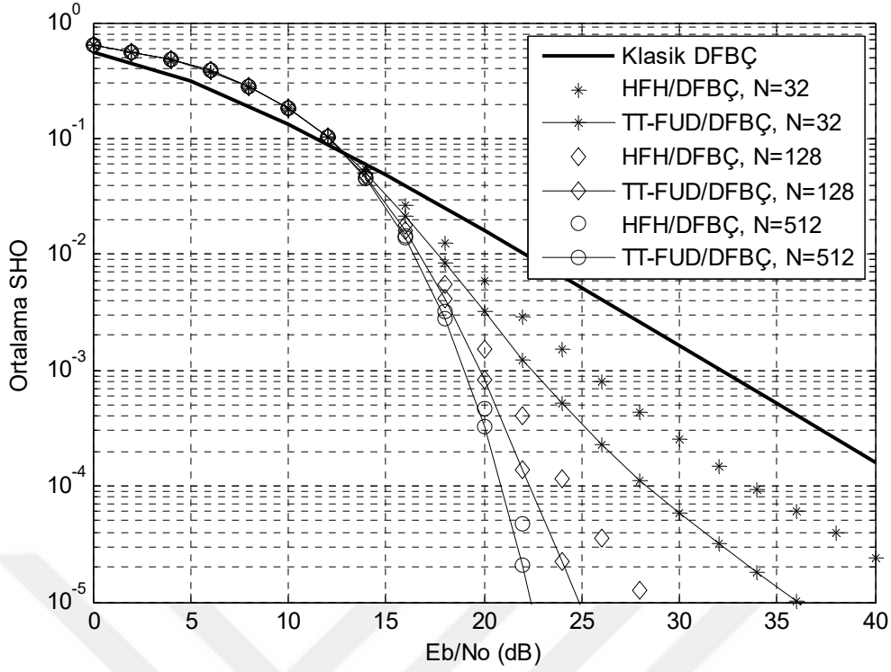
Şekil 6.14 16-DöGM'li işaretlerin frekans seçici yavaş sönümlmeli Nakagami- m kanalda SHO başarımlarını karşılaştırması, EKOKH denkleştirme, m=1 .
