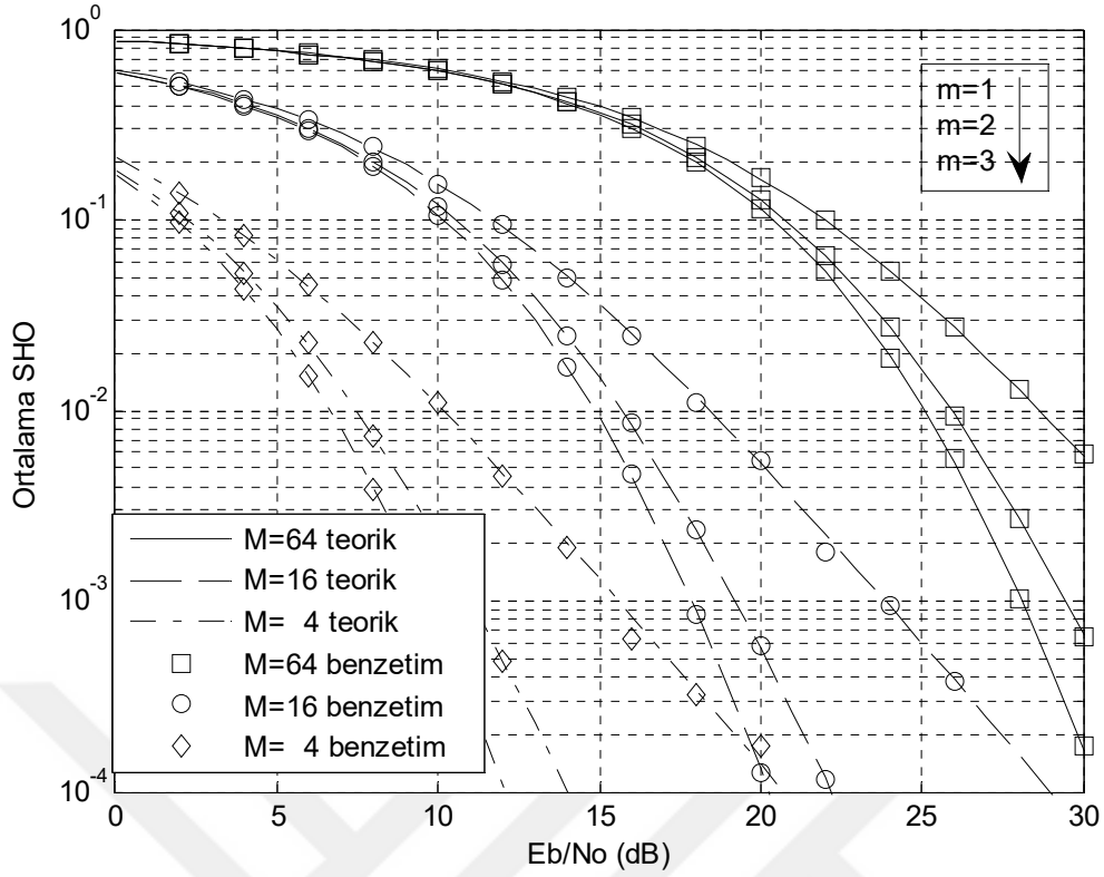
Şekil 4.8 2 \times 1 Alamouti UZBK/DFBC sisteminin yavaş sönmlemeli Nakagami- m kanalda başarımı ( N=64 ).
