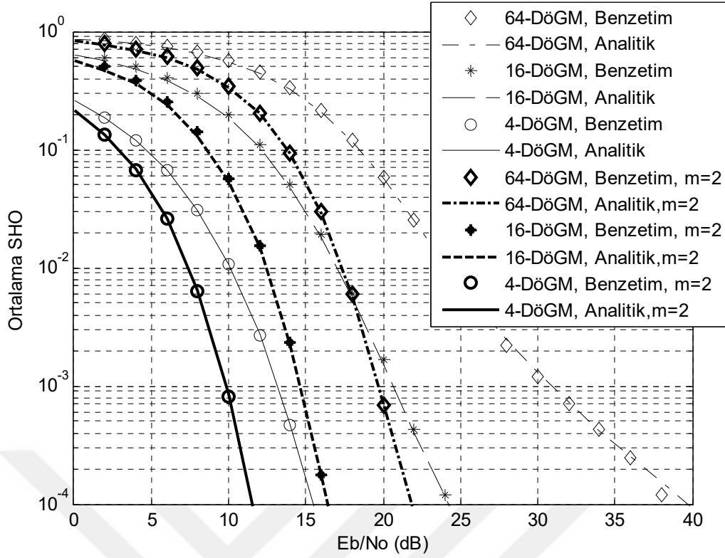
Şekil 6.10 HFH/DFBC işaretlerin frekans seçici yavaş sönmülemeli Nakagami- m kanalda SHO başarımları, N=128 , EKOKH denkleştirme, m=1 , m=2 .
