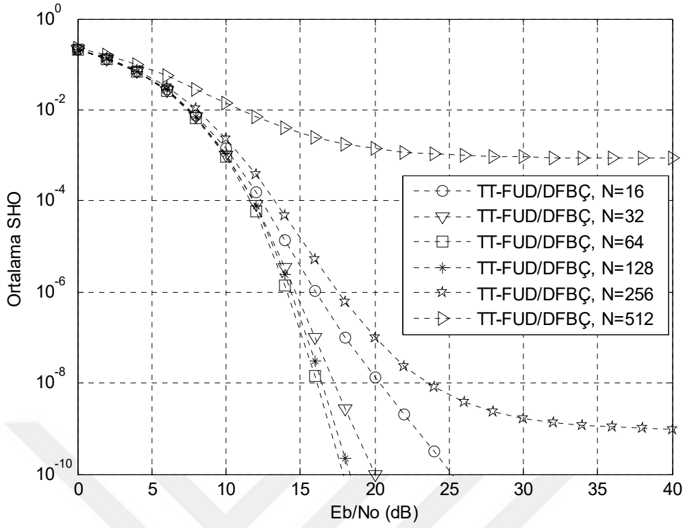
Şekil 7.10 Frekans seçici, hızlı sönmülemeli kanalda, 4-DöGM’li TT/FUD DFBC işaretlerin SHO başarımlarının karşılaştırılması, m=2 .
