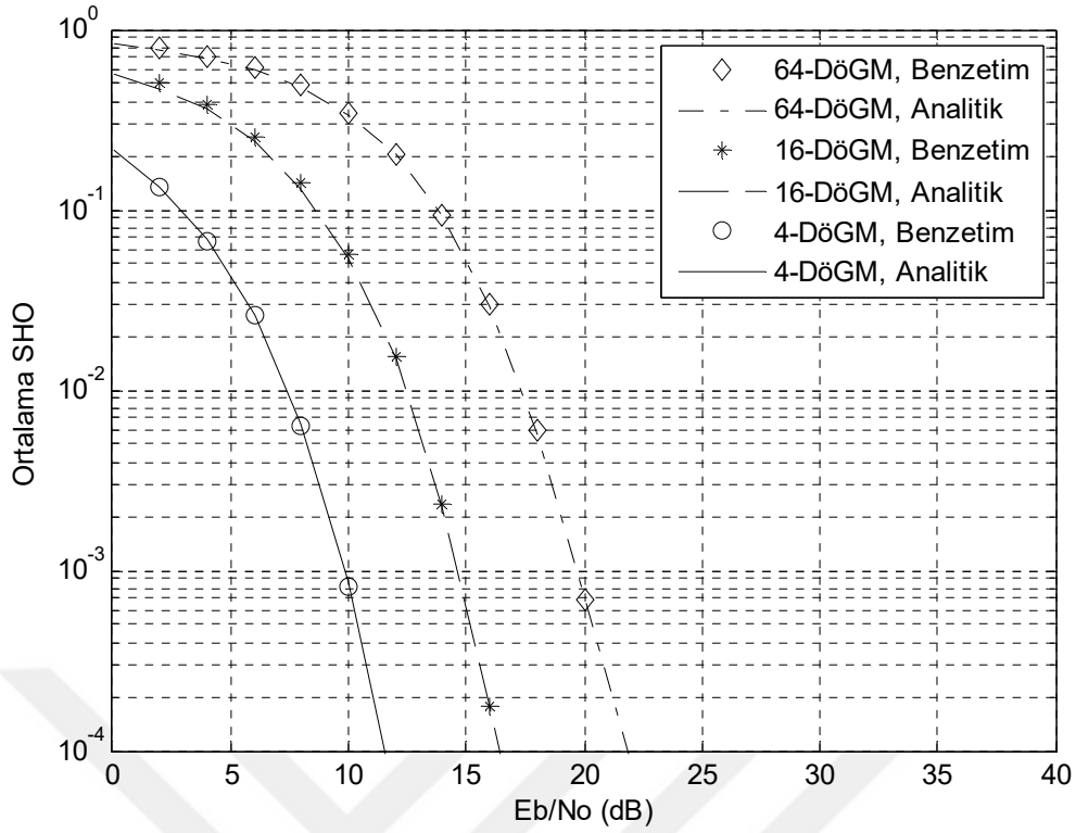
Şekil 6.8 HFH/DFBÇ işaretlerin frekans seçici yavaş sönümlemeli Nakagami- m kanalda SHO başarımları, N=128 , EKOKH denkleştirme, m=2 .
