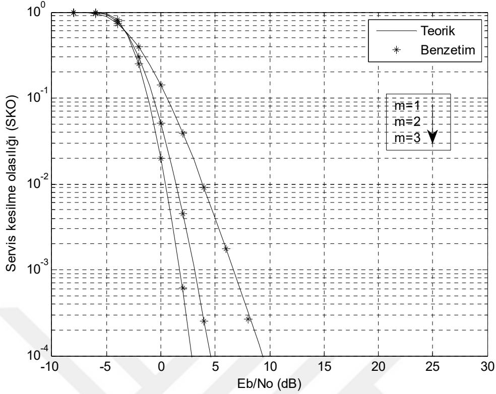
Şekil 4.17 2 \times 2 Alamouti UZBK/DFBC sisteminin yavaş sönmülemeli Nakagami- m kanalda SKO başarımlarının karşılaştırılması ( \gamma_e=0 dB).
