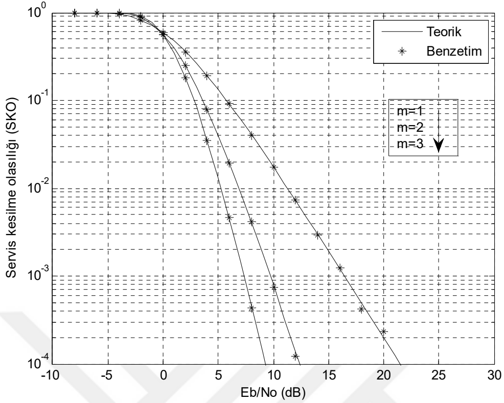
Şekil 4.16 2 \times 1 Alamouti UZBK/DFBC sisteminin yavaş sönmülemeli Nakagami- m kanalda SKO başarımlarının karşılaştırılması ( \gamma_e = 0 dB).
