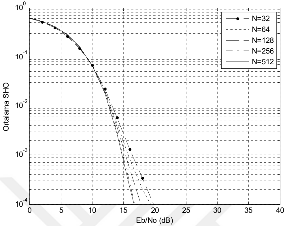
Şekil 6.4 16-DöGM’li HFH/DFBC işaretlerin frekans seçici yavaş sönmülemeli Nakagami- m kanalda SHO başarımları, SZ denkleştirme, m=2 .
