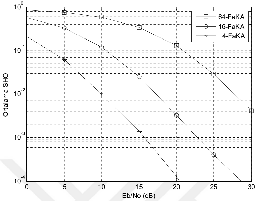
Şekil 4.26 2×1 Alamouti UFBK/DFBC sistem için benzetim sonuçları.
