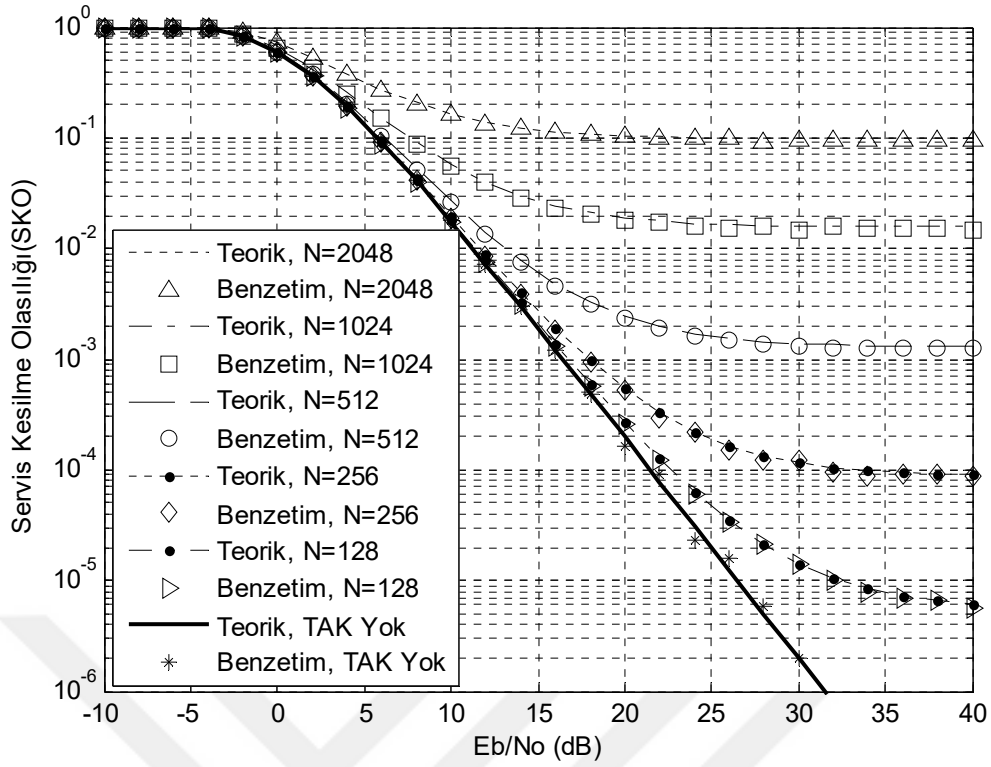
Şekil 4.18 2 \times 1 Alamouti UZBK/DFBÇ sistemlerinin hızlı sönümlmeli Rayleigh kanalda analitik ve benzetim SKO başarımlarının karşılaştırılması ( \gamma_e = 0 dB, f_d = 176 \times 2 Hz).
