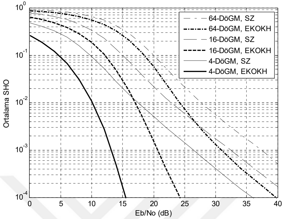
Şekil 6.17 Frekans seçici yavaş sönümlmeli Rayleigh kanalda HFH/DFBÇ'nin SZ ve EKOKH denkleştirme için SHO başarımlar karşılaştırması, ( N=128 ).
