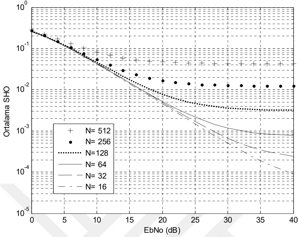
Şekil 7.6 Frekans seçici, hızlı sönmlemeli kanalda, 4-DöGM’li klasik DFBC işaretlerin SHO başarımlarının karşılaştırılması, f_d=176 \times 2 Hz (76 km/sa), m=1 .
