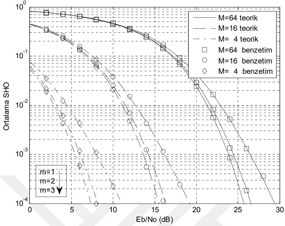
Şekil 4.9 2×2 Alamouti UZBK/DFBC sisteminin yavaş sönmlemeli Nakagami- m kanalda başarımı ( N=64 ).
