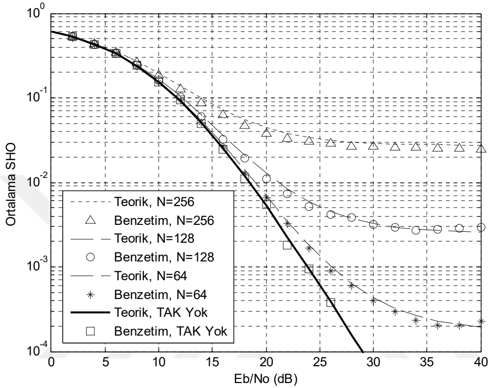
Şekil 4.11 2 \times 1 Alamouti UZBK/DFBÇ sisteminin hızlı sönmlemeli Nakagami- m kanalda 16-FaKA için teorik ve benzetim sonuçlarının karşılaştırılması ( m=1, f_d=176 \times 2 Hz).
