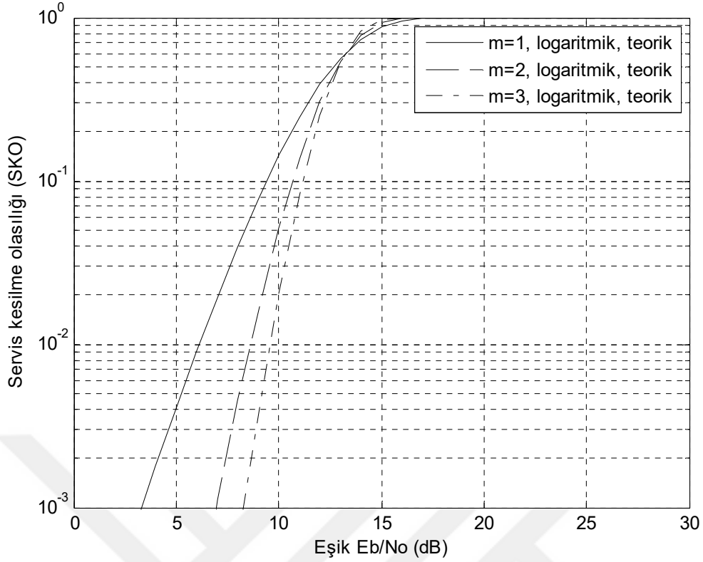
Şekil 4.23 2 \times 2 Alamouti UZBK/DFBC sisteminin yavaş sönmülemeli Nakagami- m kanalda logaritmik ölçekte SKO başarımları ( E_b/N_0 = 10 dB).
