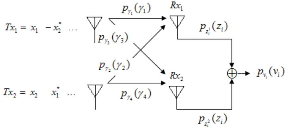
Şekil 4.7 2x2 Alamouti UZBK yapısının olasılık yoğunluk fonksiyonu gösterimi.
