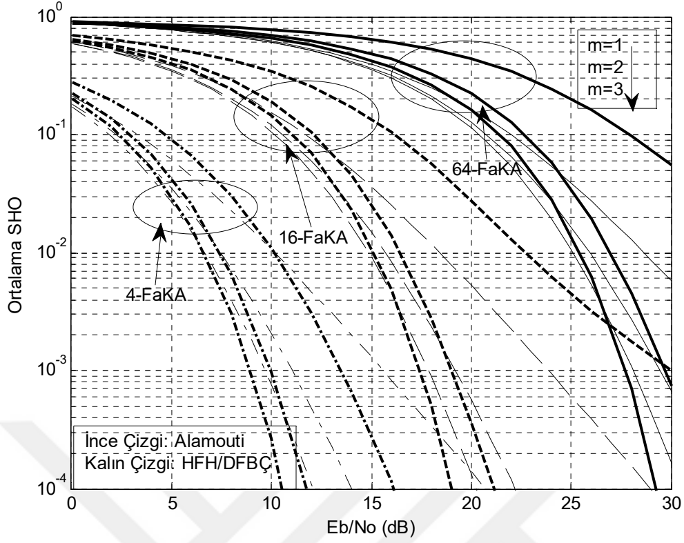
Şekil 6.19 2×1 Alamouti UZBK/DFBC sisteminin HFH/DFBC sistem ile Frekans seçici yavaş sönmlemeli Nakagami- m kanalda başarımı ( N=64 ).
