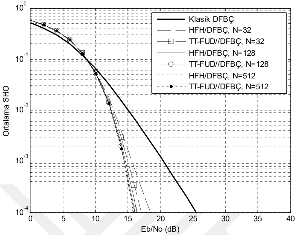
Şekil 6.16 16-DöGM’li işaretlerin frekans seçici yavaş sönmülemeli Nakagami- m kanalda SHO başarımlar karşılaştırması, EKOKH denkleştirme, m=2 .
