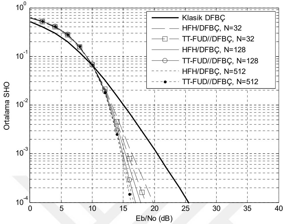
Şekil 6.12 16-DöGM’li işaretlerin frekans seçici yavaş sönümlmeli Nakagami- m kanalda SHO başarımlar karşılaştırması, SZ denkleştirme, m=2 .
