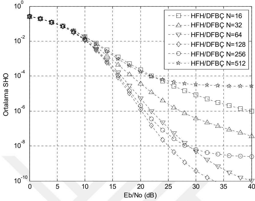
Şekil 7.4 Frekans seçici, hızlı sönmülemeli kanalda, 4-DöGM’li HFH/DFBÇ işaretlerin SHO başarımlarının karşılaştırılması, f_d=176 \times 2 Hz (76 km/sa), m=1 .
