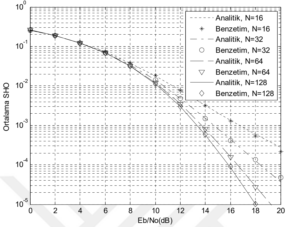
Şekil 7.1 Frekans seçici, hızlı sönmlemeli kanalda, 4-DöGM’li HFH/DFBÇ işaretlerin SHO başarımlarının karşılaştırılması, f_d=176 \times 2 Hz (76 km/sa), m=1 .
