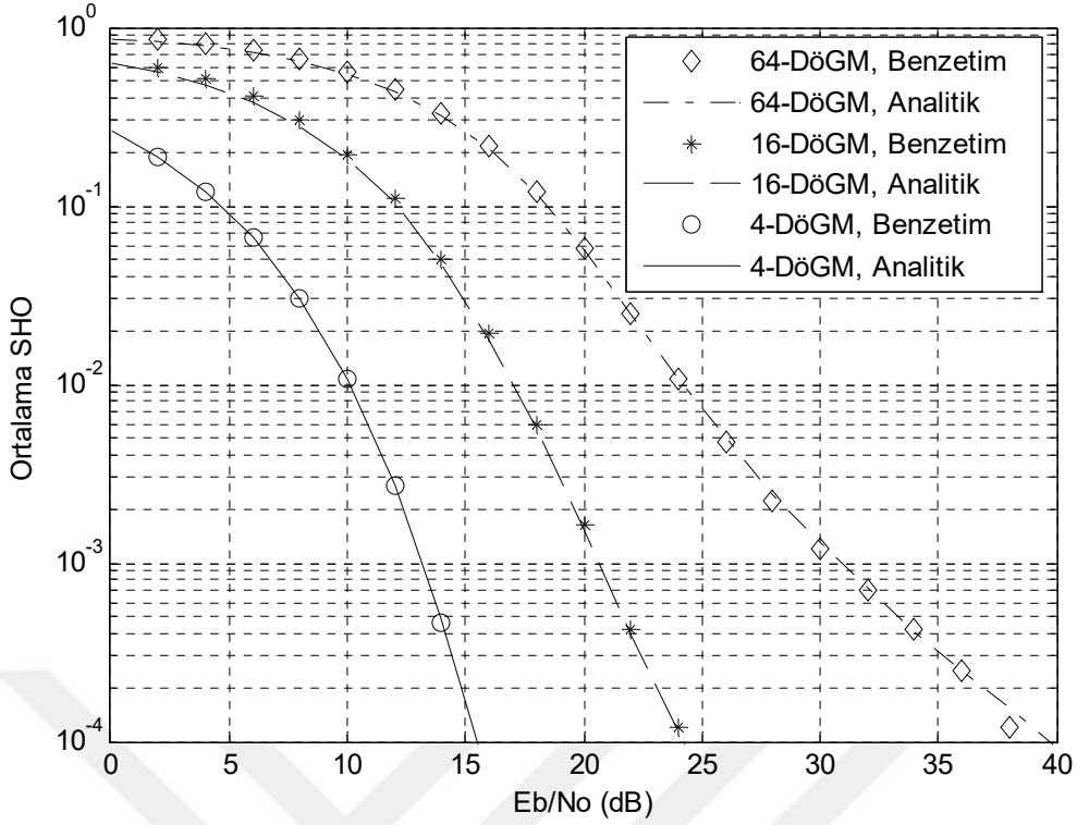
Şekil 6.6 HFH/DFBÇ işaretlerin frekans seçici yavaş sönmülemeli Nakagami- m kanalda SHO başarımları, N=128 , EKOKH denkleştirme, m=1 .
