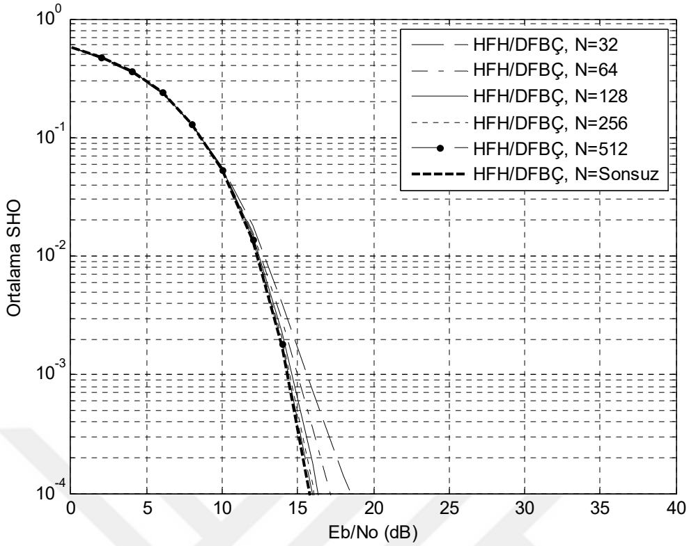
Şekil 6.9 16-DöGM’li HFH/DFBÇ işaretlerin frekans seçici yavaş sönmülemeli Nakagami- m kanalda SHO başarımları, EKOKH denkleştirme, m=2 .
