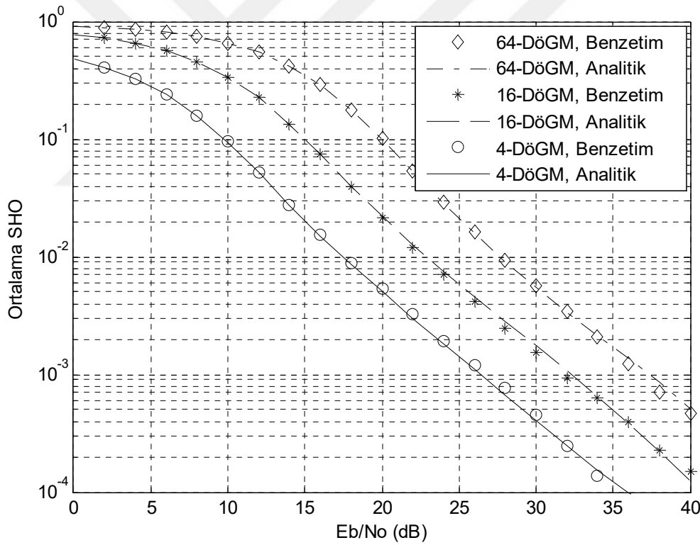
Şekil 6.1 HFH/DFBÇ işaretlerin frekans seçici yavaş sönümlemeli kanalda SHO başarımları, N=128 , SZ denkleştirme, m=1 .
