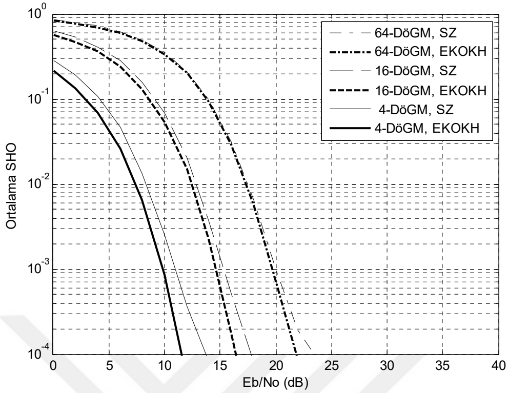
Şekil 6.18 Frekans seçici yavaş sönümlemeli Nakagami- m kanalda HFH/DFBÇ 'nin SZ ve EKOKH denkleştirme için SHO başarımlarını karşılaştırması, ( N=128 , m=2 ).
