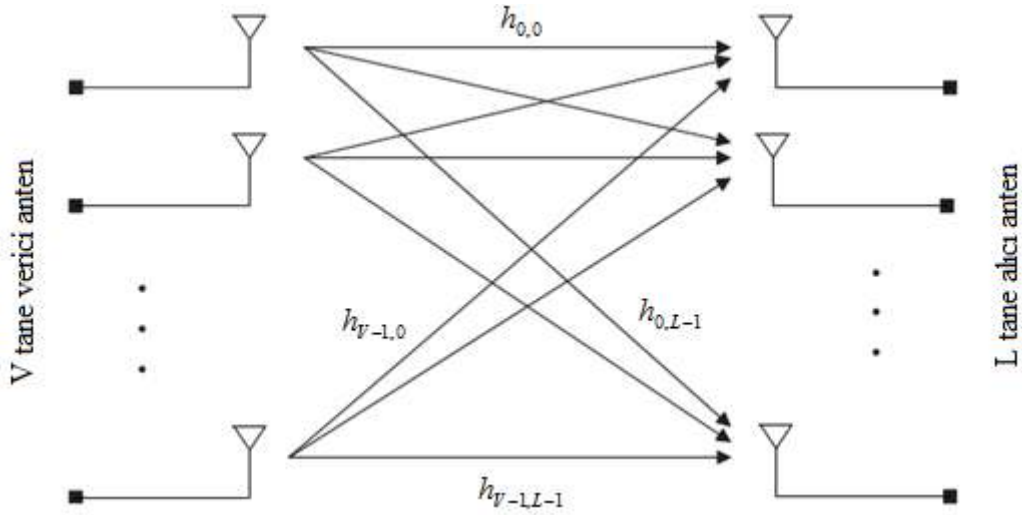
Şekil 4.1 ÇGÇÇ Sistem.
