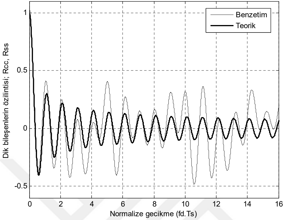
Şekil 2.3 Rayleigh sönümleme sinyalinin dik bileşenlerinin öziliintisi, N = 1024 , T_s = 0.1 \text{ ms} , J=8 sinüsoidal.
