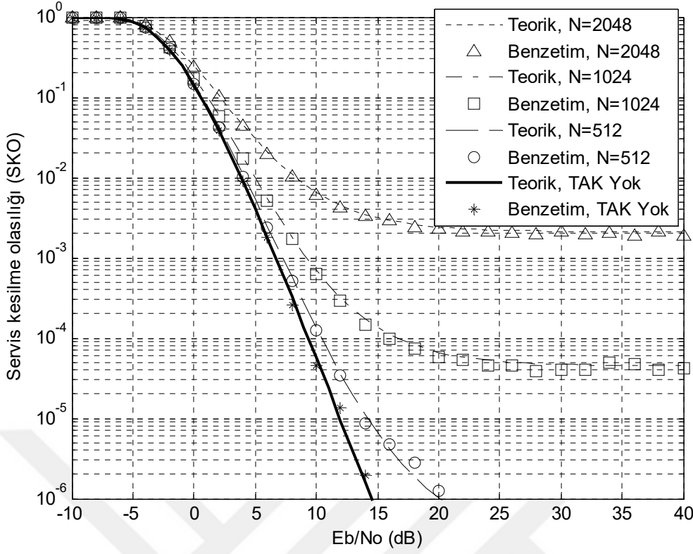
Şekil 4.19 2 \times 2 Alamouti UZBK/DFBÇ sistemlerinin hızlı sönmülemeli Rayleigh kanalda analitik ve benzetim SKO başarımlarının karşılaştırılması ( \gamma_e=0 dB, f_d=176 \times 2 Hz).
