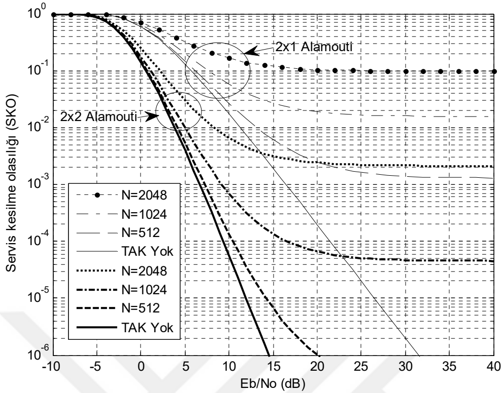
Şekil 4.20 2×1 ve 2×2 Alamouti UZBK/DFBC sistemlerinin hızlı sönümlmeli Rayleigh kanalda analitik SKO başarımlarının karşılaştırılması ( \gamma_e=0 dB, f_d=176\times 2 Hz).
