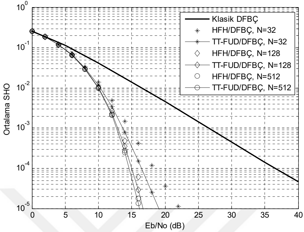
Şekil 6.15 4-DöGM’li işaretlerin frekans seçici yavaş sönümlmeli Nakagami- m kanalda SHO başarımlar karşılaştırması, EKOKH denkleştirme, m=1 .
