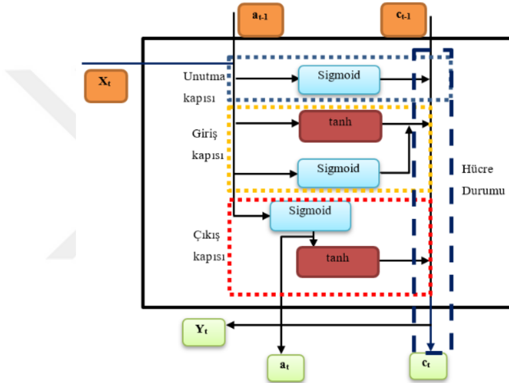
Şekil 3.19. LSTM hücre yapısı.
