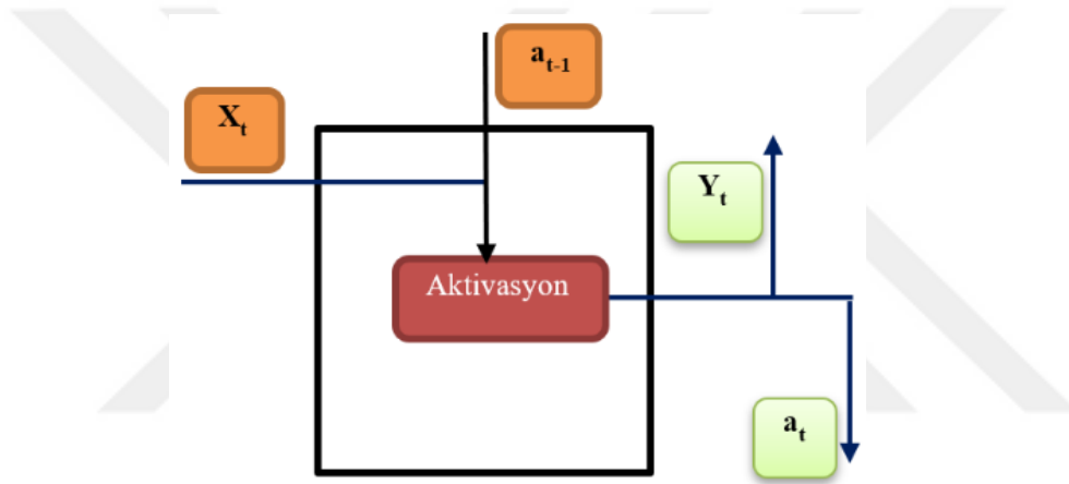
Şekil 3.17. RNN hücre yapısı
