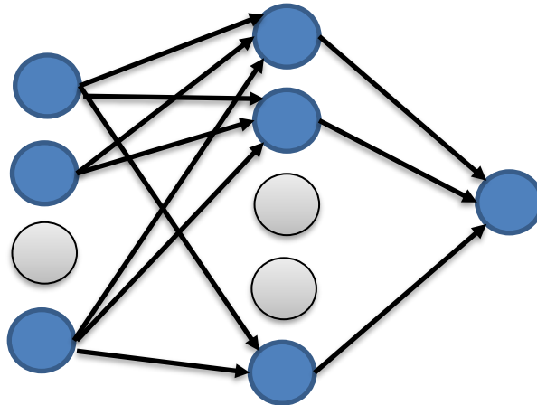
Şekil 3.5. Nöron seyreltme.
