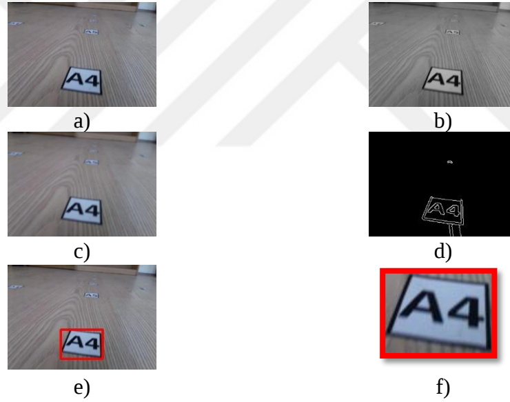
Şekil 3.21. Görüntü işleme adımları. a) Alınan görüntü, b) Grileşme, c) Bulanıklık, d) Otsu ve Canny, e) İşaret tespiti, f) Kırpılmış işaretçi görüntüsü.
