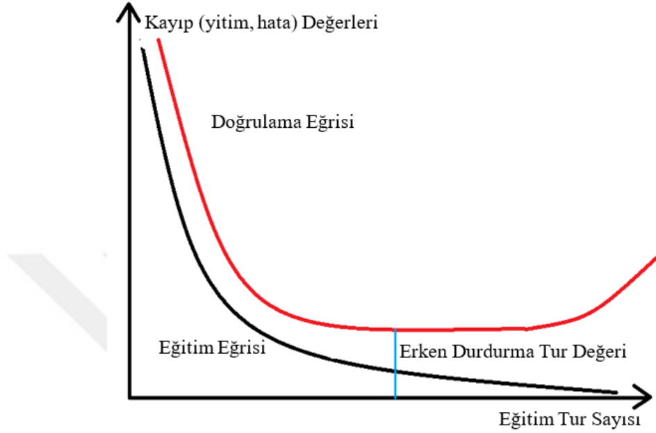
Şekil 3.6. Erken durdurmanın belirlenmesi.
