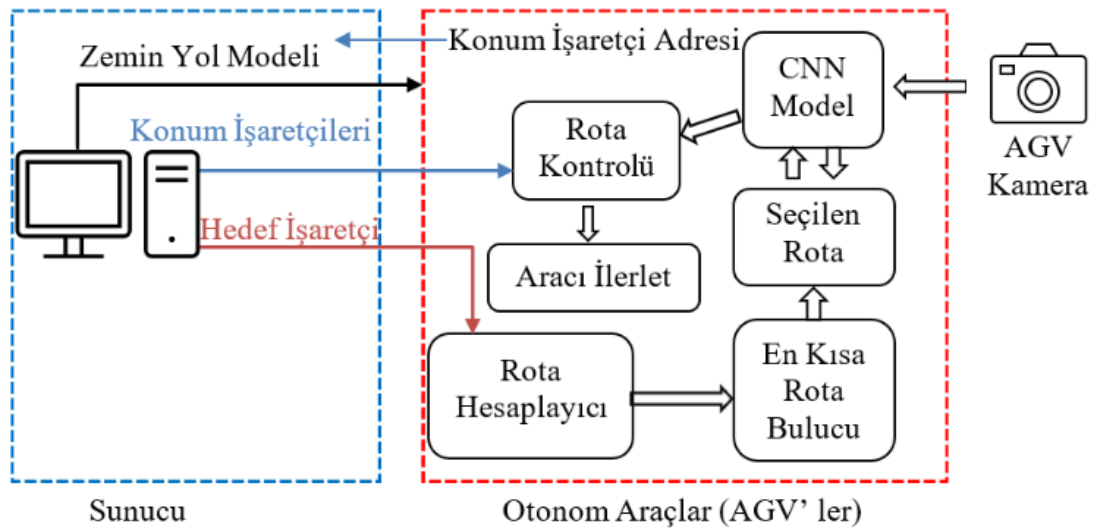
Şekil 3.25. Sistemin blok şeması.
