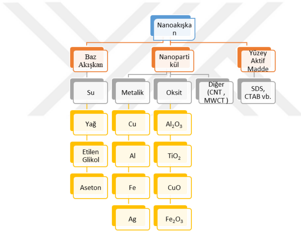
Şekil 3.1. Nanoakışkanın sentezlenmesi için yaygın baz akışkanlar, nanopartiküller ve yüzey aktif cisimleri
