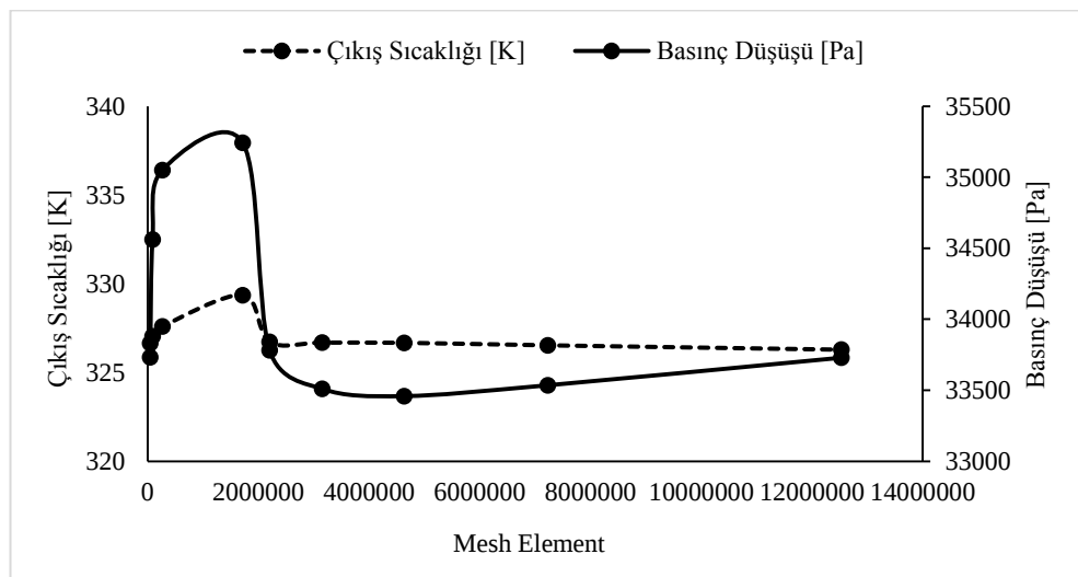
Şekil 4.4. MK(ST) \text{Al}_2\text{O}_3 Çözüm ağı bağımsızlığı
