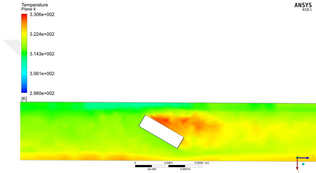
Şekil 5. 2 MK(ST) Al_2O_3 HAD Analizi; Kanatçık çevresinde sıcaklık bölgeleri
