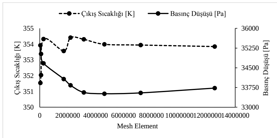
Şekil 4.14. MK(SA) Al 2 O 3 Çözüm ağı bağımsızlığı
