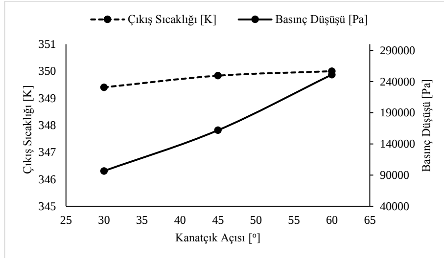
Şekil 4.5. Kanatçık açısının sonuçlara etkisi
