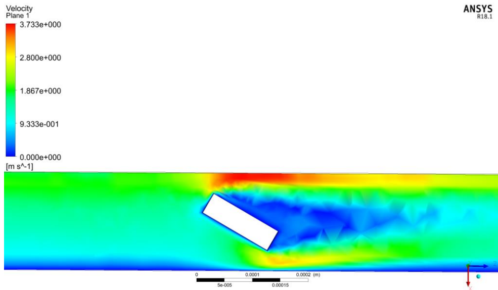
Şekil 5.1. MK(ST) Al 2 O 3 HAD Analizi; Hız bölgeleri
