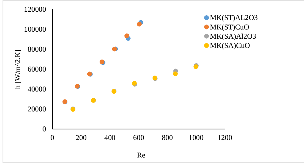
Şekil 5.11. Reynolds sayısının ısı taşınım katsayısına etkisi
