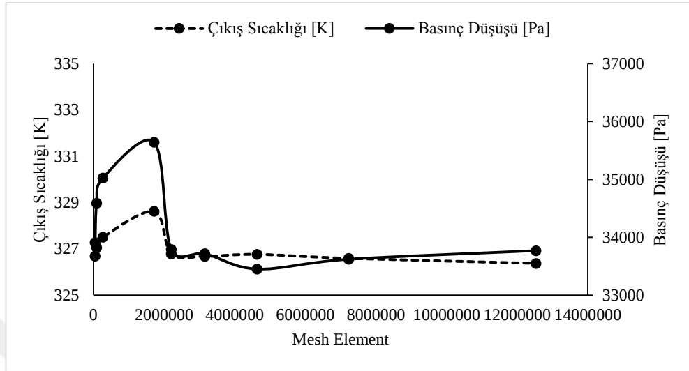
Şekil 4.9. MK(ST) CuO Çözüm ağı bağımsızlığı
