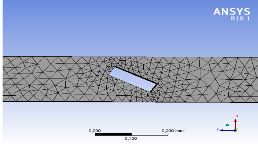
Şekil 4.3. \text{Al}_2\text{O}_3 Nanoakışkan Sabit Sıcaklıkta Çözüm Ağı
