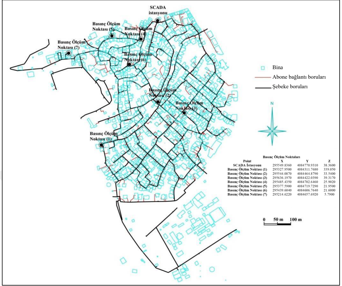
Şekil 3.1. Çalışma sahasında basınç ölçüm noktalarının konumları (Not: Z: Basınç ölçüm noktasının kotu, koordinatlar UTM cinsindendir) (Muhammetoğlu 2017’den alınmıştır)
