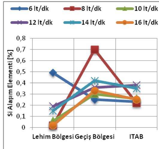
Şekil 6.67. Alın birleştirmedeki farklı gaz debilerinde birleştirilen galvanizli 1315 IF sacının Cu, Al ve Si alaşımlarının bölgelere göre dağılımı
