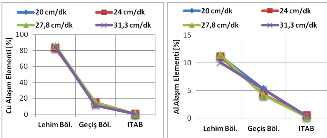
Şekil 6.149. Bindirme birleştirmedeki farklı lehim ilerleme hızlarında birleştirilen galvanizsiz 7116 IF sacının Cu ve Al alaşım elementlerinin bölgelere göre dağılımları
