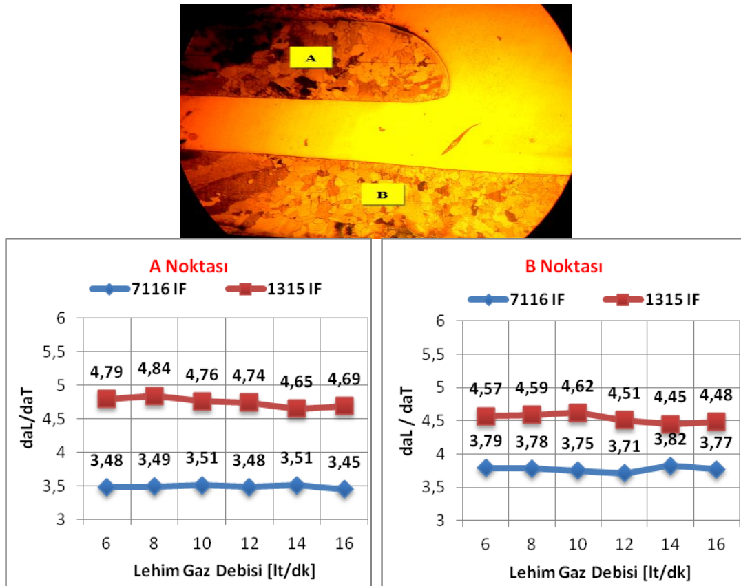
Şekil 6.134. Bindirme birleştirmedeki farklı gaz debilerinde birleştirilen IF saclarının ITAB bölgesindeki tanelerinin d_{\alpha L}/d_{\alpha T} oranı
