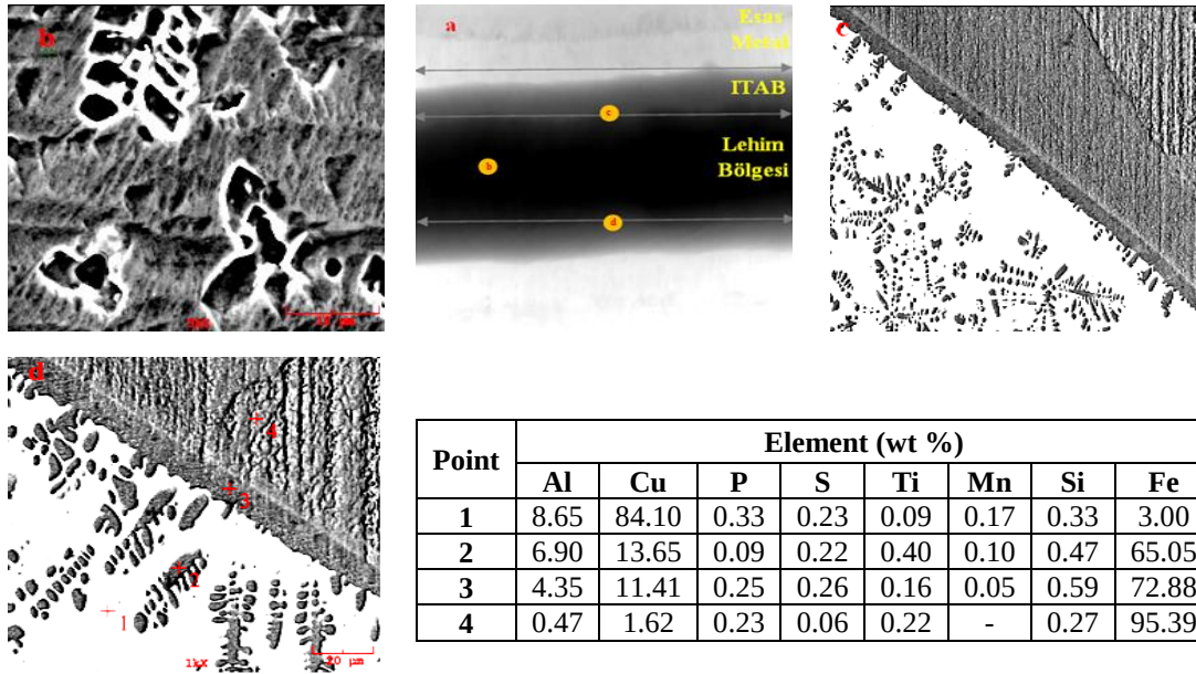
Şekil 6.51. Alın altına geometride birleştirilen galvanizli 1315 IF sacın 55 A akım şiddetindeki (a: Bilgisayarlı X-Ray tomografisi, b: Lehim bölgesi SEM görüntüsü, c: Lehim-ITAB bölgesi SEM görüntüsü, d: Lehim-ITAB bölgesi EDS analizi)
