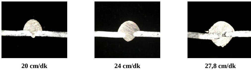
Şekil 6.33. Galvanizli 1315 IF sacının farklı lehim ilerleme hızları uygulanarak birleştirilen makro görüntüleri
