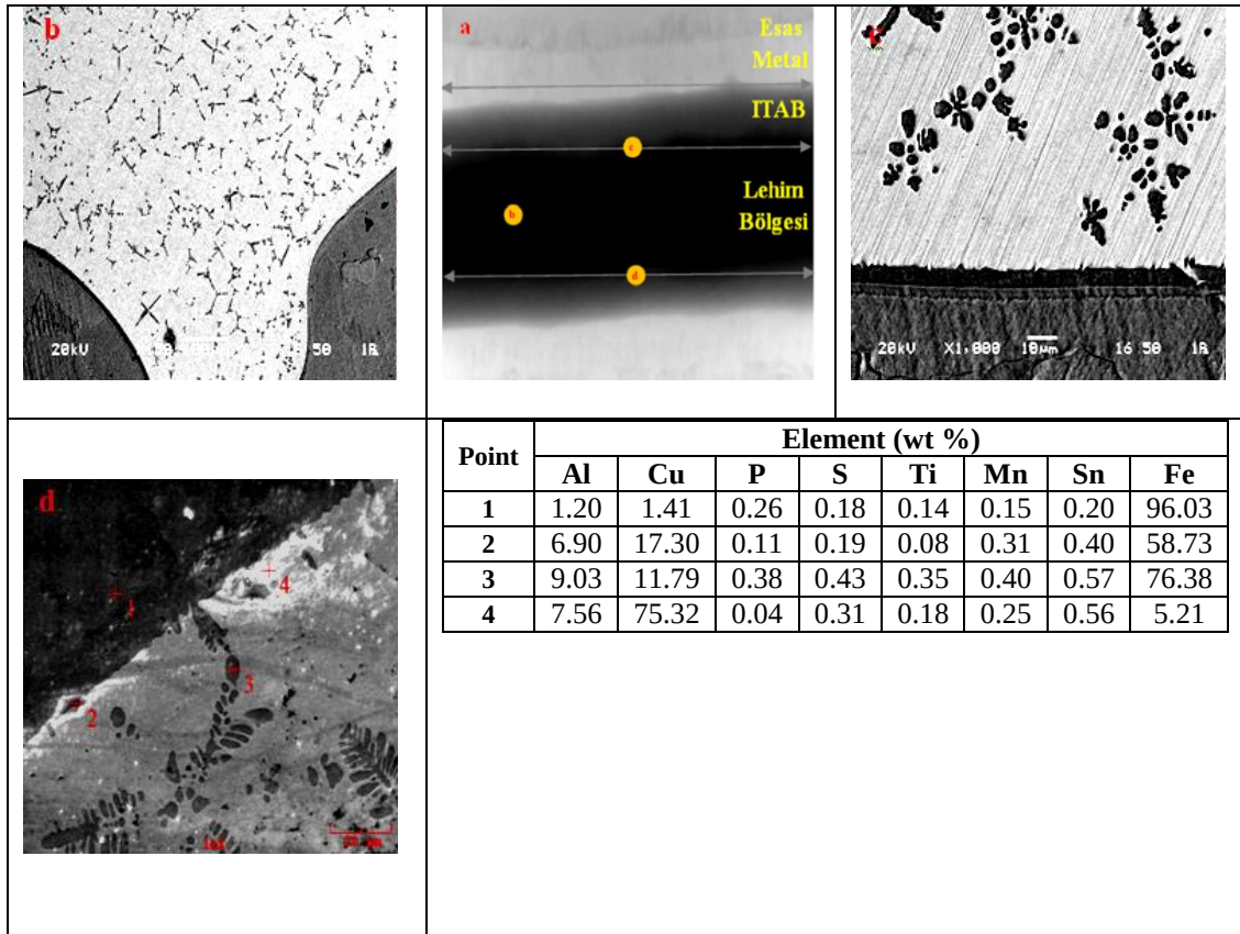
Şekil 6.47. Alın altına geometride birleştirilen galvanizsiz 7116 IF sacın 60 A akım şiddetindeki (a: Bilgisayarlı X-Ray tomografisi, b-c: Lehim-ITAB bölgesi SEM görüntüsü, d: Lehim-ITAB bölgesi EDS analizi)
