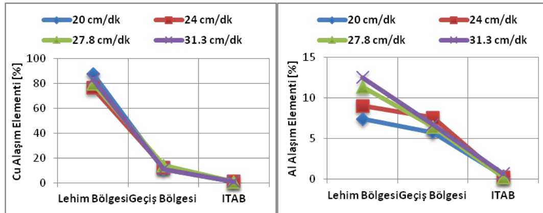
Şekil 6.79. Alın birleştirmedeki Farklı lehim ilerleme hızlarında birleştirilen galvanizsiz 7116 IF sacının Cu ve Al alışımının bölgelere göre dağılımları
