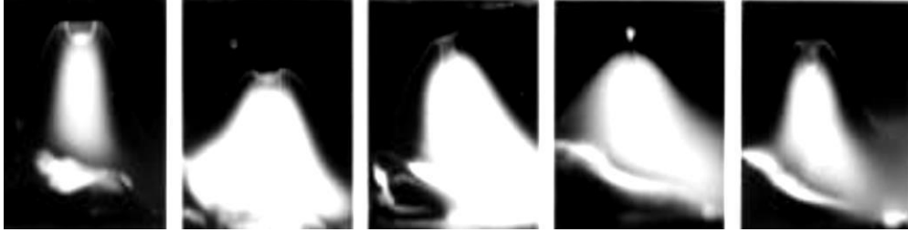
Şekil 4.9. Darbeli ark yönteminde elektrodun erimesi
