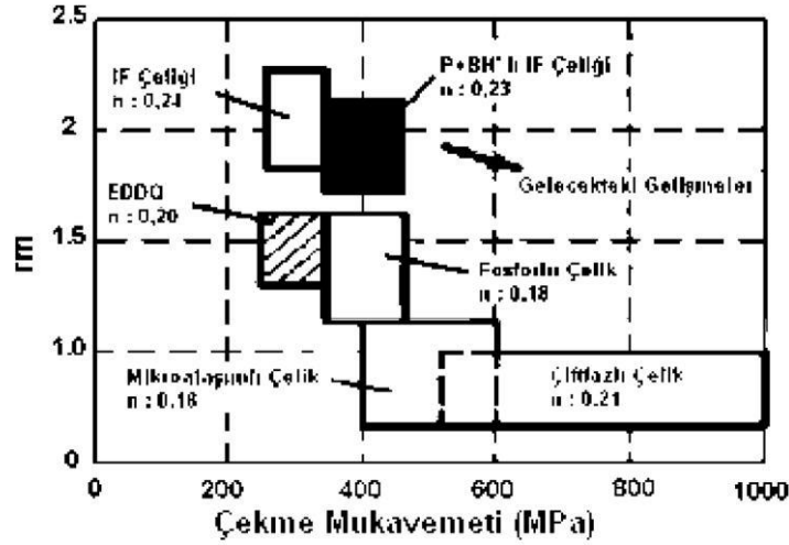
Şekil 3.2. Çeşitli sac çeliklerinin çekme mukavemeti ve anizotropi (r m ) katsayısı arasındaki ilişki [55]
