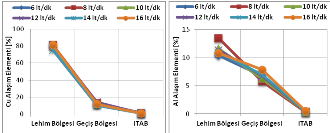
Şekil 6.64. Alın birleştirmedeki farklı gaz debilerinde birleştirilen galvanizsiz 7116 IF sacının Cu ve Al alaşımlarının bölgelere göre dağılımları
