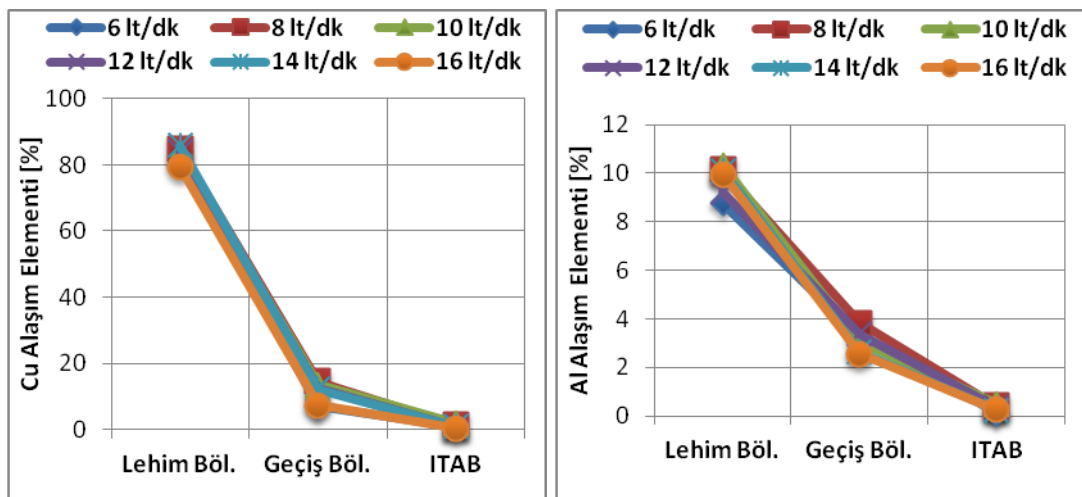
Şekil 6.137. Bindirme birleştirmedeki farklı gaz debilerinde birleştirilen galvanizsiz 7116 IF sacının Cu ve Al alaşımlarının bölgelere göre dağılımları
