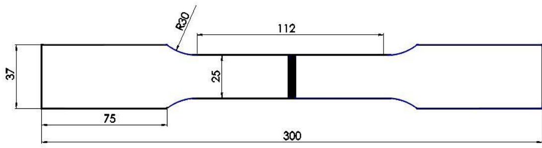
Şekil 5.12. Çekme deneyi numunesi boyutları
