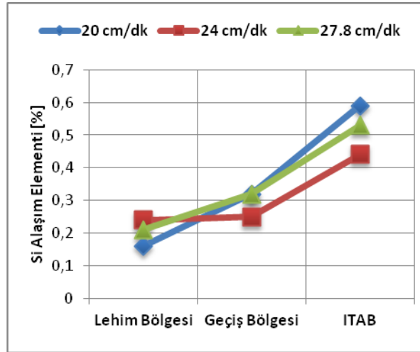
Şekil 6.82. Farklı akım şiddetlerinde birleştirilen 1315 IF sacının Cu, Al ve Si alaşımlarının difüzyon yüzdeleri
