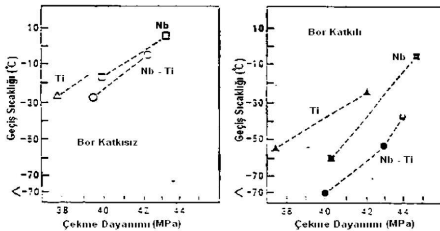
Şekil 3.3. IF-HSS çeliklerinde çekme dayanımı ile geçiş sıcaklığı arasındaki ilişki [55]
