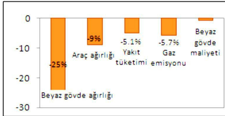
Şekil 2.5. Otomobil imalatında dikkat edilen 5 önemli unsurun AHSS çeliği kullanımıyla değişimi [43]
