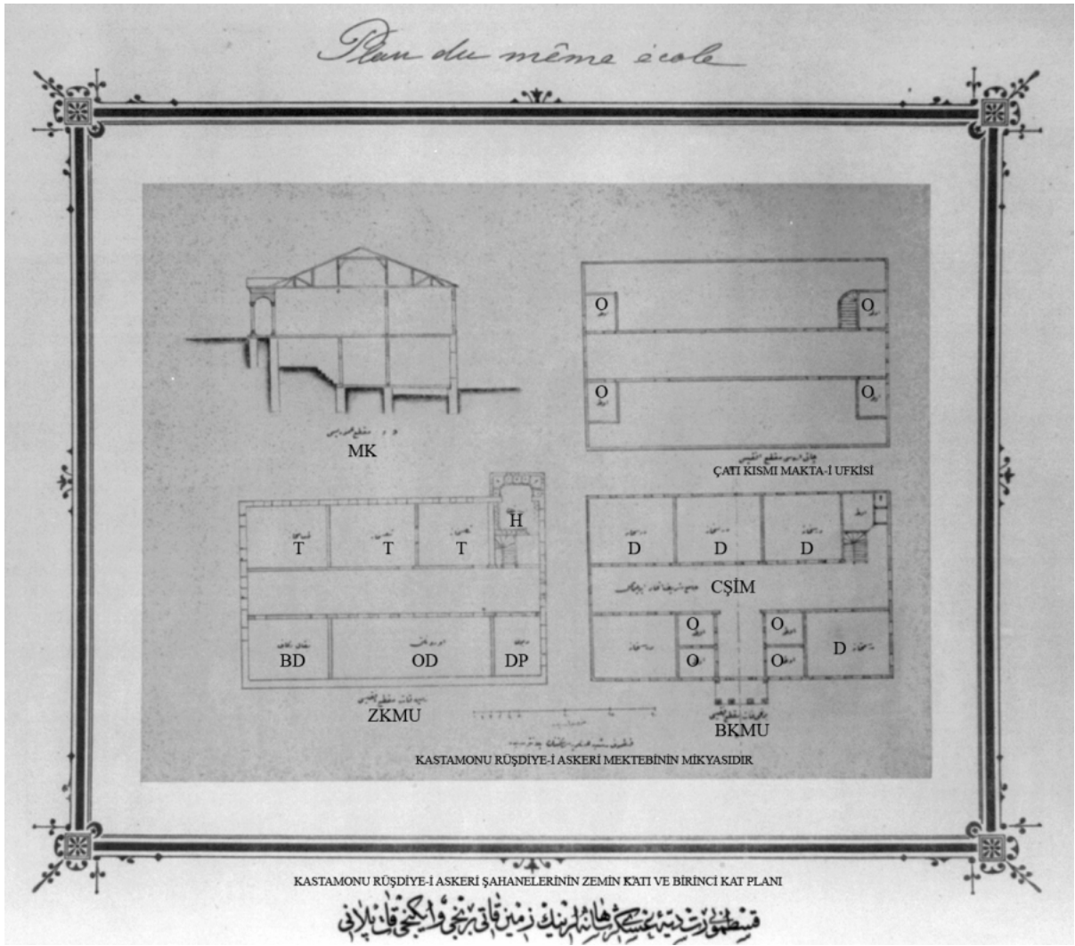
Fotoğraf No 100: Kastamonu Rüşdiye-i Askeri-i Şahaneleri Zemin Katı ve Birinci Kat Planı
