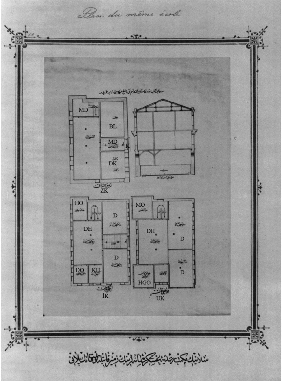
Fotoğraf No 150: Selanik Mekteb-i Rüşdiyye-i Askeri Şahaneleri Zemin Katla Üst Katın Planı
