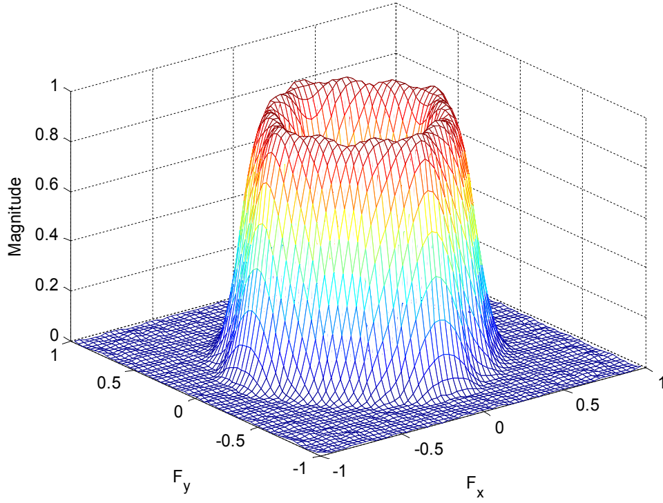
Şekil 6.7. 0.3 ve 0.6 arasındaki bir bantı geçiren; yaklaşık dairesel simetrik 2-D BGF
