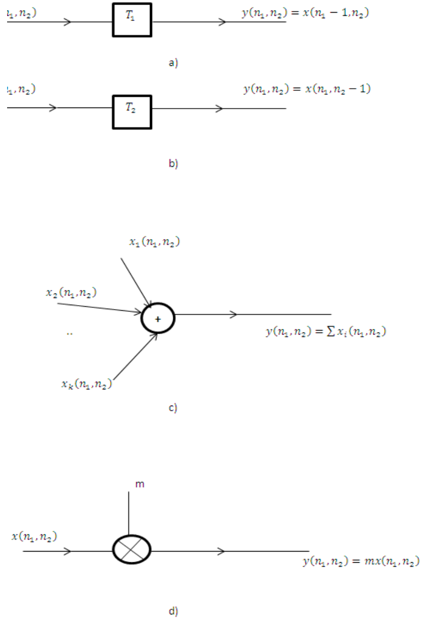
Şekil 3.4 2-D filtreler için temel elemanların sembolleri; a) Yatay kaydırıcı, b) Dikey kaydırıcı, c) Toplayıcı, d) Çarpıcı.
