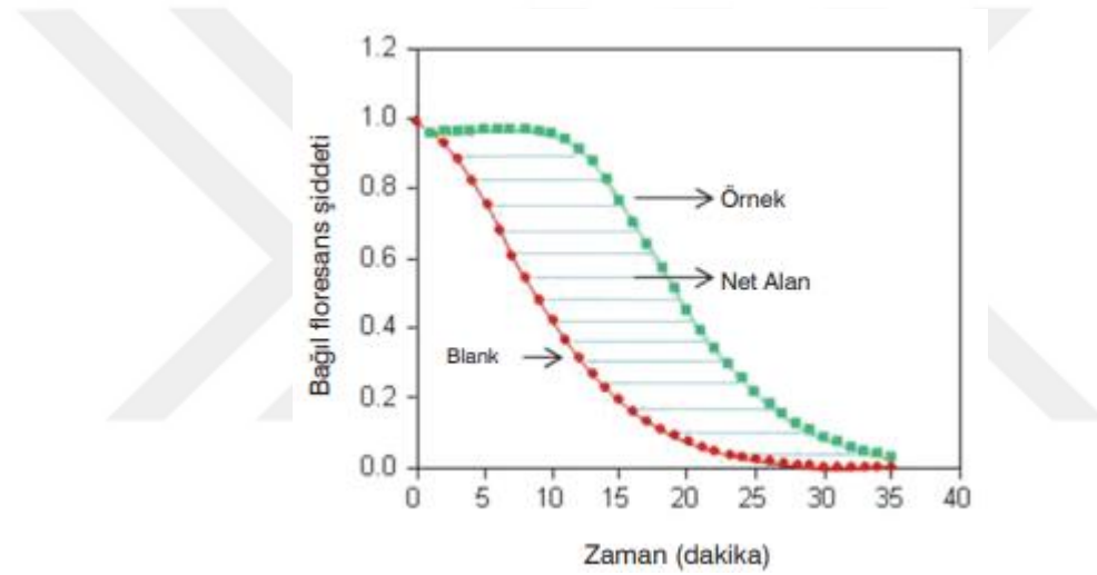
Şekil 2.1. ORAC yöntemiyle antioksidanın koruyucu etkisinin, floresans bozunma eğrisinin altındaki integre edilmiş net alandan hesaplanması.
