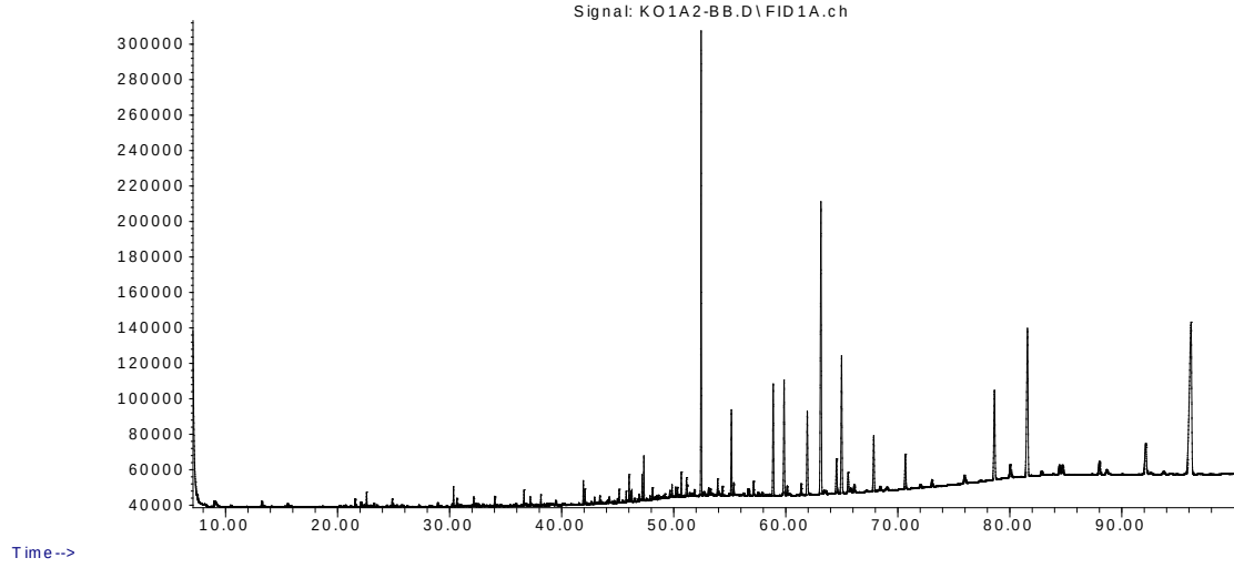
Şekil 4.10. SP-1 yaprak kısımlarından elde edilen sabit yağın yağ asitleri metil esterleri kromatogramı
