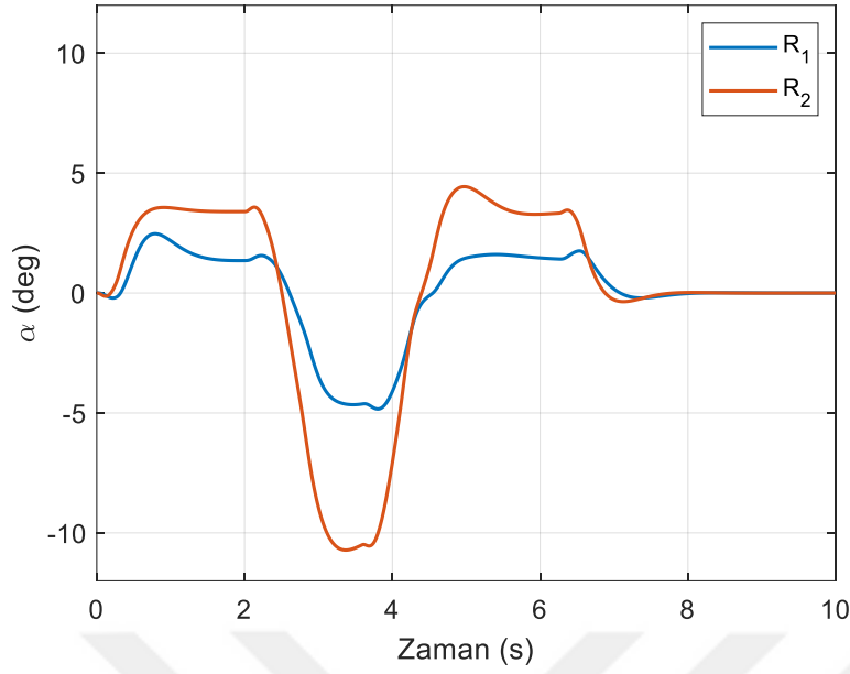
Şekil 6.35. SDRE kontrol yönteminde kabın açısı (yörünge II)
