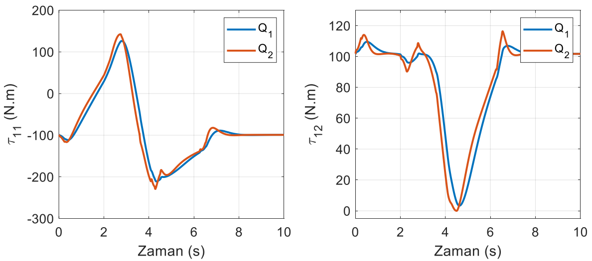
Şekil 6.88. LQR tekniğinde birinci robotun eklem torkları (yörünge II)
