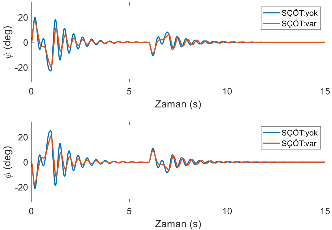
Şekil 6.116. Empedans kontrol yönteminde sıvı çalkalanma büyüklüğü (yörünge II)
