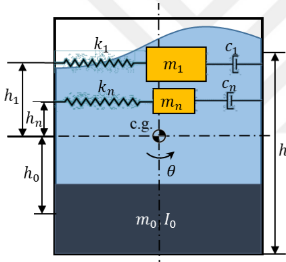
Şekil 2.1. Eşdeğer kütle-yay-damper mekanik modeli
