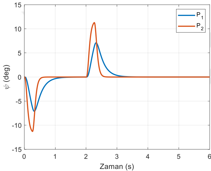
Şekil 6.48. Kutup yerleştirme tekniğinde sıvı çalkalanma büyüklüğü (yörünge I)
