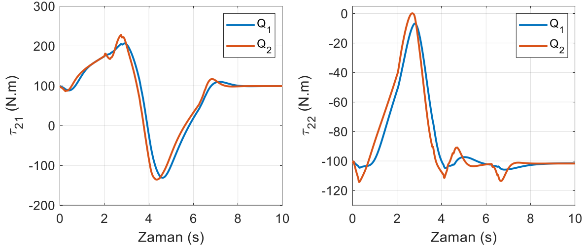
Şekil 6.47. SDRE kontrol yönteminde birinci robotun eklem torkları (yörünge II)
