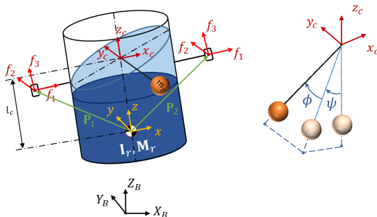
Şekil 4.3. Üç boyutlu çalkalanma: sarkaç modeli
