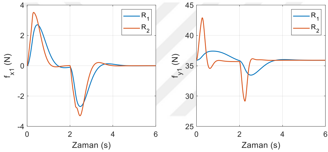
Şekil 6.23. SDRE kontrol yönteminde birinci robot kolundan kaba uygulanan kuvvetler (yörünge I)
