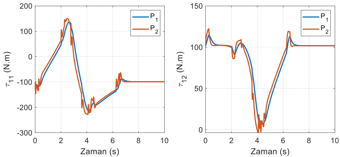
Şekil 6.60. Kutup yerleştirme tekniğinde birinci robotun eklem torkları (yörünge II)
