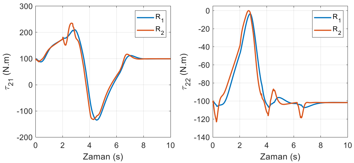
Şekil 6.40. SDRE kontrol yönteminde ikinci robotun eklem torkları (yörünge II)
