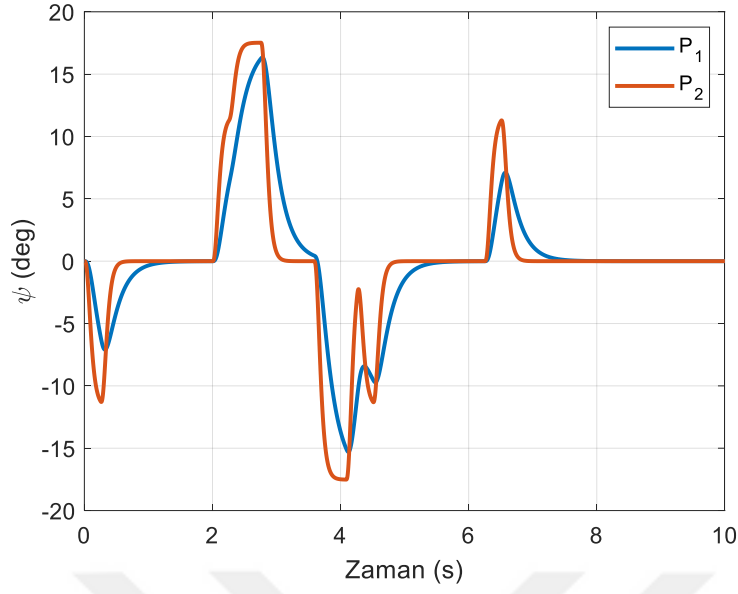
Şekil 6.55. Kutup yerleştirme tekniğinde sıvı çalkalanma büyüklüğü (yörünge II)
