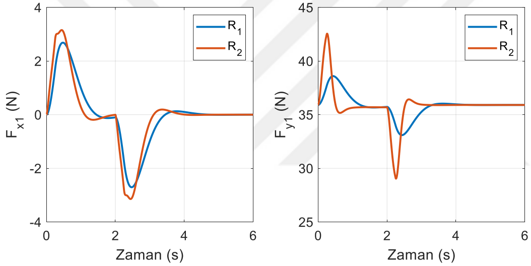
Şekil 6.65. LQR tekniğinde birinci robot kolundan kaba uygulanan kuvvetler (yörünge I)
