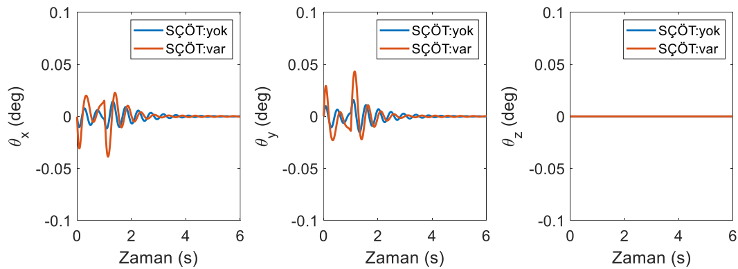
Şekil 6.113. Empedans kontrol yönteminde kabın oryantasyonu (yörünge I)
