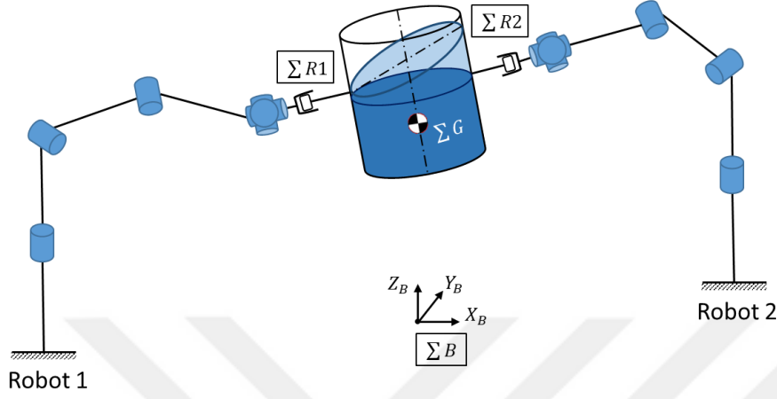
Şekil 3.2. Altı serbestlik dereceli iki robot kol ve birlikte taşıdıkları sıvı dolu kabın şematik gösterimi
