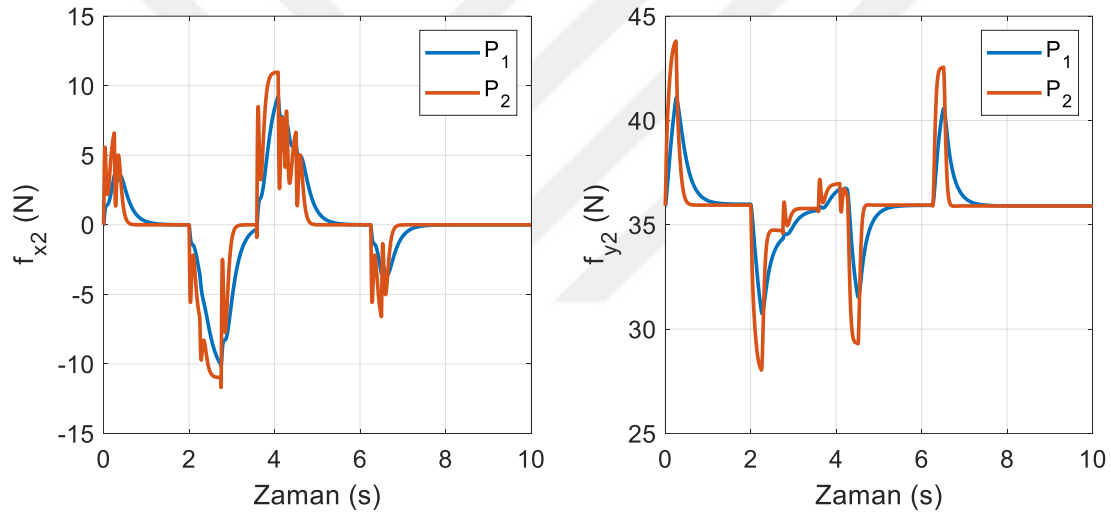
Şekil 6.59. Kutup yerleştirme tekniğinde ikinci robot kolundan kaba uygulanan kuvvetler (yörünge II)
