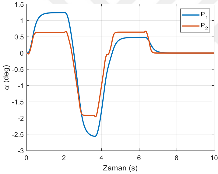
Şekil 6.56. Kutup yerleştirme tekniğinde kabın açısı (yörünge II)
