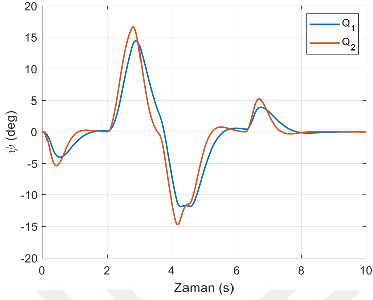
Şekil 6.41. SDRE kontrol yönteminde sıvı çalkalanma büyüklüğü (yörünge II)
