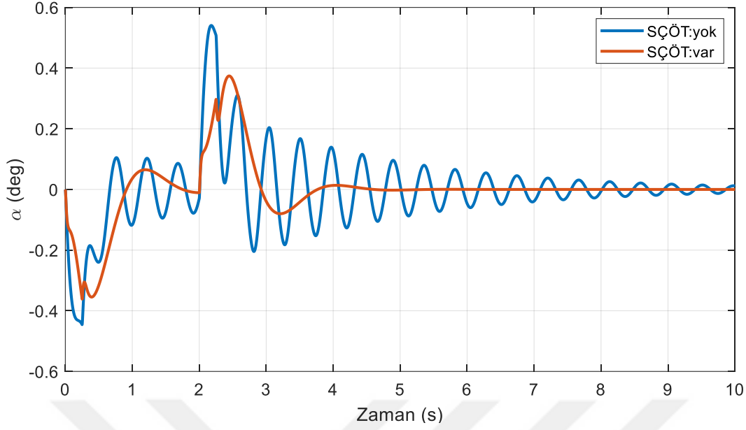
Şekil 6.11. Empedans kontrol yönteminde sıvı kabın açısı (yörünge I)
