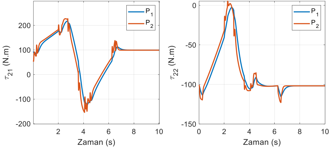
Şekil 6.61. Kutup yerleştirme tekniğinde ikinci robotun eklem torkları (yörünge II)
