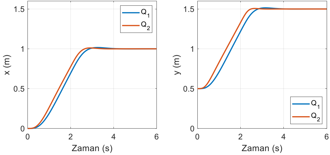
Şekil 6.71. LQR tekniğinde kabın konumu (yörünge I)
