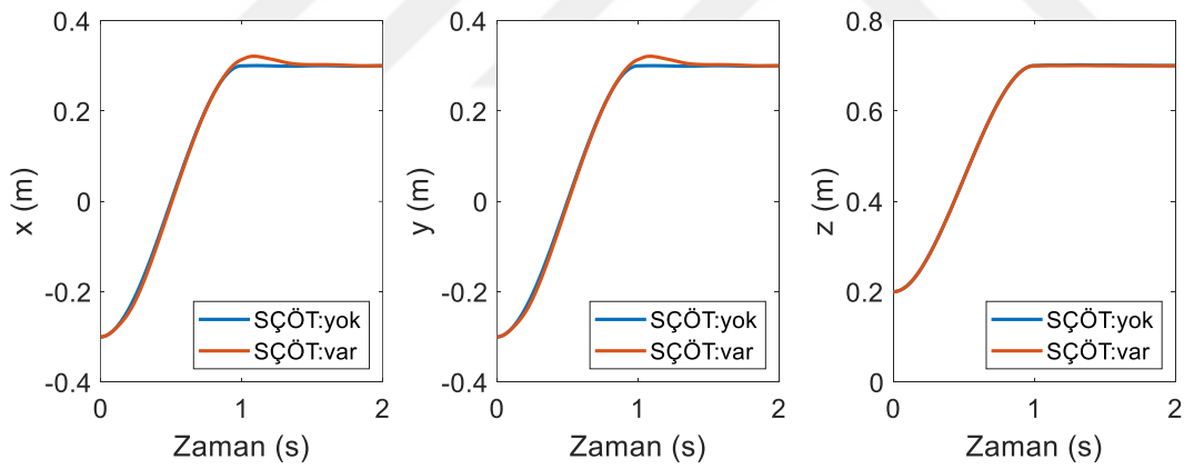
Şekil 6.112. Empedans kontrol yönteminde katı kütlenin ağırlık merkezinin konumu (yörünge I)
