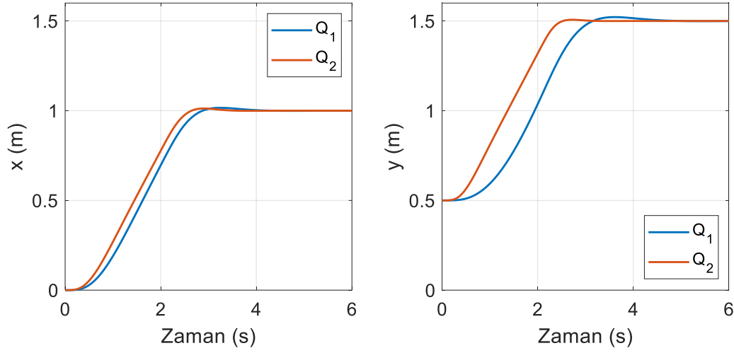
Şekil 6.29. SDRE kontrol yönteminde katı kütlenin ağırlık merkezinin konumu (yörünge I)
