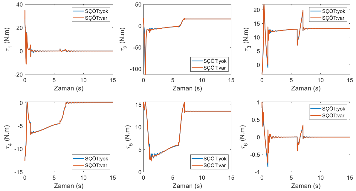
Şekil 6.119. Empedans kontrol yönteminde birinci robotun eklem torkları (yörünge II)
