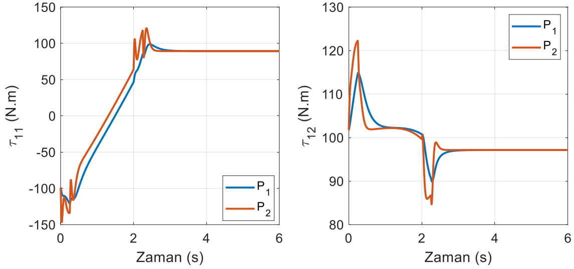
Şekil 6.53. Kutup yerleştirme tekniğinde birinci robotun eklem torkları (yörünge I)
