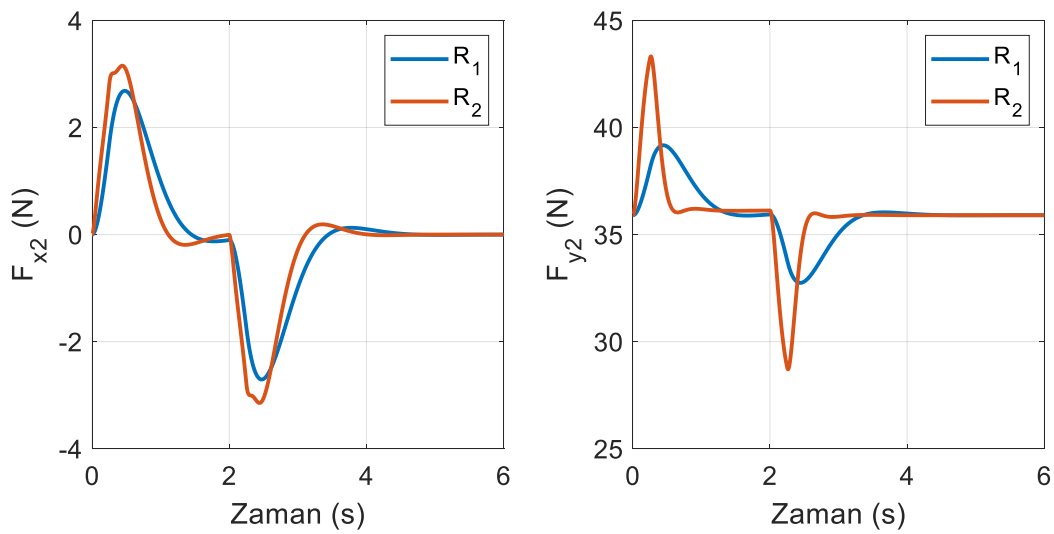
Şekil 6.66. LQR tekniğinde ikinci robot kolundan kaba uygulanan kuvvetler (yörünge I)
