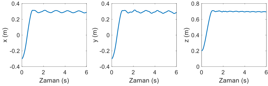
Şekil 6.105.Katı kütlenin ağırlık merkezinin konumu (yörünge I)
