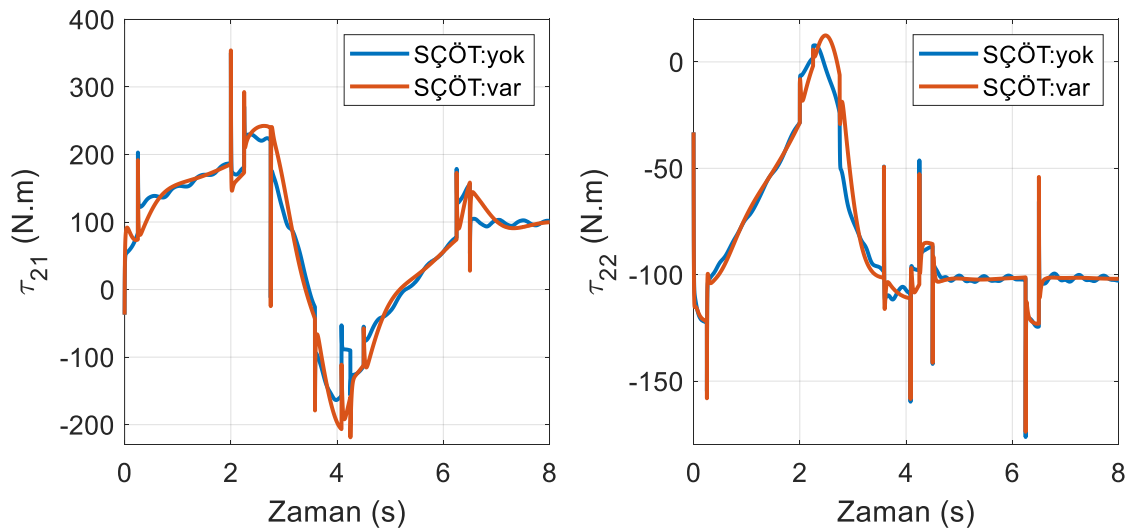
Şekil 6.19. Empedans kontrol yönteminde ikinci robotun eklem torkları (yörünge II)
