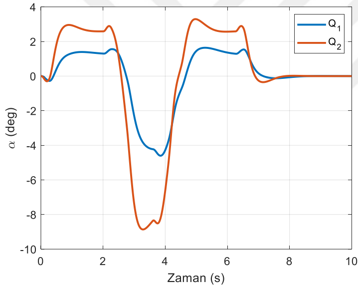
Şekil 6.84. LQR tekniğinde kabın açısı (yörünge II)
