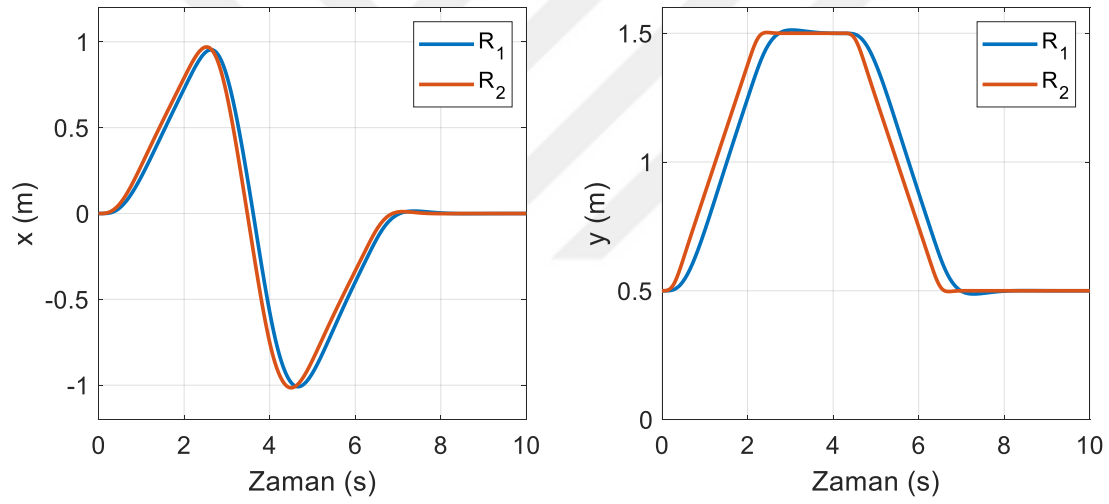
Şekil 6.78. LQR tekniğinde sıvı kabın konumu (yörünge II)
