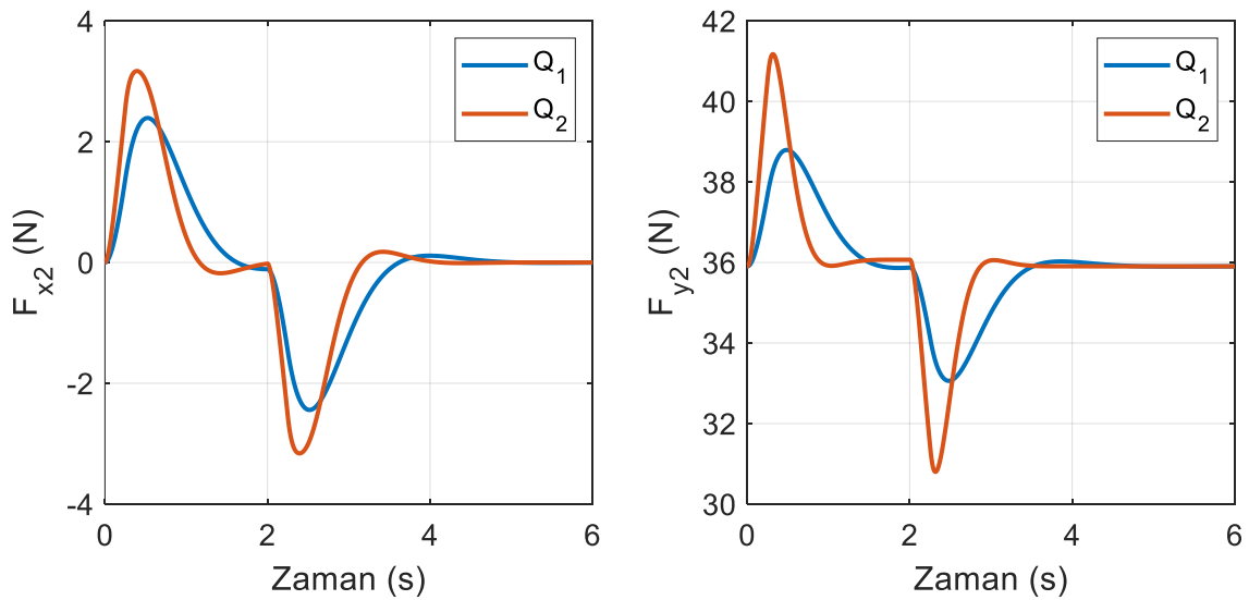
Şekil 6.73. LQR tekniğinde ikinci robot kolundan kaba uygulanan kuvvetler (yörünge I)
