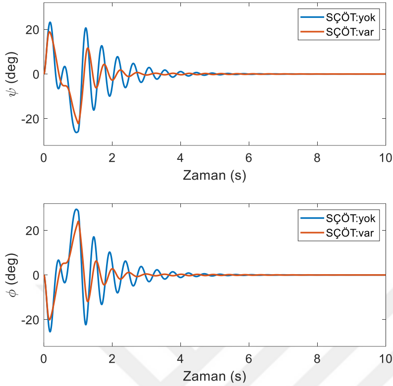
Şekil 6.111. Empedans kontrol yönteminde sıvı çalkalanma büyüklüğü (yörünge I)
