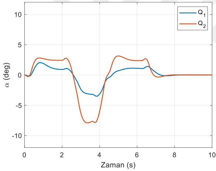
Şekil 6.42. SDRE kontrol yönteminde kabın açısı (yörünge II)
