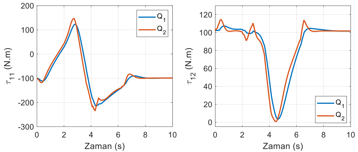
Şekil 6.46. SDRE kontrol yönteminde birinci robotun eklem torkları (yörünge II)
