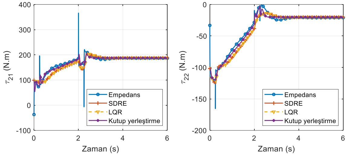
Şekil 6.94. İkinci robot kolun eklem torkları (yörünge I)
