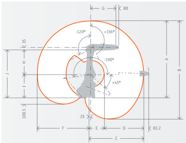
Şekil 3.4. KUKA KR6 R900'ün link yapısı
