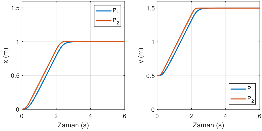
Şekil 6.50. Kutup yerleştirme tekniğinde kabın konumu (yörünge I)
