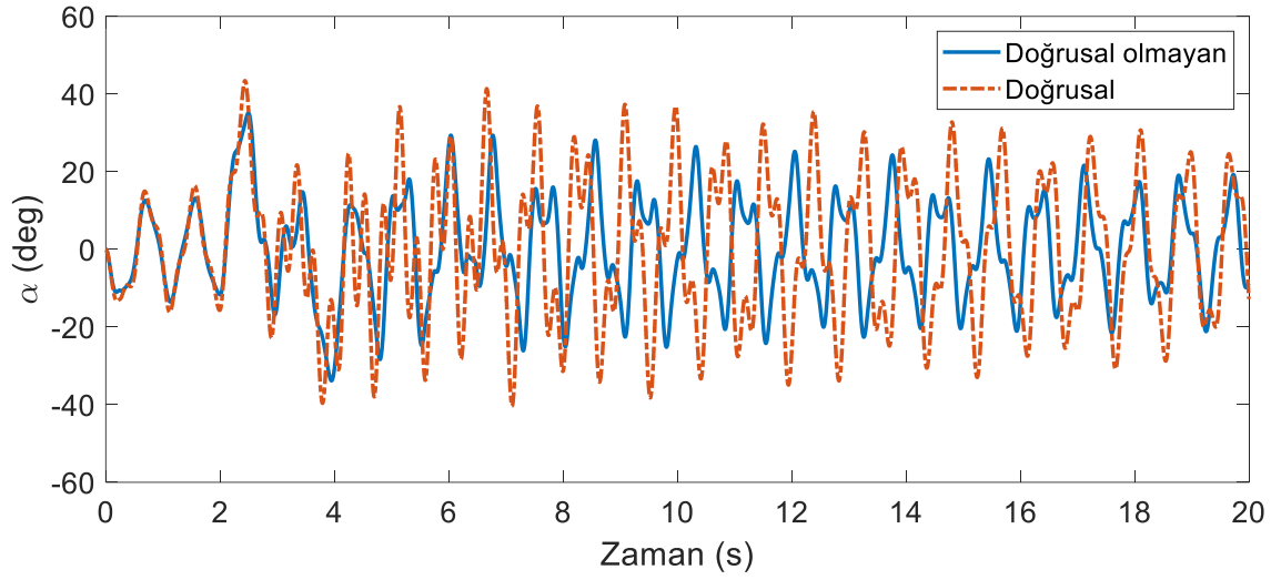
Şekil 6.8. Kabın açısı
