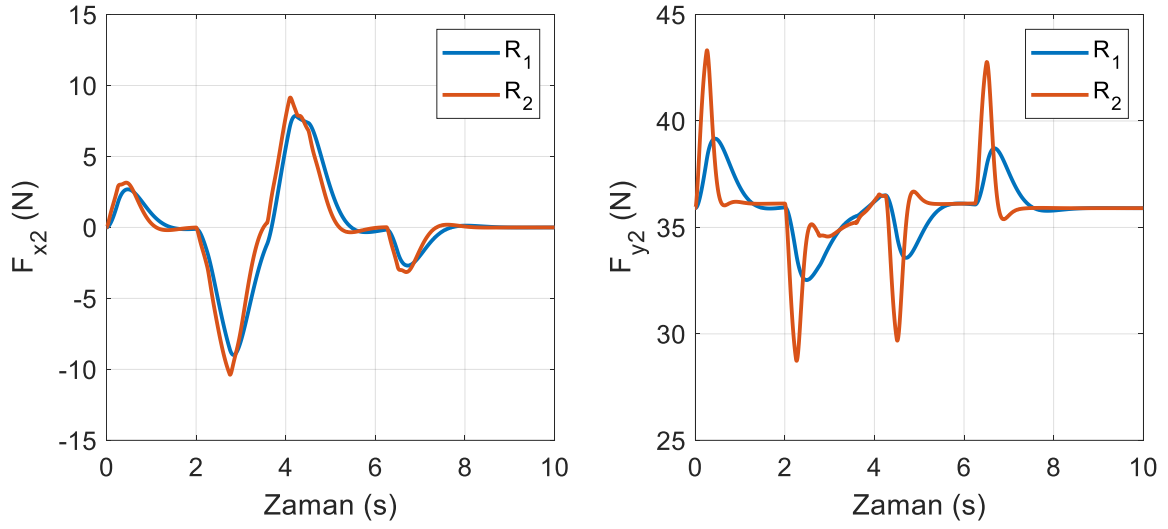
Şekil 6.80. LQR tekniğinde ikinci robot kolundan kaba uygulanan kuvvetler (yörünge II)
