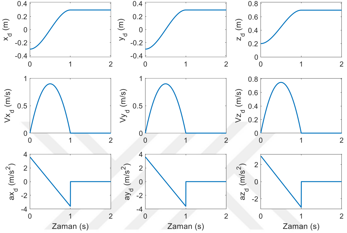
Şekil 6.103. Katı kütlenin ağırlık merkezinin izlenmesi istenen hareket profilleri
