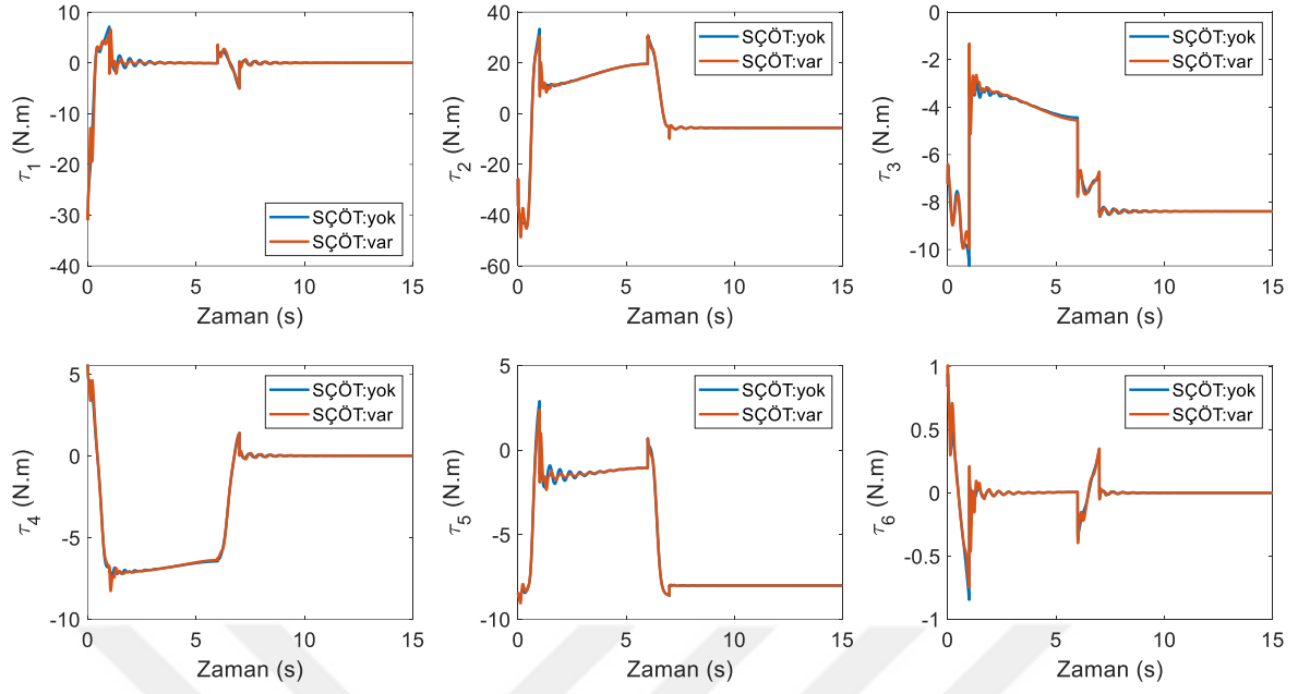
Şekil 6.120. Empedans kontrol yönteminde ikinci robotun eklem torkları (yörünge II)
