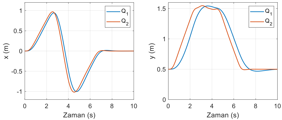
Şekil 6.43. SDRE kontrol yönteminde kabın konumu (yörünge II)
