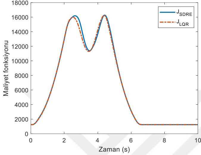
Şekil 6.101. SDRE ve LQR yöntemlerinin maliyet fonksiyonu (yörünge II)
