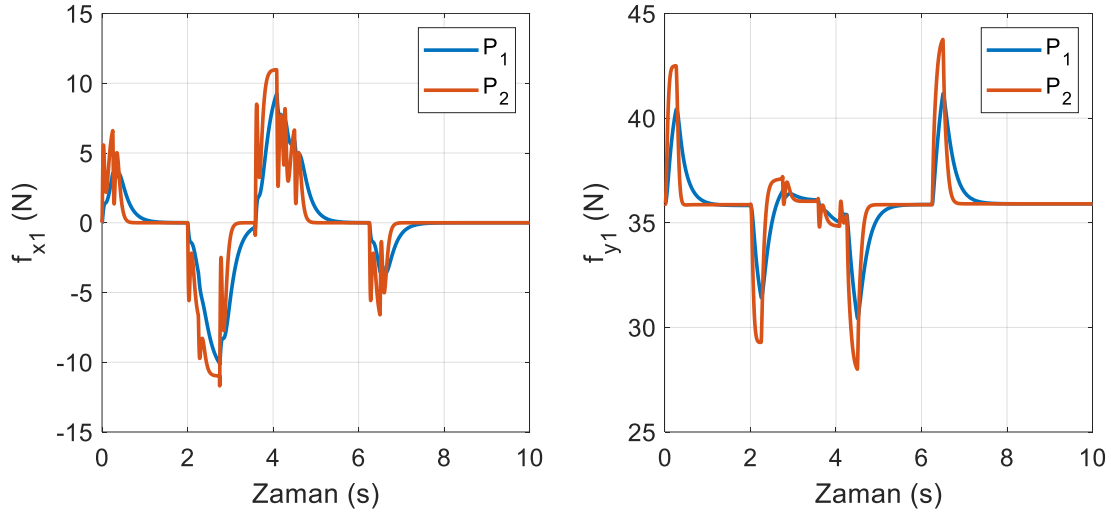
Şekil 6.58. Kutup yerleştirme tekniğinde birinci robot kolundan kaba uygulanan kuvvetler (yörünge II)
