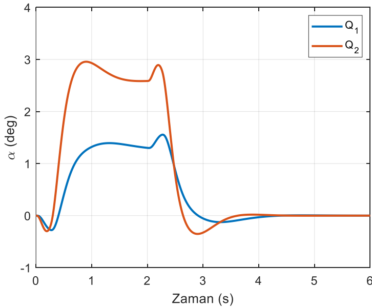
Şekil 6.70. LQR tekniğinde sıvı kabın açısı (yörünge I)
