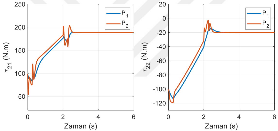
Şekil 6.54. Kutup yerleştirme tekniğinde ikinci robotun eklem torkları (yörünge I)
