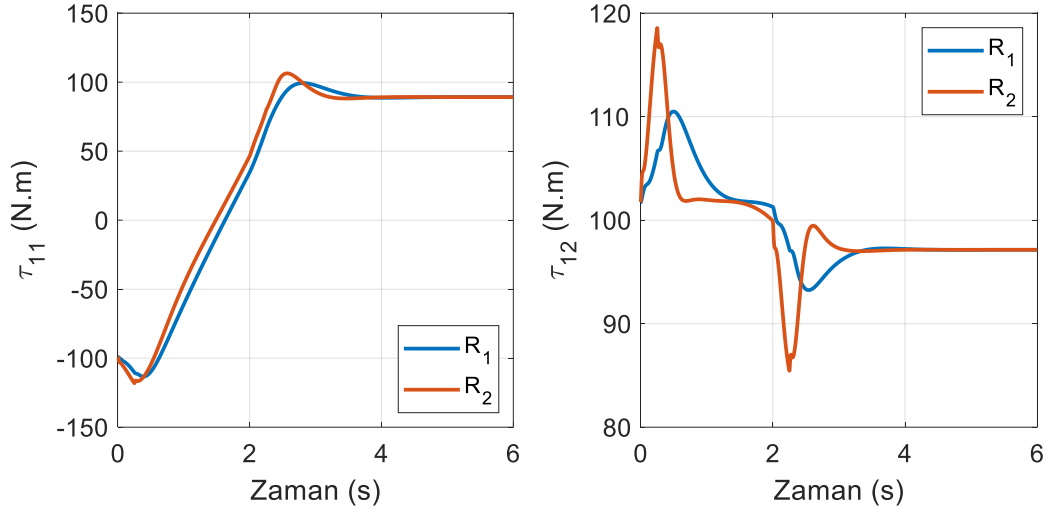
Şekil 6.67. LQR tekniğinde birinci robotun eklem torkları (yörünge I)
