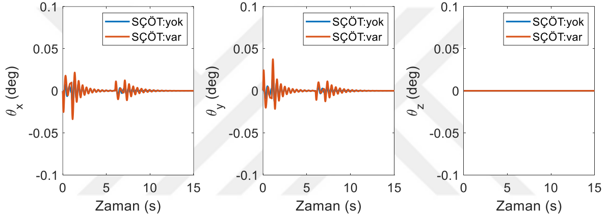
Şekil 6.118. Empedans kontrol yönteminde kabın oryantasyonu (yörünge II)
