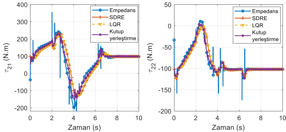
Şekil 6.100. İkinci robot kolun eklem torkları (yörünge II)
