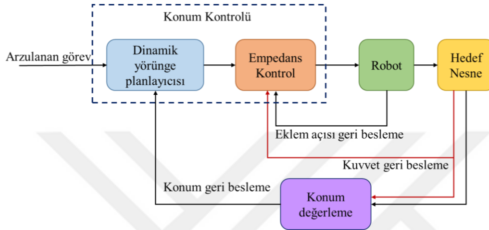
Şekil 2.6. Empedans kontrol blok diyagramı
