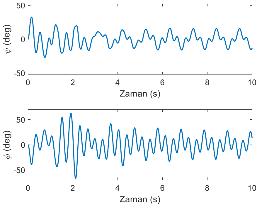
Şekil 6.104. Sıvı çalkalanmanın büyüklüğü (yörünge I)
