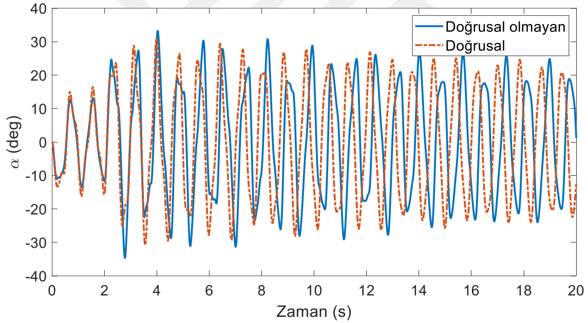
Şekil 6.3. Kabın açısı
