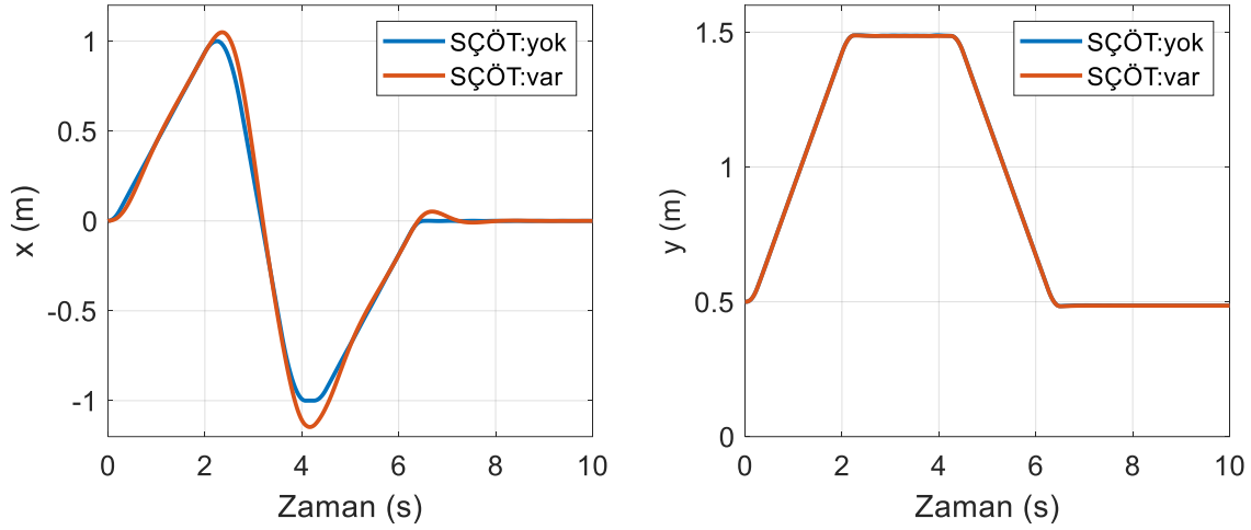
Şekil 6.17. Empedans kontrol yönteminde katı kütlenin ağırlık merkezinin konumu (yörünge II)
