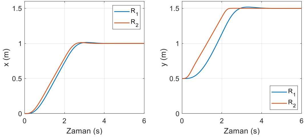
Şekil 6.22. SDRE kontrol yönteminde katı kütlenin ağırlık merkezinin konumu (yörünge I)
