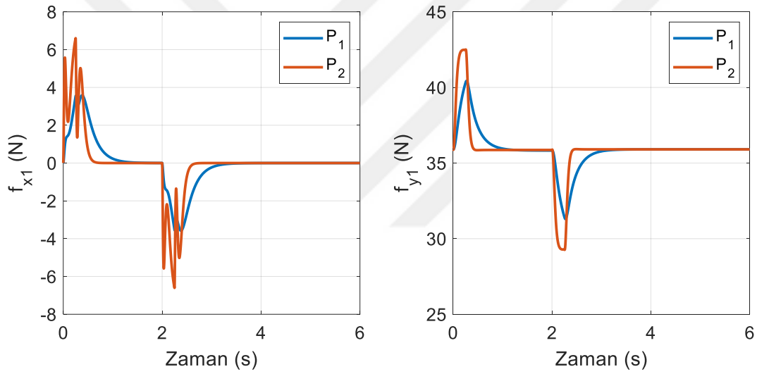
Şekil 6.51. Kutup yerleştirme tekniğinde birinci robot kolundan kaba uygulanan kuvvetler (yörünge I)
