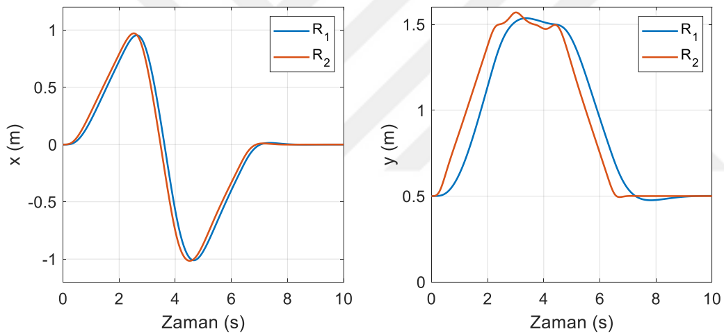
Şekil 6.36. SDRE kontrol yönteminde kabın konumu (yörünge II)
