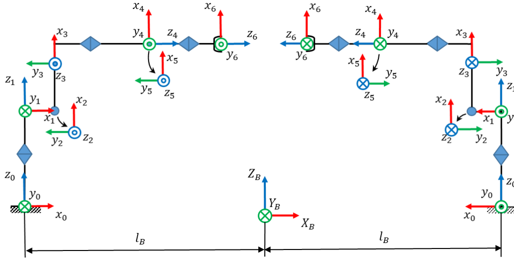
Şekil 3.5. İki KUKA KR6 R900 robot kollarının eksen takımlarının gösterimi
