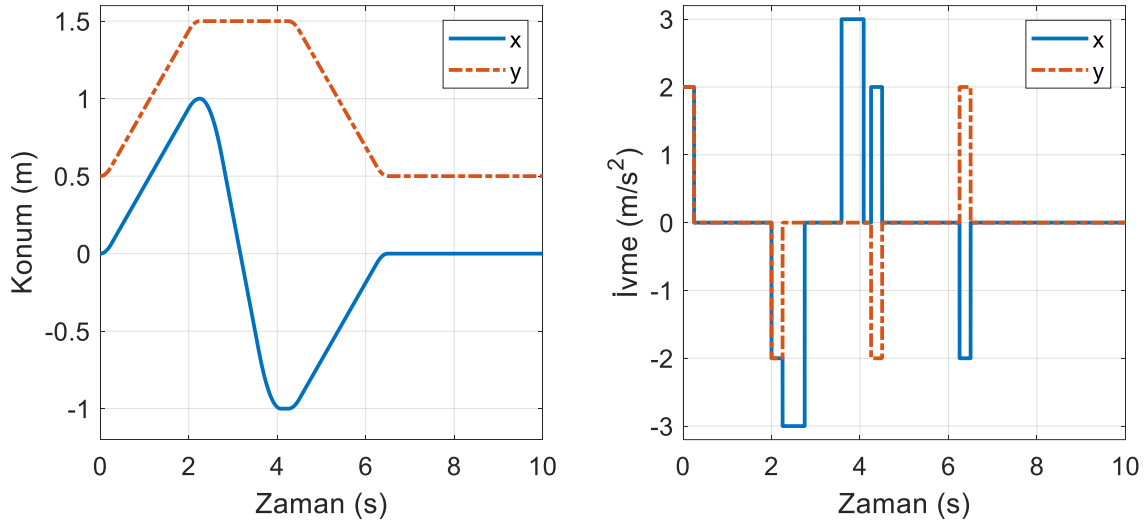
Şekil 6.6. Katı kütleli ağırlık merkezinin izlenmesi istenen çoklu hareket profili
