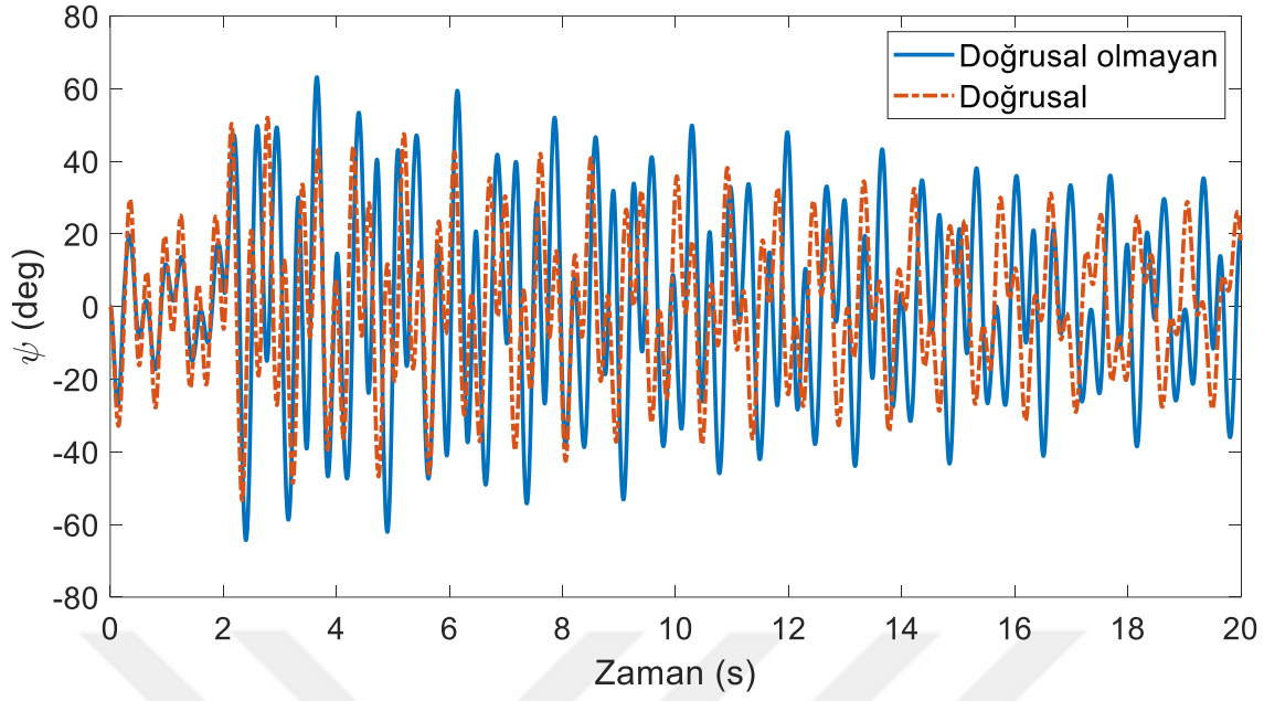
Şekil 6.2. Çalkalanmanın büyüklüğü (Sarkacın açısı)
