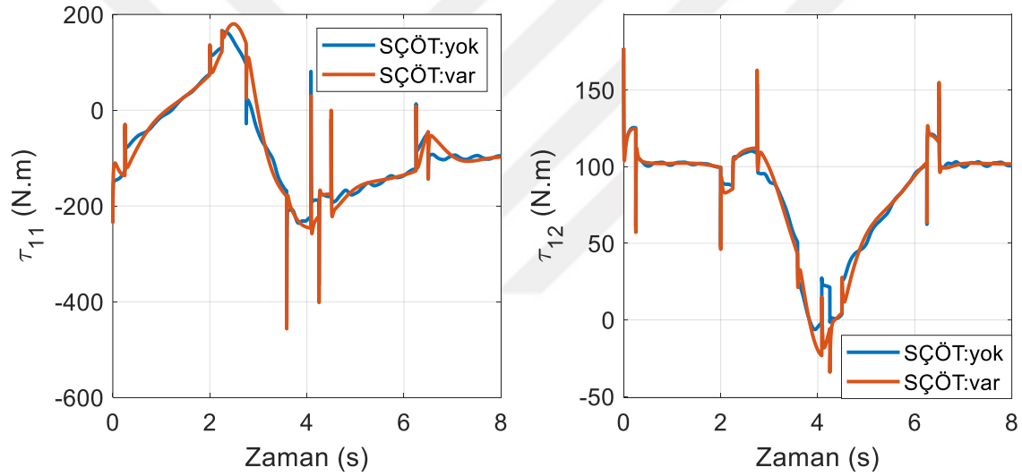
Şekil 6.18. Empedans kontrol yönteminde birinci robotun eklem torkları (yörünge II)
