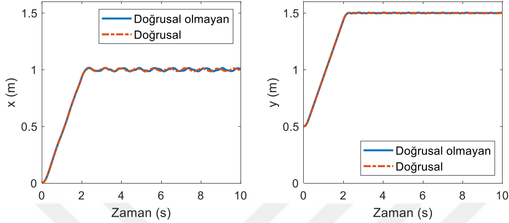
Şekil 6.4. Kabın konumu
