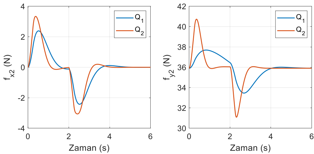
Şekil 6.31. SDRE kontrol yönteminde ikinci robot kolundan kaba uygulanan kuvvetler (yörünge I)
