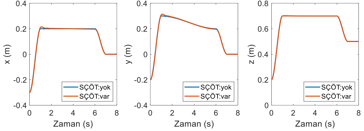
Şekil 6.117. Empedans kontrol yönteminde katı kütlenin ağırlık merkezinin konumu (yörünge II)
