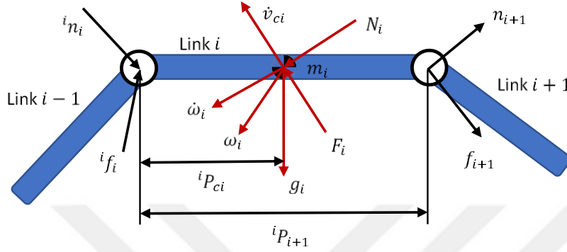
Şekil 4.1. Linklere etkileyen kuvvet ve momentler
