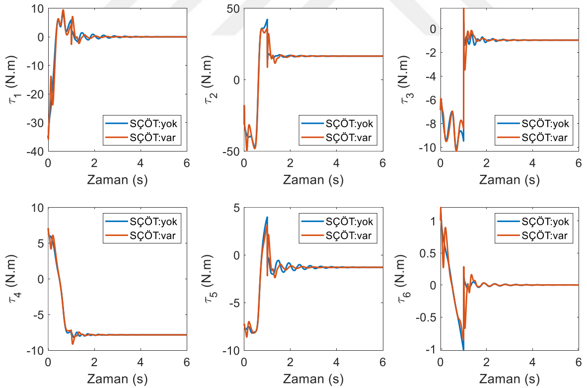
Şekil 6.115. Empedans kontrol yönteminde ikinci robotun eklem torkları (yörünge I)
