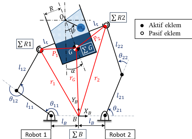
Şekil 3.6. İki düzlemsel kooperatif robot, sıvı kap ve kısıtlama vektörlerinin şematığı
