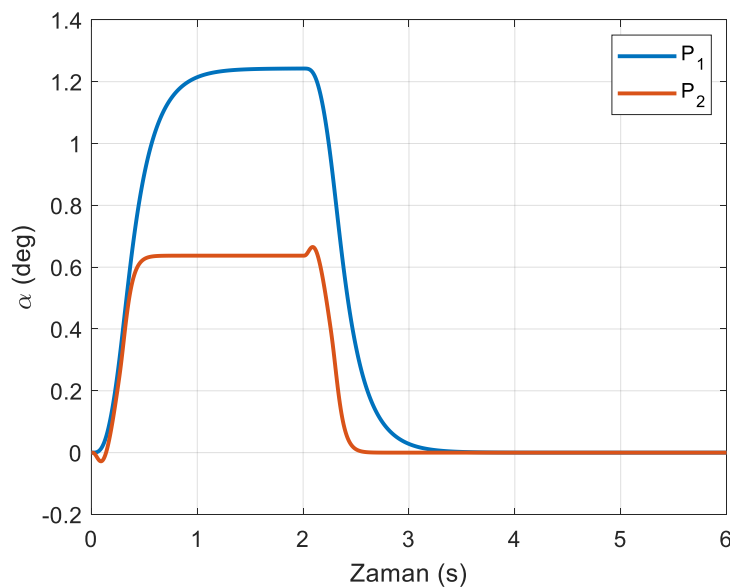
Şekil 6.49. Kutup yerleştirme tekniğinde kabın açısı (yörünge I)
