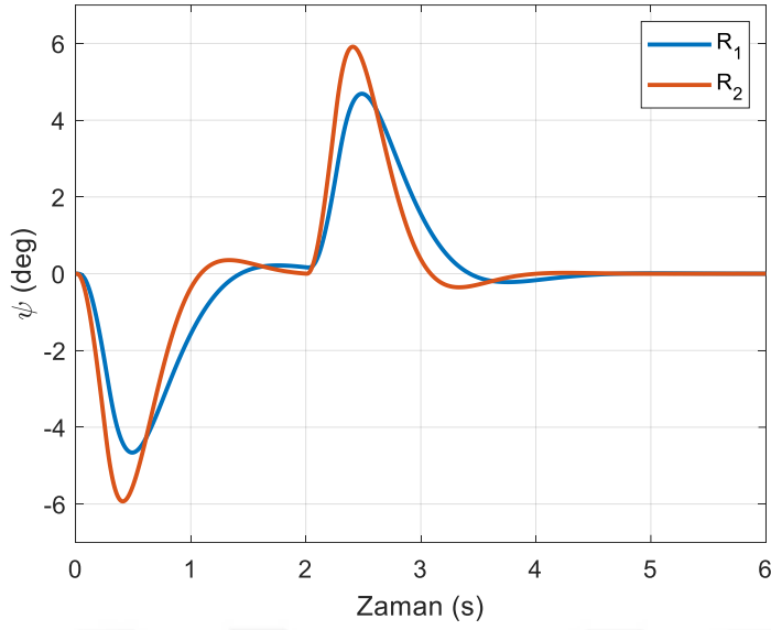
Şekil 6.62. LQR tekniğinde sıvı çalkalanma büyüklüğü (yörünge I)
