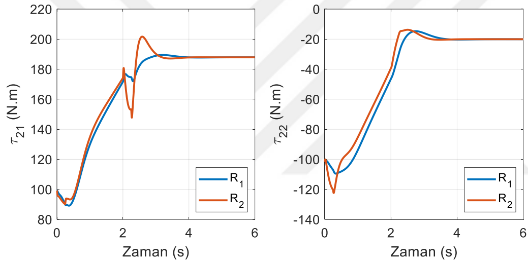
Şekil 6.68. LQR tekniğinde ikinci robotun eklem torkları (yörünge I)
