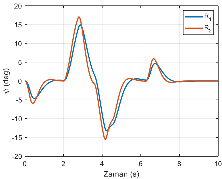
Şekil 6.76. LQR tekniğinde sıvı çalkalanma büyüklüğü (yörünge II)
