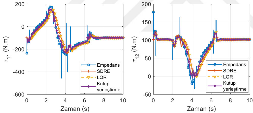
Şekil 6.99. Birinci robot kolun eklem torkları (yörünge II)
