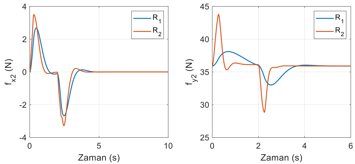
Şekil 6.24. SDRE kontrol yönteminde ikinci robot kolundan kaba uygulanan kuvvetler (yörünge I)
