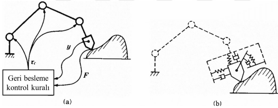
Şekil 2.5. Aktif empedans yöntemi. (a) geri bildirim kontrol sistemi. (b) mekanik empedansı (a)'dan gerçekleştirilmektedir [118].
