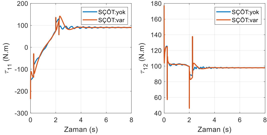
Şekil 6.13. Empedans kontrol yönteminde birinci robotun eklem torkları (yörünge I)
