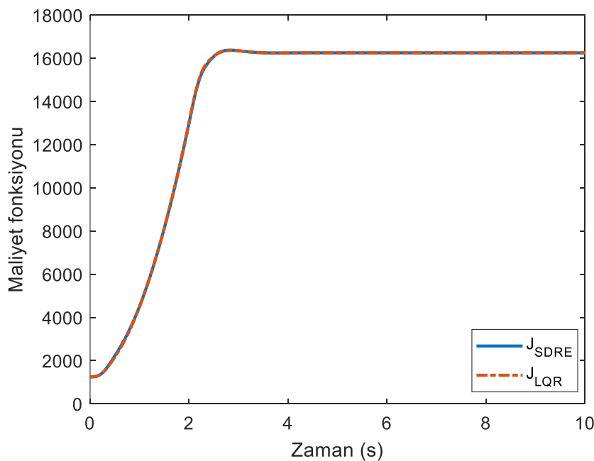
Şekil 6.95. SDRE ve LQR yöntemlerinin maliyet fonksiyonu (yörünge I)
