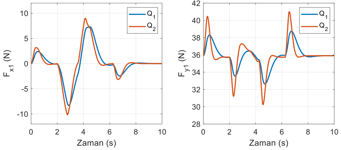
Şekil 6.86. LQR tekniğinde birinci robot kolundan kaba uygulanan kuvvetler (yörünge II)
