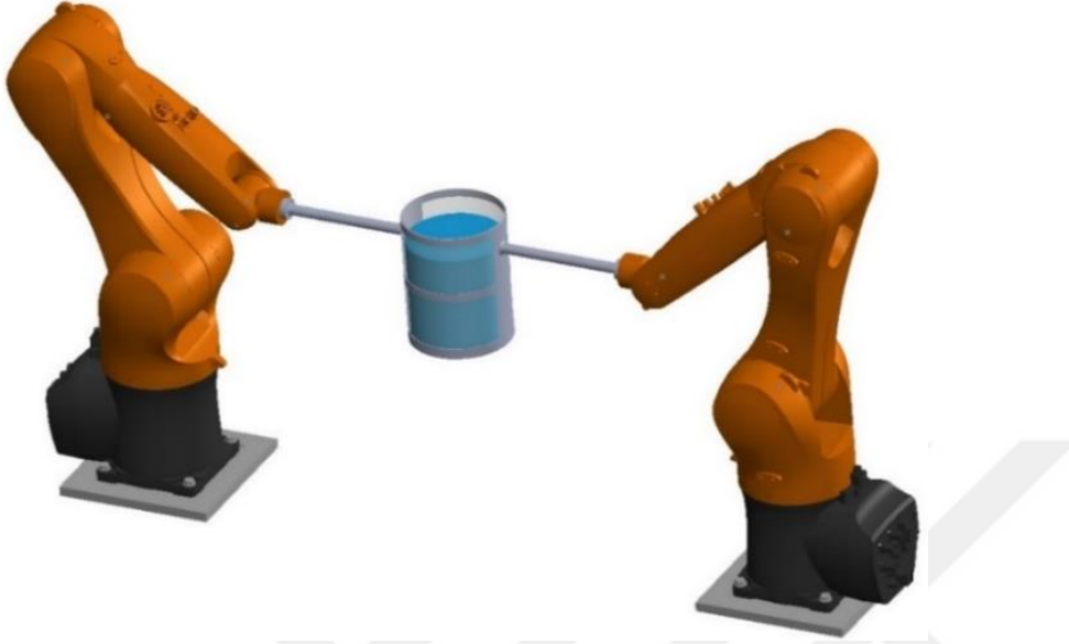
Şekil 6.102. İki KUKA KR 6 R900 robot kolu ile sıvı dolu silindirik kabın taşınımı
