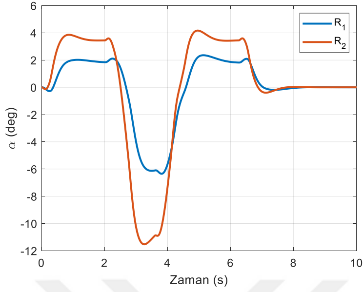
Şekil 6.77. LQR tekniğinde kabın açısı (yörünge II)
