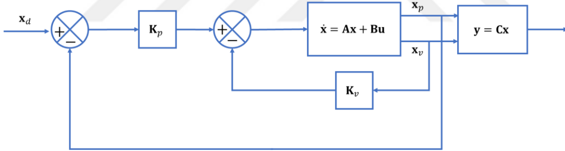
Şekil 5.1. Geri beslemeli kutup yerleştirme kontrol blok diyagramı
