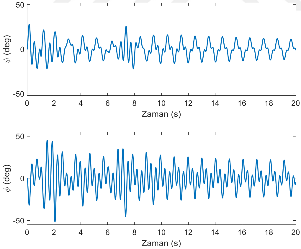
Şekil 6.108. Sıvı çalkalanma büyüklüğü (yörünge II)
