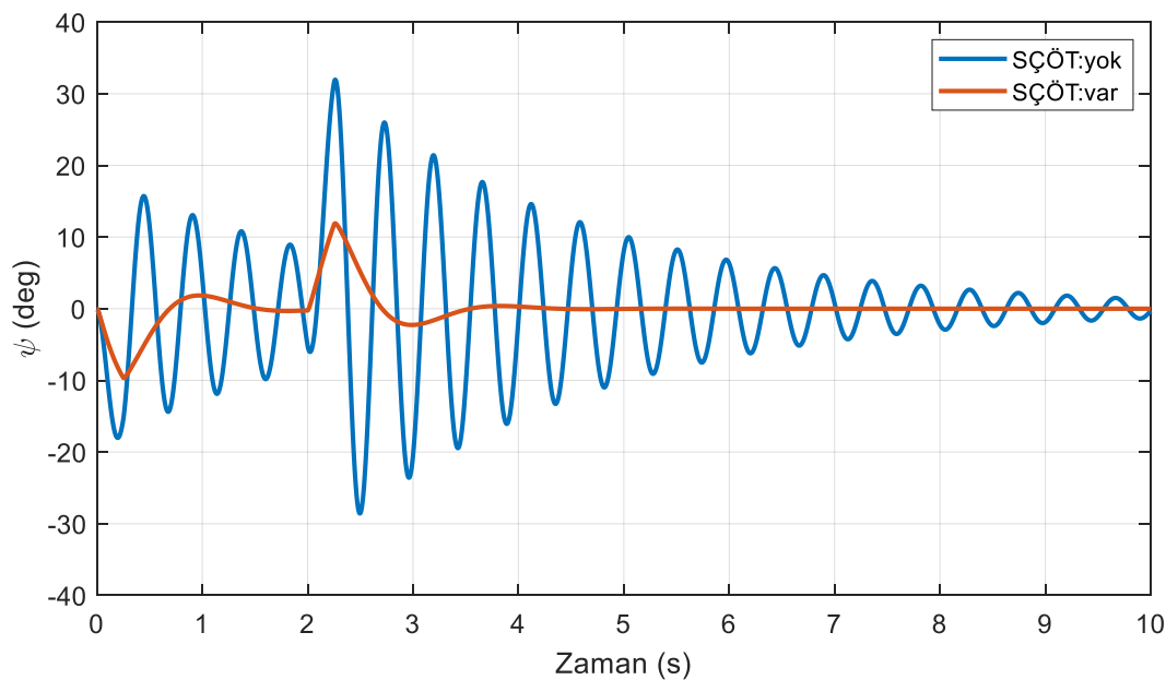
Şekil 6.10. Empedans kontrol yönteminde sıvı çalkalanma büyüklüğü (yörünge I)
