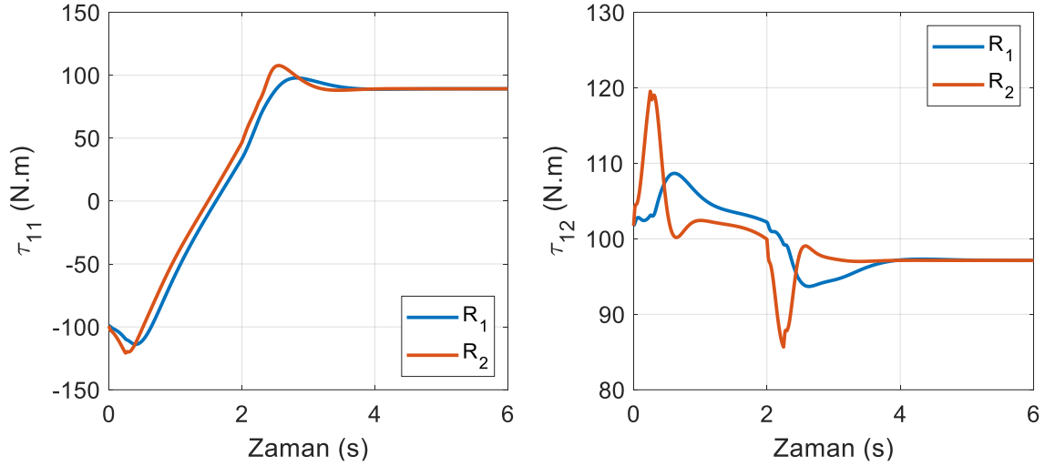
Şekil 6.25. SDRE kontrol yönteminde birinci robotun eklem torkları (yörünge I)
