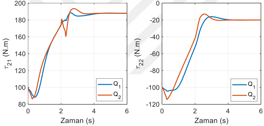
Şekil 6.33. SDRE kontrol yönteminde ikinci robotun eklem torkları (yörünge I)
