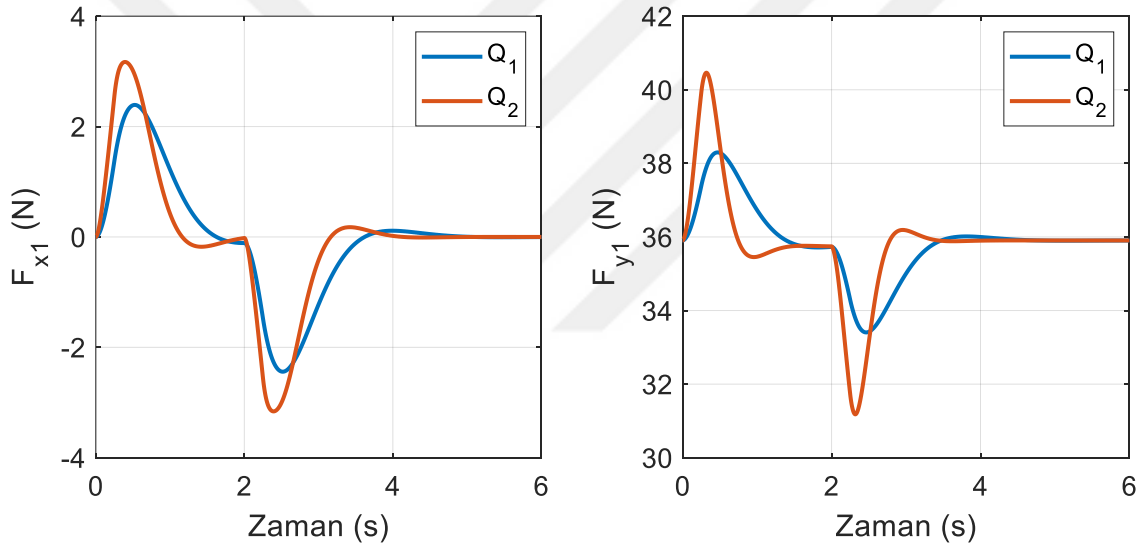
Şekil 6.72. LQR tekniğinde birinci robot kolundan kaba uygulanan kuvvetler (yörünge I)
