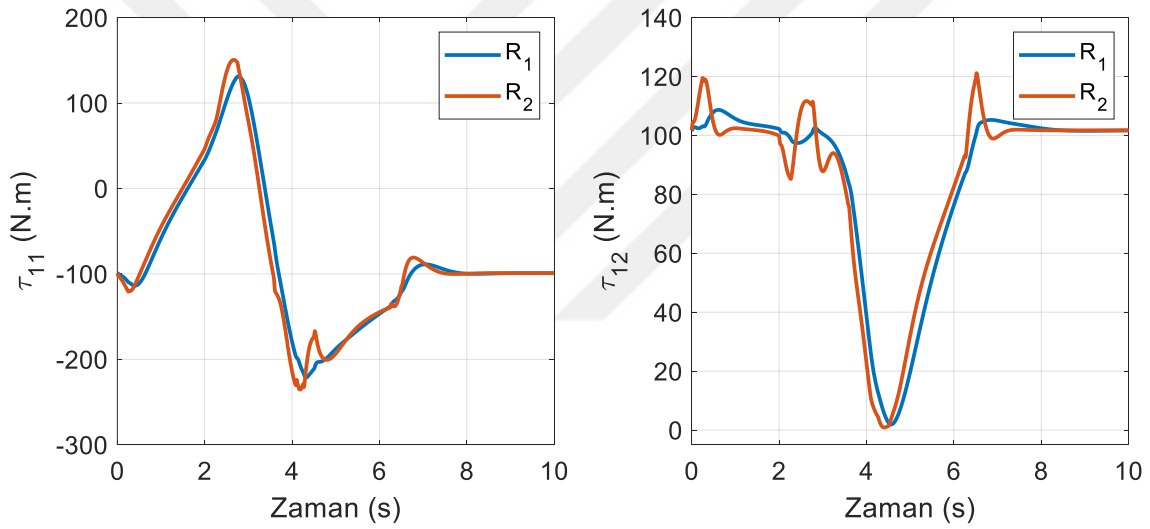
Şekil 6.39. SDRE kontrol yönteminde birinci robotun eklem torkları (yörünge II)
