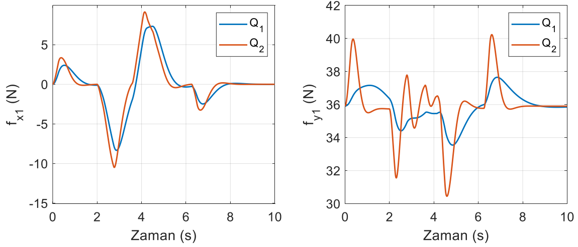
Şekil 6.44. SDRE kontrol yönteminde birinci robotun kaba uyguladığı kuvvetler (yörünge II)
