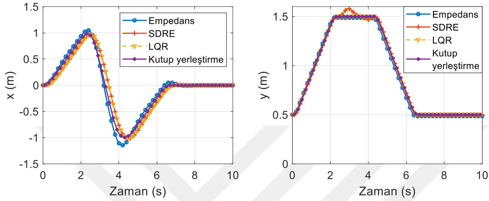
Şekil 6.98. Katı kütlenin ağırlık merkezinin konumu (yörünge II)
