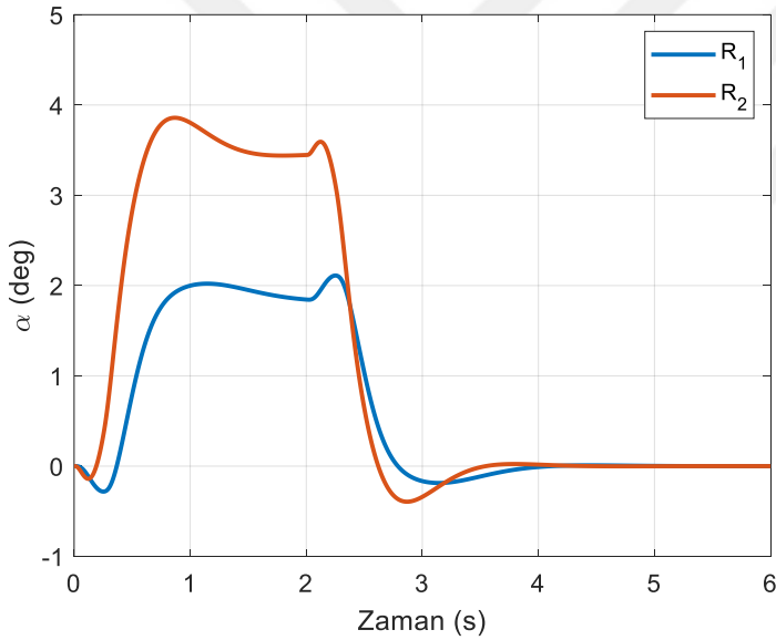
Şekil 6.63. LQR tekniğinde sıvı kabın açısı (yörünge I)
