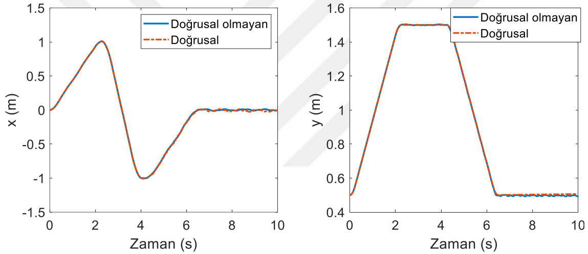
Şekil 6.9. Kabın konumu
