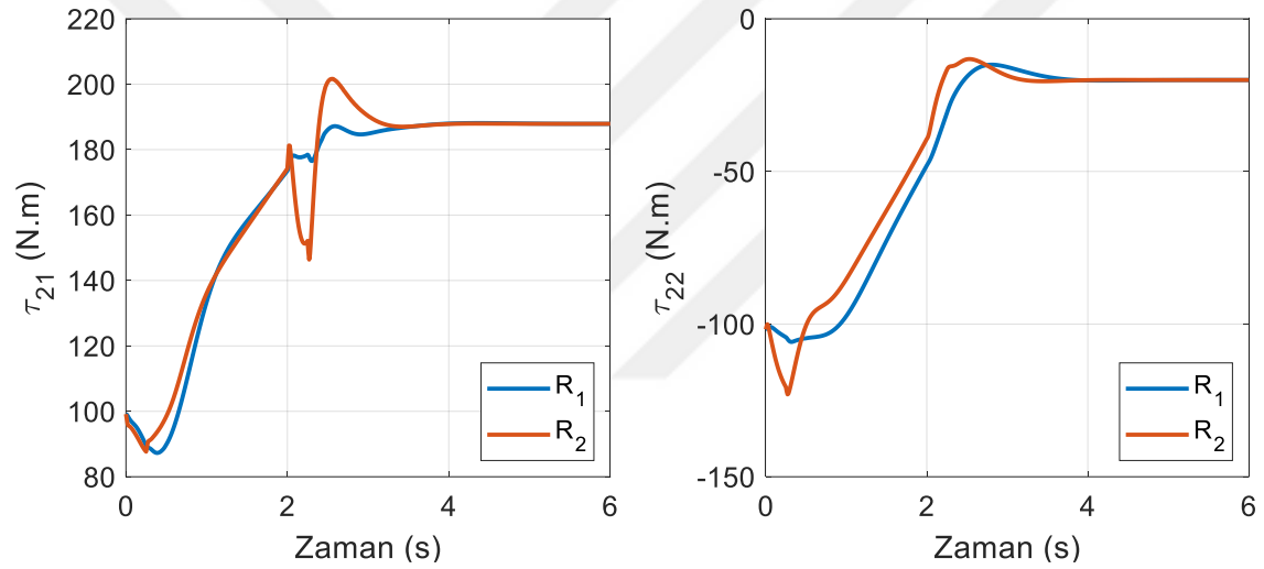
Şekil 6.26. SDRE kontrol yönteminde ikinci robotun eklem torkları (yörünge I)
