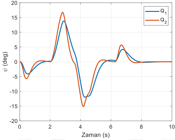
Şekil 6.83. LQR tekniğinde sıvı çalkalanma büyüklüğü (yörünge II)
