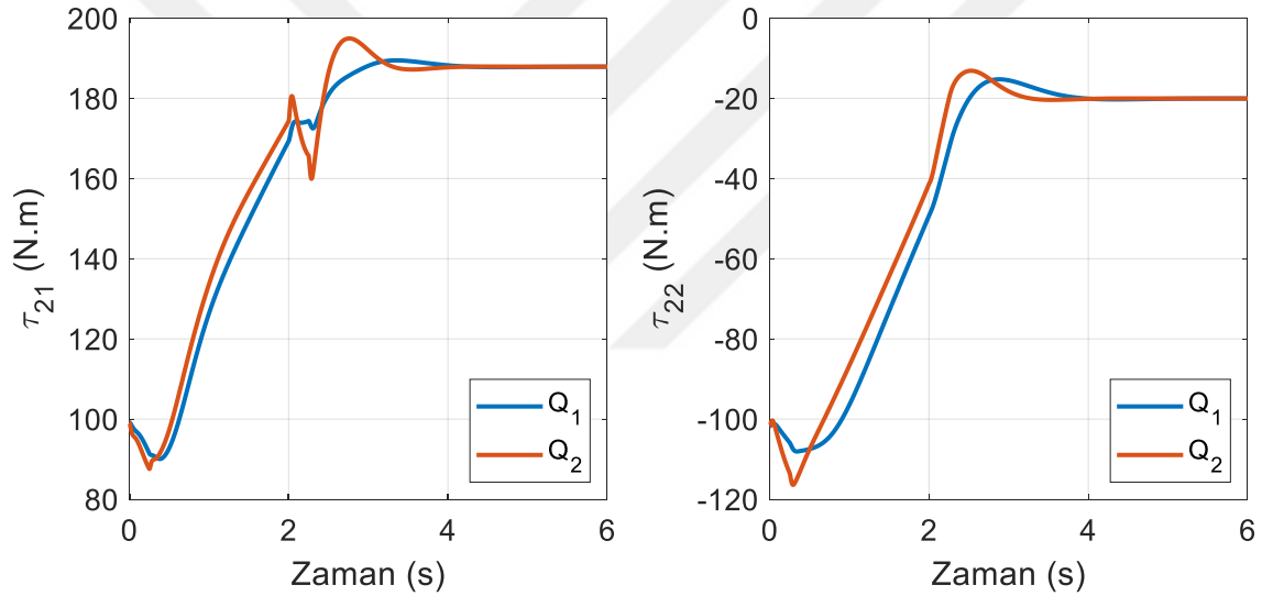
Şekil 6.75. LQR tekniğinde ikinci robotun eklem torkları (yörünge I)
