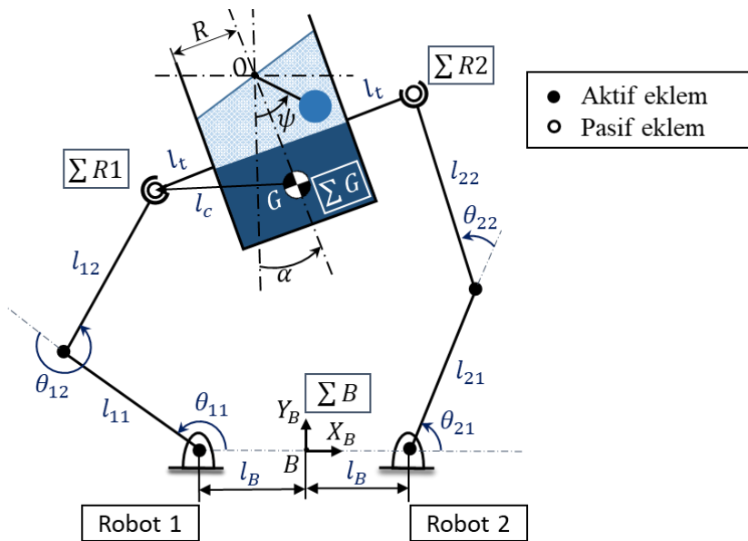
Şekil 3.1. Düzlemsel iki robot kol ve birlikte taşıdıkları sıvı dolu kabın şematik gösterimi
