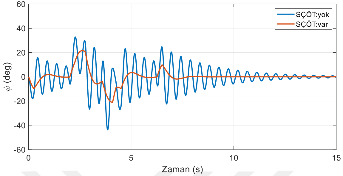
Şekil 6.15. Empedans kontrol yönteminde sıvı çalkalanma büyüklüğü (yörünge II)
