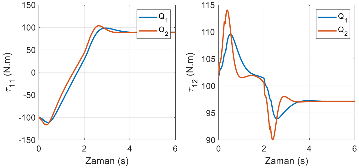
Şekil 6.74. LQR tekniğinde birinci robotun eklem torkları (yörünge I)
