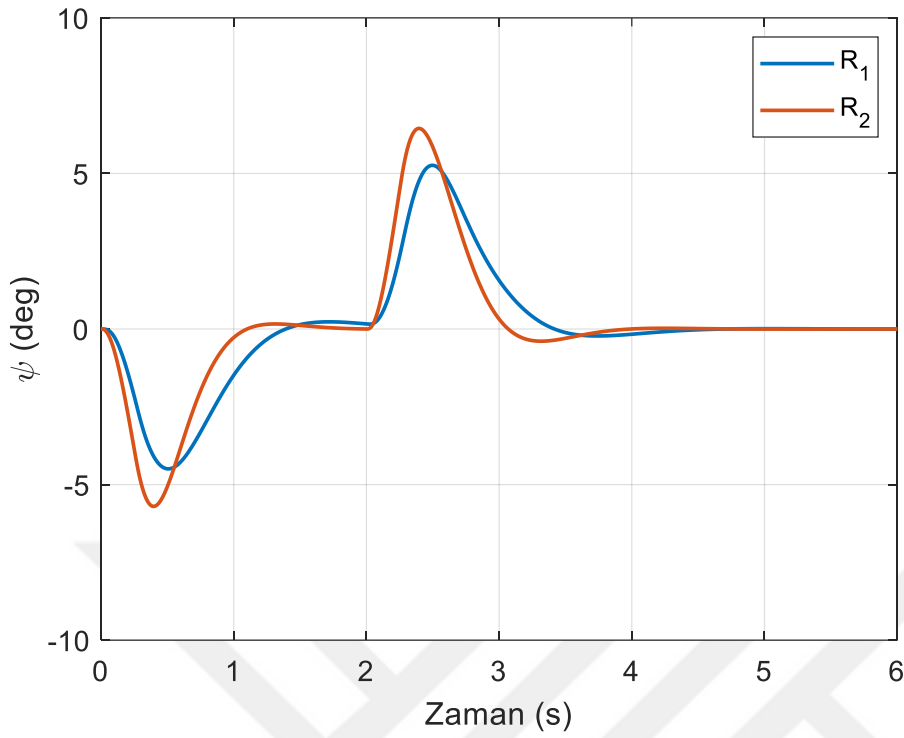
Şekil 6.20. SDRE kontrol yönteminde sıvı çalkalanma büyüklüğü (yörünge I)
