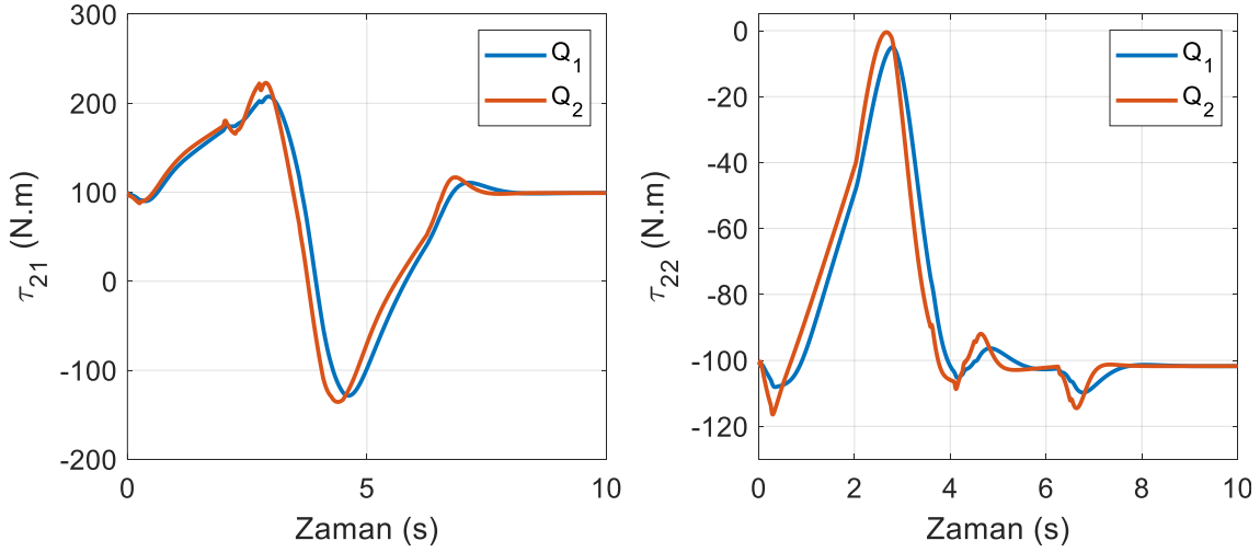
Şekil 6.89. LQR tekniğinde ikinci robotun eklem torkları (yörünge II)
