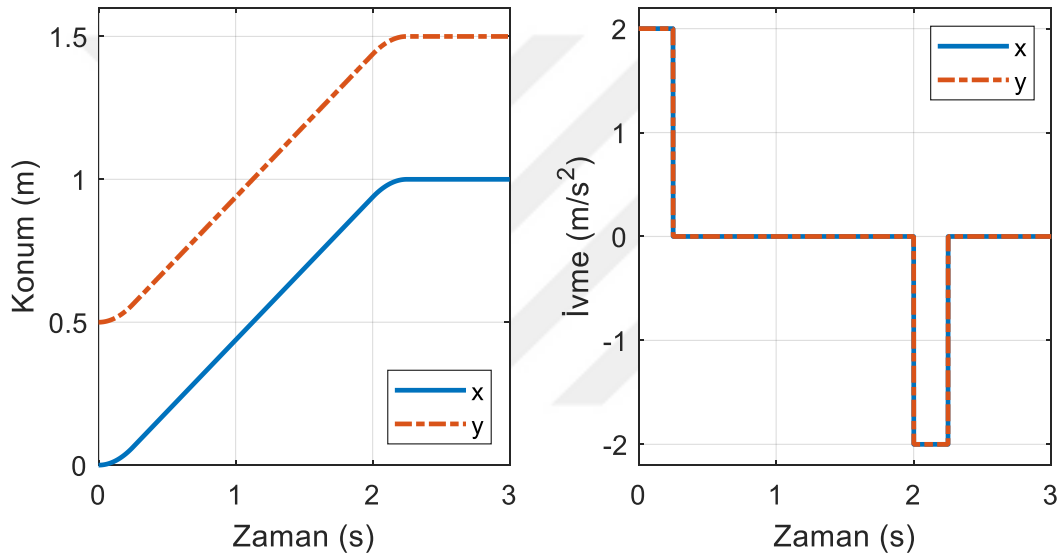
Şekil 6.1. Katı kütle merkezinin izlenmesi istenen yörünge konum-ivme profili
