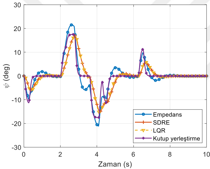
Şekil 6.96. Sıvı çalkalanma büyüklüğü (yörünge II)
