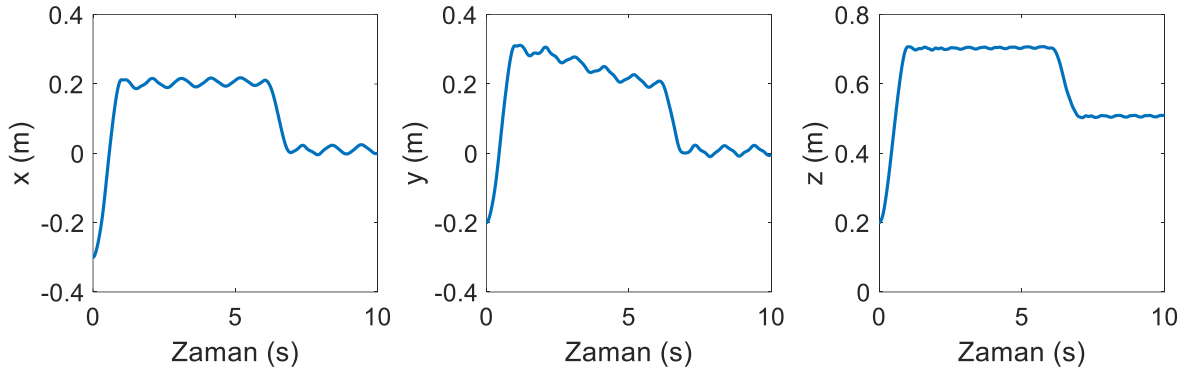
Şekil 6.109. Katı kütlenin ağırlık merkezinin konumu (yörünge II)
