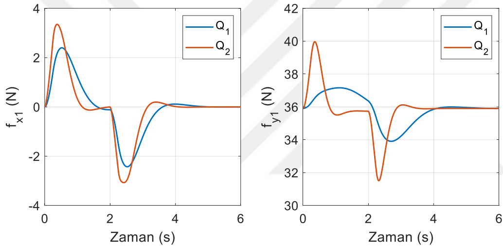
Şekil 6.30. SDRE kontrol yönteminde birinci robot kolundan kaba uygulanan kuvvetler (yörünge I)
