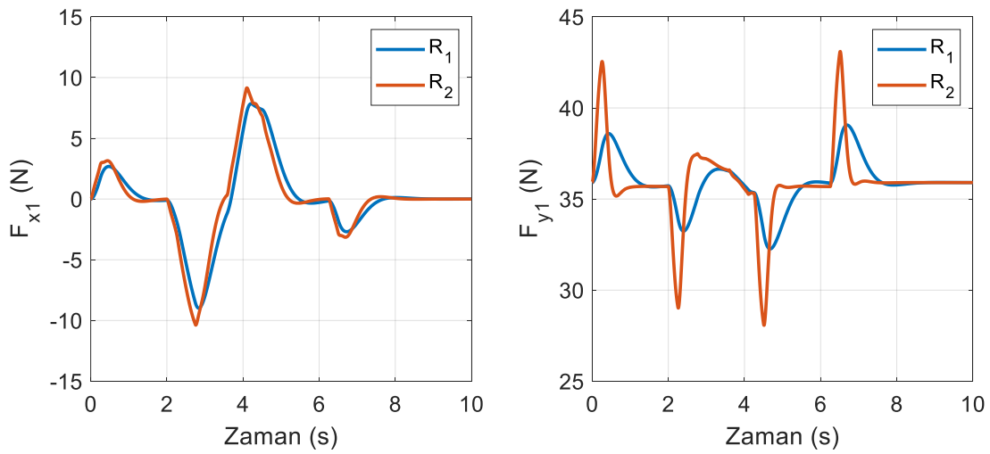
Şekil 6.79. LQR tekniğinde birinci robot kolundan kaba uygulanan kuvvetler (yörünge II)
