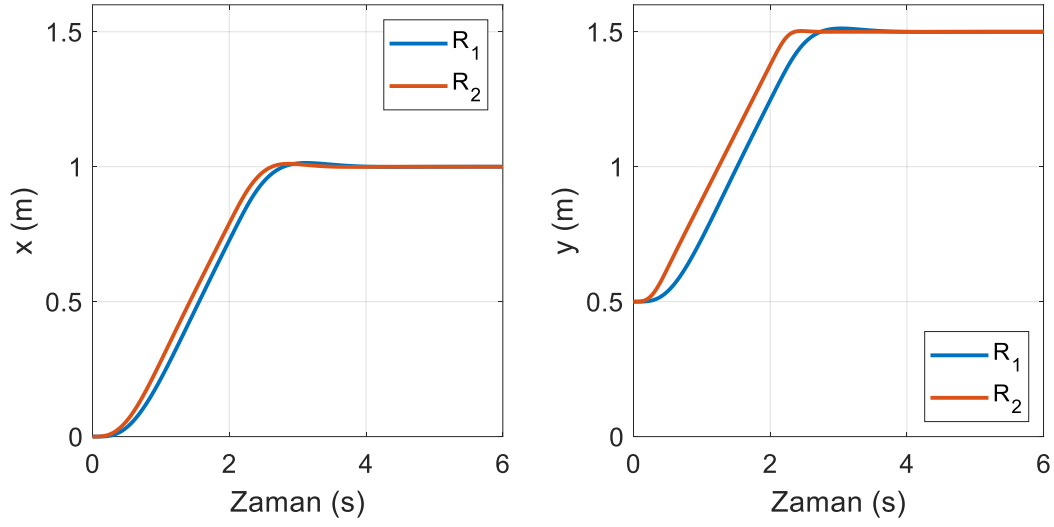
Şekil 6.64. LQR tekniğinde kabın konumu (yörünge I)
