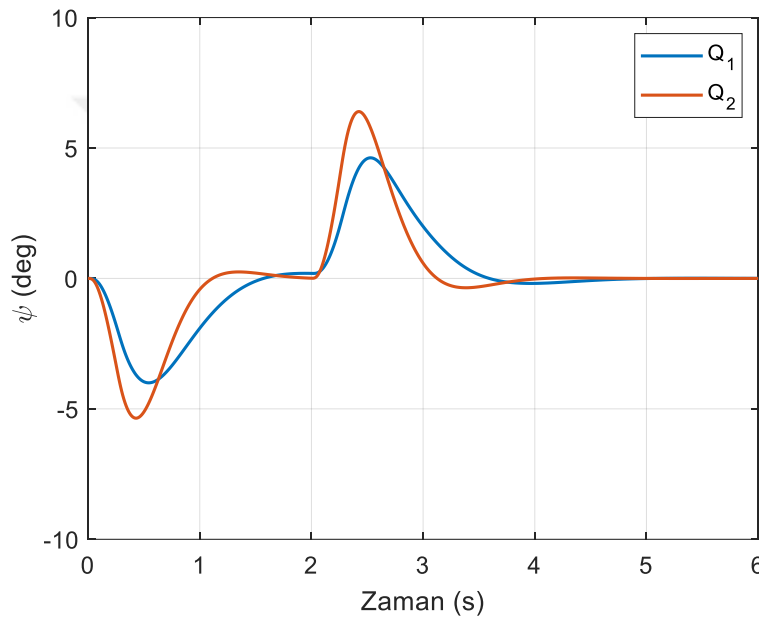
Şekil 6.27. SDRE kontrol yönteminde sıvı çalkalanma büyüklüğü (yörünge I)
