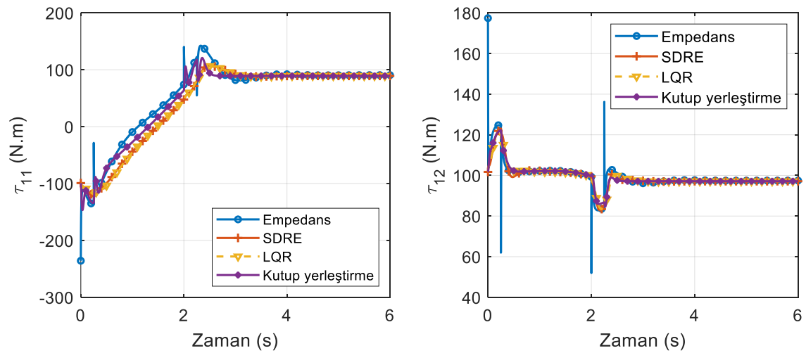
Şekil 6.93. Birinci robot kolun eklem torkları (yörünge I)
