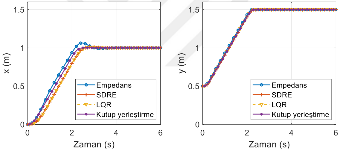
Şekil 6.92. Katı kütlenin ağırlık merkezinin konumu (yörünge I)
