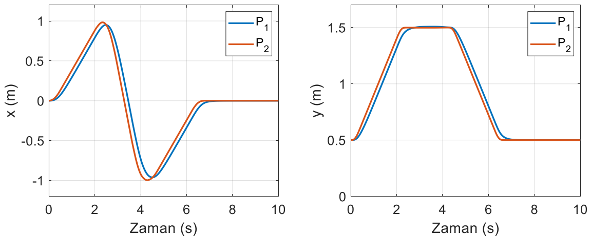
Şekil 6.57. Kutup yerleştirme tekniğinde sıvı kabın konumu (yörünge II)
