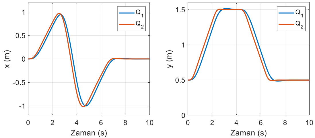
Şekil 6.85. LQR tekniğinde sıvı kabın konumu (yörünge II)
