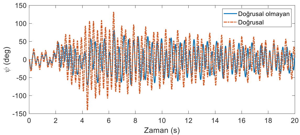
Şekil 6.7. Çalkalanmanın büyüklüğü (Sarkacın açısı)
