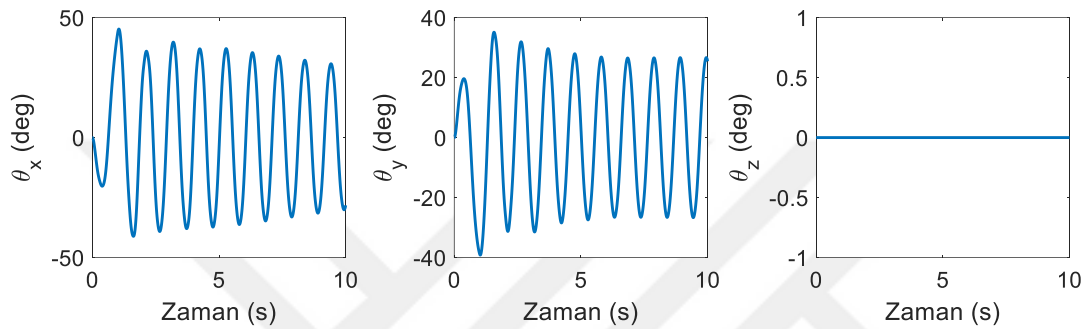
Şekil 6.106. Katı kütlenin oryantasyonu (yörünge I)
