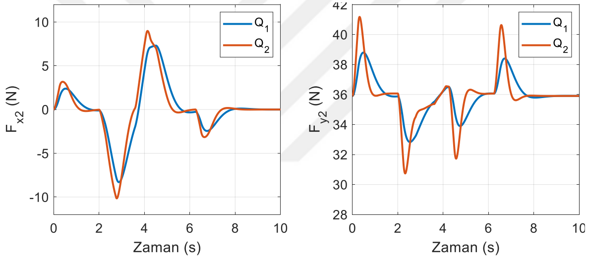
Şekil 6.87. LQR tekniğinde ikinci robot kolundan kaba uygulanan kuvvetler (yörünge II)
