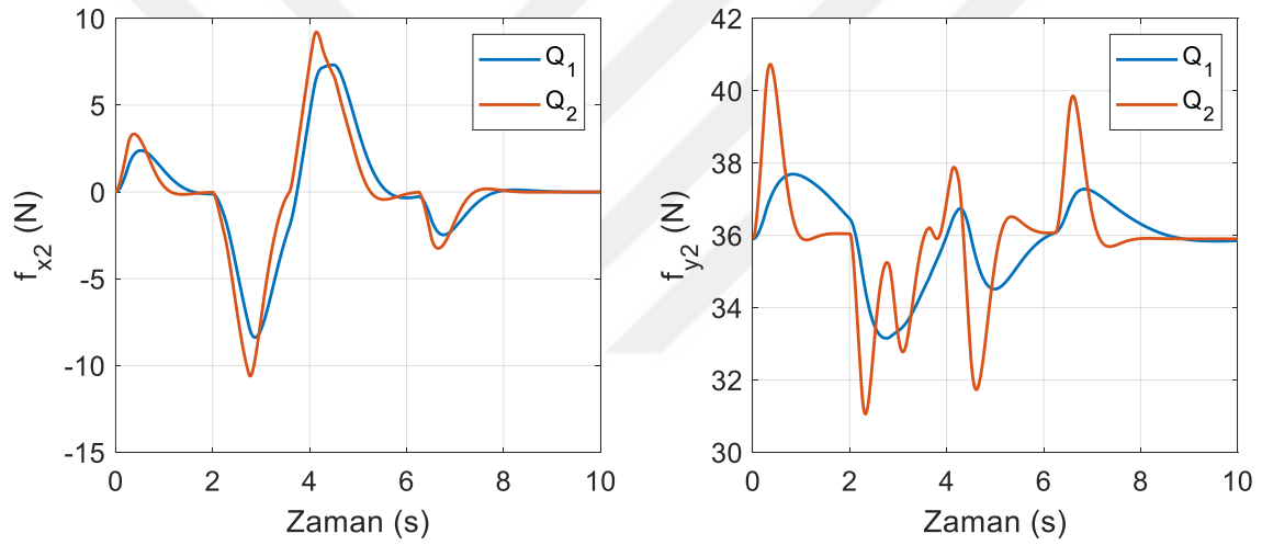
Şekil 6.45. SDRE kontrol yönteminde ikinci robotun kaba uyguladığı kuvvetler (yörünge II)
