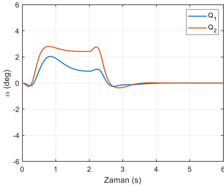
Şekil 6.28. SDRE kontrol yönteminde sıvı kabın açısı (yörünge I)
