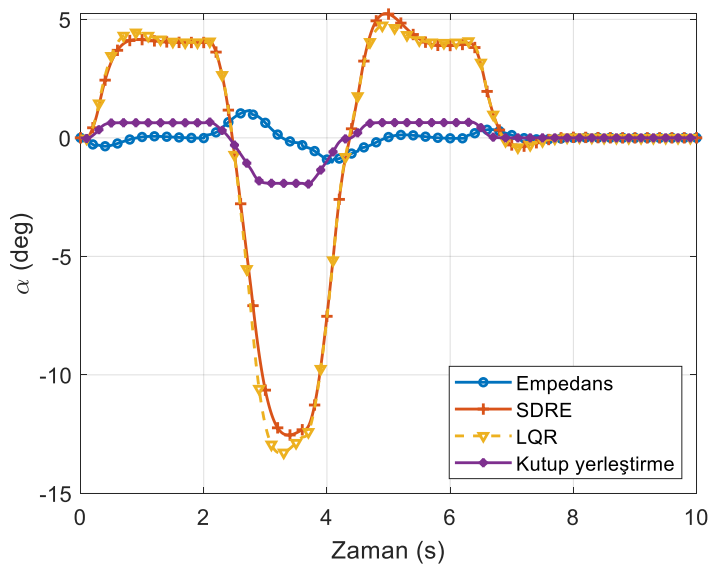
Şekil 6.97. Kabın açısı (yörünge II)
