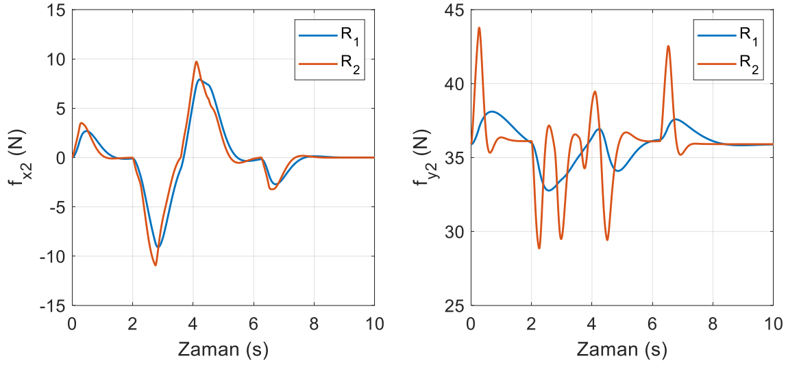
Şekil 6.38. SDRE kontrol yönteminde ikinci robotun kaba uyguladığı kuvvetler (yörünge II)
