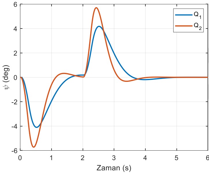
Şekil 6.69. LQR tekniğinde sıvı çalkalanma büyüklüğü (yörünge I)
