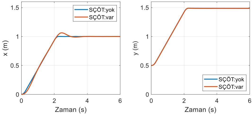
Şekil 6.12. Empedans kontrol yönteminde katı kütlenin ağırlık merkezinin konumu (yörünge I)
