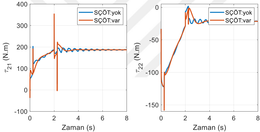
Şekil 6.14. Empedans kontrol yönteminde ikinci robotun eklem torkları (yörünge I)
