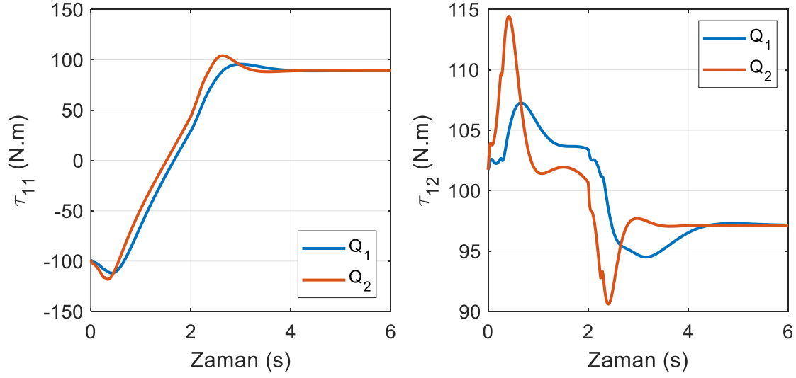
Şekil 6.32. SDRE kontrol yönteminde birinci robotun eklem torkları (yörünge I)
