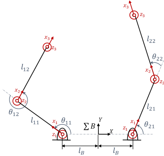
Şekil 3.3. İki düzlemsel robot
