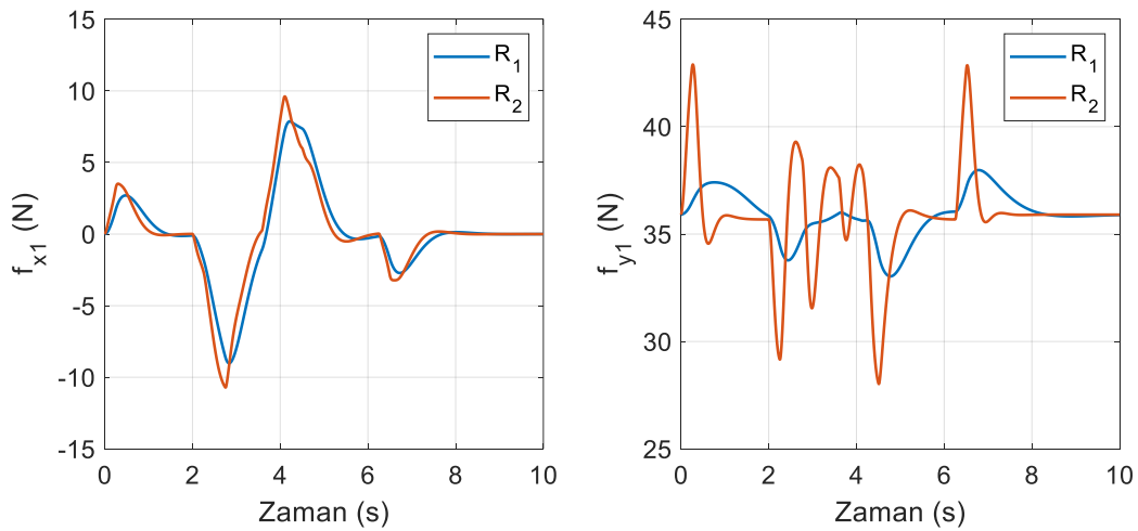
Şekil 6.37. SDRE kontrol yönteminde birinci robotun kaba uyguladığı kuvvetler (yörünge II)
