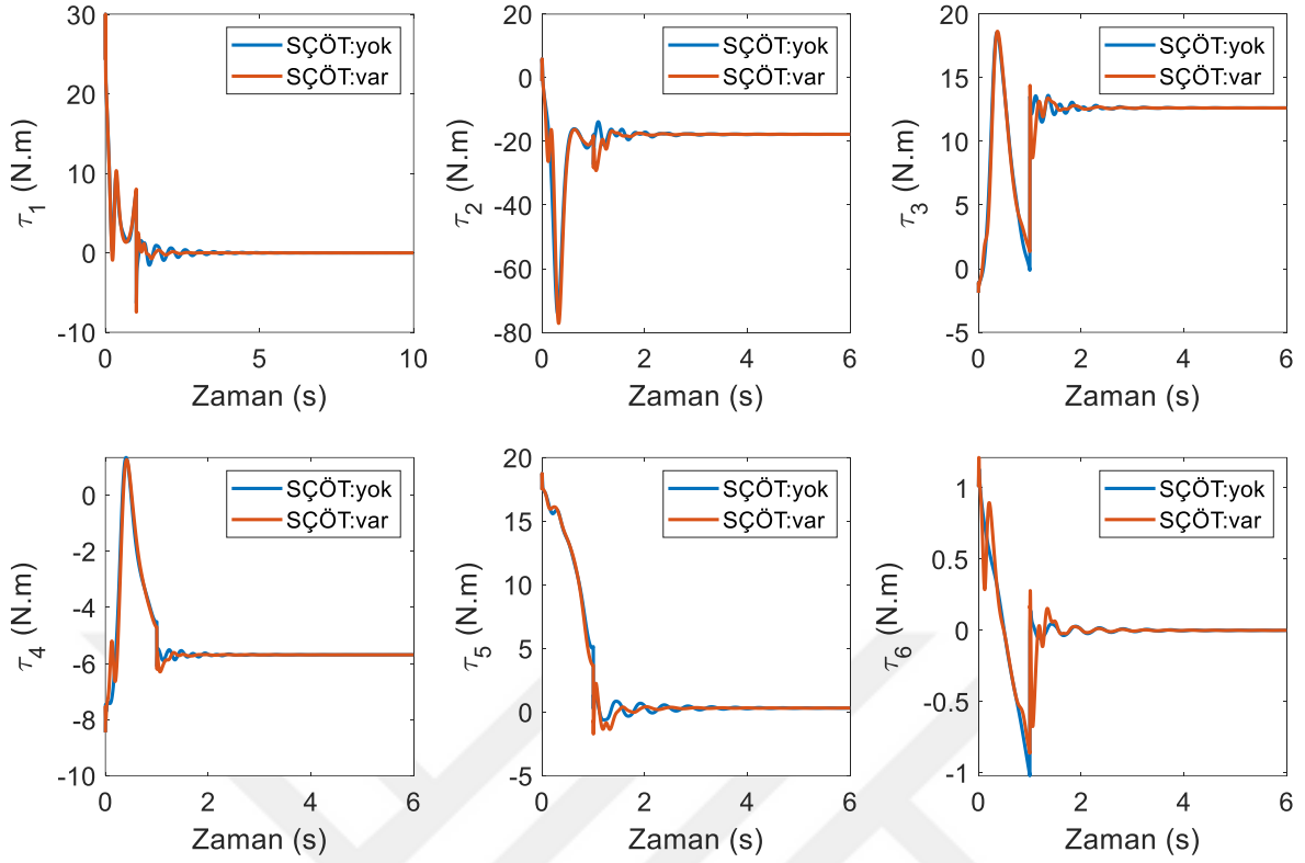
Şekil 6.114. Empedans kontrol yönteminde birinci robotun eklem torkları (yörünge I)
