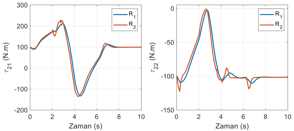
Şekil 6.82. LQR tekniğinde ikinci robotun eklem torkları (yörünge II)
