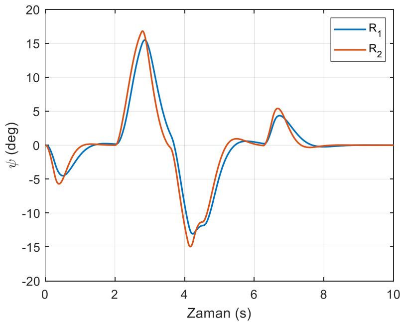
Şekil 6.34. SDRE kontrol yönteminde sıvı çalkalanma büyüklüğü (yörünge II)
