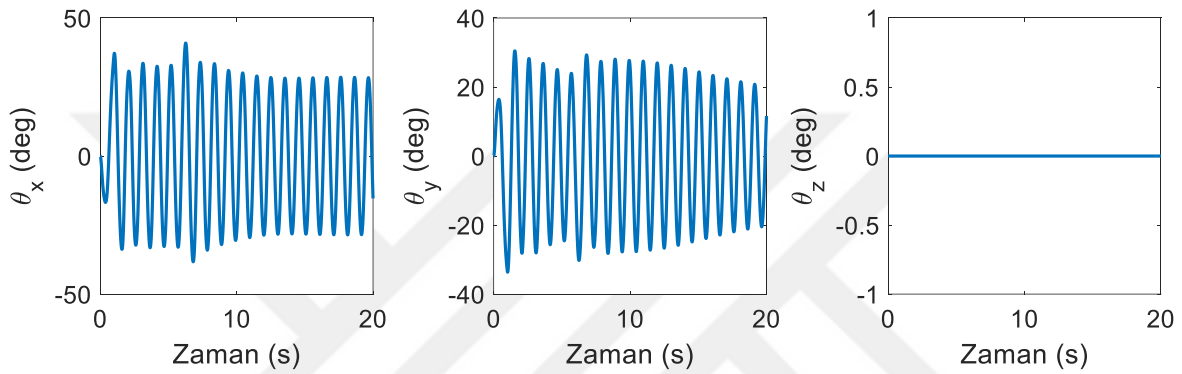
Şekil 6.110. Katı kütlenin oryantasyonu (yörünge II)
