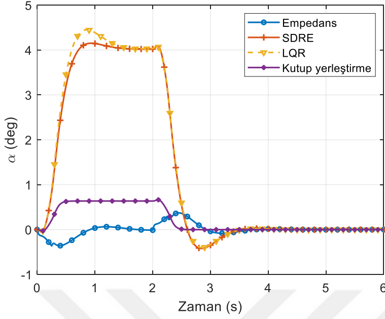
Şekil 6.91. Kabın açısı (yörünge I)
