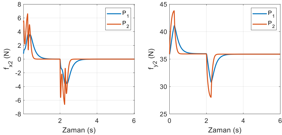
Şekil 6.52. Kutup yerleştirme tekniğinde ikinci robot kolundan kaba uygulanan kuvvetler (yörünge I)
