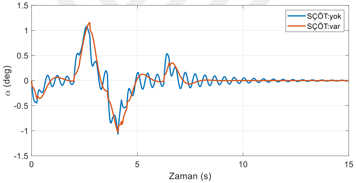
Şekil 6.16. Empedans kontrol yönteminde kap açısı (yörünge II)
