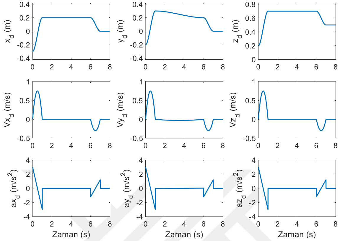
Şekil 6.107. Katı kütlelinin ağırlık merkezinin izlenmesi istenen çoklu hareket profili
