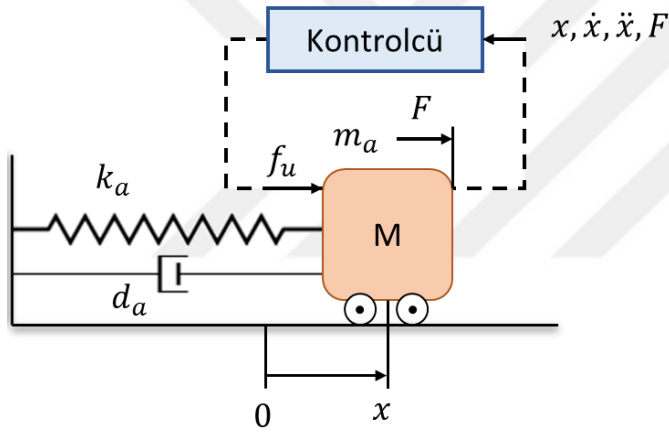
Şekil 2.3. Bir serbestlik dereceli sistemin aktif empedans kontrolü [118]
