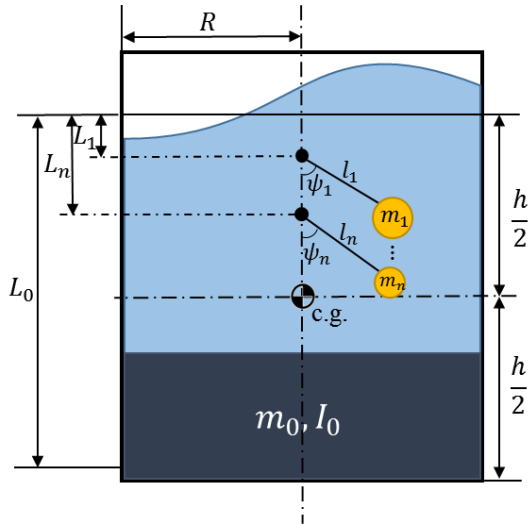
Şekil 2.2. Sarkaç modeli [116]
