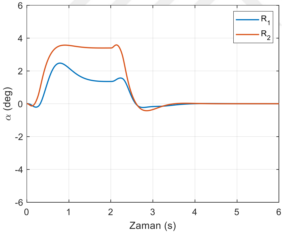
Şekil 6.21. SDRE kontrol yönteminde kabın açısı (yörünge I)
