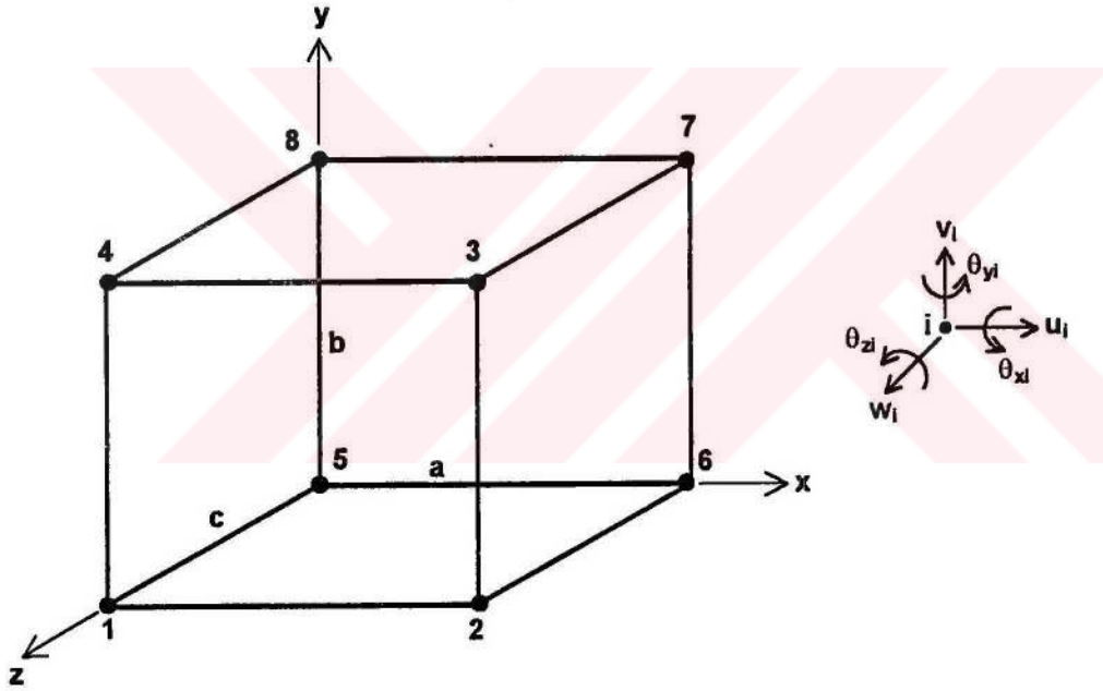
Şekil D.1. Üç boyutlu geçiş elemanı ve düğüm deplasmanları
