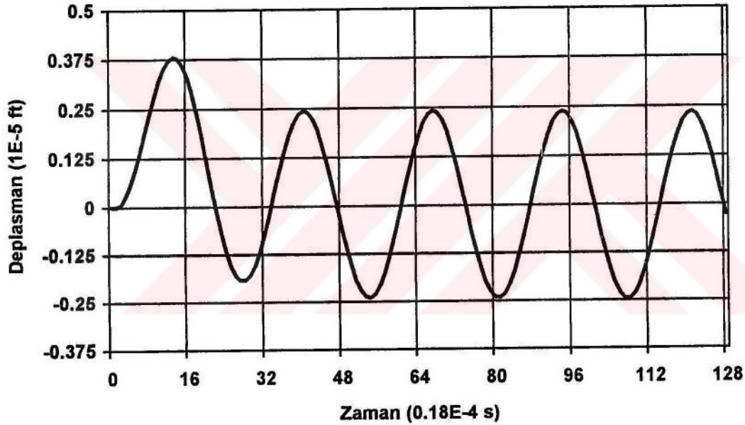
Şekil 4.36. Sinüzoidal yükten dolayı düşey deplasmanın zamanla değişimi
