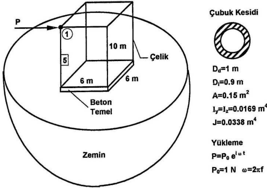
Şekil 4.22. Elastik zemin üzerinde tek katlı çerçeve
