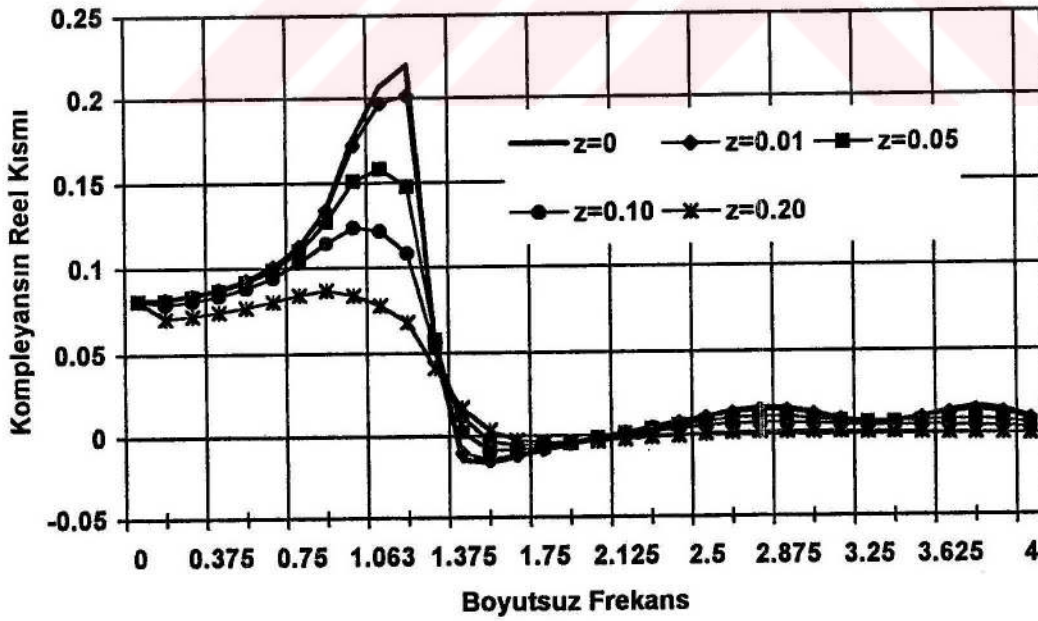
Şekil 4.20. Düşey komplemansın reel kısmının sönüm ile değişimi
