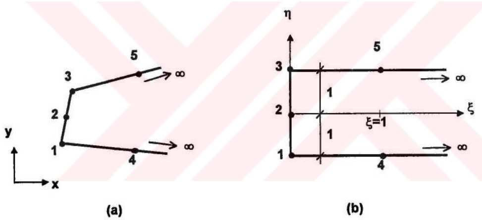
Şekil 3.8. 5 düğümlü sonsuz eleman (a) Gerçek eleman (b) Referans elemanı
