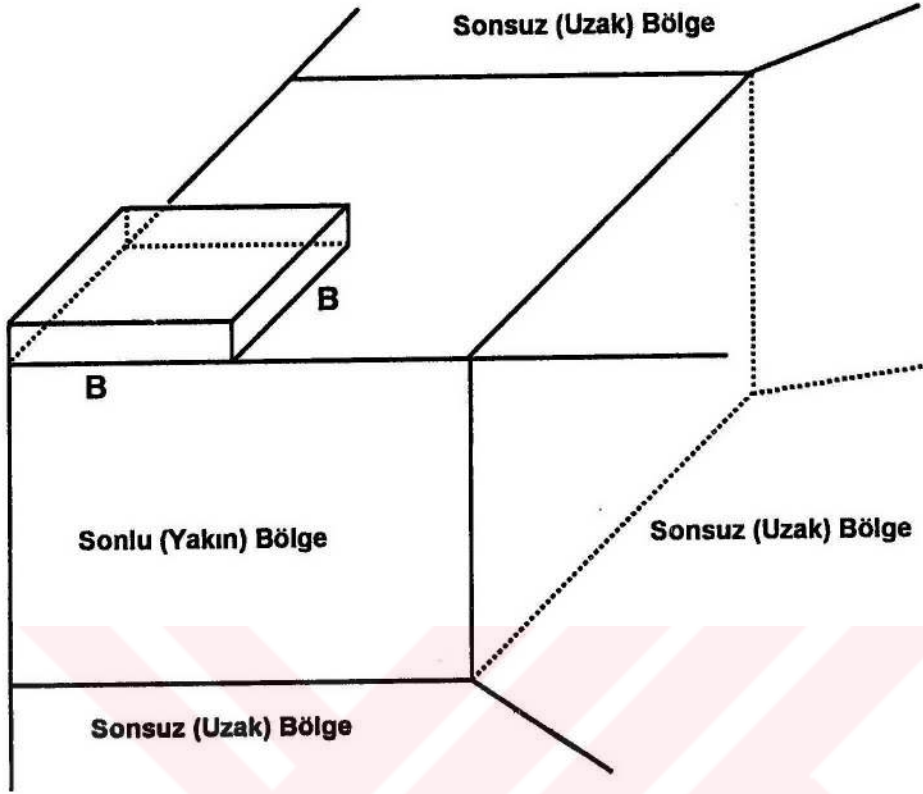
Şekil 4.9. Elastik zemin üzerinde kare temel (1/4 bölge)
