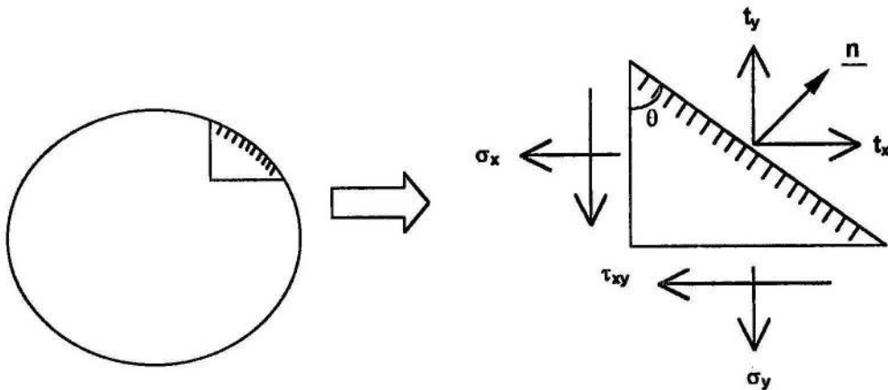
Şekil 3.1. Sınır şartları
