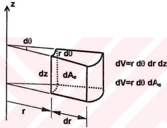
Şekil 3.4. Eksenel simetrik sonlu eleman
