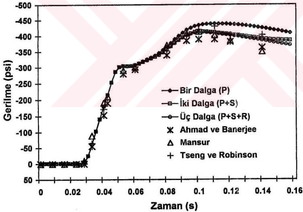
Şekil 3.28. B noktasındaki düşey gerilmenin zamanla değişimi
