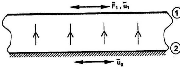
Şekil 5.3. Yer hareketine maruz zemin tabakası
