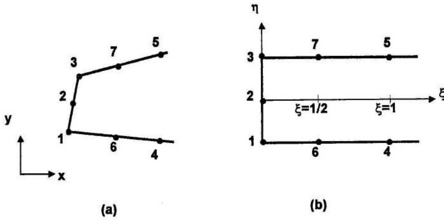
Şekil 3.10. 7 düğümlü sonsuz eleman (a) Gerçek eleman (b) Referans elemanı
