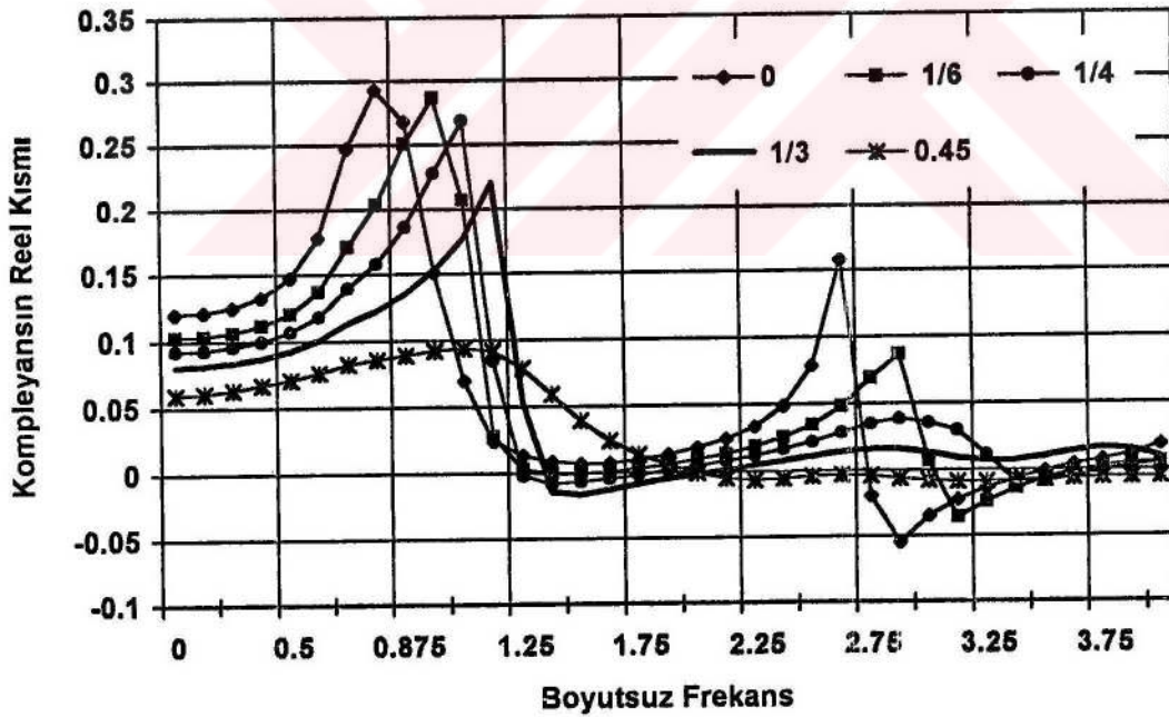
Şekil 4.18. Düşey kompleyansın reel kısmının Poisson oranı ile değişimi
