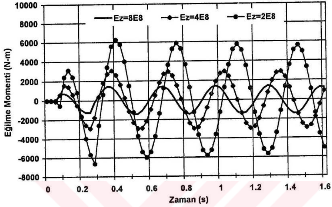
Şekil 4.49. Eğilme momentinin zemin rijitliği ile değişimi
