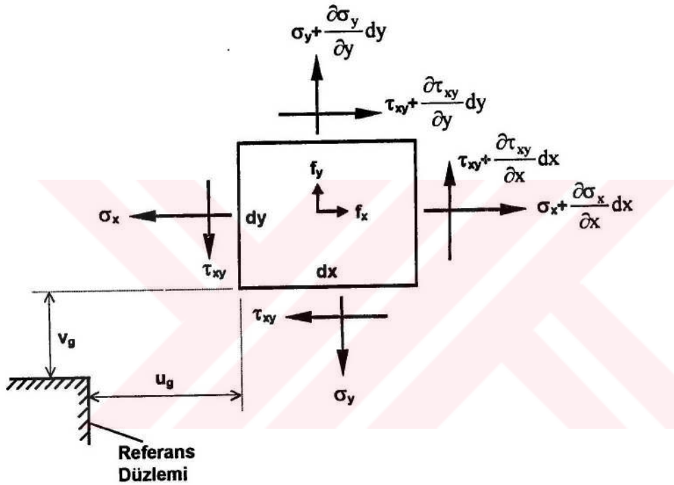
Şekil 5.1. Elemaner düzlem elemanı serbest cisim diyagramı
