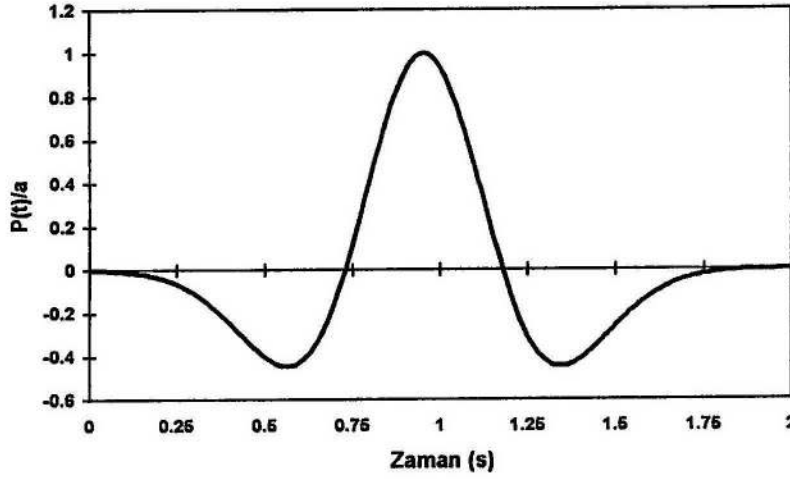
Şekil 3.42. Ricker Wavelet yüklemesi
