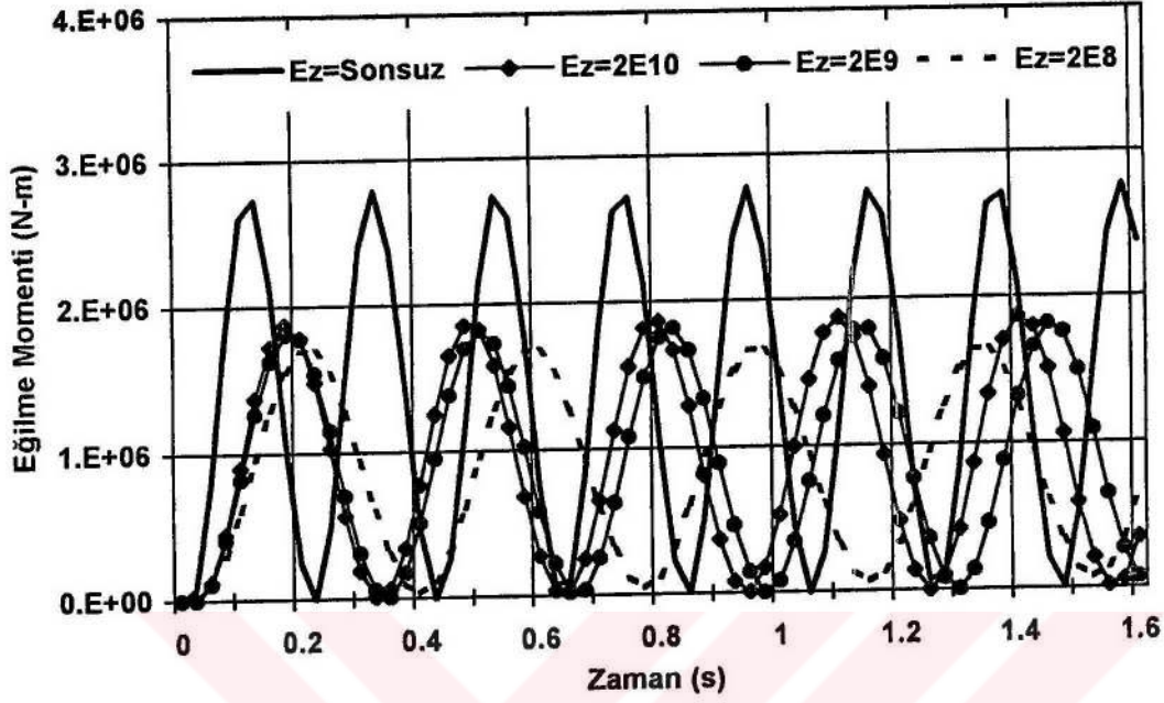
Şekil 4.42. Eğilme momentinin zamanla değişimi
