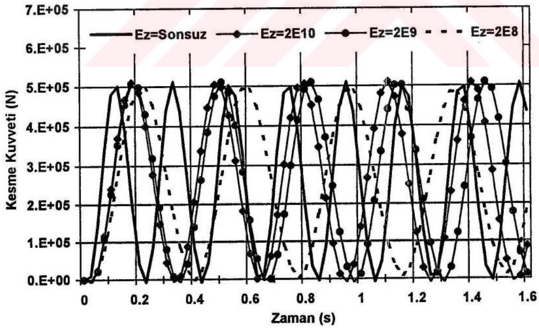
Şekil 4.41. Kesme kuvvetinin zamanla değişimi
