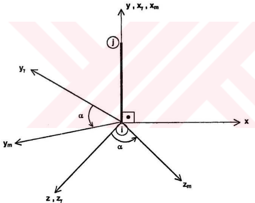
Şekil C.3. Düşey konumdaki çubuk elemanın transformasyonu
