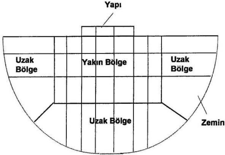
Şekil 3.6. Yapı-zemin etkileşim modeli
