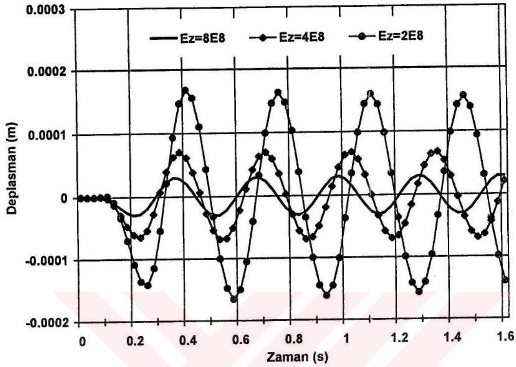
Őekil 4.47. Yatay deplasmanın zemin rijitliđi ile deđiŐimi
