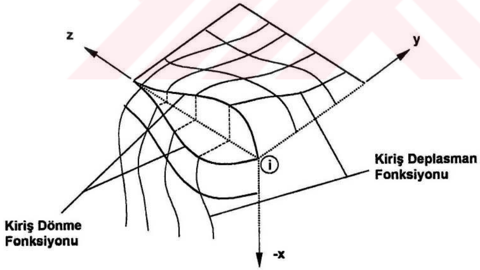
v deplasmanının dağılımı
