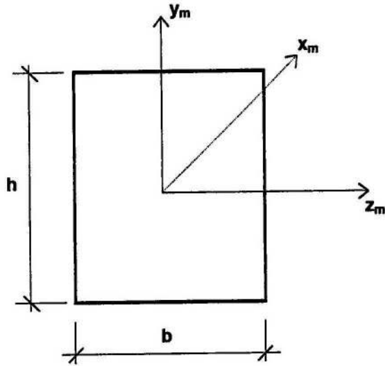
Şekil 4.4. Dikdörtgen kesitli çubuk
