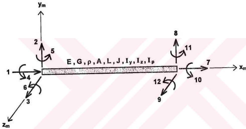
Şekil 4.2. Üç boyutlu prizmatik çubuk eleman
