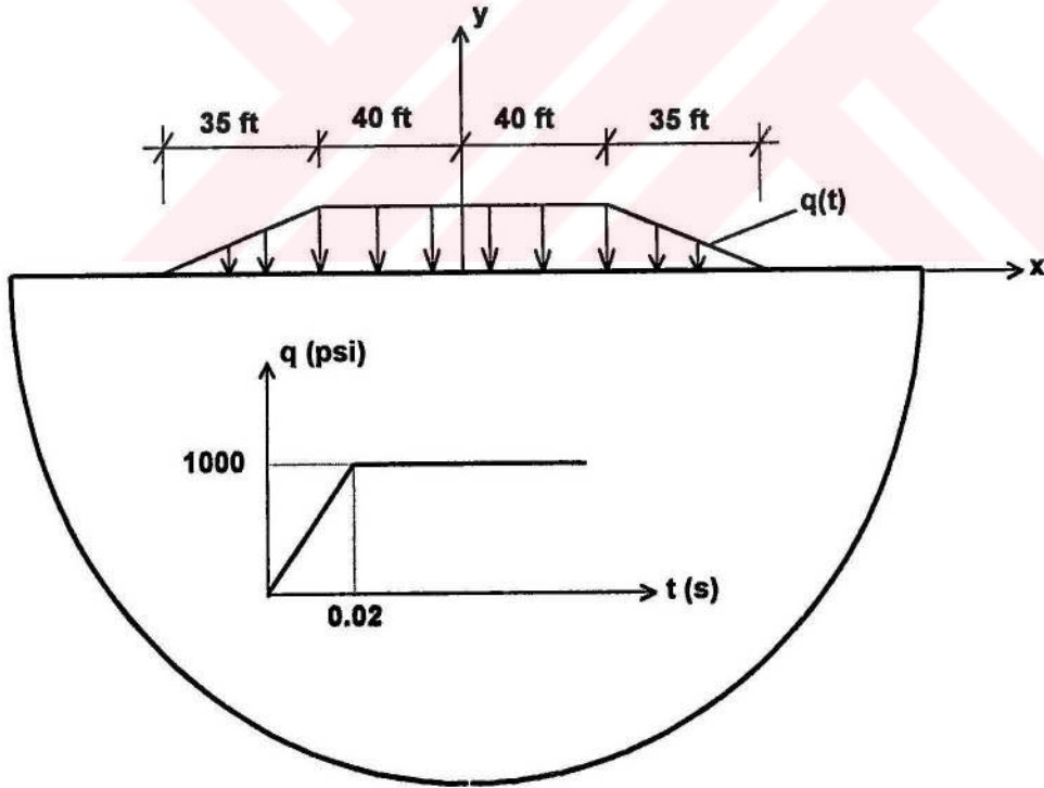
Şekil 3.26. Trapez yüklemeye maruz yarı sonsuz zemin
