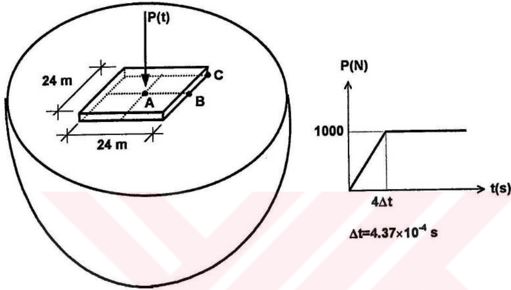
Şekil 4.37. Esnek kare temelin geometrisi ve yüklemesi
