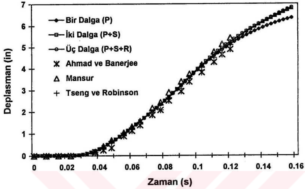
Şekil 3.31. F noktasındaki düşey deplasmanın zamanla değişimi
