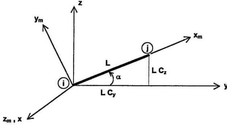
Şekil C.6. z_m // x durumu
