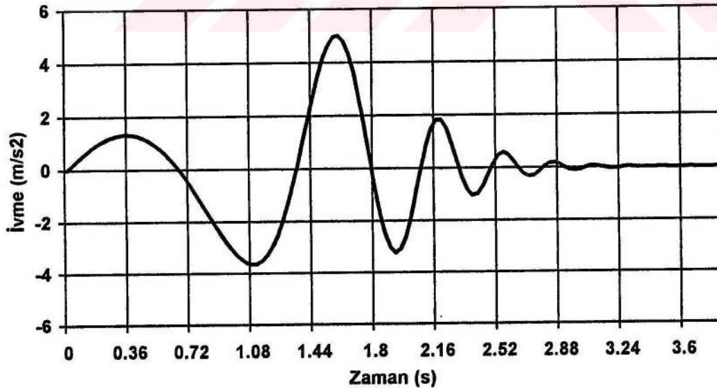
Şekil 5.4. Zemin tabanına etkiyen ivmenin zamanla değişimi
