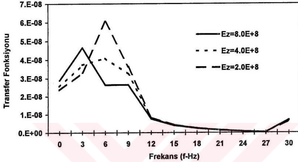
Şekil 4.26. Deplasman transfer fonksiyonunun zemin rijitliğiyle değişimi
