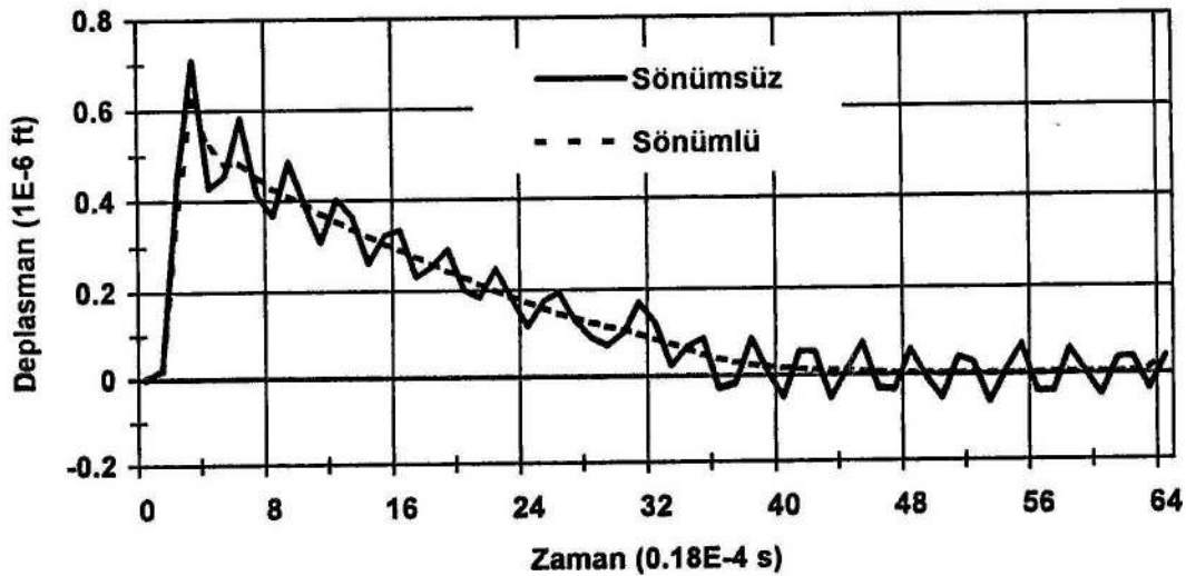
Şekil 4.35. Temelin altındaki deplasmanın zamanla değişimi
