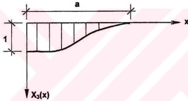
Şekil D.4. Kiriş deplasman fonksiyonu
