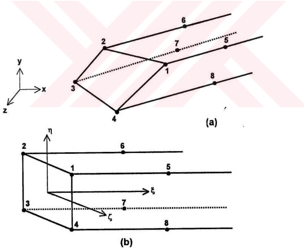
Şekil 4.6. 8 düğümlü sonsuz eleman (a) Gerçek eleman (b) Referans elemanı
