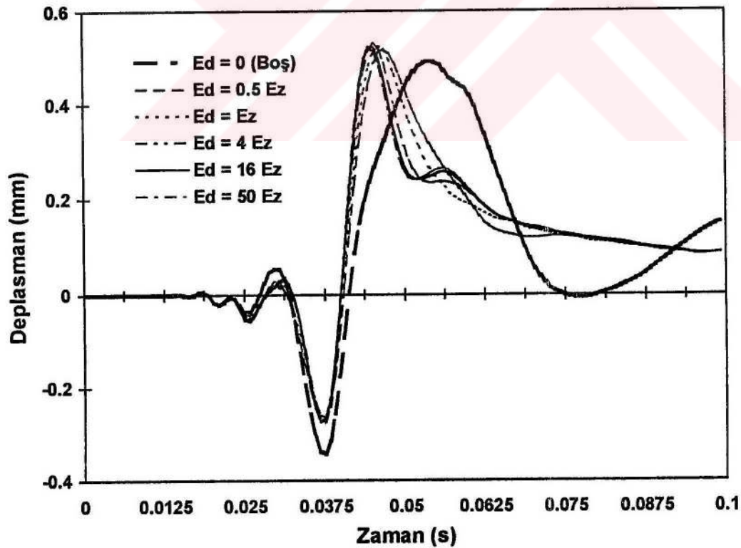
Şekil 3.38. Çeşitli dolgu malzemeleri için A noktasının deplasmanı
