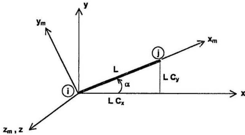
Şekil C.4. z_m // z durumu
