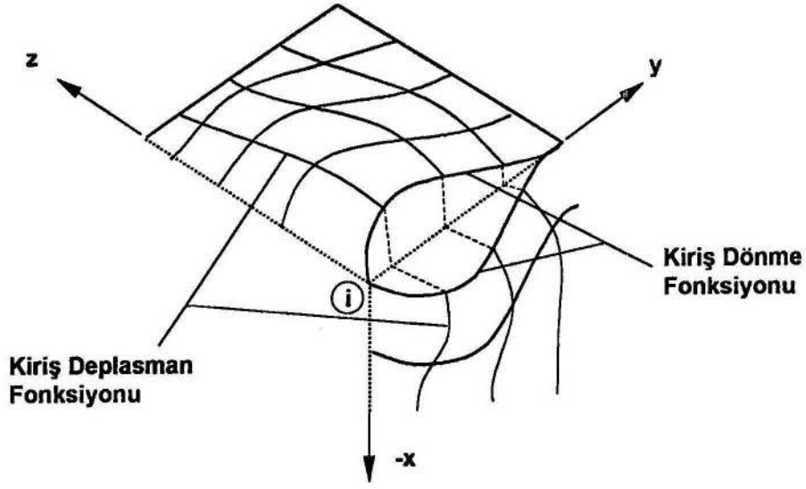
w deplasmanının dağılımı
