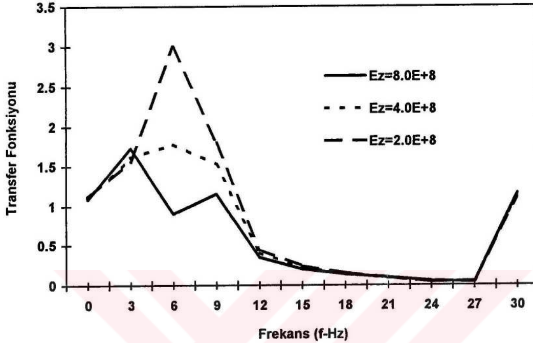
Şekil 4.28. Eğilme momenti transfer fonksiyonunun zemin rijitliğiyle değişimi
