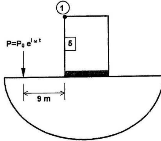
Şekil 4.29. Elastik zemin üzerinde tek katlı çerçeve (karşıdan görünüş)
