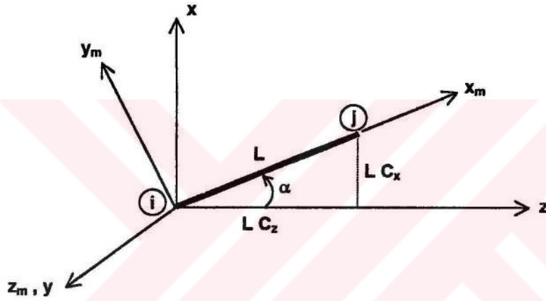
Şekil C.5. z_m // y durumu
