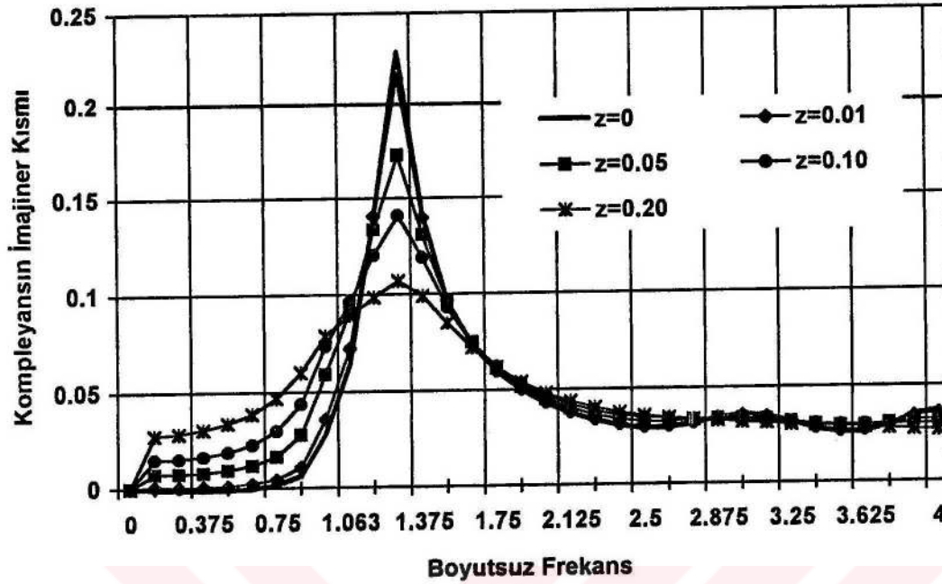
Şekil 4.21. Düşey komplekansın imajiner kısmının sönüm ile değişimi
