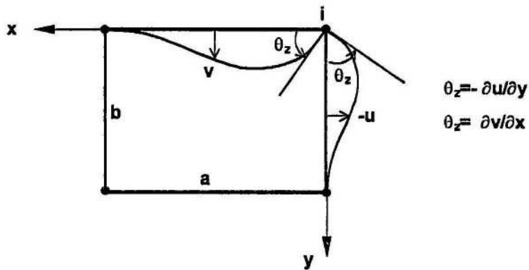
Şekil D.7. \theta_z dönmesi durumu
