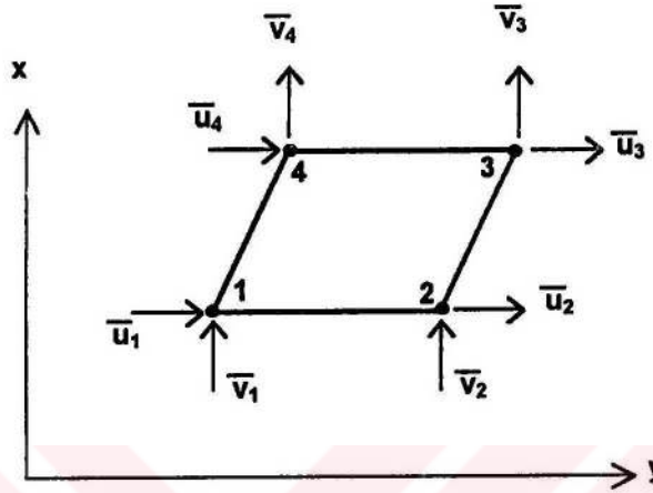
Şekil 3.2. Tipik bir sonlu eleman
