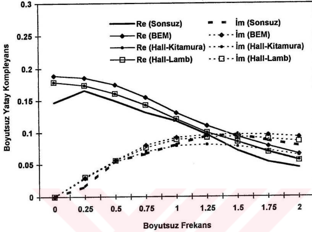
Şekil 4.11. Boyutsuz yatay kompleyansın frekans ile değişimi
