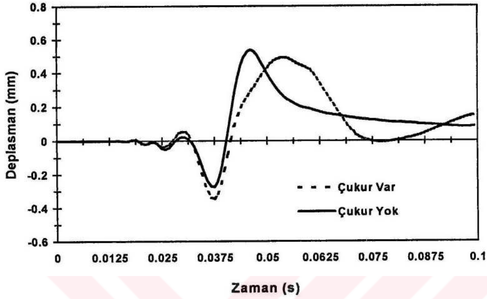
Şekil 3.36. A noktası için titreşim izolasyonu
