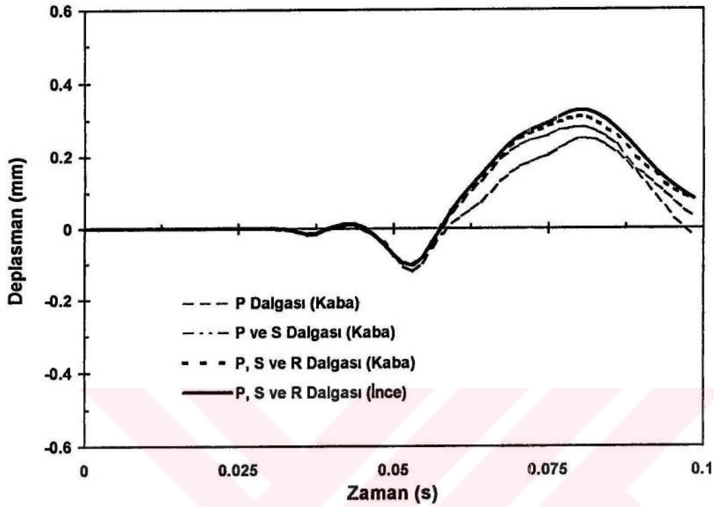
Şekil 3.35. B noktasının (çukurun ötesinde) düşey deplasmanı
