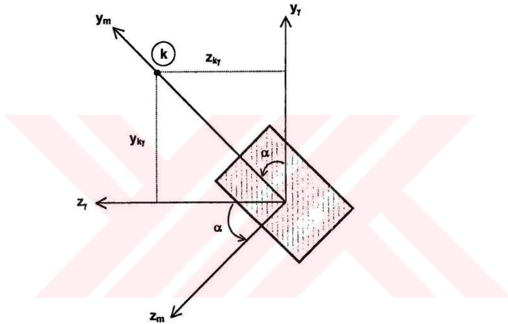
Şekil C.2. Üç boyutlu çubuğun x_m eksenini etrafındaki dönmesi
