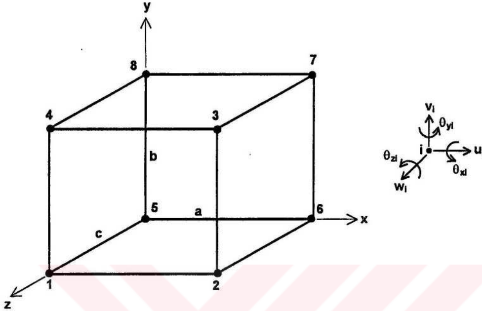
Şekil 4.5. Üç boyutlu geçiş elemanı (Rotational brick)
