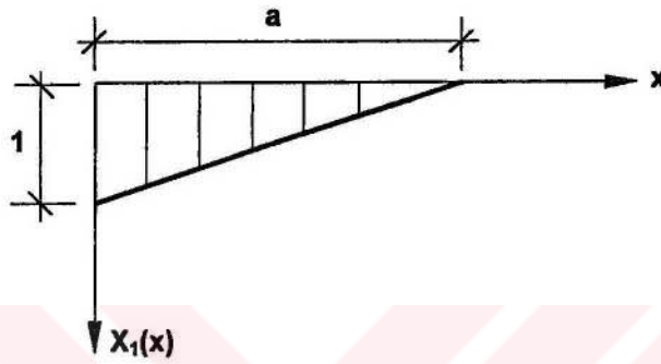
Şekil D.2. Lineer deplasman fonksiyonu
