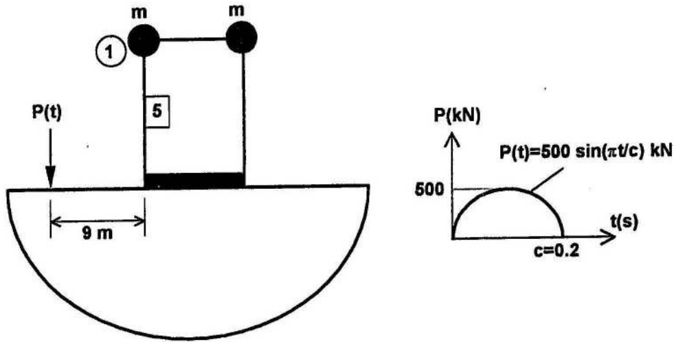
Şekil 4.43. Elastik zemin üzerinde çerçeve (karşıdan görünüş) ve yüklemesi
