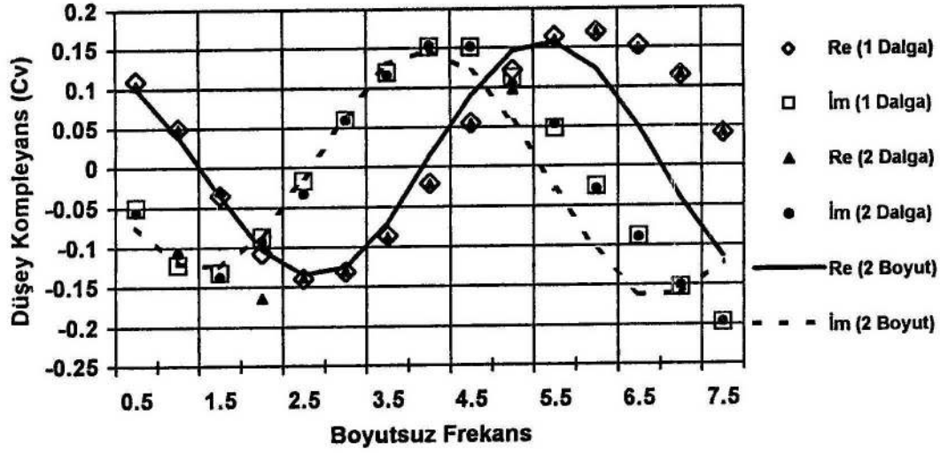
Şekil 4.8. Düşey komplekansın frekansla değişimi
