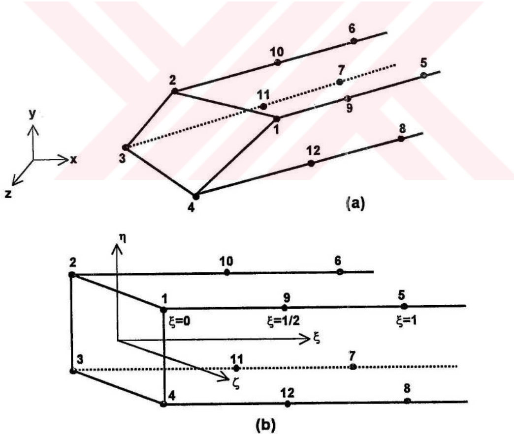
Şekil 4.7. 12 düğümlü sonsuz eleman (a) Gerçek eleman (b) Referans elemanı
