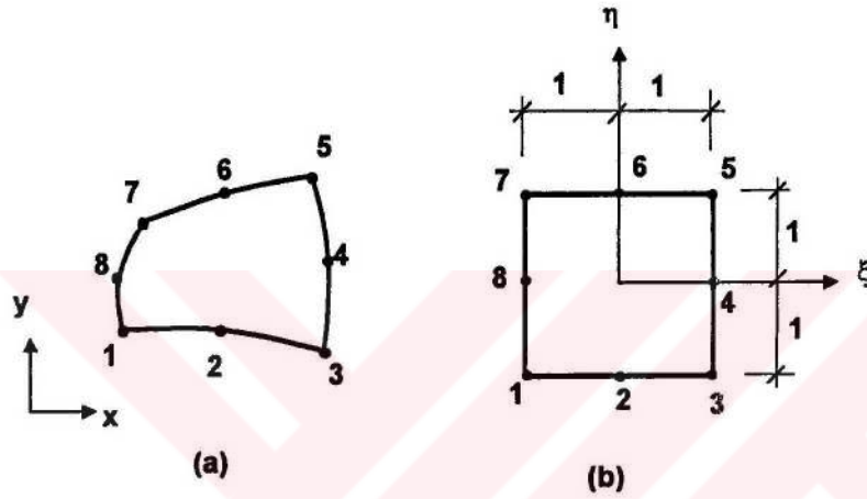
Şekil 3.3. 8 düğümlü izoparametrik, kuadratik sonlu eleman (a) Gerçek eleman (b) Referans elemanı
