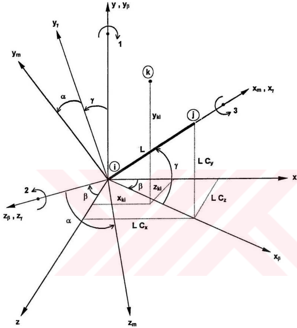
Şekil C.1. Üç boyutlu çubuğun eksenlerinin döndürülmesi
