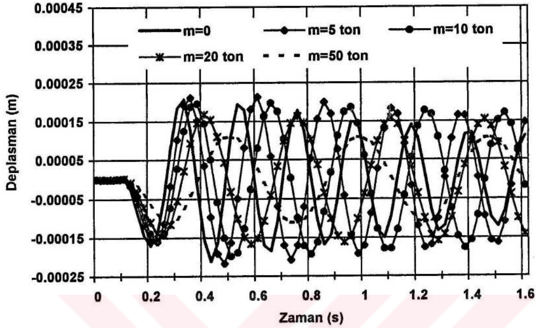
Şekil 4.44. Yatay deplasmanın kütle ile değişimi
