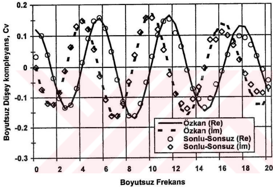
Şekil 3.17. Boyutsuz düşey komplemansın boyutsuz frekansla değişimi
