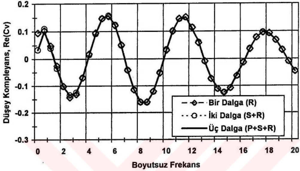
Şekil 3.15. Düşey komplemansın reel kısmı
