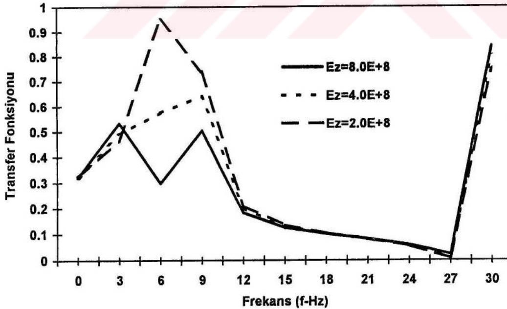
Şekil 4.27. Kesme kuvveti transfer fonksiyonunun zemin rijitliğiyle değişimi
