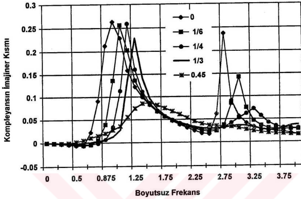
Şekil 4.19. Düşey komplemansın imajiner kısmının Poisson oranı ile değişimi
