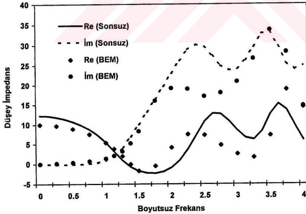
Şekil 4.16. Boyutsuz düşey impedansın karşılaştırılması
