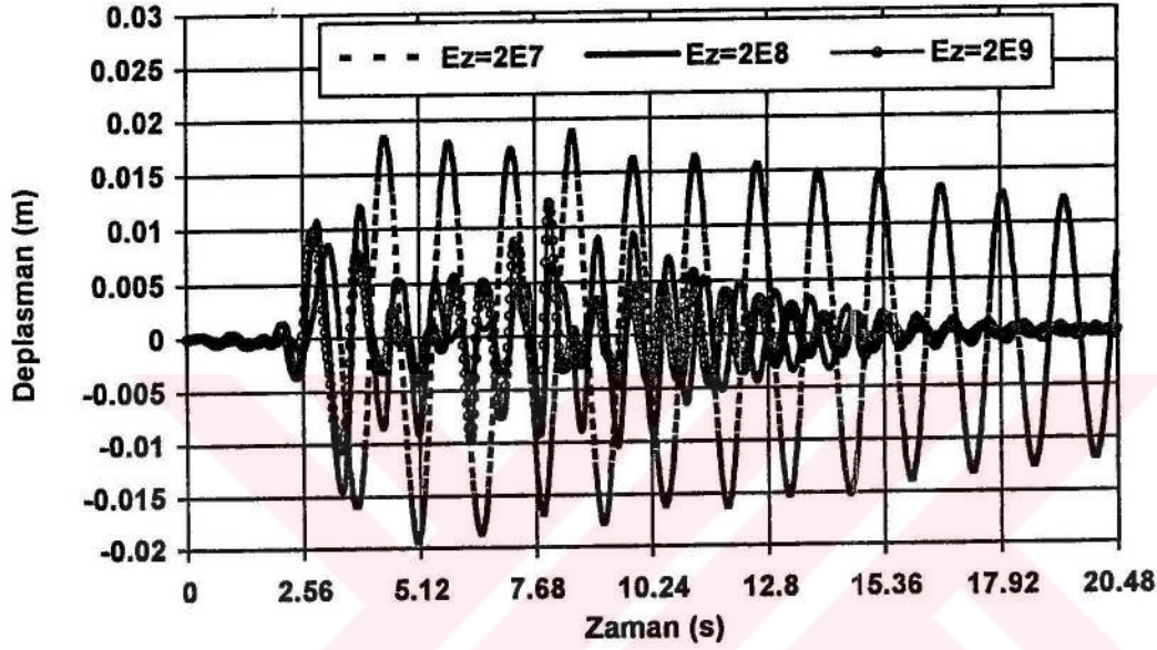
Şekil 5.16. Yatay deplasmanın zeminin rijitliği ile değişimi
