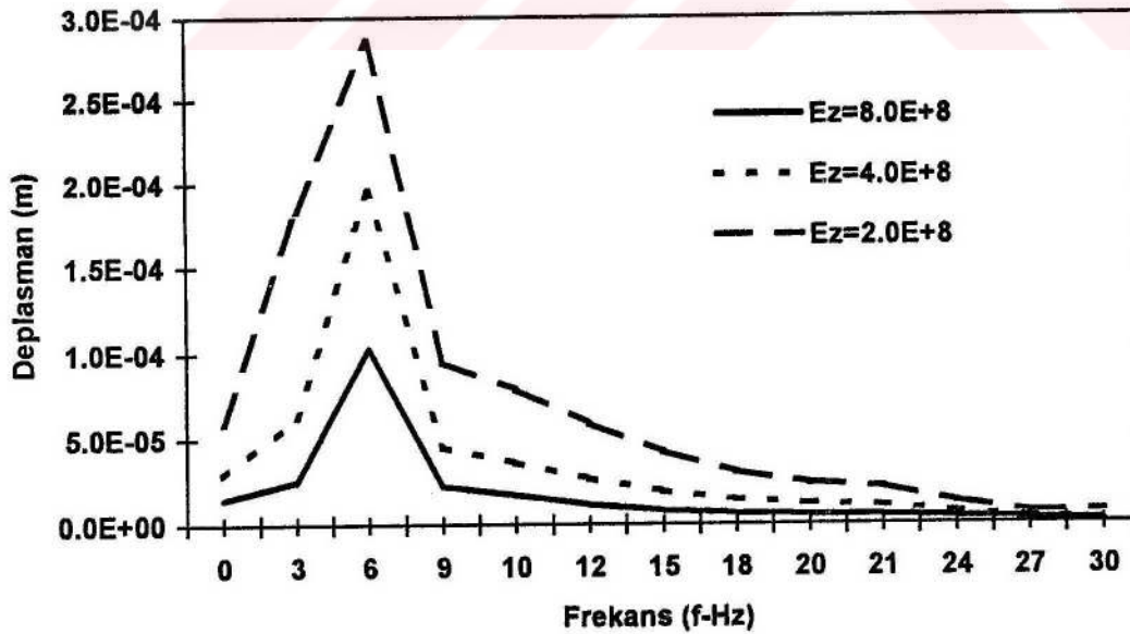
Şekil 4.30. Yatay deplasmanın frekansla değişimi
