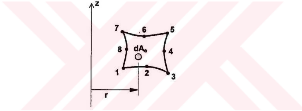
Şekil 3.5. 8 düğümlü, kuadratik sonlu eleman
