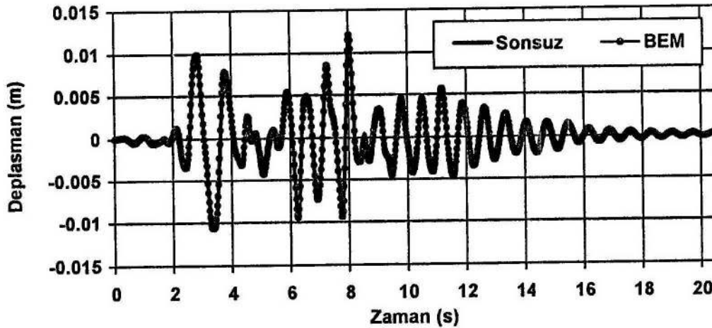
Şekil 5.15. Değişik impedanslarla bulunan deplasmanın karşılaştırılması
