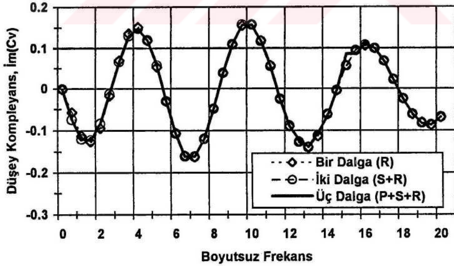
Şekil 3.16. Düşey komplemansın imajiner kısmı
