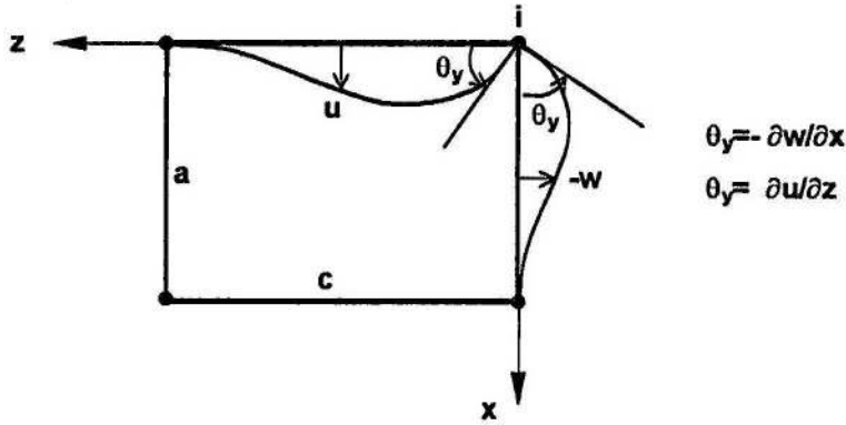
Şekil D.6. \theta_y dönmesi durumu
