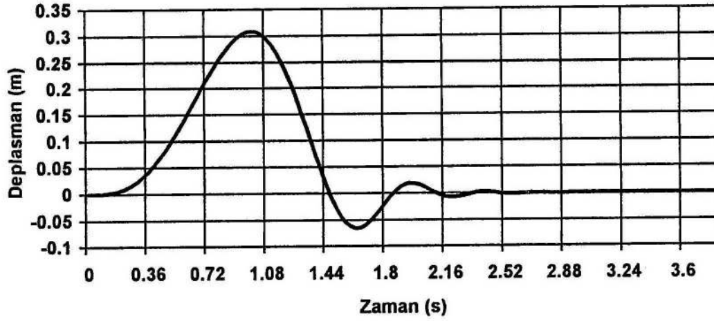
Şekil 5.5. Zemin tabanına etkiyen deplasmanın zamanla değişimi
