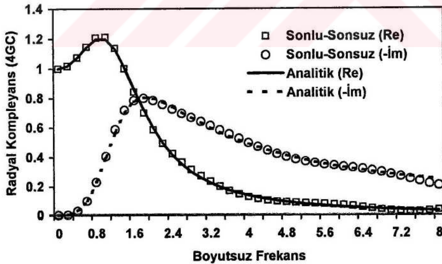
Şekil 3.13. Radyal kompleyansın boyutsuz frekansla değişimi
