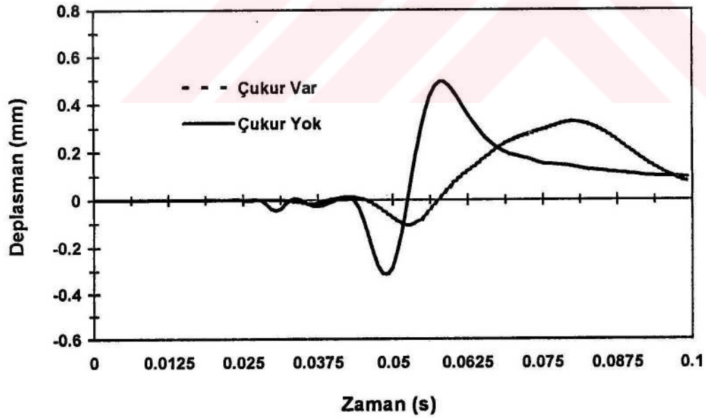
Şekil 3.37. B noktası için titreşim izolasyonu
