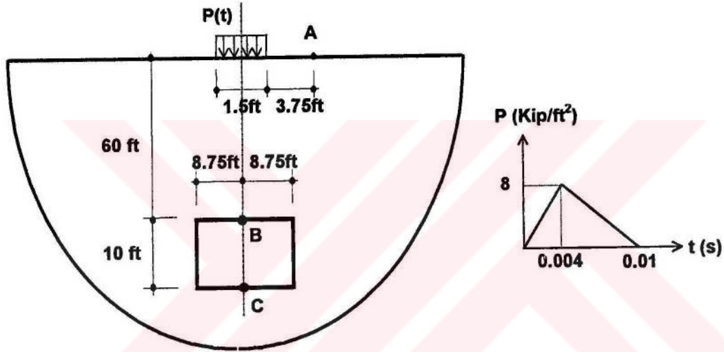
Şekil 3.40. Yarı sonsuz zemin içinde tünel, geometrisi ve yüklemesi
