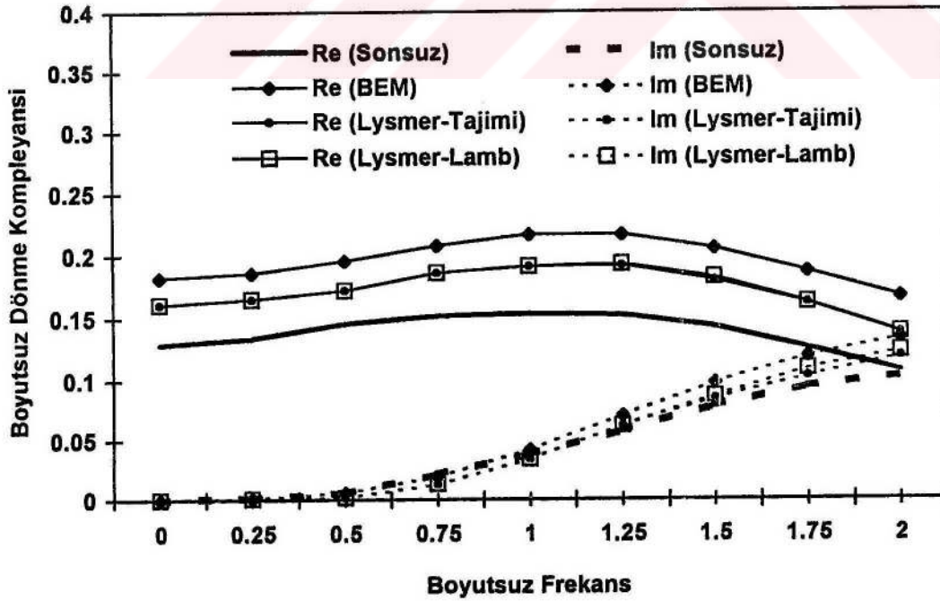
Şekil 4.12. Boyutsuz dönme kompleyansının frekans ile değişimi
