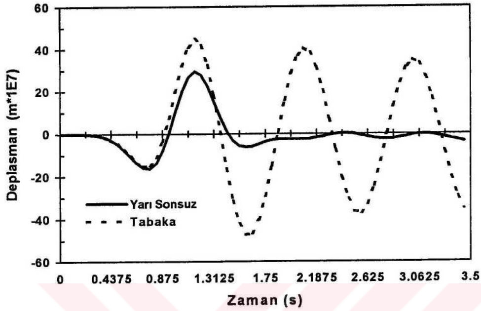
Şekil 3.44. Düşey yükten dolayı düşey deplasman
