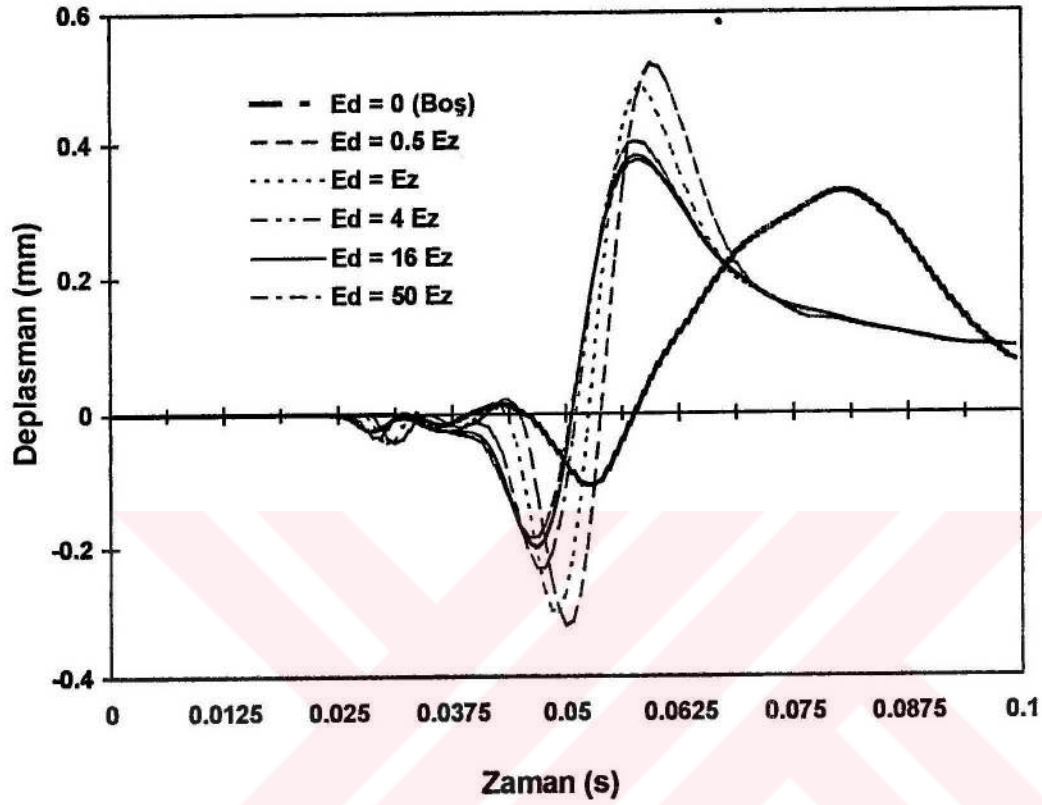
Şekil 3.39. Çeşitli dolgu malzemeleri için B noktasının deplasmanı
