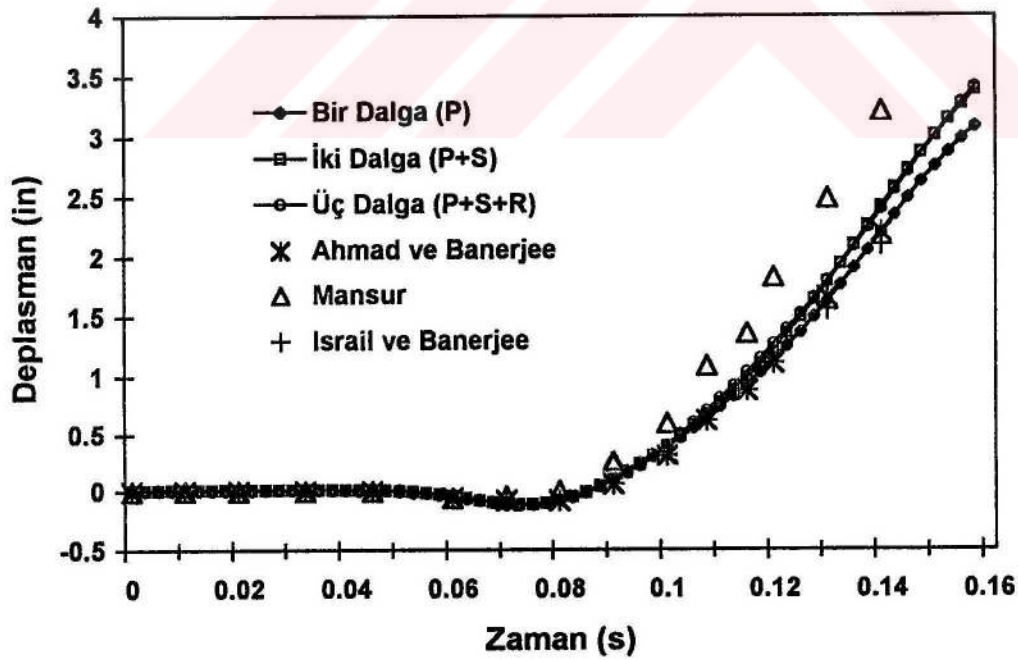
Şekil 3.32. G noktasındaki düşey deplasmanın zamanla değişimi
