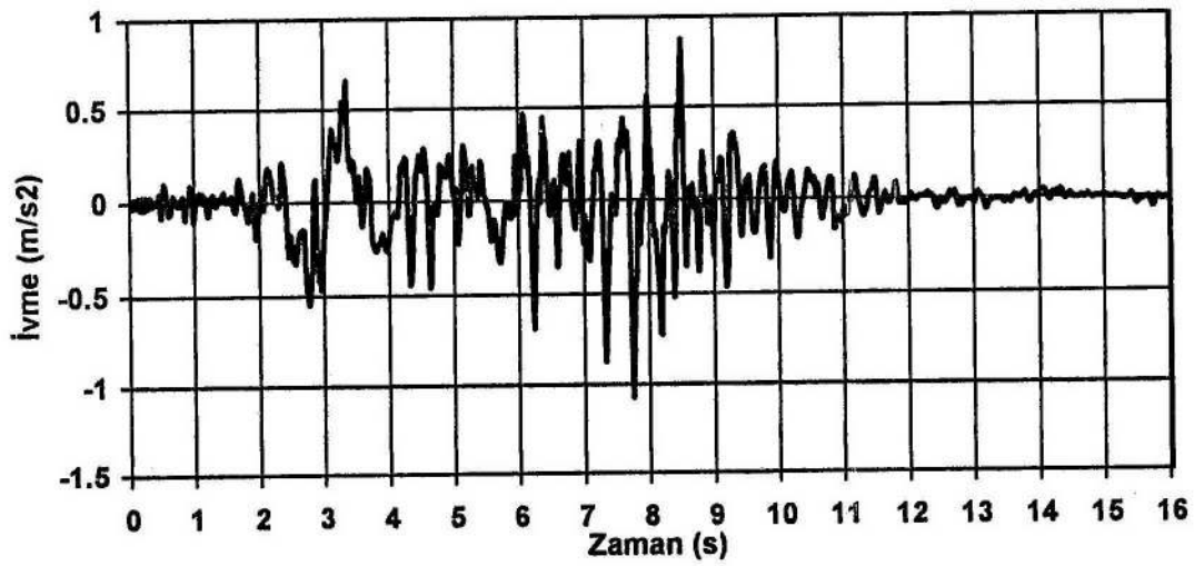
Şekil 5.14. PACOIMA depremi ivme kaydı
