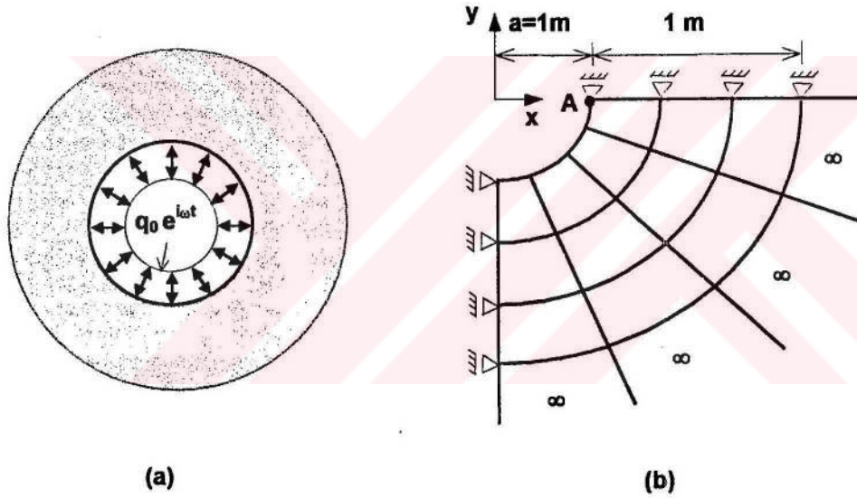
Şekil 3.12. İçerisinde küresel oyuk bulunan sonsuz zemin
