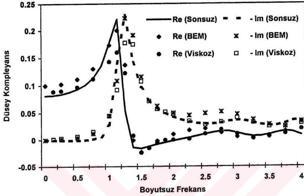
Şekil 4.15. Boyutsuz düşey kompleyansın karşılaştırılması
