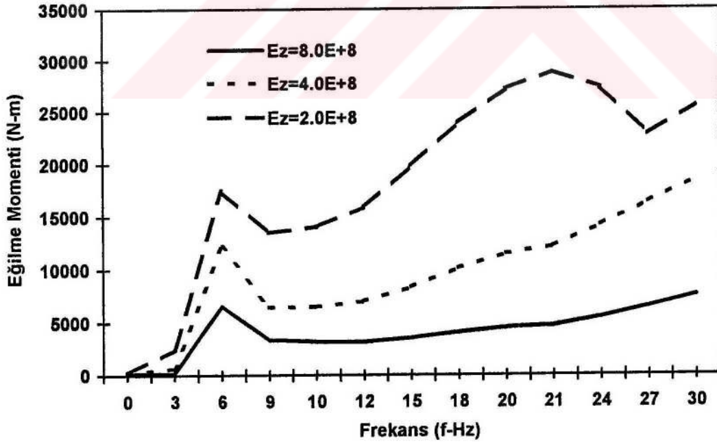
Şekil 4.32. Eğilme Momentinin frekansla değişimi
