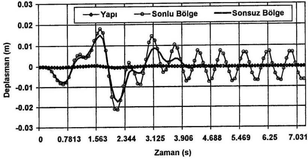
Şekil 5.9. B noktasındaki deplasmanın zamanla değişimi
