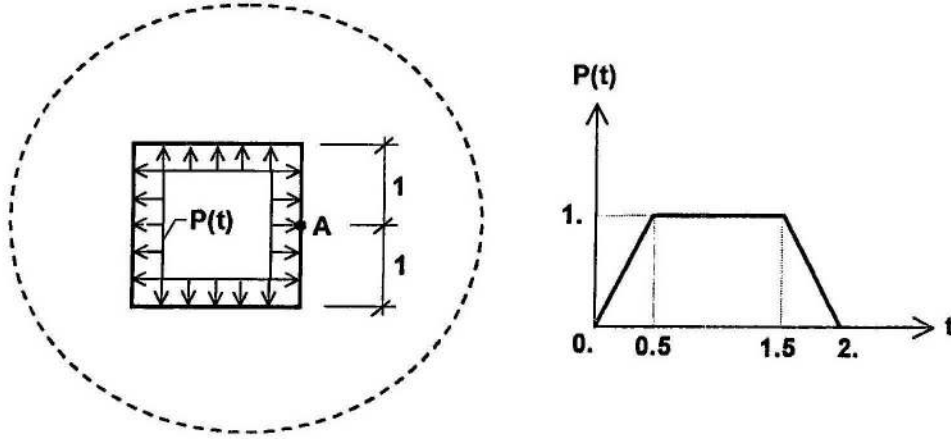
Şekil 3.24. Ortasında kare delik bulunan sonsuz levha
