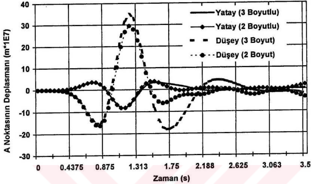
Şekil 4.33. A noktasının yatay ve düşey deplasmanı
