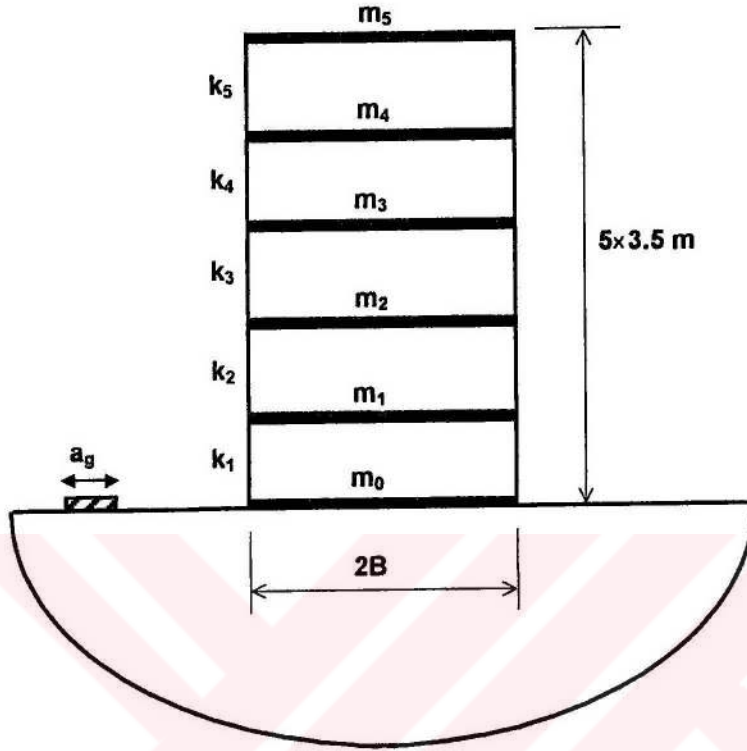
Şekil 5.13. 5 katlı kesme tipi bina
