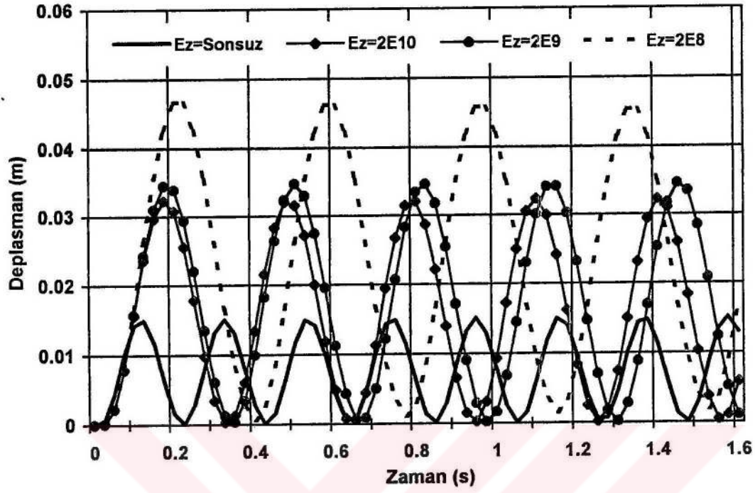
Şekil 4.40. Yatay deplasmanın zamanla değişimi
