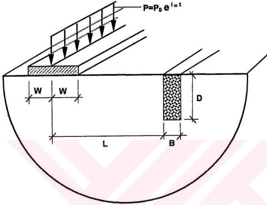
Şekil 3.21. Pasif izolasyon problemi
