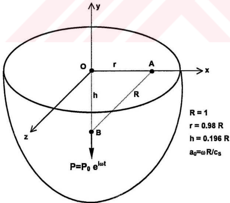
Şekil 3.14. Gömülü tekil yüklemeye maruz yarı sonsuz zemin
