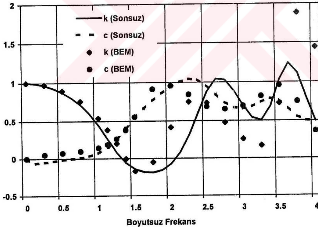
Şekil 4.17. k ve c değerlerinin frekansla değişimi
