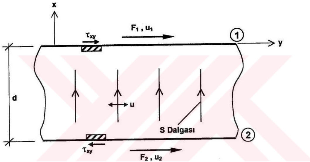
Şekil 5.2. Zemin tabakasında dalga yayılması
