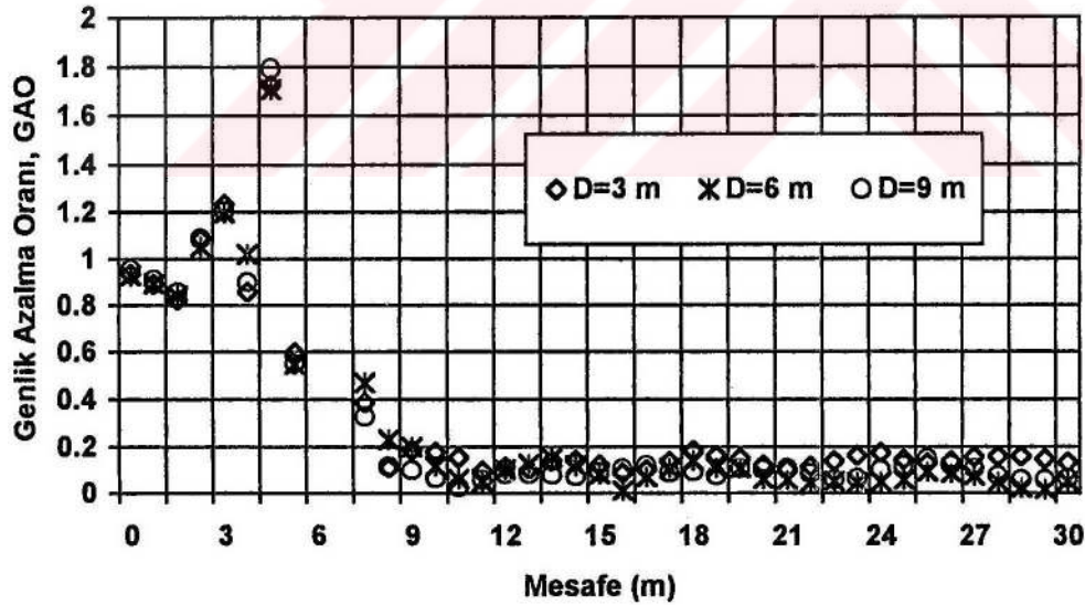
Şekil 3.19. Aktif izolasyonda çukur boş iken genlik azalma oranları
