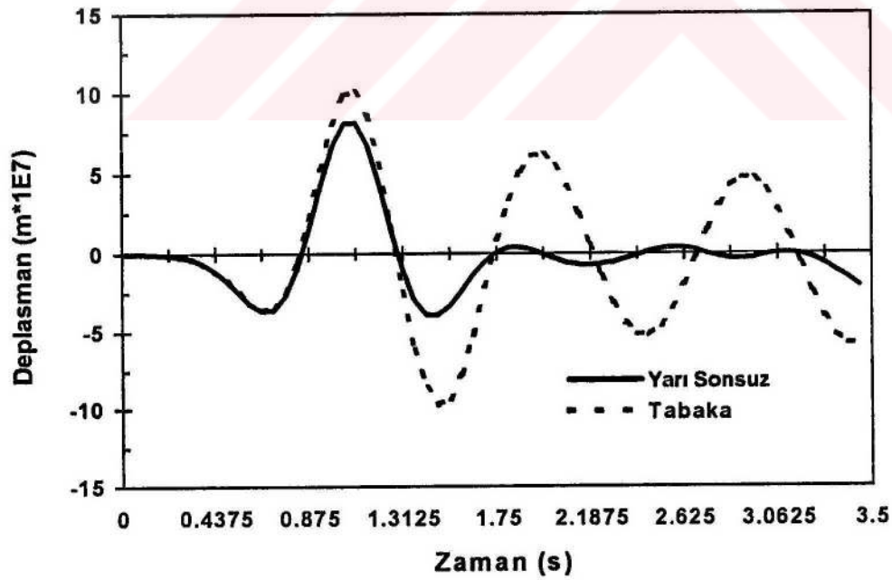
Şekil 3.45. Düşey yükten dolayı yatay deplasman
