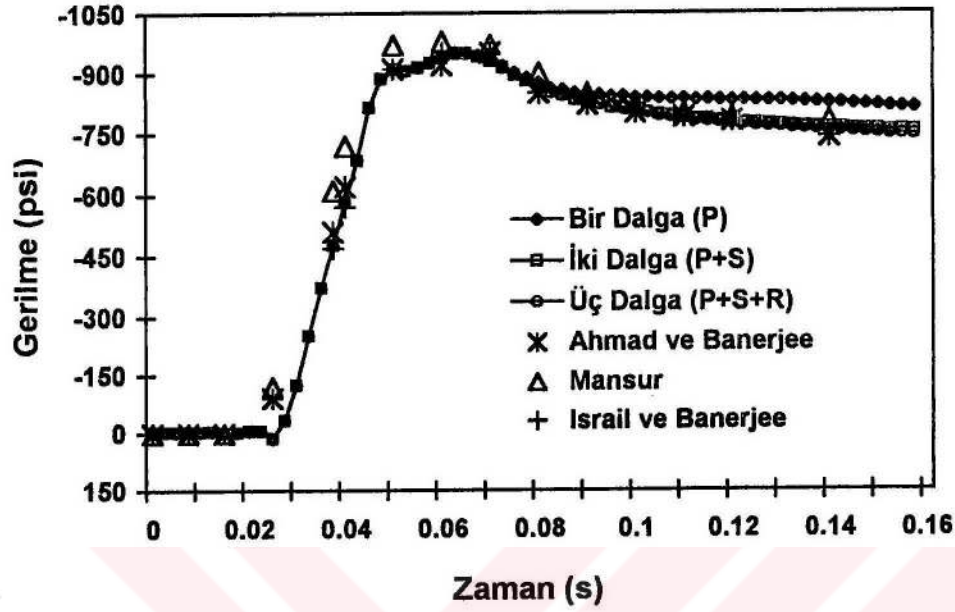
Şekil 3.29. C noktasındaki düşey gerilmenin zamanla değişimi
