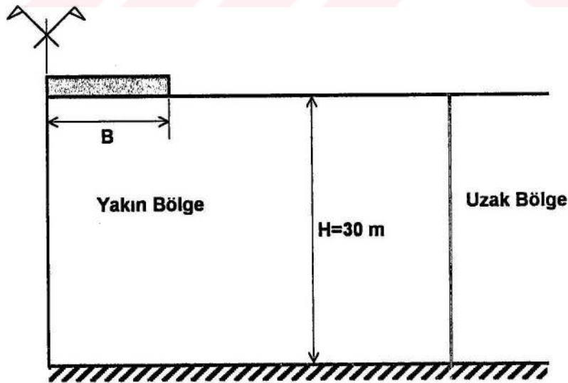
Şekil 4.13. Elastik zemin tabakası üzerinde kare temel (karşıdan görünüş)
