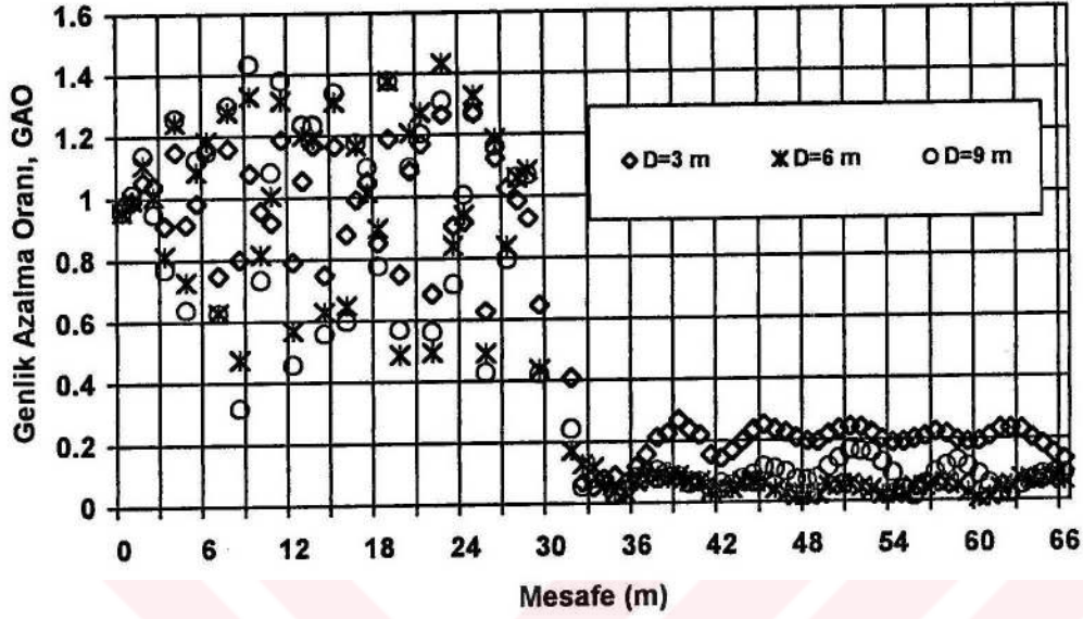
Şekil 3.22. Pasif izolasyonda çukur boş iken genlik azalma oranları
