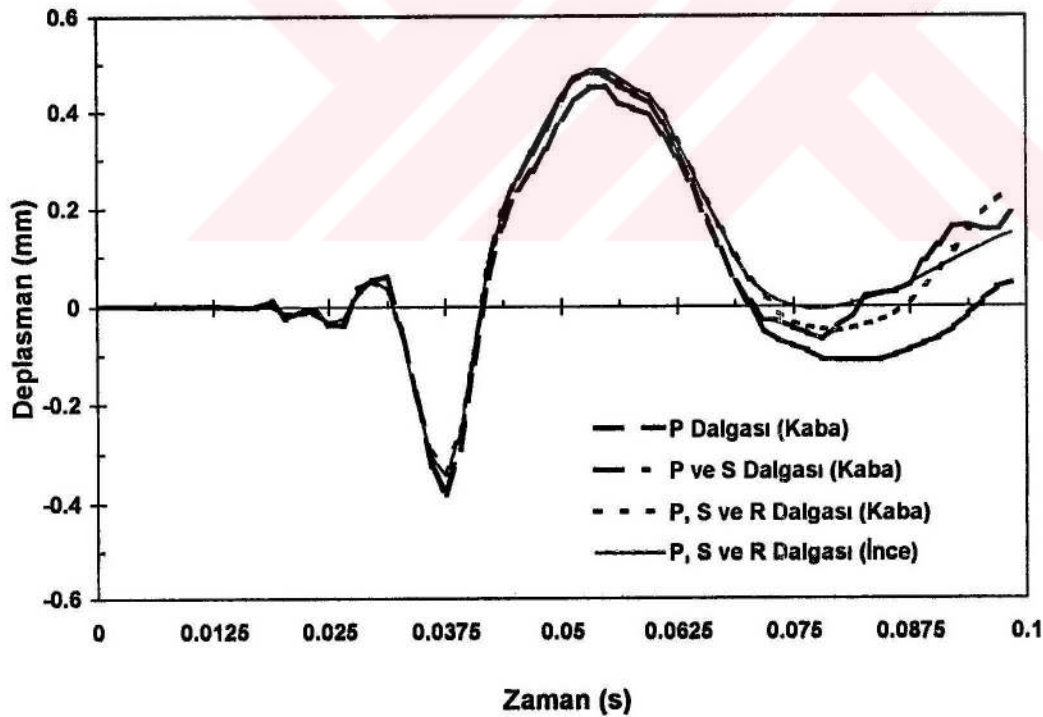
Şekil 3.34. A noktasının (çukurun gerisinde) düşey deplasmanı
