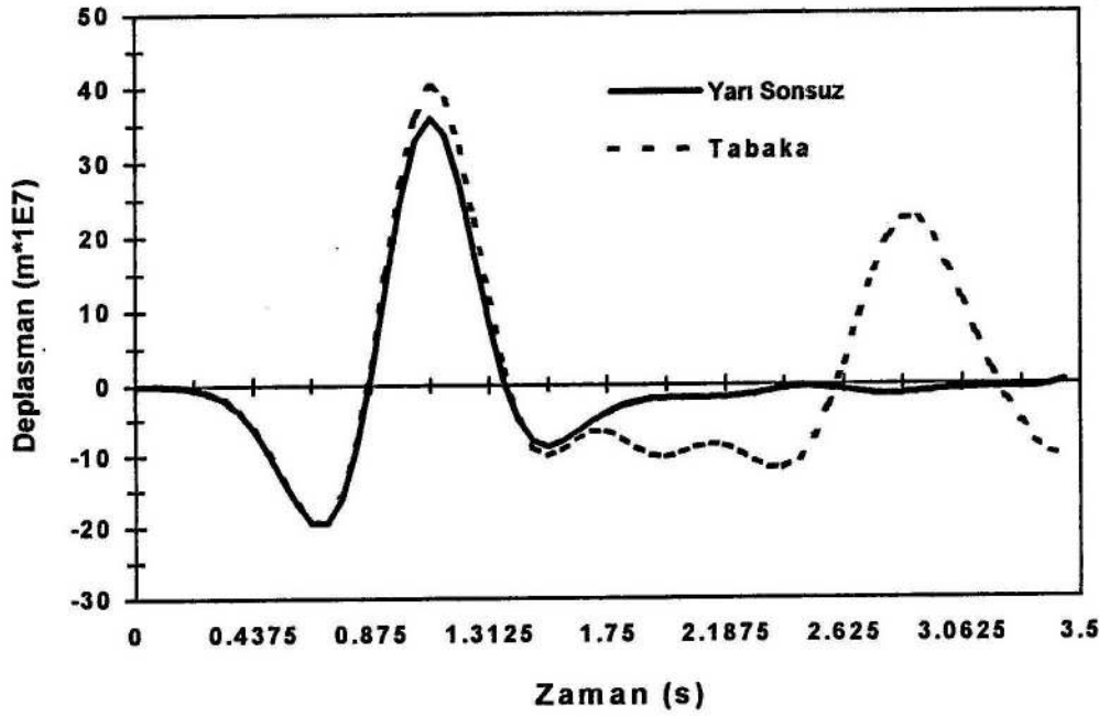
Şekil 3.46. Yatay yükten dolayı yatay deplasman
