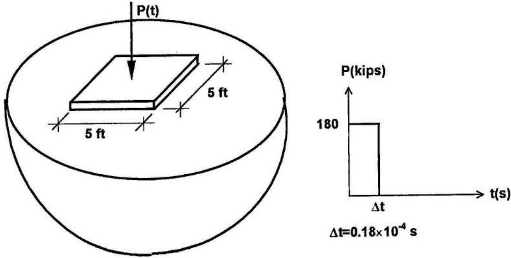
Şekil 4.34. Yarı sonsuz zemin üzerindeki temelin geometri ve yüklemesi
