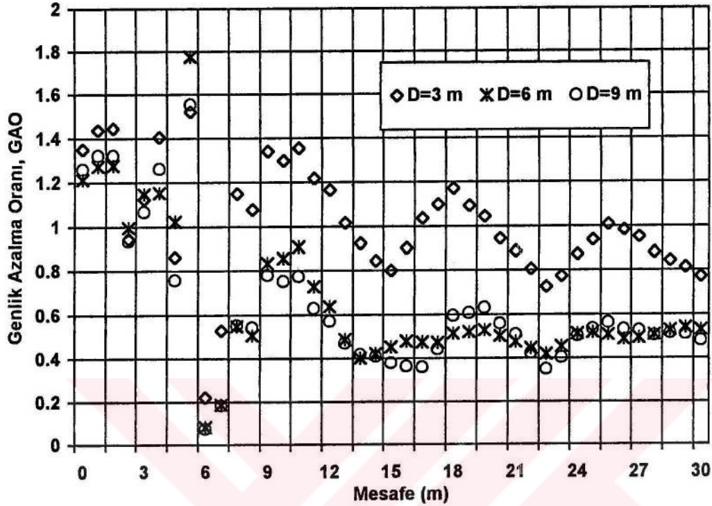
Şekil 3.20. Aktif izolasyonda çukur beton dolu iken genlik azalma oranları
