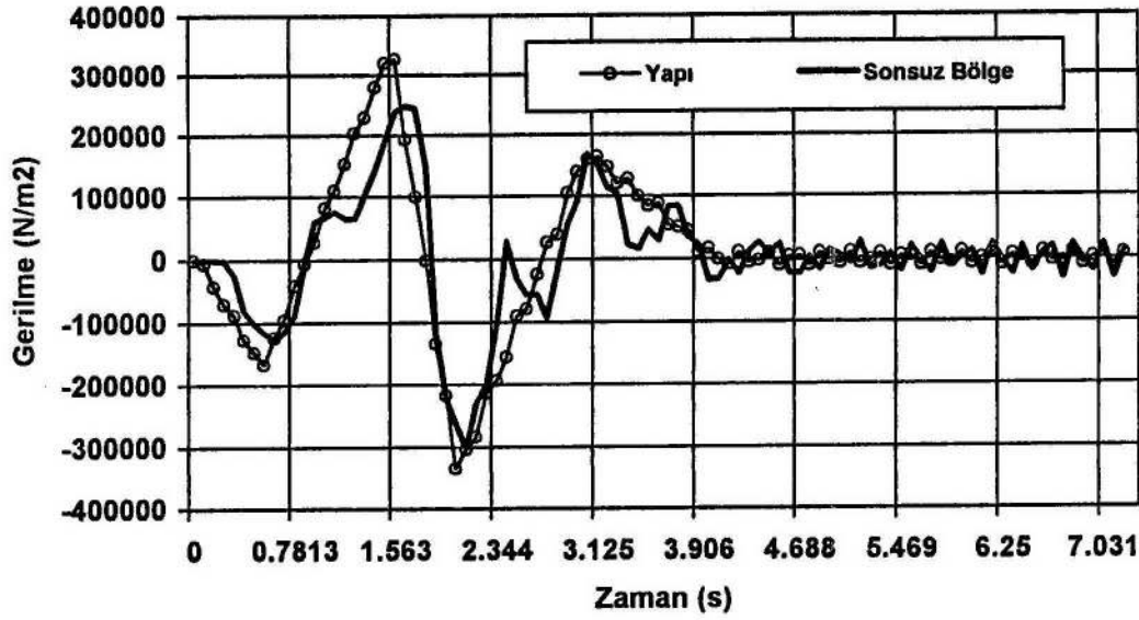
Şekil 5.11. A noktasındaki düşey gerilmenin zamanla değişimi
