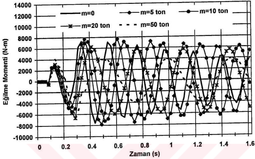
Şekil 4.46. Eğilme momentinin kütle ile değişimi
