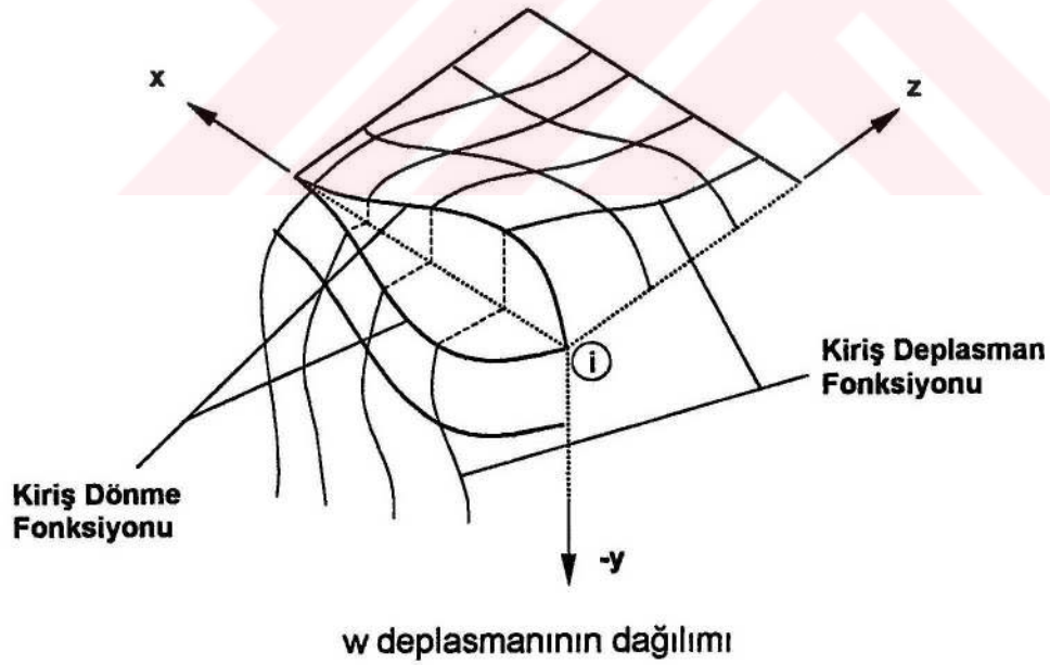
Şekil D.10. \theta_y dönmesinden dolayı deplasmanların yüzey boyunca değişimi
