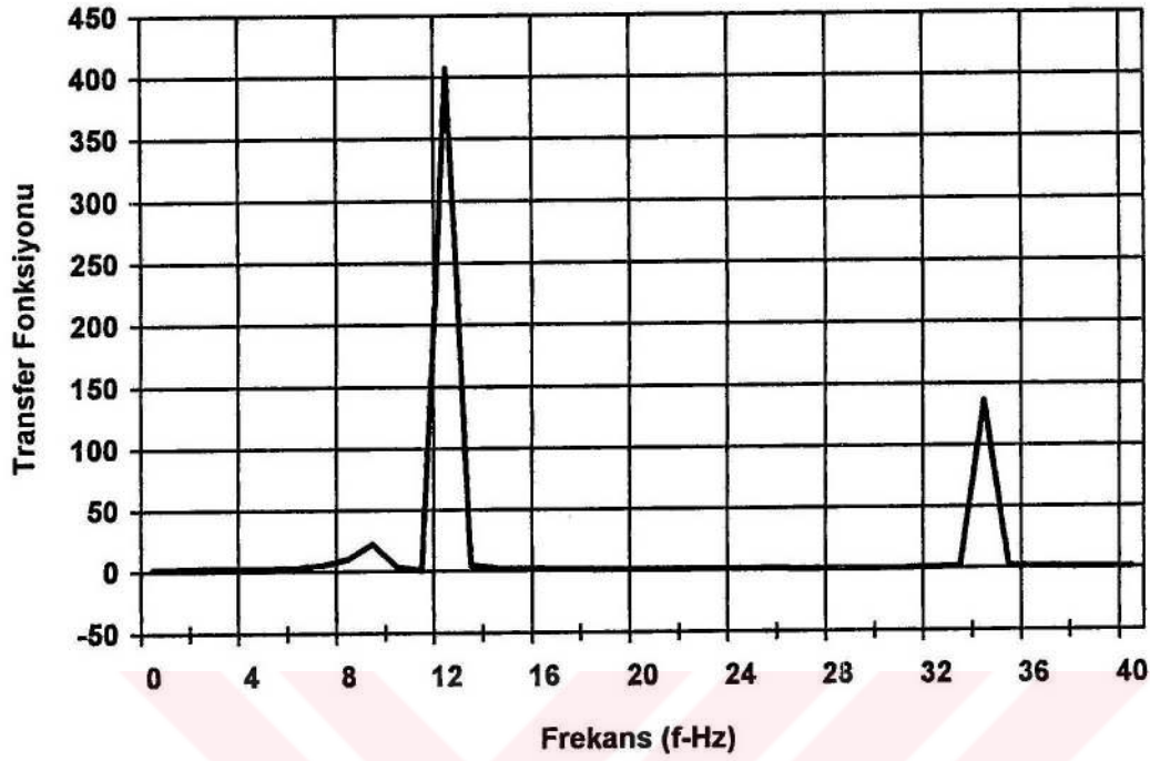
Şekil 4.25. Eğilme momenti transfer fonksiyonu
