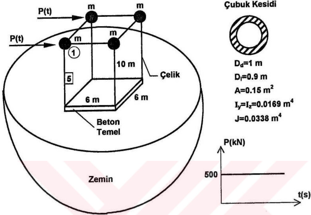
Şekil 4.39. Adım tipi yüklemeye maruz çerçeve
