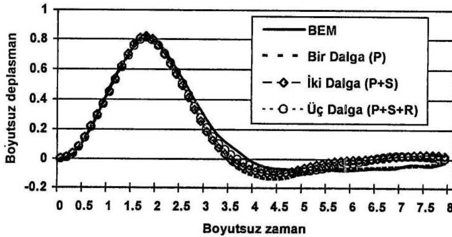
Şekil 3.25. A noktasındaki yatay deplasmanın zamanla değişimi
