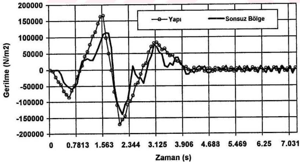
Şekil 5.10. A noktasındaki yatay gerilmenin zamanla değişimi
