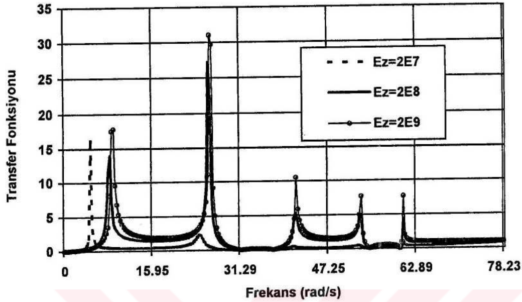
Şekil 5.17. 5. katın çeşitli zeminler için transfer fonksiyonu
