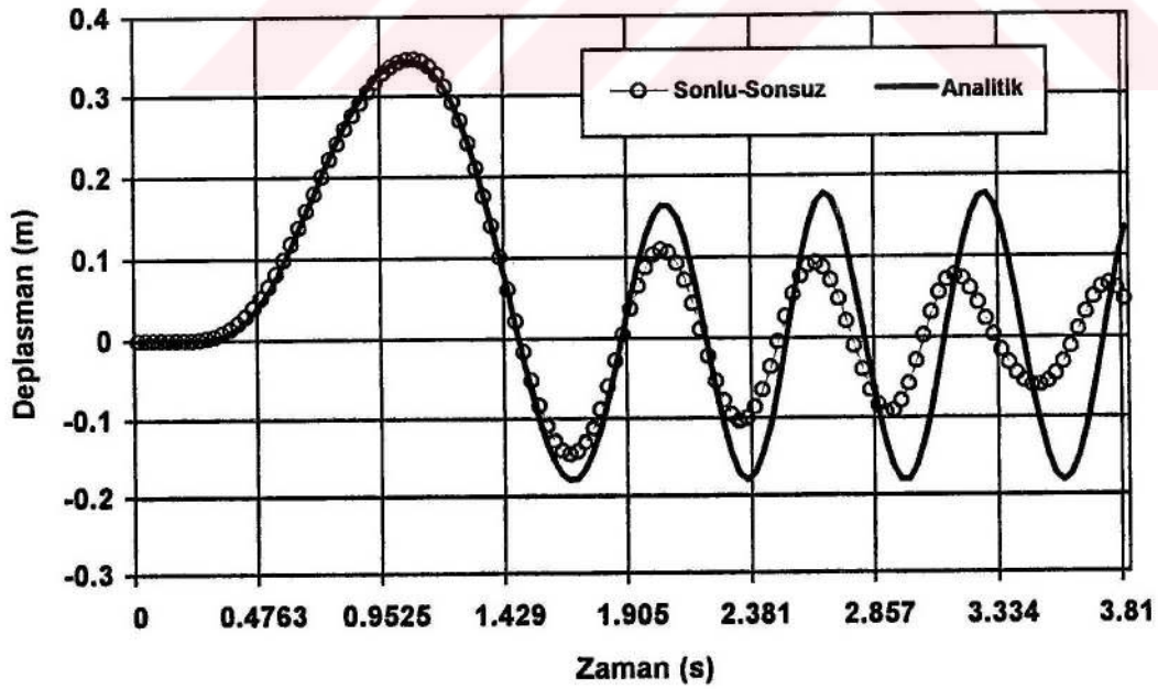
Şekil 5.6. Zeminin üst noktasındaki deplasmanın zamanla değişimi
