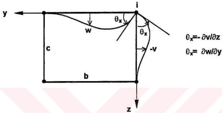
Şekil D.5. \theta_x dönmesi durumu
