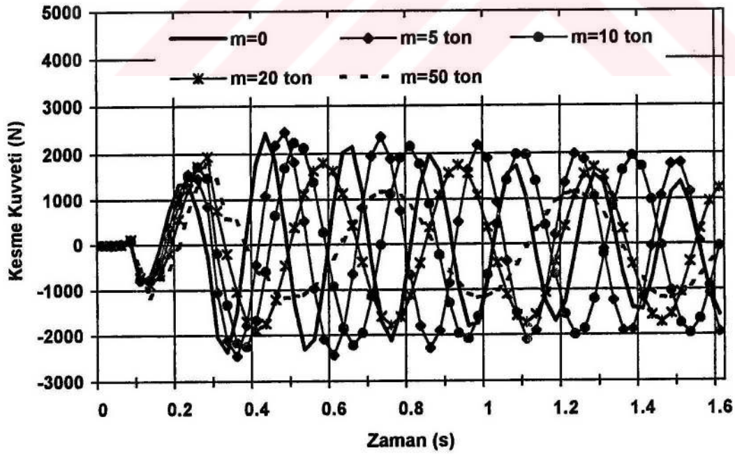
Şekil 4.45. Kesme kuvvetinin kütle ile değişimi
