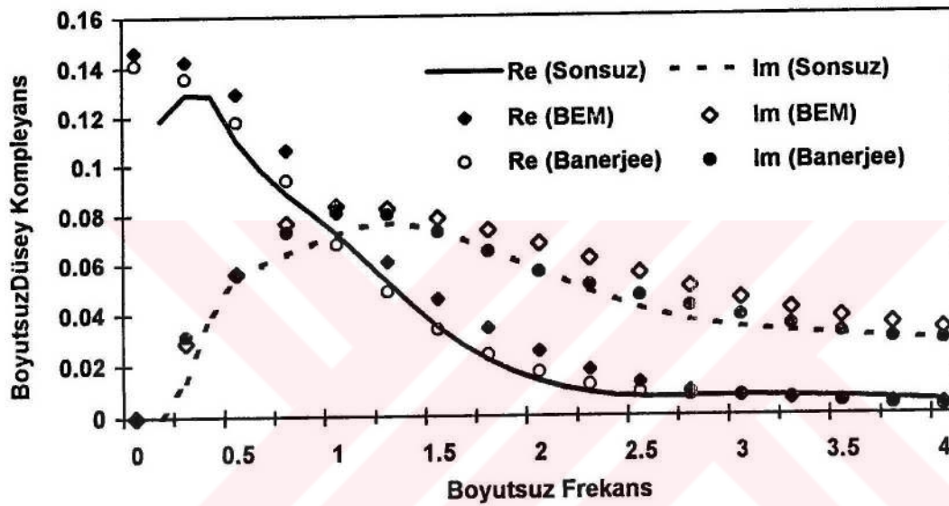
Şekil 4.10. Boyutsuz düşey komplekansın frekans ile değişimi
