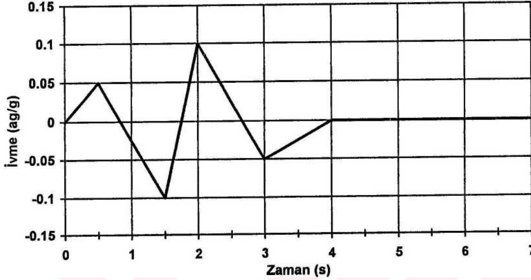
Şekil 5.8. İvmenin zamanla değişimi
