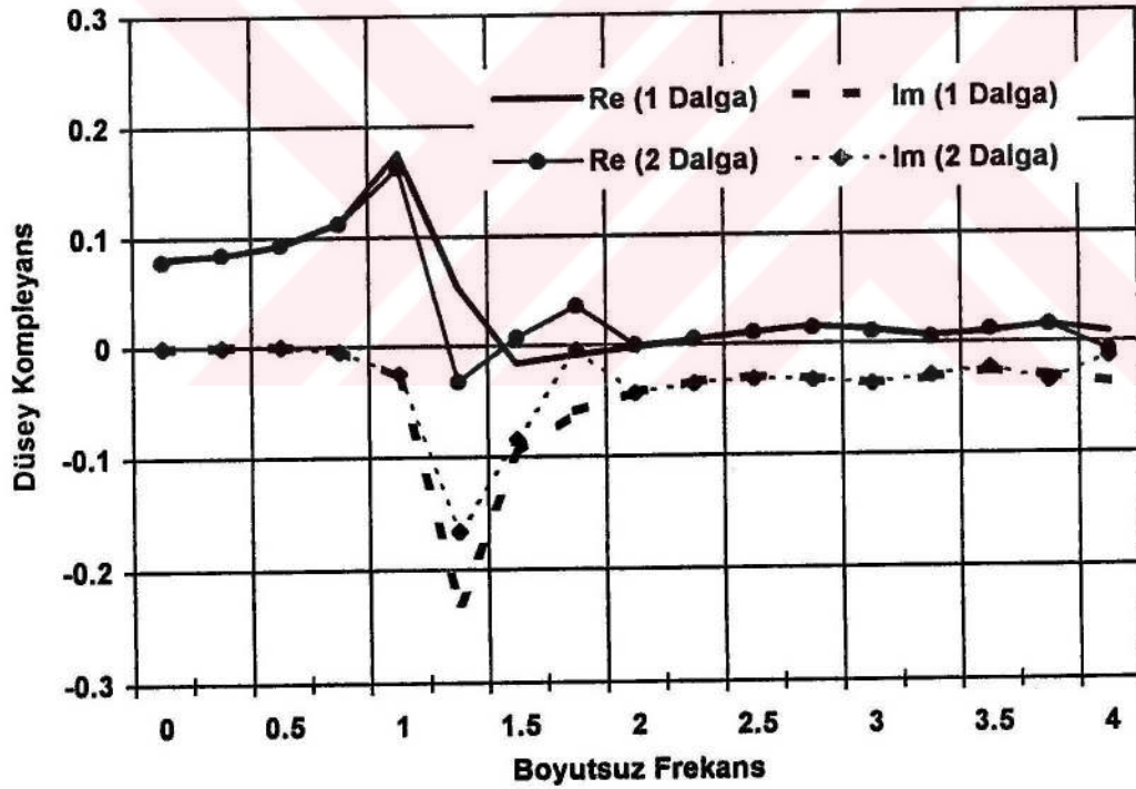
Şekil 4.14. Boyutsuz düşey kompleyansın frekansla değişimi
