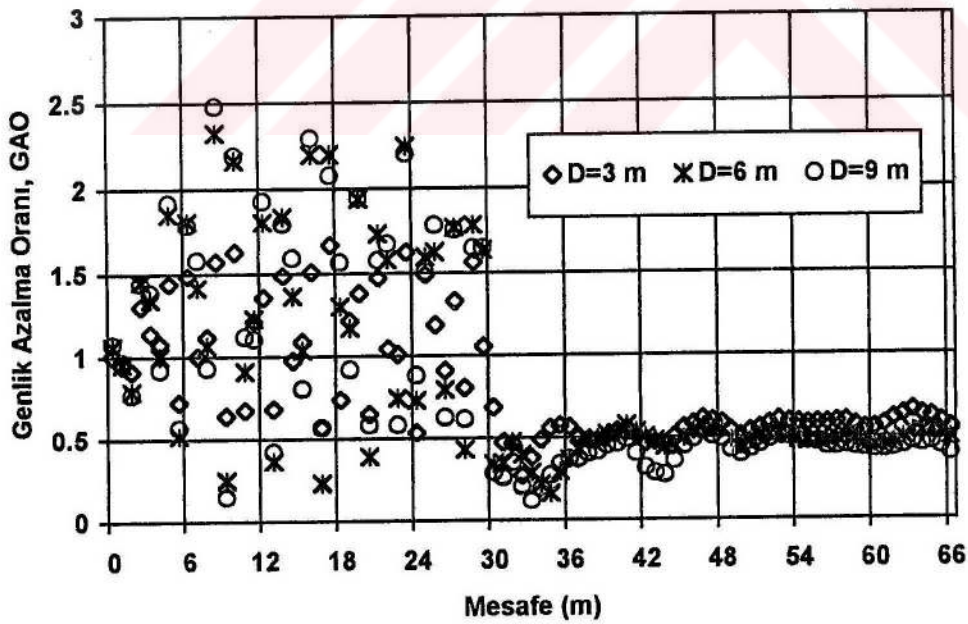
Şekil 3.23. Pasif izolasyonda çukur beton dolu iken genlik azalma oranları
