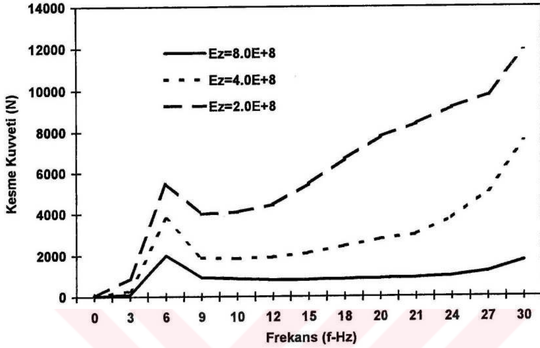
Şekil 4.31. Kesme kuvvetinin frekansla değişimi
