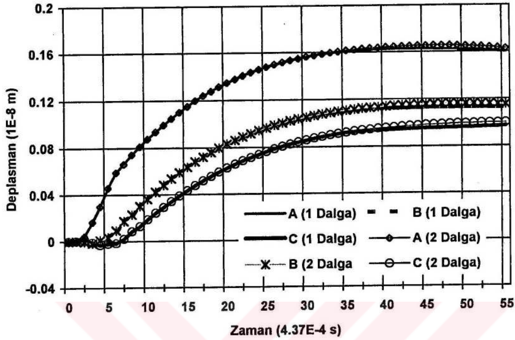
Şekil 4.38. A, B ve C noktalarının düşey deplasmanları
