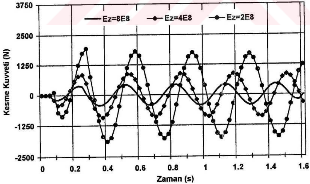
Őekil 4.48. Kesme kuvvetinin zemin rijitliđi ile deđiŐimi
