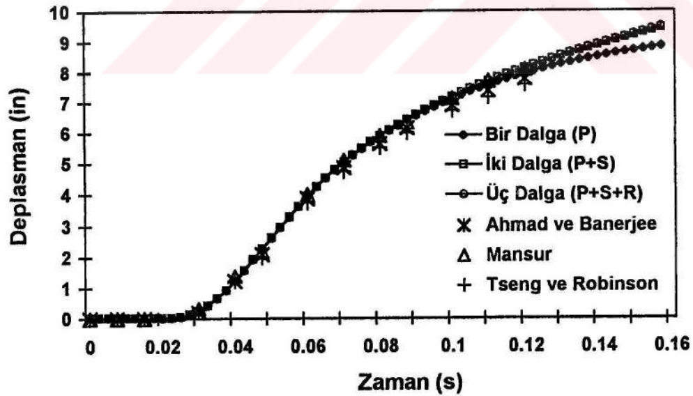
Şekil 3.30. E noktasındaki düşey deplasmanın zamanla değişimi
