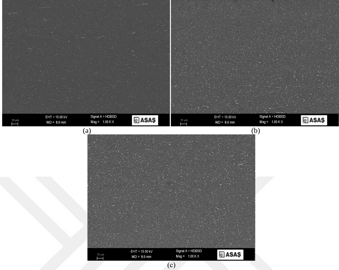
Şekil 4.36. 3105 alaşıma ait (1-C prosesi) dikey kesit kenar bölge SEM mikroyapı görüntüleri; a) 280°C b) 300°C c) 320°C nihai tav sonrası.
