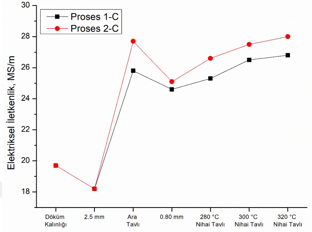
Şekil 4.41. 3105 alaşım elektriksel iletkenlik ölçüm sonuçları.
