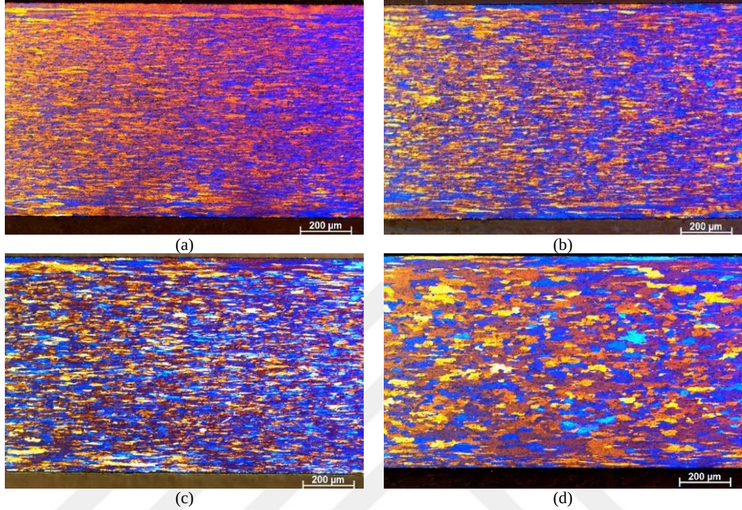
Şekil 4.9. 500°C ara tavlı 3004 alaşım (2-B prosesi); a) Nihai tavsız b) 280°C c) 300°C d) 320°C nihai tavlı numunenin hadde yönüne dik polarize ışık optik mikroyapı görüntüleri.
