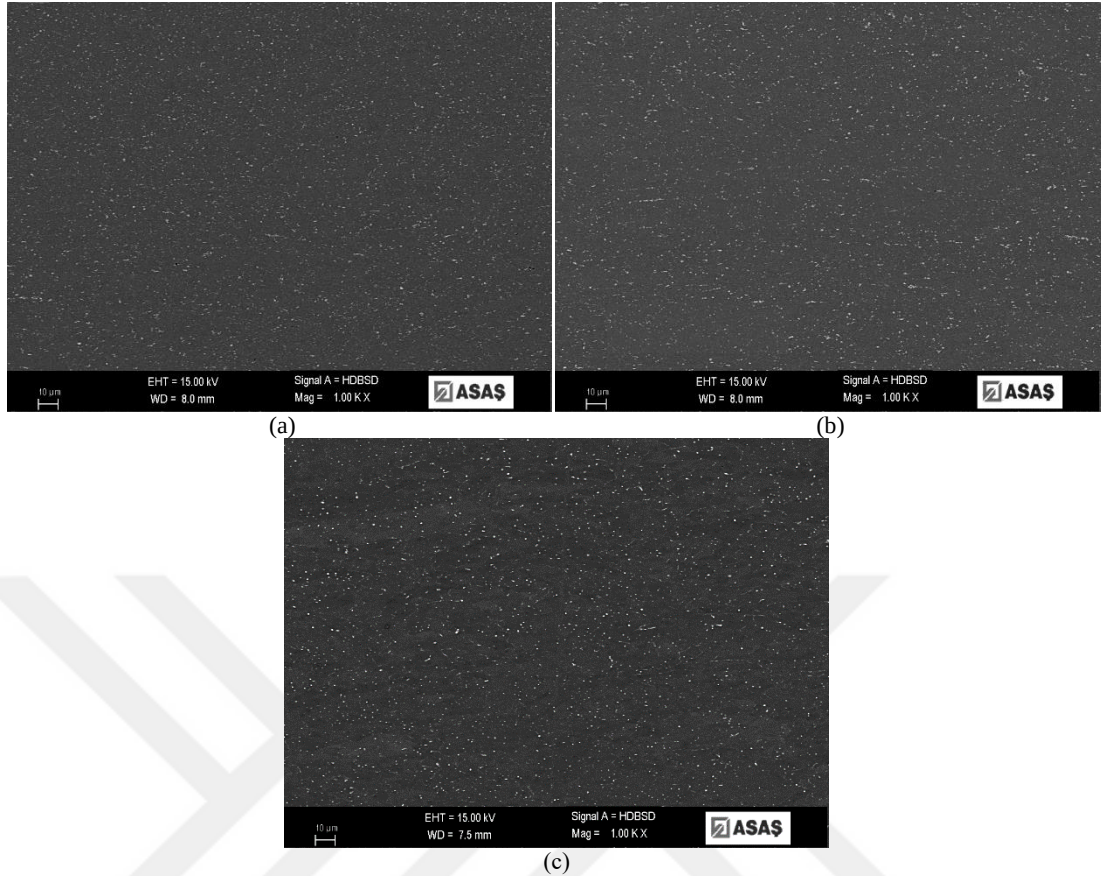
Şekil 4.28. 3005 alaşıma ait (2-A prosesi) dikey kesit kenar bölge SEM mikroyapı; a) 280°C b) 300°C c) 320°C nihai tav sonrası.
