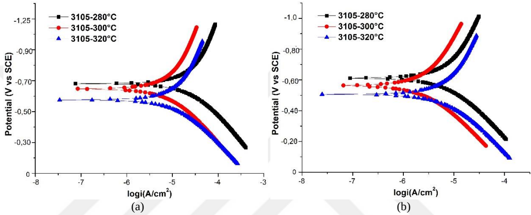
Şekil 4.60. 280°C, 300°C ve 320°C nihai tav sonrası 3105 alaşım tafel polarizasyon eğrileri; a) 450°C ara tavlı 1-C b) 500°C ara tavlı 2-C prosesi.
