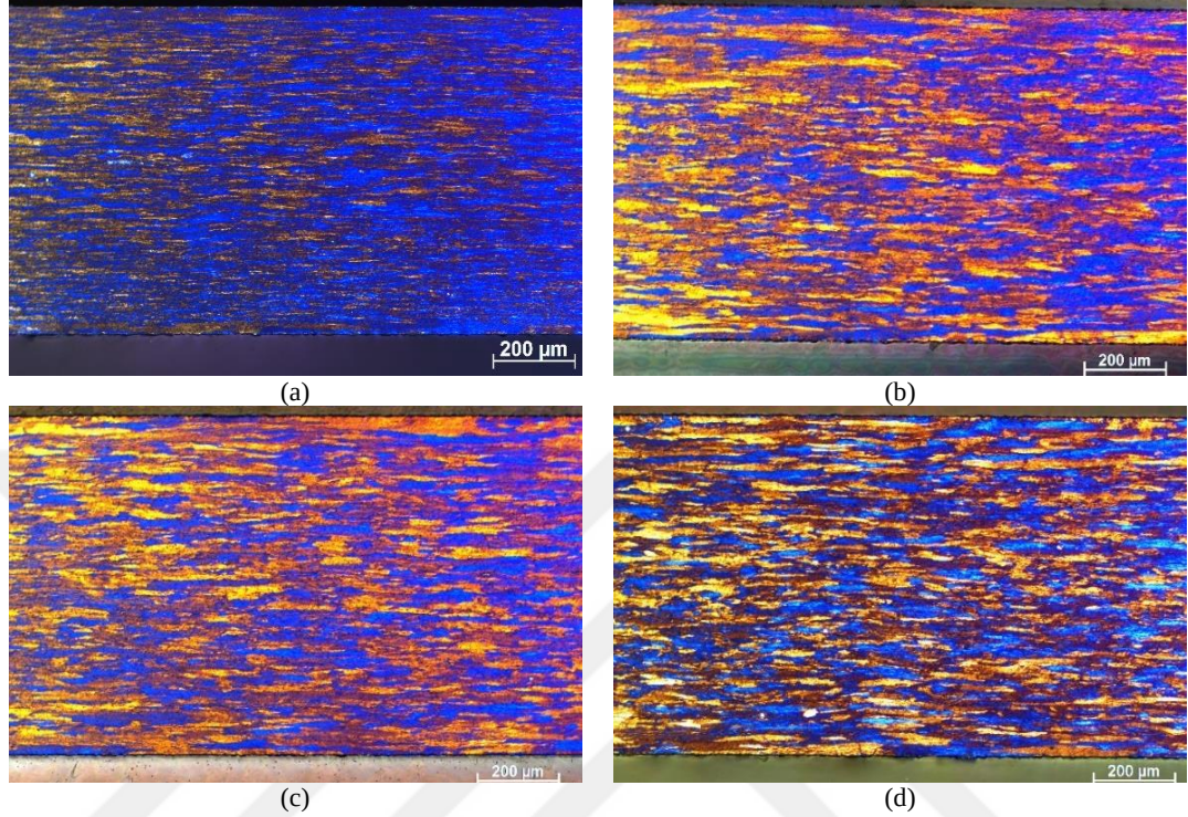
Şekil 4.5. 500°C ara tavlı 3005 alaşım (2-A prosesi); a) Nihai tavsız b) 280°C c) 300°C d) 320°C nihai tavlı numunenin hadde yönüne dik polarize ışık optik mikroyapı görüntüleri.
