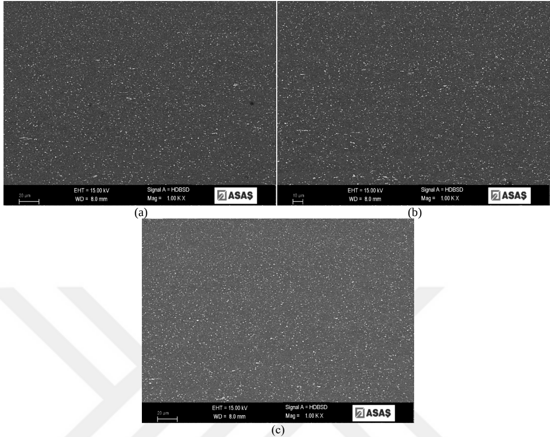
Şekil 4.30. 3004 alaşıma ait (1-B prosesi) dikey kesit kenar bölge SEM mikroyapı; a) 280°C b) 300°C c) 320°C nihai tav sonrası.
