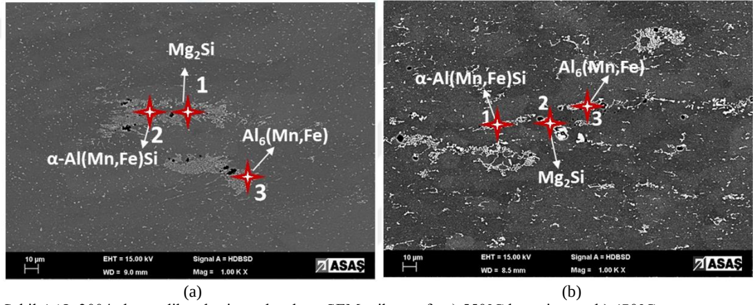
Şekil 4.18. 3004 alaşım dikey kesit merkez hattı SEM mikrografı; a) 550°C homojen tav b) 450°C ara tav sonrası.
