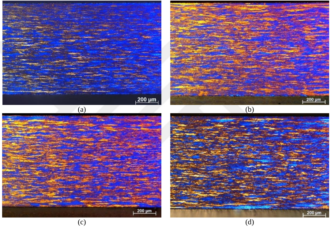
Şekil 4.4. 450°C ara tavlı 3005 alaşım (1-A prosesi); a) Nihai tavsız b) 280°C c) 300°C d) 320°C nihai tavlı numunenin hadde yönüne dik polarize ışık optik mikroyapı görüntüleri.
