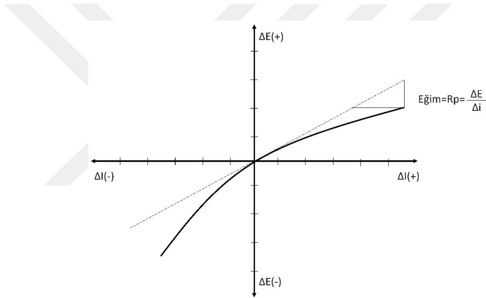
Şekil 2.20. Lineer polarizasyon yöntemi kapsamında R_p 'nin bulunması [56].
