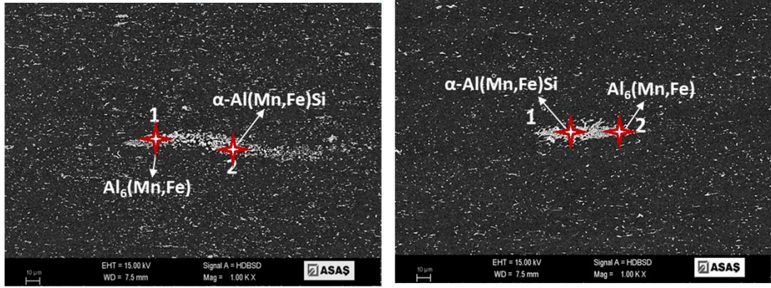
(a) (b) Şekil 4.23. 3105 alaşım dikey kesit merkez hattı SEM mikrografı; a) 450°C b) 500°C ara tav sonrası.
