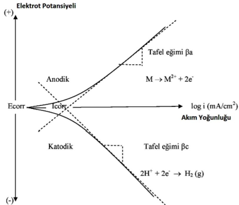
Şekil 2.19. Tafel ekstrapolasyon grafiği [56].
