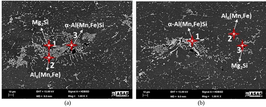
Şekil 4.16. 3004 alaşım dikey kesit merkez hattı SEM mikroyapısı; a) 450°C b) 500°C ara tav sonrası.
