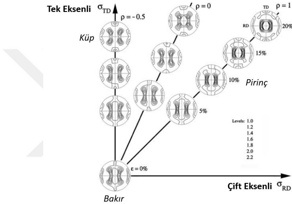
Şekil 2.17. 111 kutup figürü ile gösterilen çeşitli gerinim yolları altında alüminyumun doku gelişimi [47].
