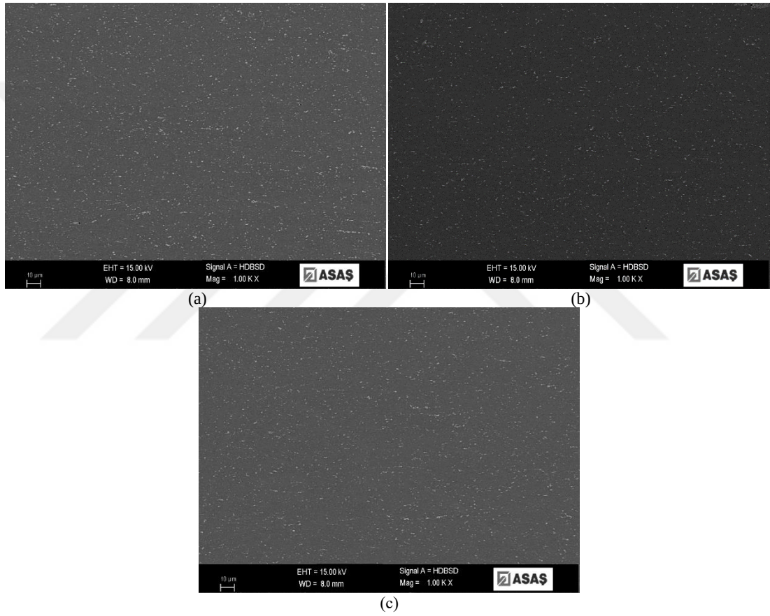
Şekil 4.26. 3005 alaşıma ait (1-A prosesi) dikey kesit kenar bölge SEM mikroyapısı; a) 280°C b) 300°C c) 320°C nihai tav sonrası.
