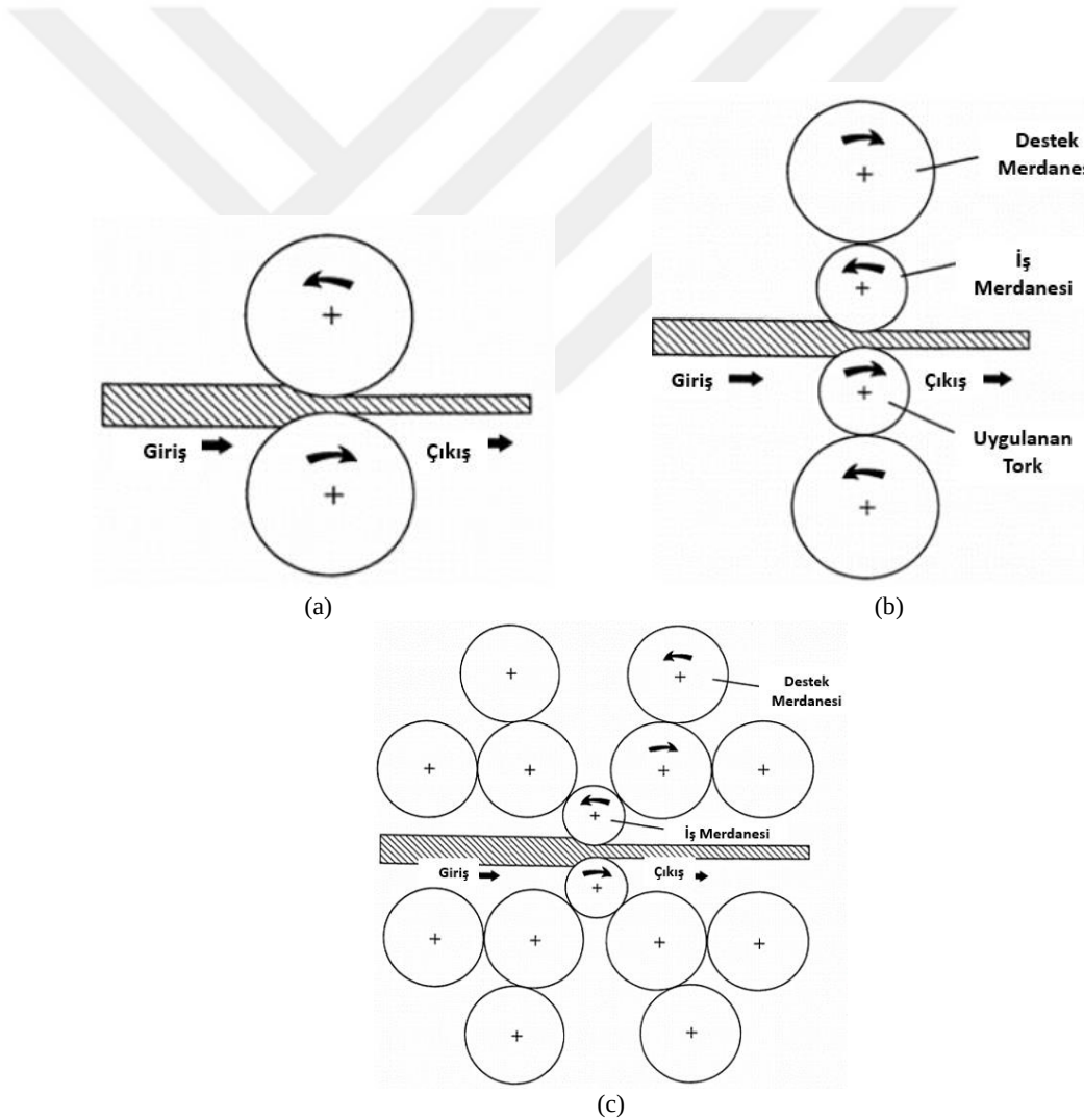
Şekil 2.8. Soğuk hadde merdane düzen tipleri; a) ikili düzen, b) dörtlü düzen ve c) çoklu kümelenme düzen [26].
