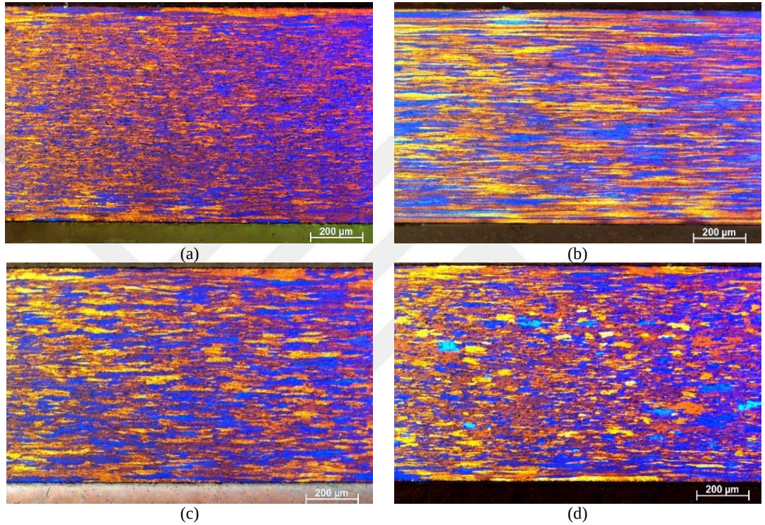
Şekil 4.8. 450°C ara tavlı 3004 alaşım (1-B prosesi); a) Nihai tavsız b) 280°C c) 300°C d) 320°C nihai tavlı numunenin hadde yönüne dik polarize ışık optik mikroyapı görüntüleri.
