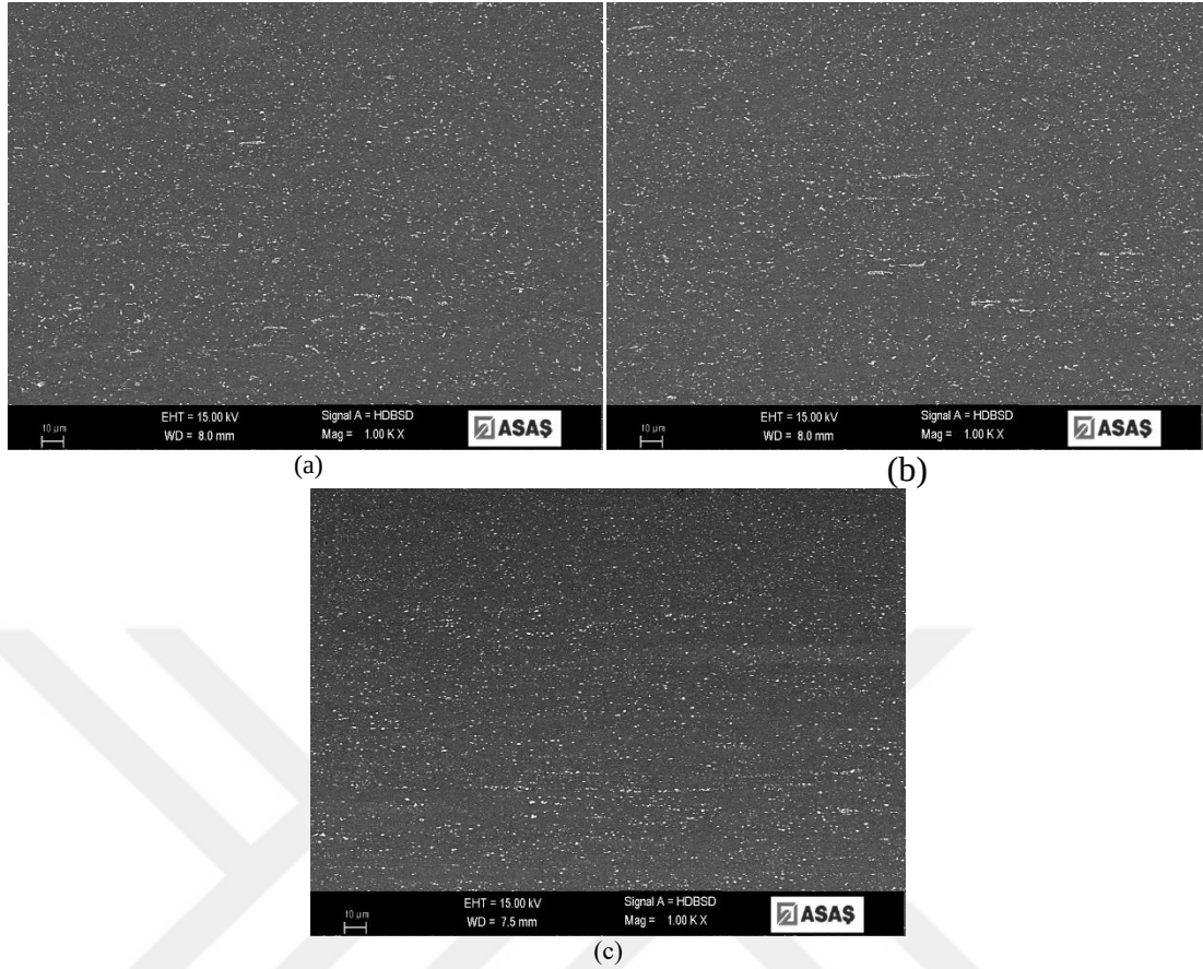
Şekil 4.15. Döküm halde dikey kesit kenar bölge SEM mikroyapısı; a) 3004 b) 3005 c) 3105 alaşım.
