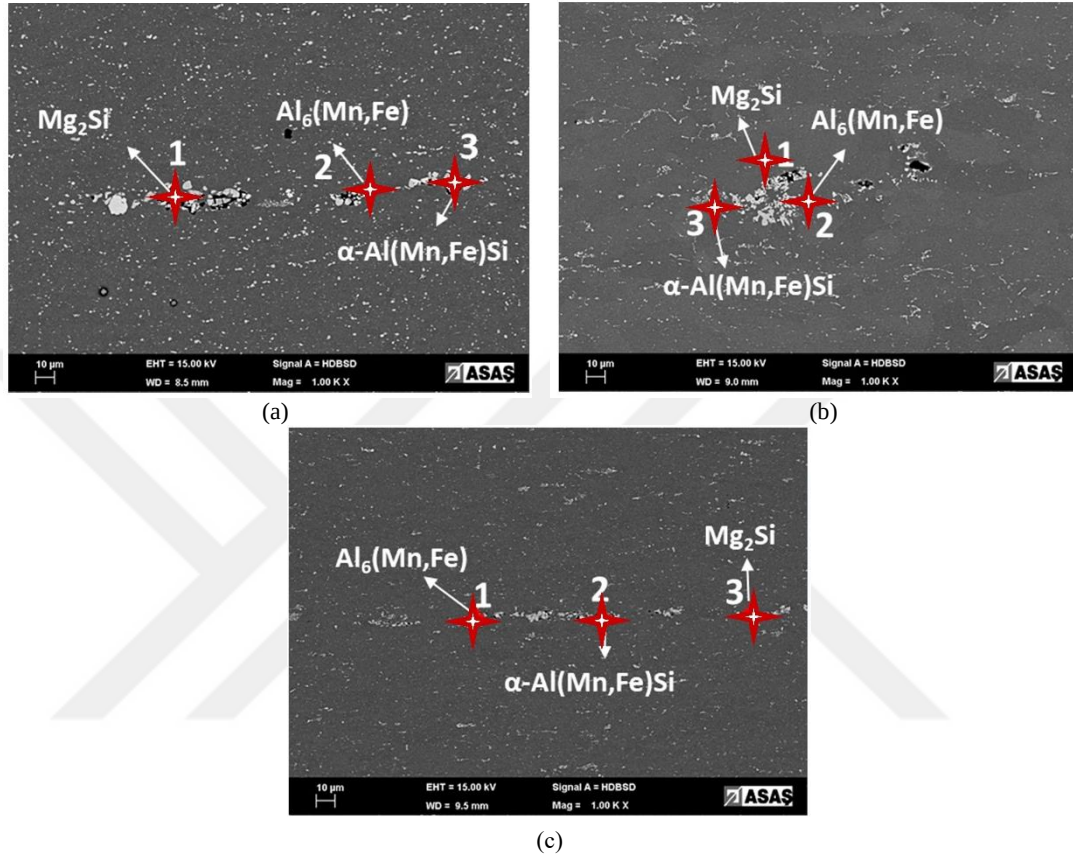
Şekil 4.31. 3004 alaşıma ait (2-B prosesi) dikey kesit merkez hattı SEM mikrofotografı; a) 280°C b) 300°C c) 320°C nihai tav sonrası.
