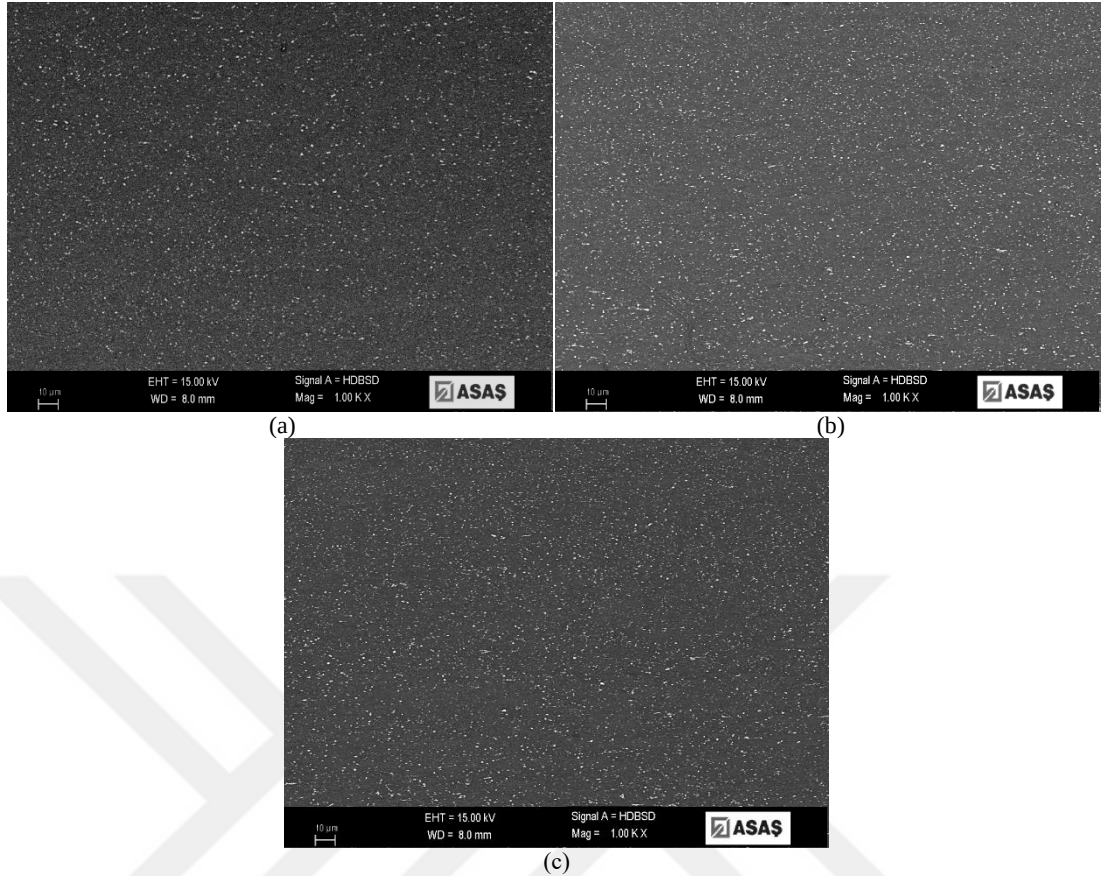
Şekil 4.32. 3004 alaşıma ait (2-B prosesi) dikey kesit kenar bölge SEM mikroyapı; a) 280°C b) 300°C c) 320°C nihai tav sonrası.
