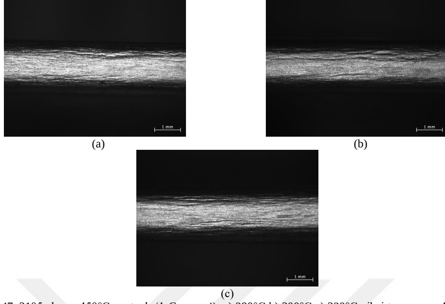
Şekil 4.47. 3105 alaşım 450°C ara tavlı (1-C prosesi); a) 280°C b) 300°C c) 320°C nihai tav sonrası 180° bükme stereo mikroskop makroyapı görüntüleri.
