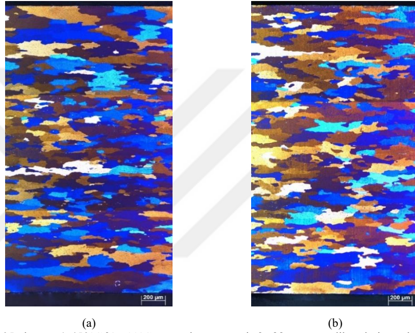
Şekil 4.11. 3105 alaşım; a) 450°C b) 500°C ara tavlı numunenin hadde yönüne dik polarize ışık optik mikroyapı görüntüleri.
