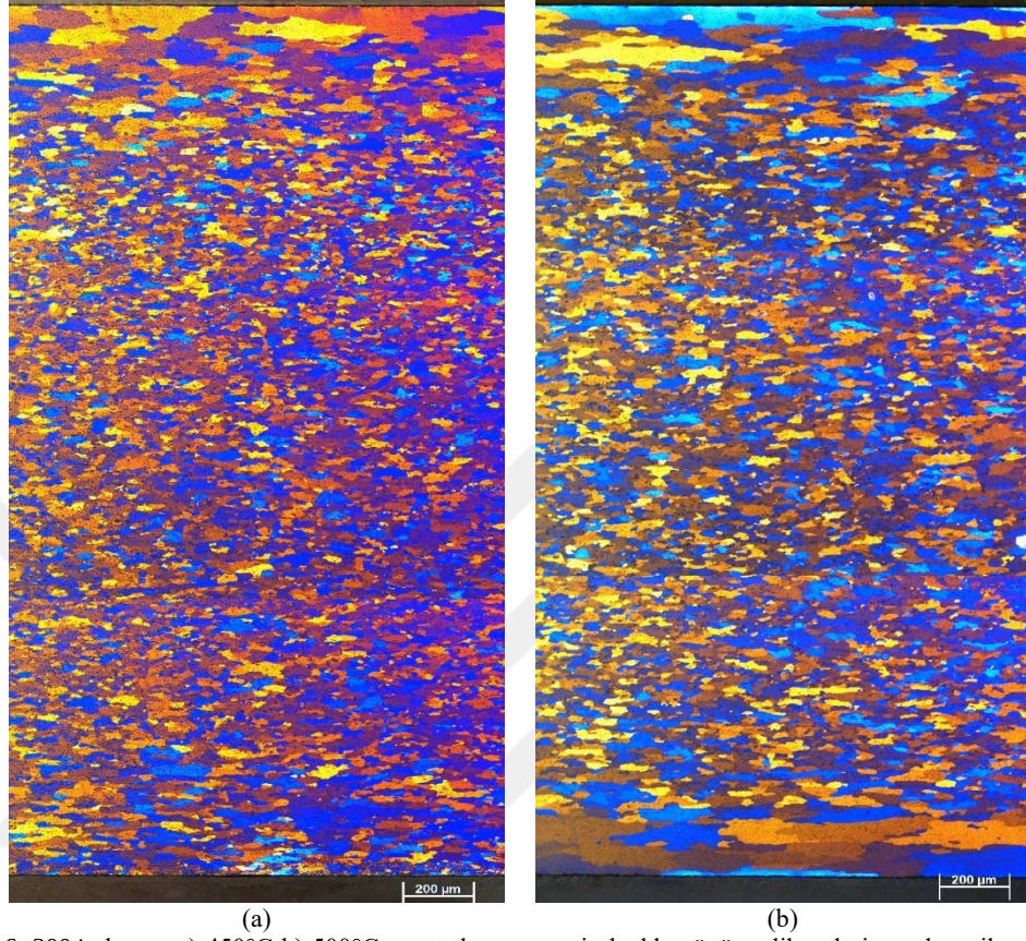
Şekil 4.6. 3004 alaşıım; a) 450°C b) 500°C ara tavlı numunenin hadde yönüne dik polarize ışık optik mikroyapı görüntüleri
