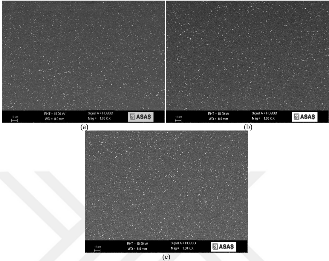
Şekil 4.34. 3004 alaşıma ait (3-B prosesi) dikey kesit kenar bölge SEM mikroyapısı; a) 280°C b) 300°C c) 320°C nihai tav sonrası.
