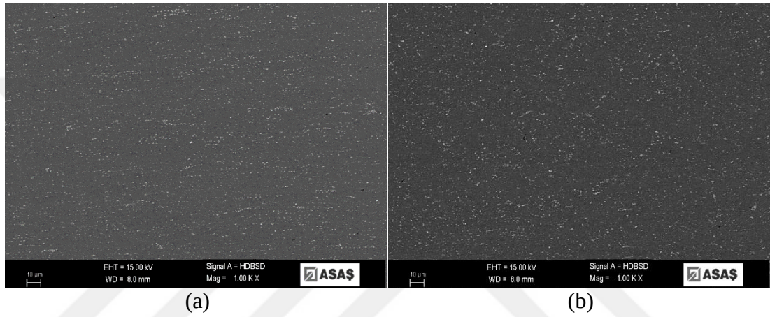
Şekil 4.22. 3005 alaşım dikey kesit kenar bölge SEM mikroyapı; a) 450°C b) 500°C ara tav sonrası.
