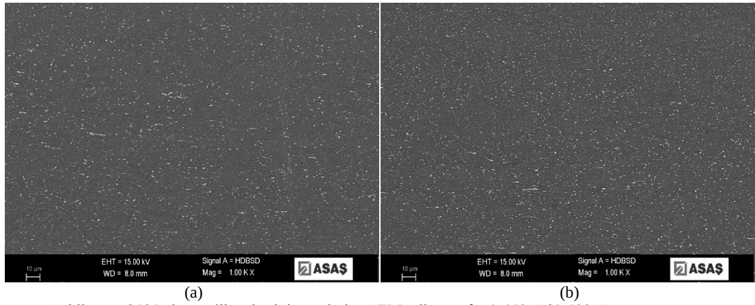
(a) (b) Şekil 4.24. 3105 alaşım dikey kesit kenar bölge SEM mikrografı; a) 450°C b) 500°C ara tav sonrası.
