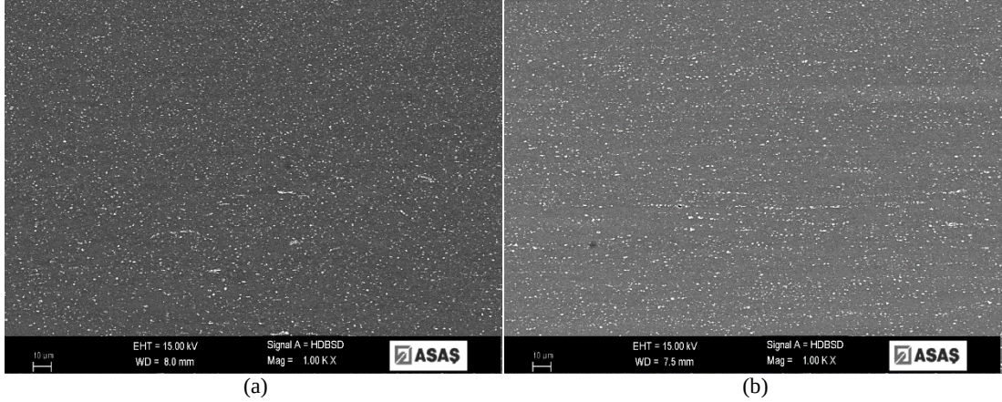
Şekil 4.19. 3004 alaşım dikey kesit kenar bölge SEM mikrofotografı; a) 550°C homojen tav b) 500°C ara tav sonrası.
