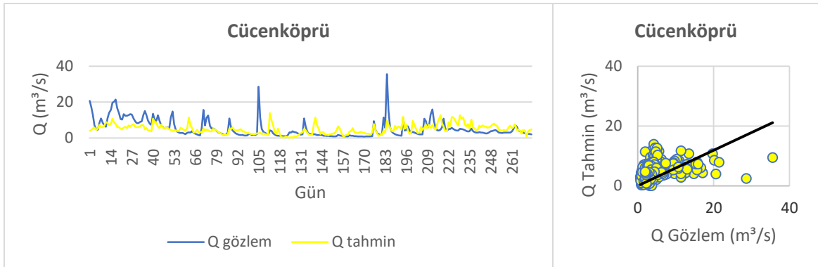
Şekil 3.38. Cücenköprü F3-M1 model değerlendirmesi
