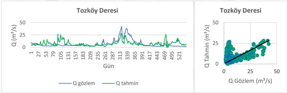
Şekil 3.11. Tozköy Deresi ANFIS M5 modeli performans değerlendirmesi
