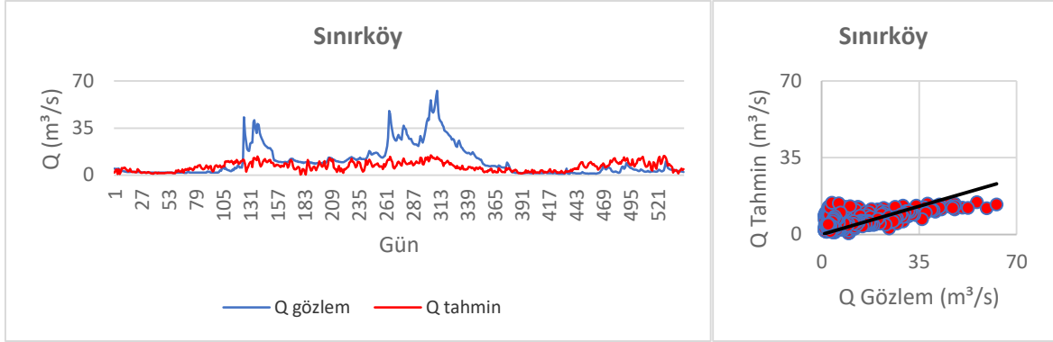
Şekil 3.61. Sınırköy MARS performans değerlendirmesi
