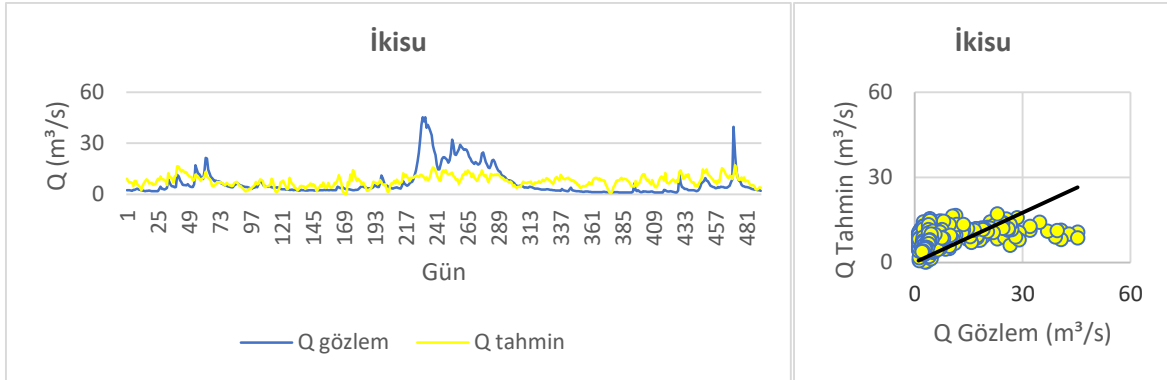
Şekil 3.54. İkisu F1-M3 model değerlendirme
