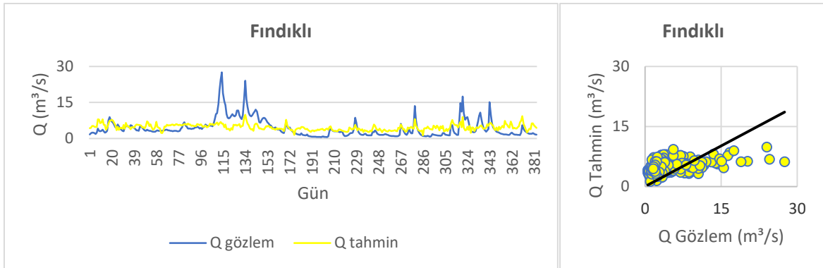
Şekil 3.30. Fındıklı F3-M3 model değerlendirmesi
