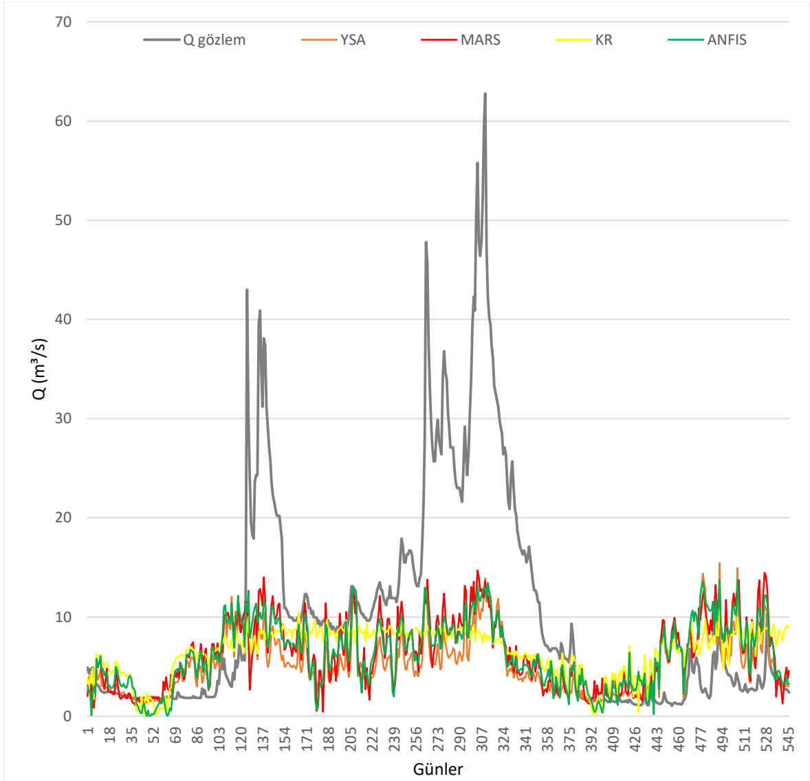
Ek Şekil 15. Sınırköy analiz konumunda kullanılan yöntemlere göre SPM debi tahmin performansı karşılaştırması
