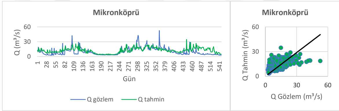
Şekil 3.47. Mikronköprü ANFIS M2 modeli performans değerlendirmesi
