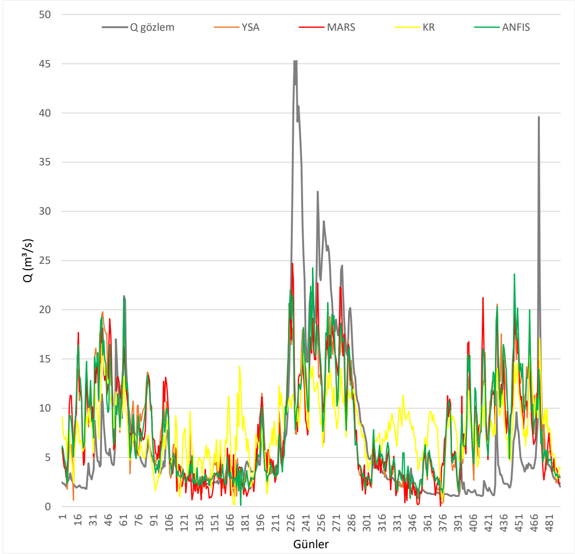
Ek Şekil 13. İkisu analiz konumunda kullanılan yöntemlere göre SPM debi tahmin performansı karşılaştırması
