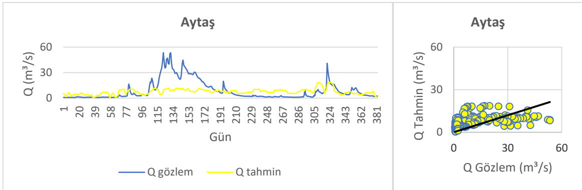
Şekil 3.34. Aytaş F2-M6 model değerlendirilmesi
