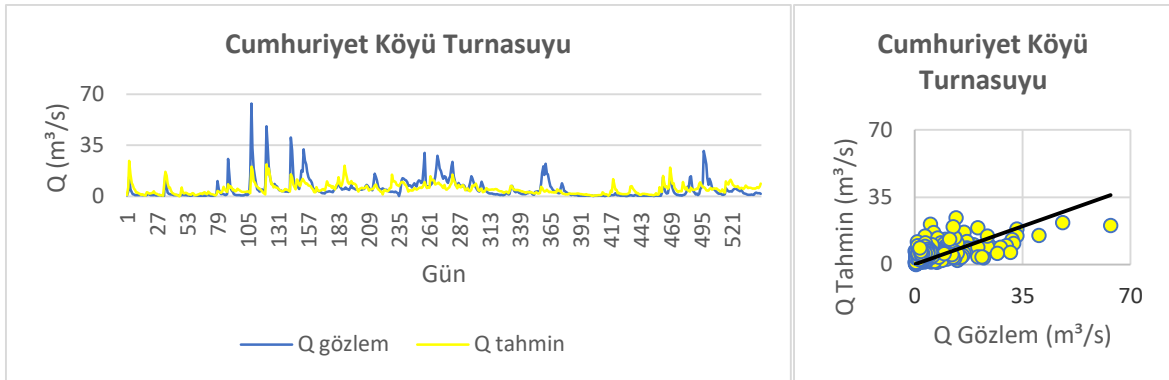
Şekil 3.70. Cumhuriyet Köyü Turnasuyu F1-M6 model değerlendirilmesi
