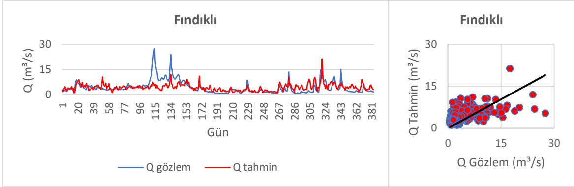
Şekil 3.29. Fındıklı MARS performans değerlendirmesi
