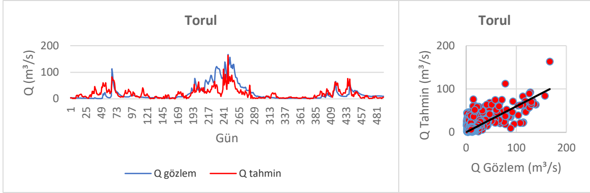
Şekil 3.25. Torul MARS performans değerlendirmesi
