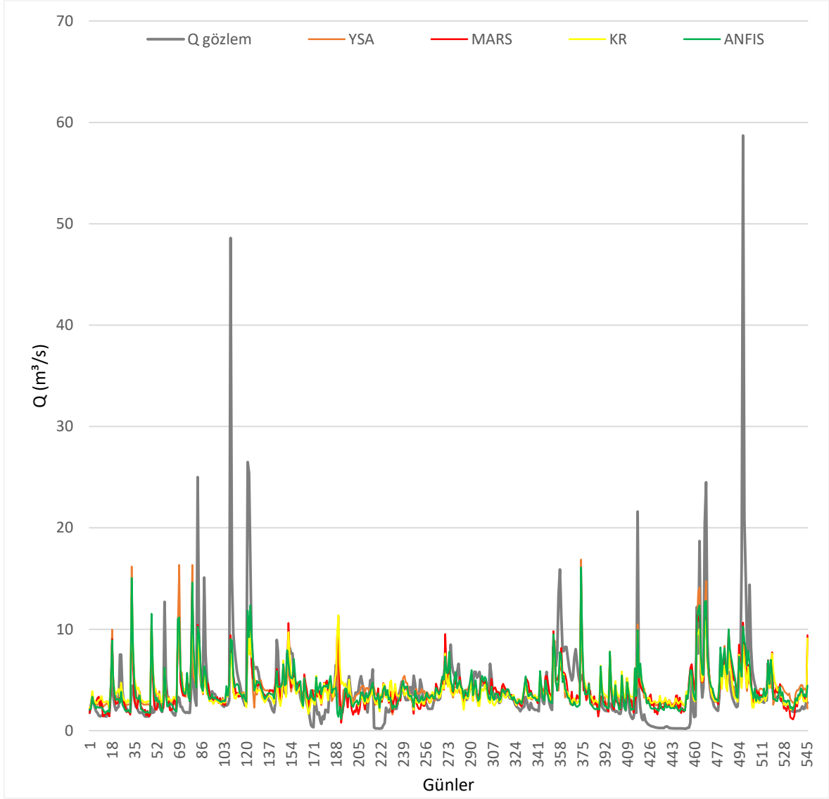
Ek Şekil 16. Kömürcüler analiz konumunda kullanılan yöntemlere göre SPM debi tahmin performansı karşılaştırması
