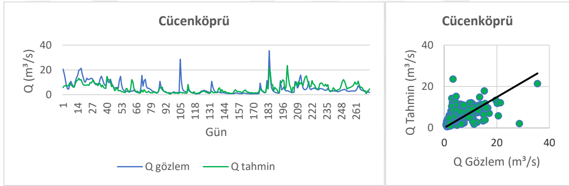
Şekil 3.39. Cücenköprü ANFIS M5 modeli performans değerlendirmesi
