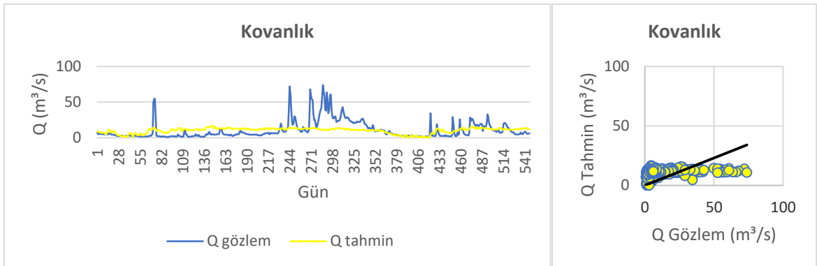
Şekil 3.50. Kovanlık F2-M1 model değerlendirme
