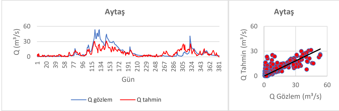
Şekil 3.33. Aytaş MARS performans değerlendirmesi
