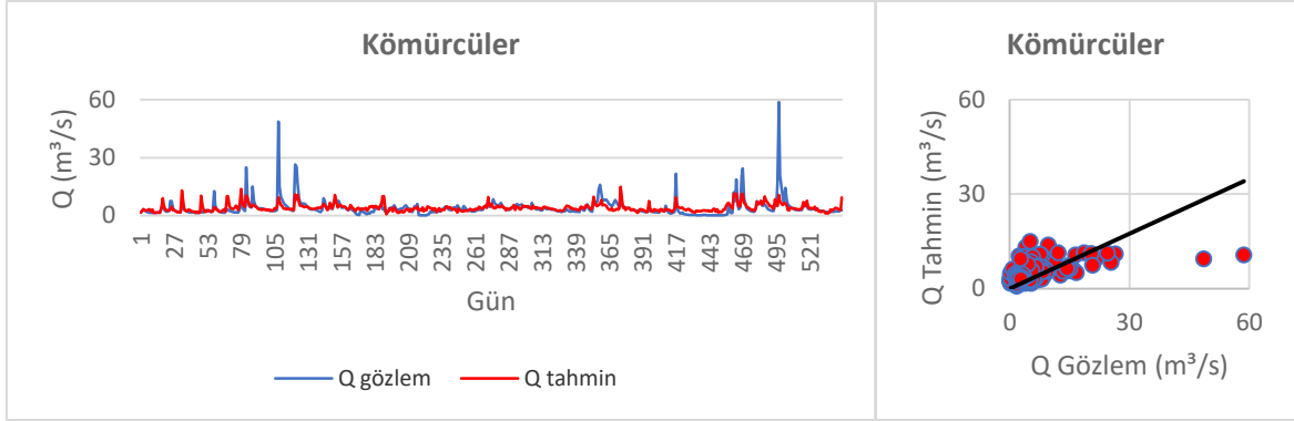
Şekil 3.65. Kömürcüler MARS performans değerlendirme
