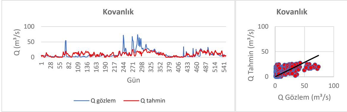
Şekil 3.49. Kovanlık MARS performans değerlendirme
