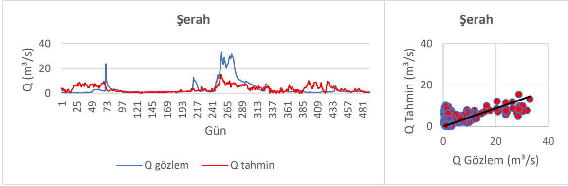
Şekil 3.21. Şerah MARS performans değerlendirilmesi
