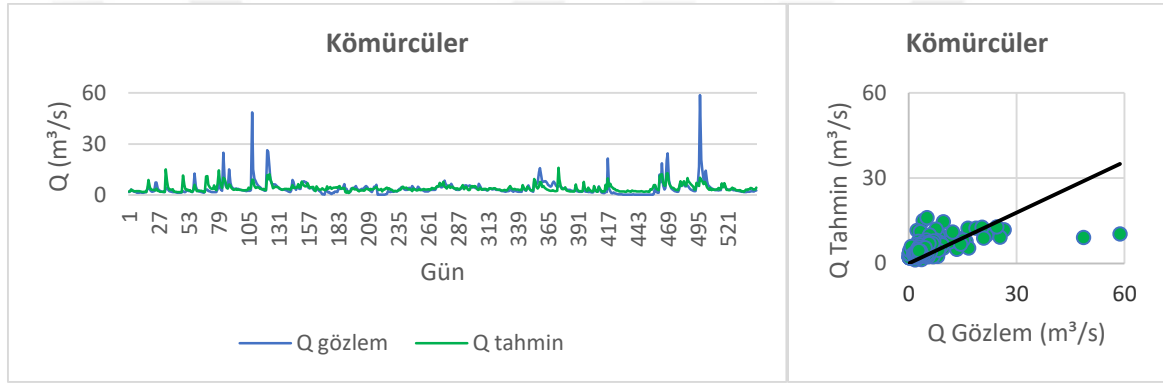
Şekil 3.67. Kömürçüler ANFIS M5 modeli performans değerlendirmesi
