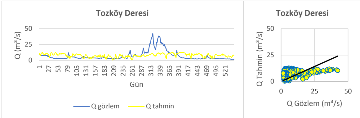
Şekil 3.10. Tozköy F2-M4 model değerlendirme
