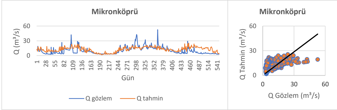
Şekil 3.44. Mikronköprü YSA M4-10 modeli değerlendirmesi
