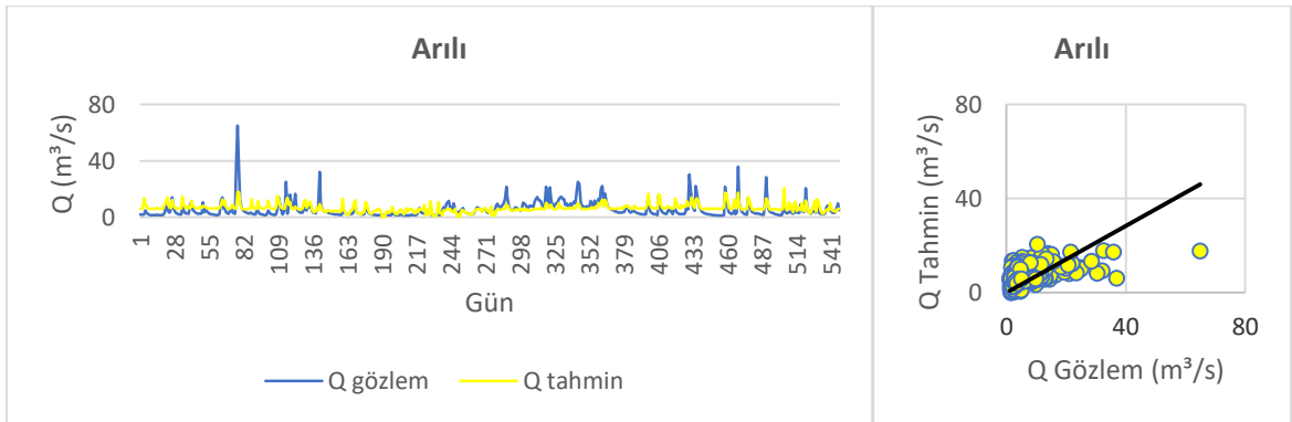
Şekil 3.58. Arılı F1-M5 model değerlendirmesi
