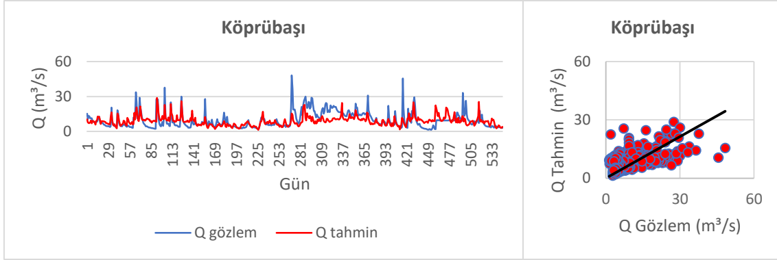
Şekil 3.17. Köprübaşı MARS performans değerlendirmesi
