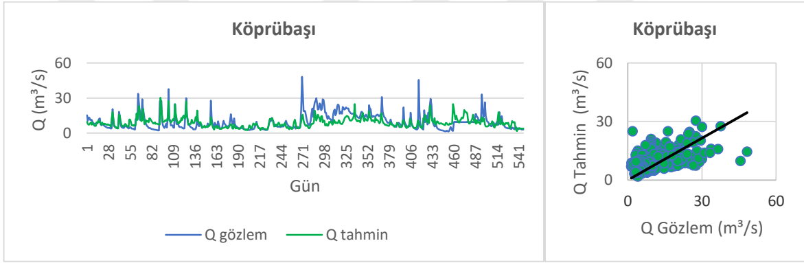
Şekil 3.19. Köprübaşı ANFIS M5 modeli performans değerlendirmesi
