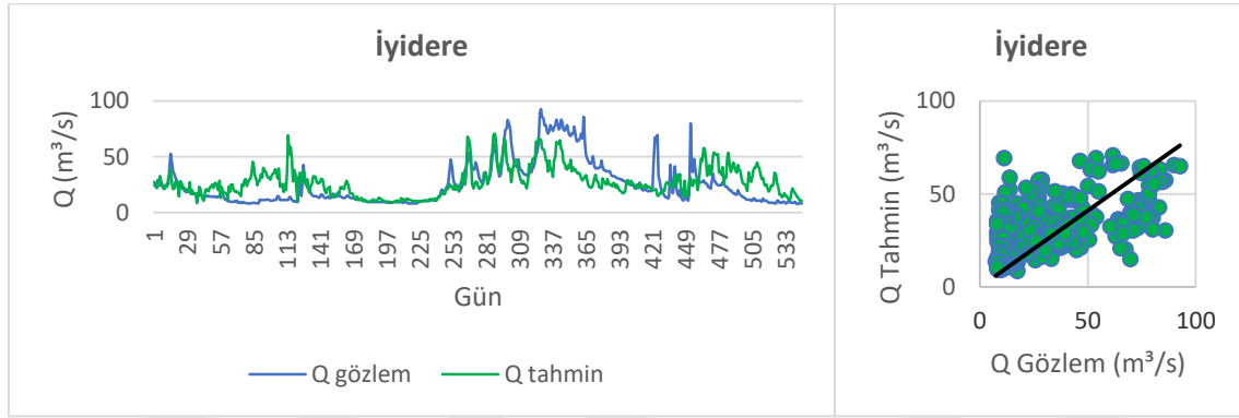
Şekil 3.7. İyidere ANFIS M5 modeli performans değerlendirmesi
