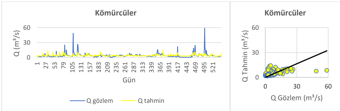
Şekil 3.66. Kömürcüler F3-M6 model değerlendirme
