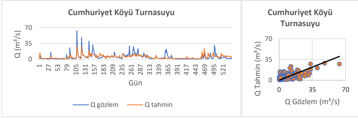
Şekil 3.68. Cumhuriyet Köyü Turnasuyu YSA M4-2 modeli değerlendirmesi
