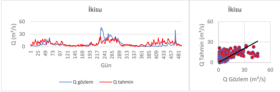
Şekil 3.53. İkisu MARS performans değerlendirmesi
