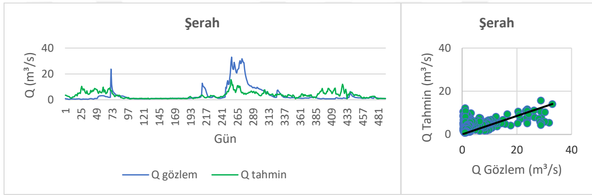
Şekil 3.23. Şerah ANFIS M5 modeli performans değerlendirmesi
