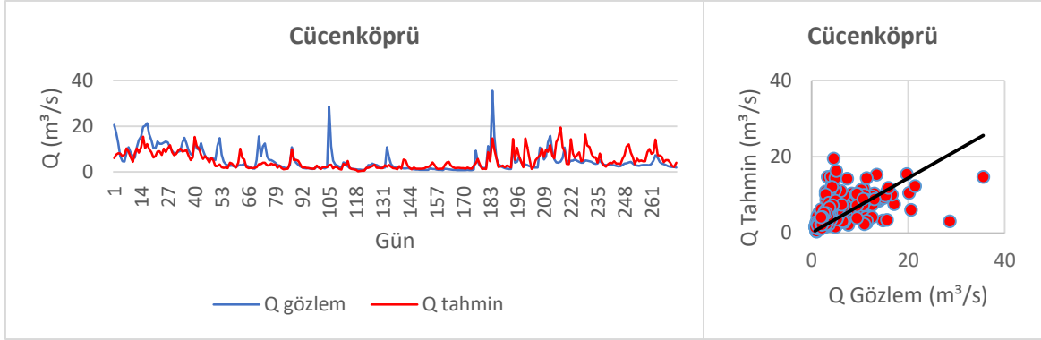
Şekil 3.37. Cücenköprü MARS performans değerlendirmesi
