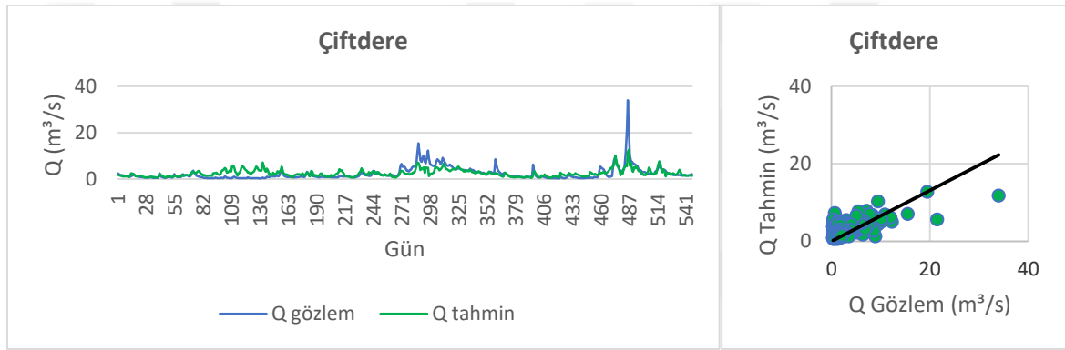
Şekil 3.43. Çiftidere ANFIS M5 modeli performans değerlendirme
