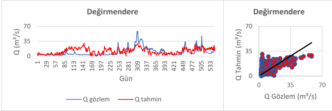
Şekil 3.13. Değirmendere MARS performans değerlendirmesi
