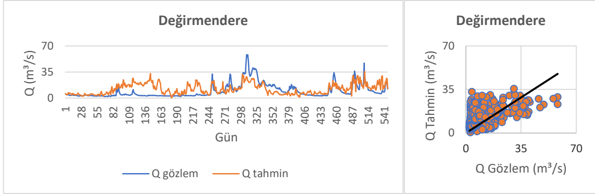
Şekil 3.12. Değirmendere YSA M4-8 modeli değerlendirmesi
