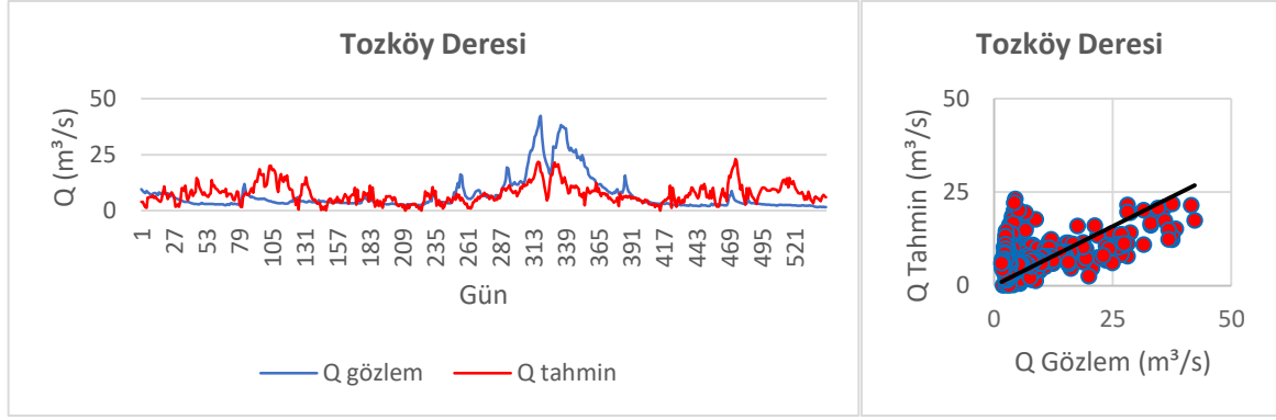
Şekil 3.9. Tozköy Deresi MARS M2 modeli performans değerlendirme
