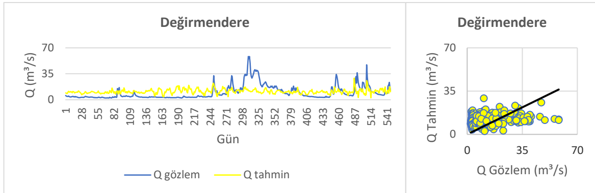
Şekil 3.14. Değirmendere F1-M4 model değerlendirmesi
