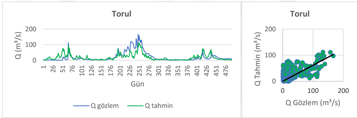
Şekil 3.27. Torul ANFIS M5 modeli performans değerlendirmesi
