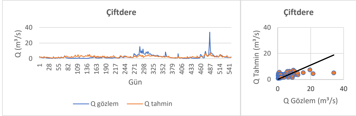
Şekil 3.40. Çiftidere YSA M6-5 modeli değerlendirilmesi
