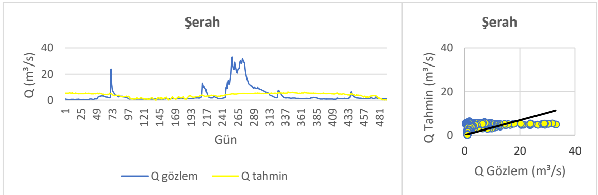
Şekil 3.22. Şerah F1-M2 model değerlendirilmesi
