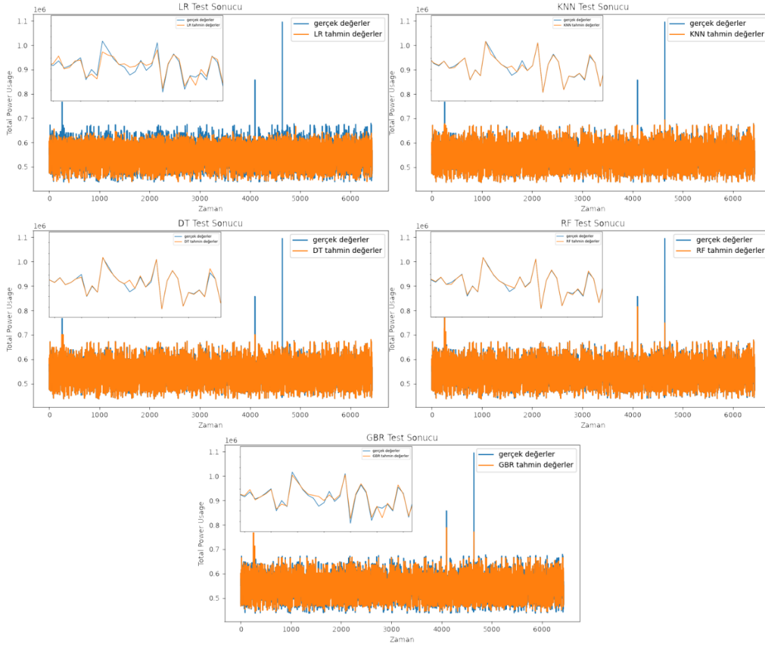
Şekil 4.1. Algoritmalarla ait tahmin grafiği.
