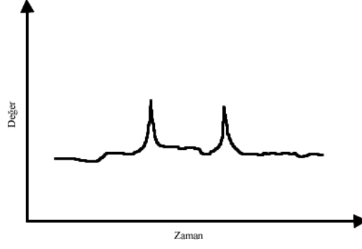
Şekil 3.1. Zaman serilerinde anomali.
