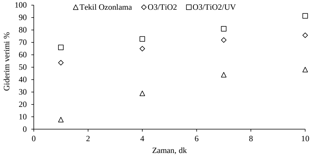
Şekil 4.30: Fotokatalitik ozonlama ve diğer proseslerin etkinliği ([E3]=100 µg/L, Katalizör dozu= 0,050 g/L, Ozon dozu= 10 mg/L, pH=6,8, Katalizör boyutu= 10 nm).
