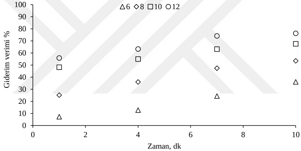
Şekil 4.19: Ozon dozlarının (mg/L) E3 giderimine etkisi ([E3]=100 µg/L, Katalizör dozu= 0,050 g/L, pH=6,8, Katalizör boyutu= 10-25 nm).
