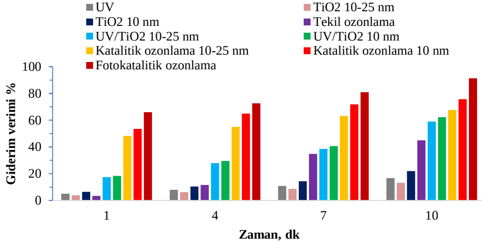
Şekil 4.11: Farklı prosesler E3 gideriminin karşılaştırılması (Optimum koşullar).
