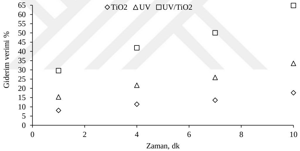
Şekil 4.39: Tekil denemeler ve fotokatalitik sistemin giderim verimine etkisi ([E1]=100 µg/L, pH= 6,8; Katalizör çapı=10-25 nm).
