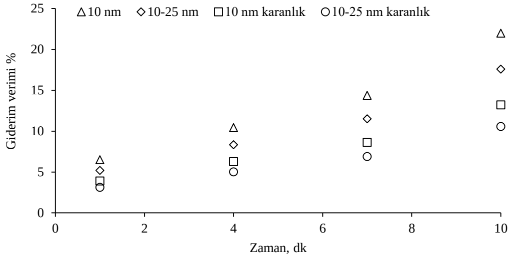
Şekil 4.33: Farklı katalizör boyutlarında karanlık ve ışıklı ortamda tekil katalizörün giderim verimine etkisi ([E3]=100 µg/L, pH= 6,8).
