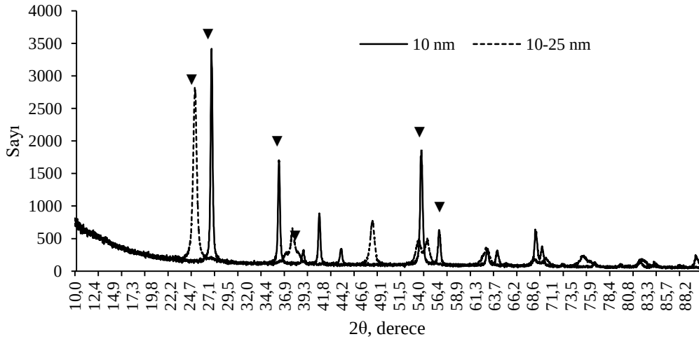
Şekil 4.1: \text{TiO}_2 maddelerinin XRD Grafiği (▼: Anataz tipi \text{TiO}_2 ).
