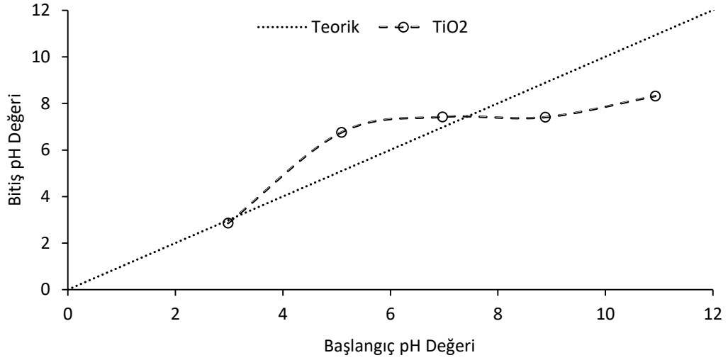
Şekil 4.3: TiO 2 katalizörünün pH pzc grafiği.
