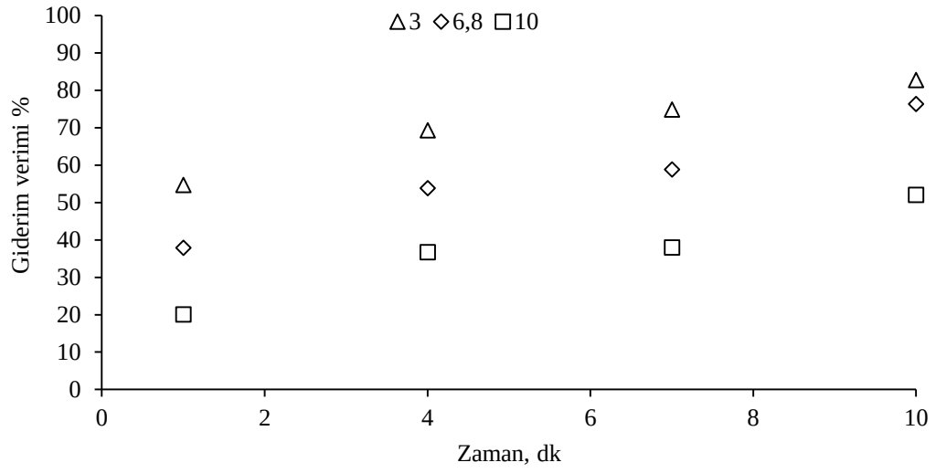
Şekil 4.21: E1 ilacının farklı pH değerlerine bağlı olarak giderim verimi ( [E1]=100 \mu\text{g/L} , Katalizör dozu= 0,050 g/L, Ozon dozu= 10 mg/L, Katalizör boyutu= 10-25 nm).
