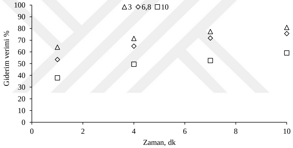
Şekil 4.22: E3 ilacının farklı pH değerlerine bağlı olarak giderim verimi ( [E3]=100 \mu\text{g/L} , Katalizör dozu= 0,050 g/L, Ozon dozu= 10 mg/L, Katalizör boyutu= 10 nm).
