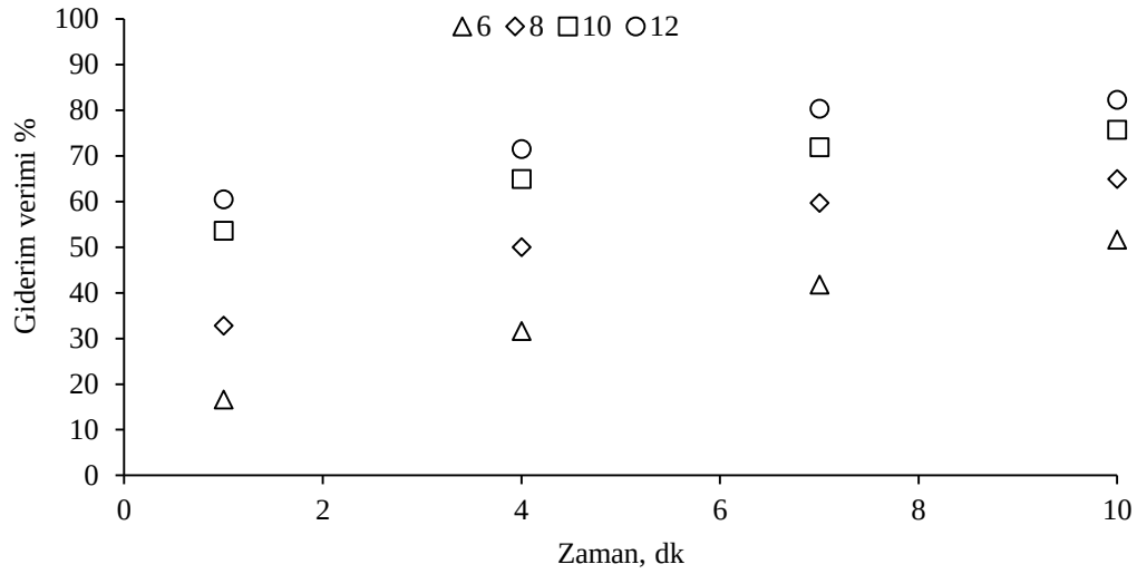
Şekil 4.18: Ozon dozlarının (mg/L) E3 giderimine etkisi ([E3]=100 µg/L, Katalizör dozu= 0,050 g/L, pH=6,8, Katalizör boyutu= 10 nm).
