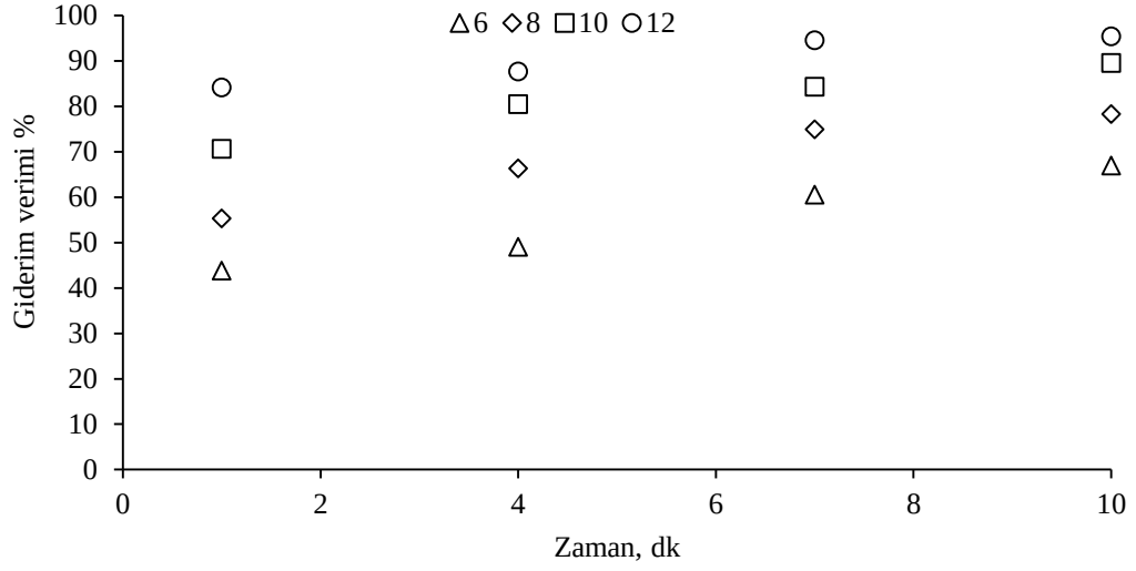
Şekil 4.16: Ozon dozlarının (mg/L) E1 giderimine etkisi ([E1]=100 µg/L, Katalizör dozu= 0,050 g/L, pH=6,8, Katalizör boyutu= 10 nm).
