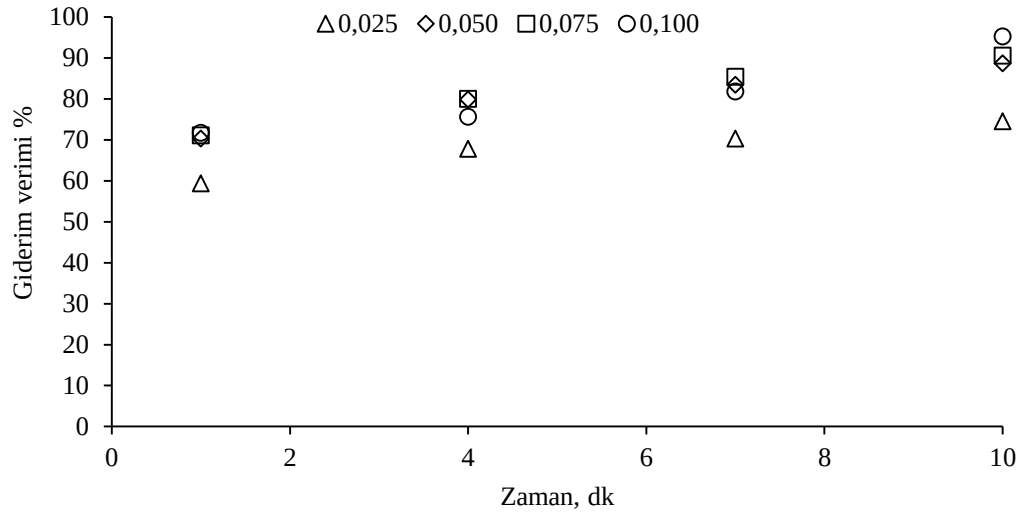
Şekil 4.13: Katalizör dozlarının (g/L) E1 giderimine etkisi ([E1]=100 µg/L, Ozon dozu= 10 mg/L, pH=6,8, Katalizör boyutu= 10-25 nm).
