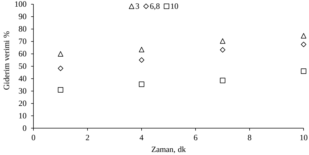
Şekil 4.23: E3 ilacının farklı pH değerlerine bağlı olarak giderim verimi ([E3]=100 µg/L, Katalizör dozu= 0,050 g/L, Ozon dozu= 10 mg/L, Katalizör boyutu= 10-25 nm).
