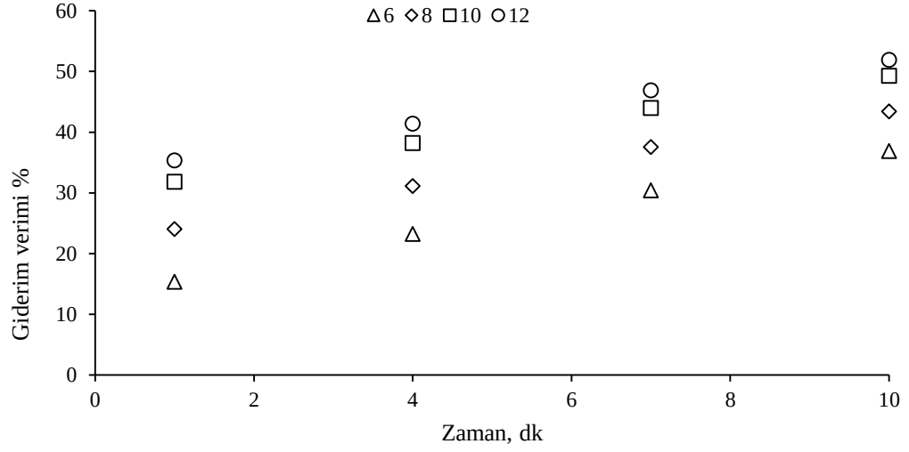
Şekil 4.8: Tekil ozonlama kontrol deneyleri ([E1]=100 µg/L, pH= 6,8).
