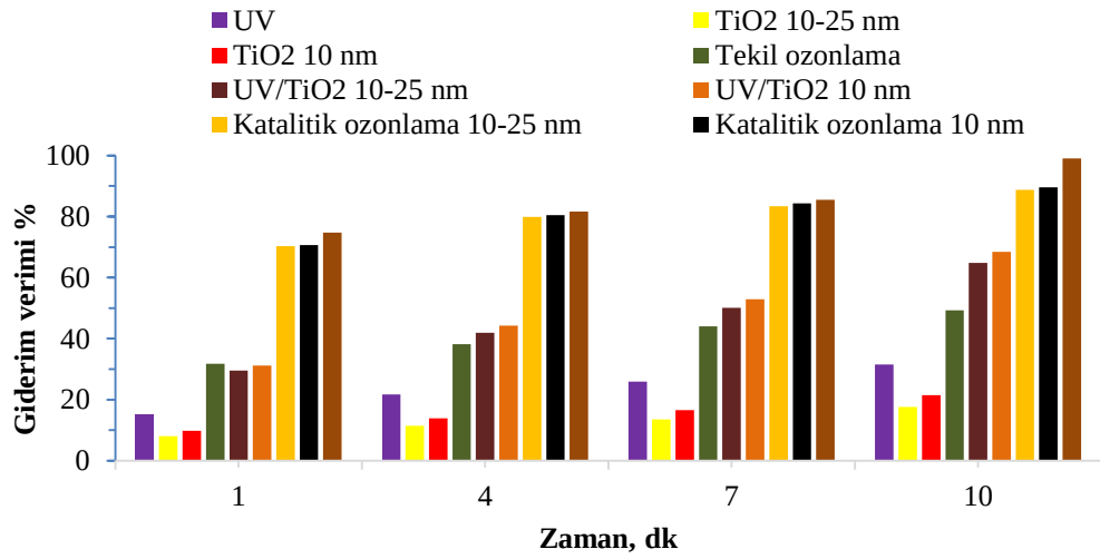
Şekil 4.10: Farklı prosesler E1 gideriminin karşılaştırılması (Optimum koşullar).
