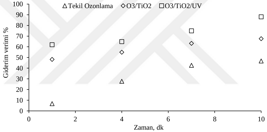
Şekil 4.31: Fotokatalitik ozonlama ve diğer proseslerin etkinliği ([E3]=100 µg/L, Katalizör dozu= 0,050 g/L, Ozon dozu= 10 mg/L, pH=6,8, Katalizör boyutu= 10-25 nm).
