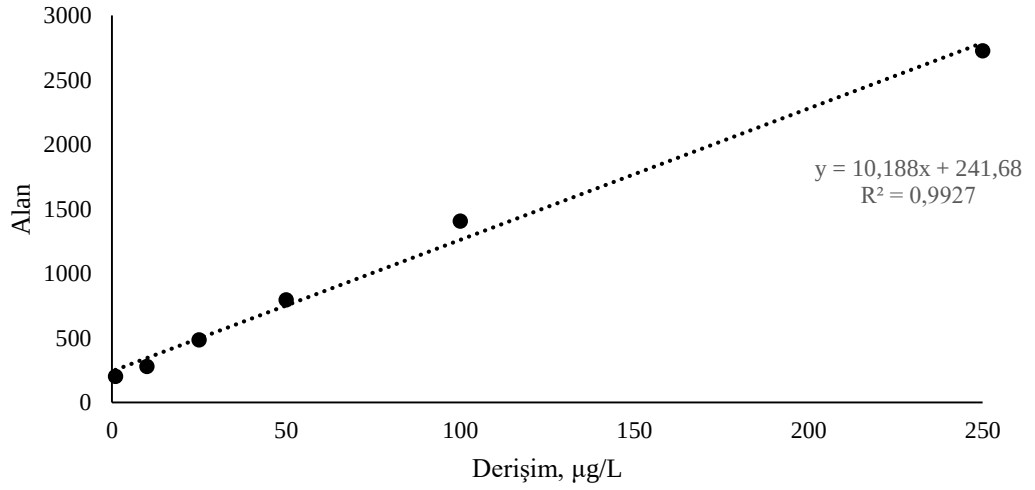
Şekil 3.2: Estrone ilacının kalibrasyonu.
