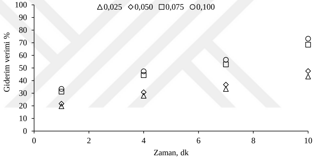
Şekil 4.34: TiO 2 10 nm katalizörünün farklı dozlarda (g/L) giderim verimine etkisi ([E1]=100 µg/L, pH= 6,8).
