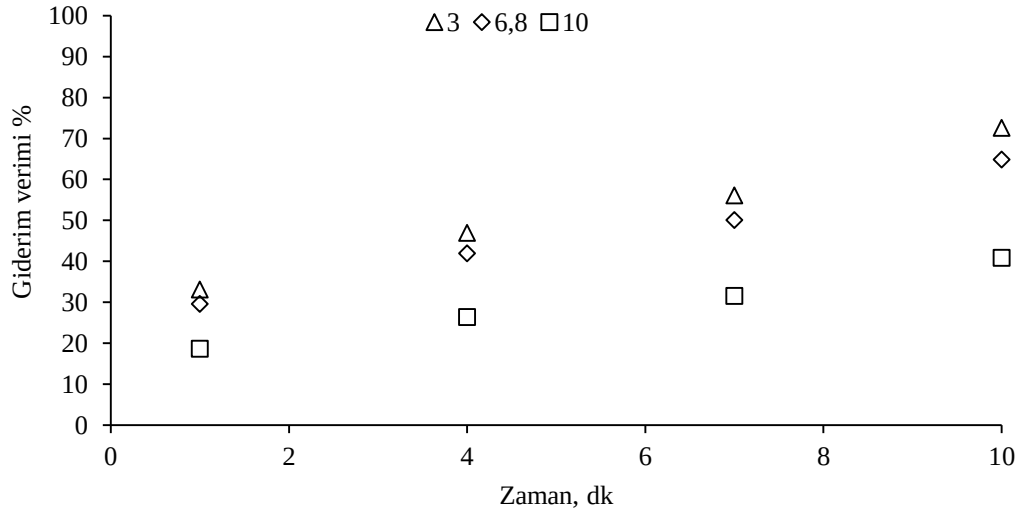
Şekil 4.41: Farklı pH değerlerinin etkisi ( [E1]=100 \mu\text{g/L} , Katalizör dozu= 0,075 \text{ g/L} Katalizör çapı= 10-25 \text{ nm} ).
