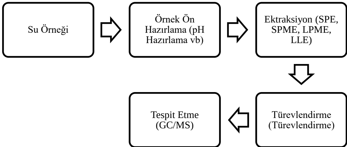
Şekil 3.1: Analitik prosedür.
