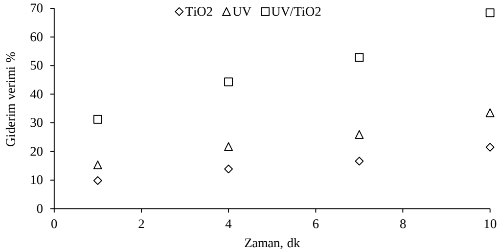
Şekil 4.38: Tekil denemeler ve fotokatalitik sistemin giderim verimine etkisi ([E1]=100 µg/L, pH= 6,8; Katalizör çapı=10 nm).
