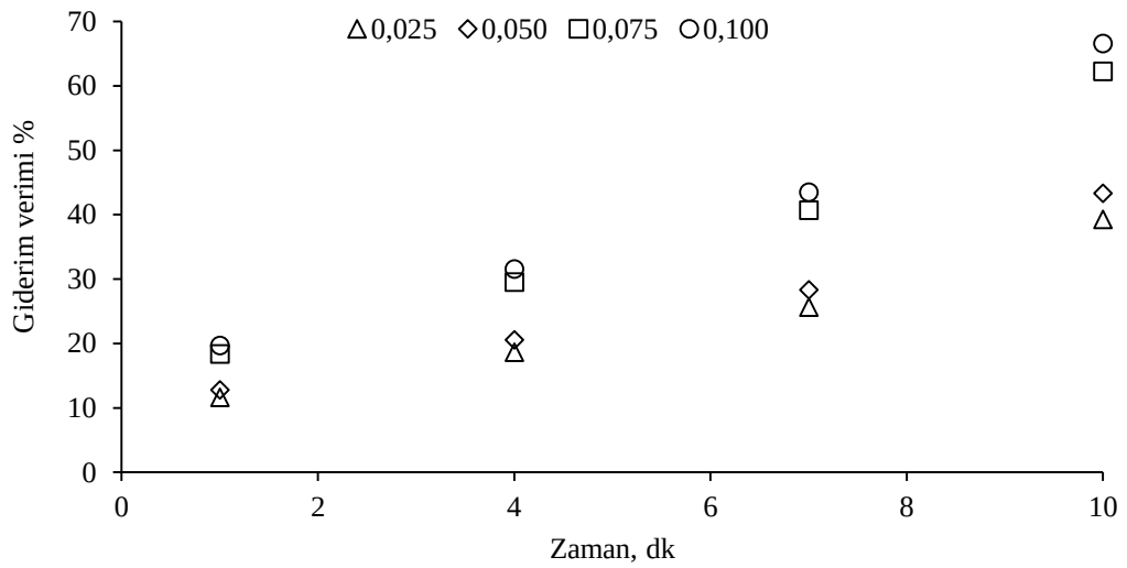
Şekil 4.35: TiO 2 10 nm katalizörünün farklı dozlarda (g/L) giderim verimine etkisi ([E3]=100 µg/L, pH= 6,8).
