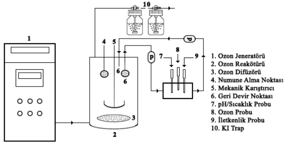
Şekil 3.7: Deney düzeneği.
