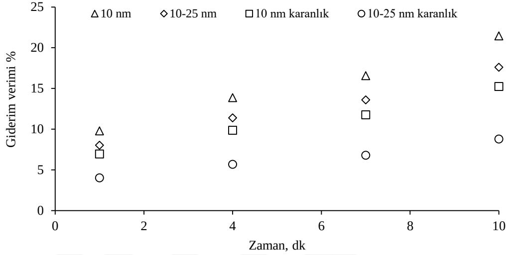
Şekil 4.6: Tekil adsorpsiyon kontrol deneyleri ([E1]=100 \mu\text{g/L} , Katalizör dozu= 0,050 g/L, pH= 6,8).
