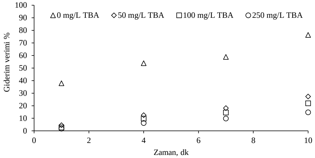
Şekil 4.26: Katalitik ozonlama prosesine TBA etkisi ( [E1]=100 \mu\text{g/L} , Katalizör dozu= 0,050 g/L, Ozon dozu= 10 mg/L, pH=6,8, Katalizör boyutu= 10-25 nm).
