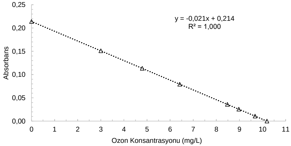
Şekil 3.5: Ozon kalibrasyon eğrisi.
