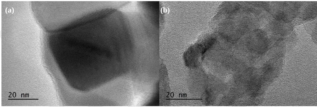
Şekil 4.5: Kullanılan katalizörlerin TEM görüntüleri; (a) TiO 2 10nm (b) TiO 2 10-25nm.
