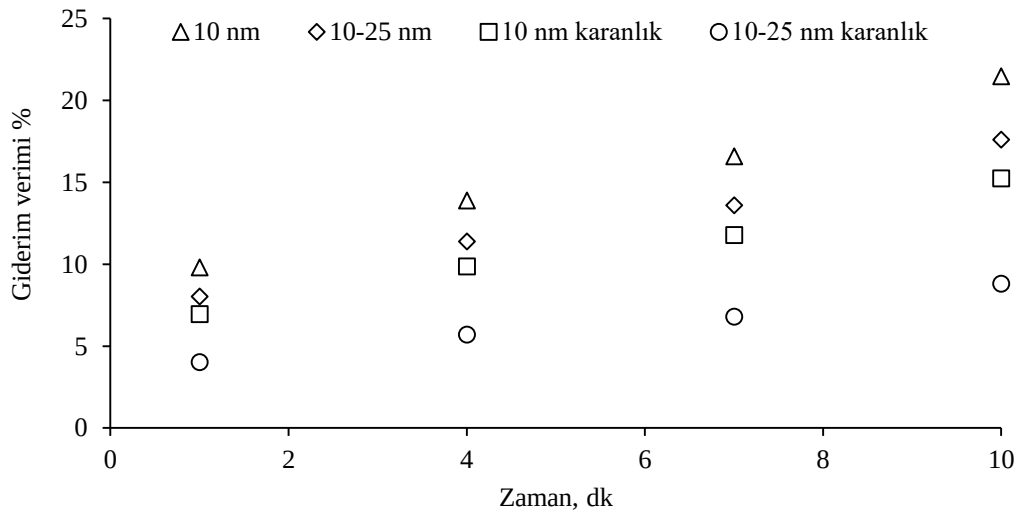
Şekil 4.32: Farklı katalizör boyutlarında karanlık ve ışıklı ortamda tekil katalizörün giderim verimine etkisi ( [E1]=100 \mu\text{g/L} , \text{pH}=6,8 ).
