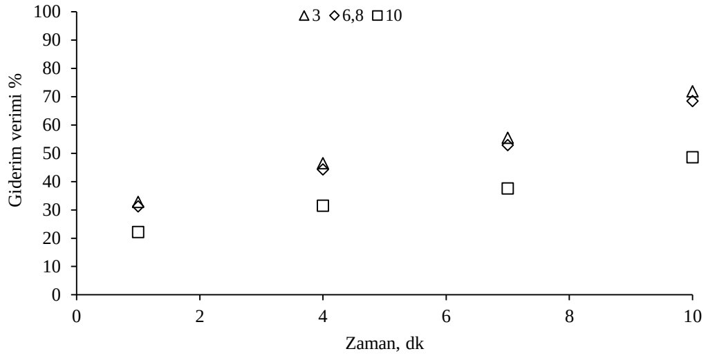
Şekil 4.40: Farklı pH değerlerinin etkisi ( [E1]=100 \mu\text{g/L} , Katalizör dozu= 0,075 \text{ g/L} Katalizör çapı= 10 \text{ nm} ).
