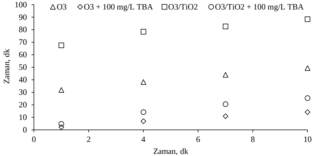
Şekil 4.25: Ozonlama ve katalitik ozonlama prosesine TBA etkisi ([E1]=100 µg/L, Katalizör dozu= 0,050 g/L, Ozon dozu= 10 mg/L, pH=6,8, Katalizör boyutu= 10 nm).
