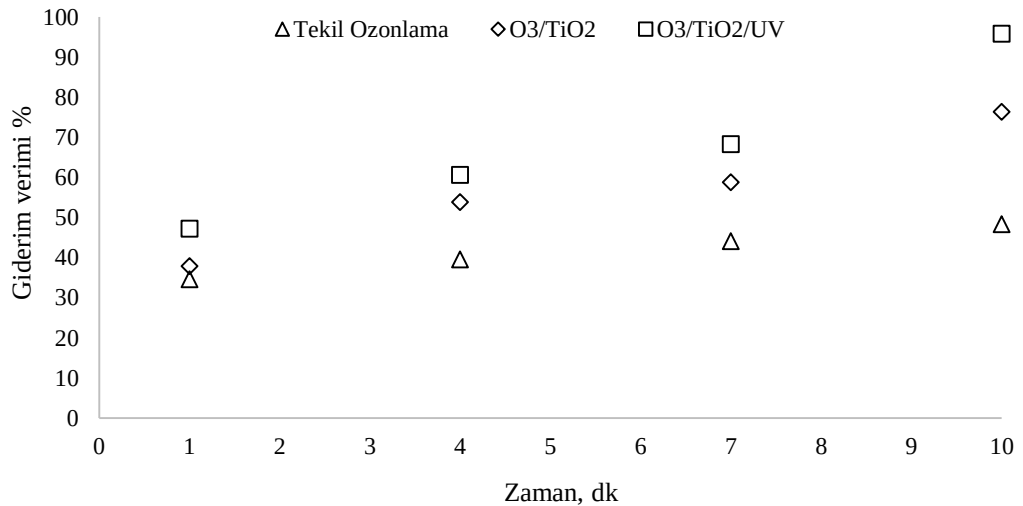
Şekil 4.29: Fotokatalitik ozonlama ve diğer proseslerin etkinliği ([E1]=100 µg/L, Katalizör dozu= 0,050 g/L, Ozon dozu= 10 mg/L, pH=6,8, Katalizör boyutu= 10-25 nm).
