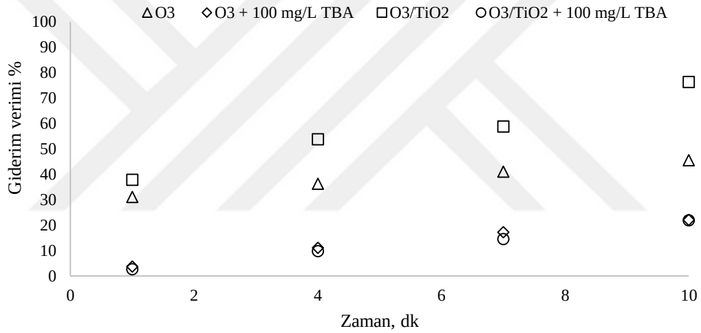
Şekil 4.27: Ozonlama ve katalitik ozonlama prosesine TBA etkisi ( [E1]=100 \mu\text{g/L} , Katalizör dozu= 0,050 g/L, Ozon dozu= 10 mg/L, pH=6,8, Katalizör boyutu= 10-25 nm).
