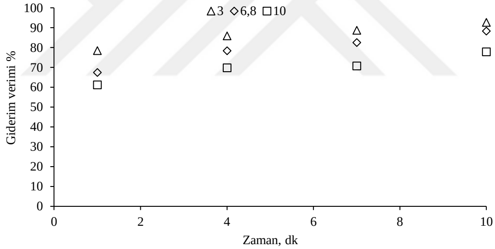
Şekil 4.20: E1 ilacının farklı pH değerlerine bağlı olarak giderim verimi ([E1]=100 µg/L, Katalizör dozu= 0,050 g/L, Ozon dozu= 10 mg/L, Katalizör boyutu= 10 nm).
