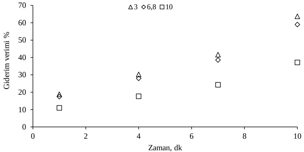
Şekil 4.43: Farklı pH değerlerinin etkisi ([E3]=100 µg/L,Katalizör dozu=0,075 g/L Katalizör çapı=10-25 nm).
