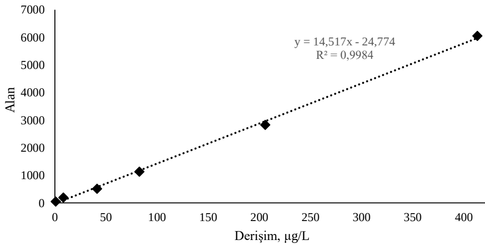
Şekil 3.3: Estriol ilacının kalibrasyonu.
