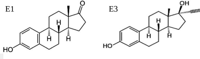
Şekil 2.1: E1 ve E3 ilaçlarının molekül yapıları.
