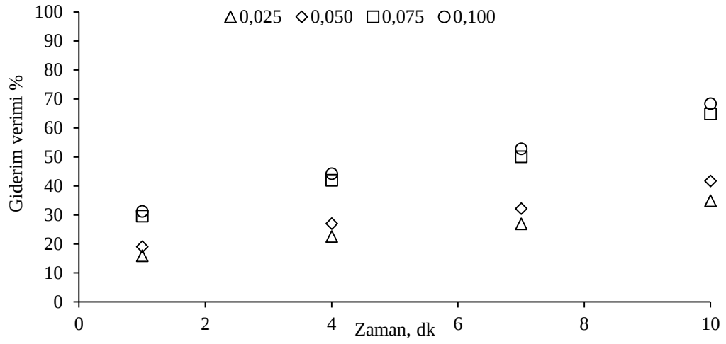
Şekil 4.36: \text{TiO}_2 10-25 nm katalizörünün farklı dozlarda (g/L) giderim verimine etkisi ([E1]=100 µg/L, pH= 6,8).
