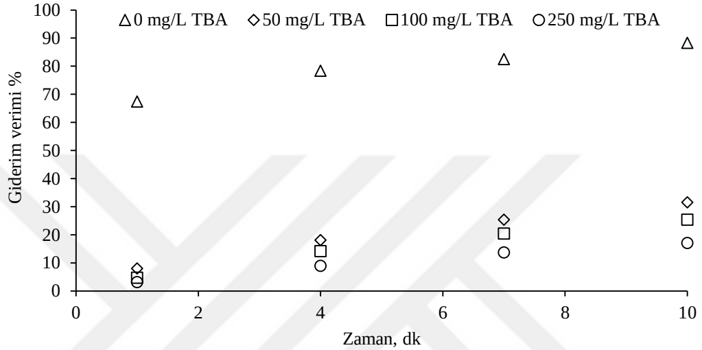
Şekil 4.24: Katalitik ozonlama prosesine TBA etkisi ([E1]=100 µg/L, Katalizör dozu= 0,050 g/L, Ozon dozu= 10 mg/L, pH=6,8, Katalizör boyutu= 10 nm).
