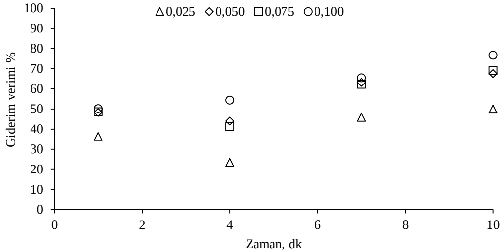
Şekil 4.15: Katalizör dozlarının (g/L) E3 giderimine etkisi ([E3]=100 µg/L, Ozon dozu= 10 mg/L, pH=6,8, Katalizör boyutu= 10-25 nm).
