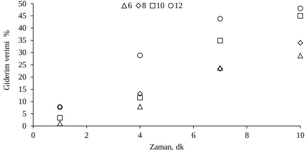
Şekil 4.9: Tekil ozonlama kontrol deneyleri ([E3]=100 µg/L, pH= 6,8).
