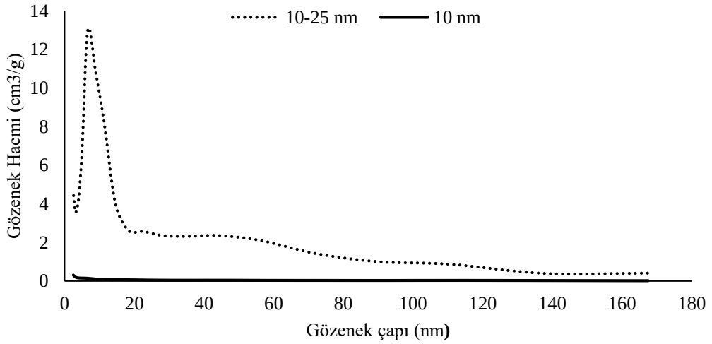
Şekil 4.4: BET ve DIS analizi.
