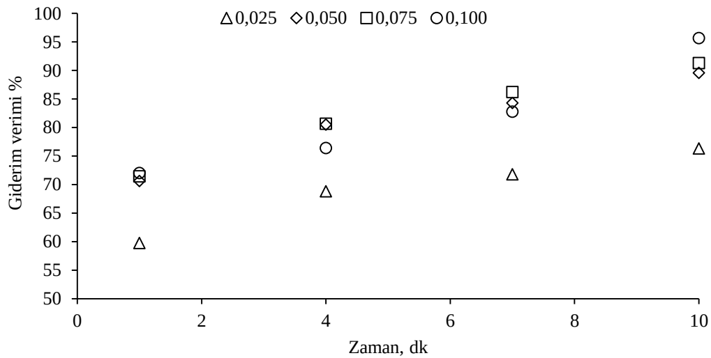
Şekil 4.12: Katalizör dozlarının (g/L) E1 giderimine etkisi ([E1]=100 µg/L, Ozon dozu= 10 mg/L, pH=6,8, Katalizör boyutu= 10 nm).
