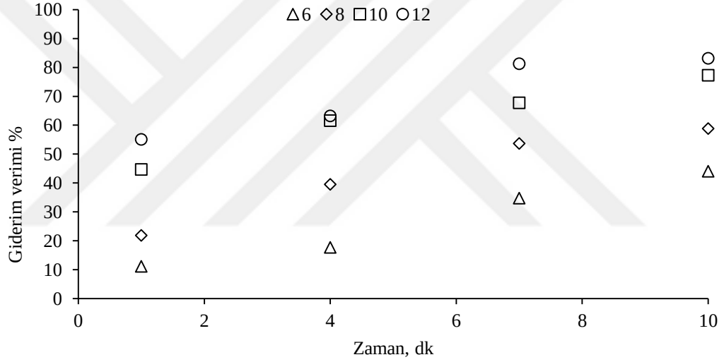
Şekil 4.17: Ozon dozlarının (mg/L) E1 giderimine etkisi ([E1]=100 µg/L, Katalizör dozu= 0,050 g/L, pH=6,8, Katalizör boyutu= 10-25 nm).
