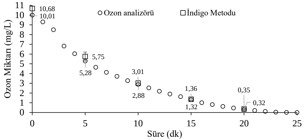
Şekil 3.6: Ozon analizi için metotların kıyaslanması.
