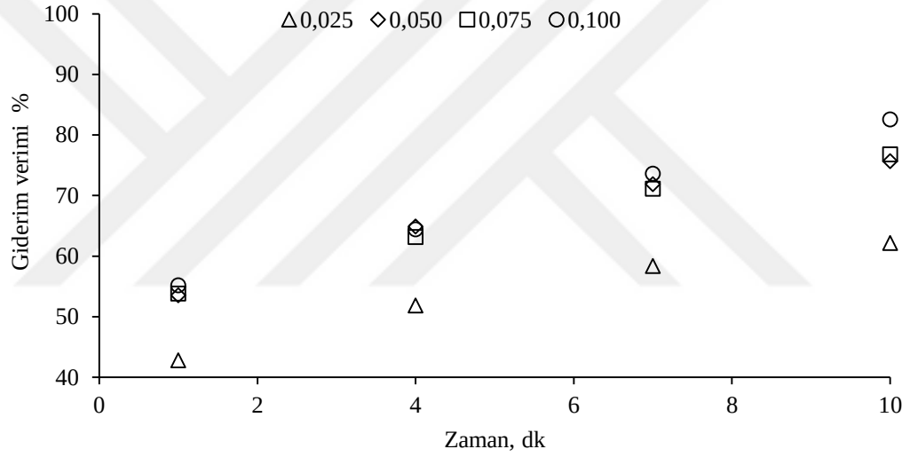
Şekil 4.14: Katalizör dozlarının (g/L) E3 giderimine etkisi ([E3]=100 µg/L, Ozon dozu= 10 mg/L, pH=6,8, Katalizör boyutu= 10 nm).
