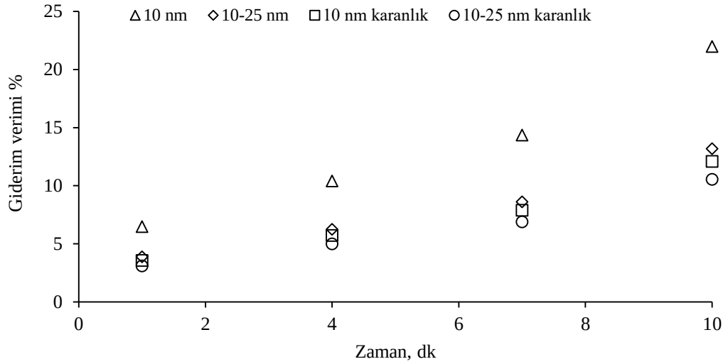
Şekil 4.7: Tekil adsorpsiyon kontrol deneyleri ([E3]=100 \mu\text{g/L} , Katalizör dozu= 0,050 g/L, pH= 6,8).
