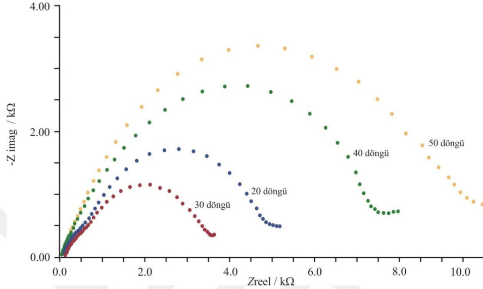
Şekil 4.15: Farklı film kalınlıklarında elde edilen PAni–kitosan kompozit yapılarının 0,5 M H 2 SO 4 çözeltisinde kaydedilen Nyquist diyagramları.
