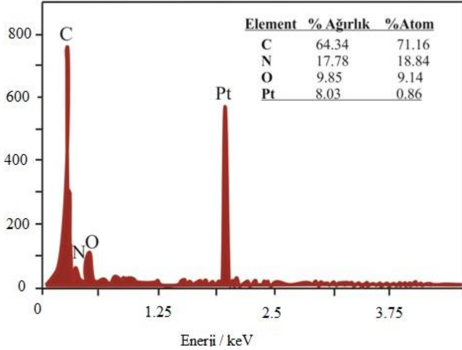
Şekil 4.2: Grafit/PANi–kitosan/Pt kompozit yapısının enerji dağılım spektrumu (EDS).
