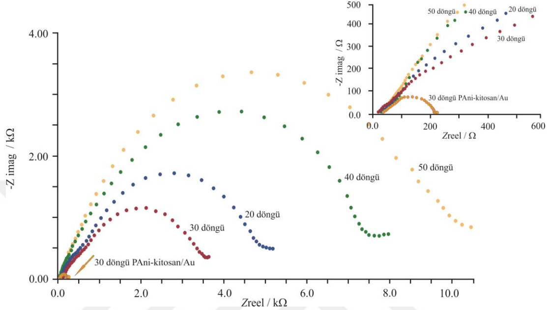
Şekil 4.16: Farklı film kalınlıklarında elde edilen PANi–kitosan kompozit yapıların ve 30 döngülük PANi–kitosan kompozit yapı üzerine Au nano parçacıklarının elektrodpozisyonuyla elde edilen kompozit yapının 0,5 M H 2 SO 4 çözeltisinde kaydedilen Nyquist diyagramları (inset diyagram).
