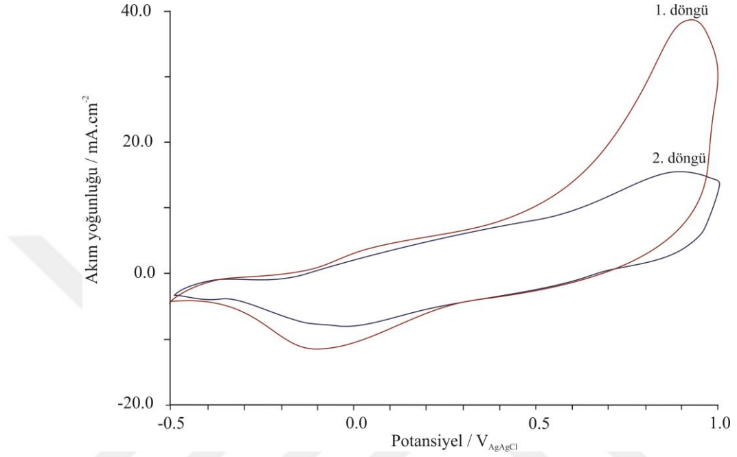
Şekil 3.12: Altın nanopartiküllerinin PPy–kitosan filmi üzerine 0,5 M H 2 SO 4 içerisinde elektrodepozisyonu ( v=50\text{mV.s}^{-1} ).
