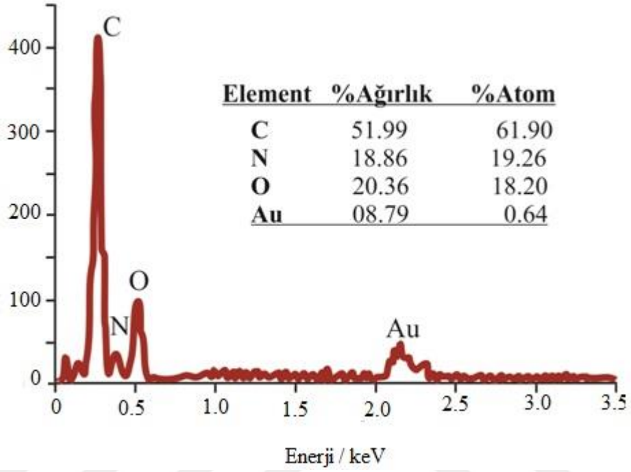
Şekil 4.9: Grafit/PPy–kitosan/Au yapısının enerji dağılım spektrumu (EDS).
