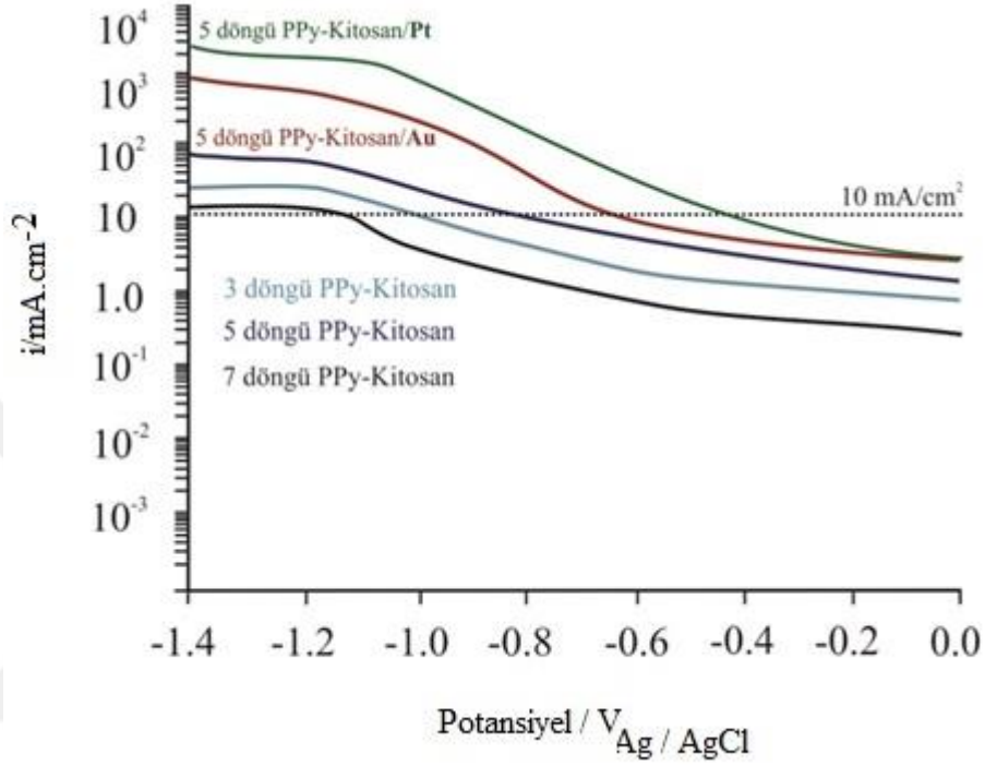
Şekil 4.23: Farklı döngü sayılarında PPy–kitosan, 5 döngü PPy–kitosan/Pt ve PPy–kitosan/Au kompozit yapılarının 0,5 M H 2 SO 4 çözeltisinde Tafel polarizasyon eğrileri ( v=1\text{mV.s}^{-1} ).
