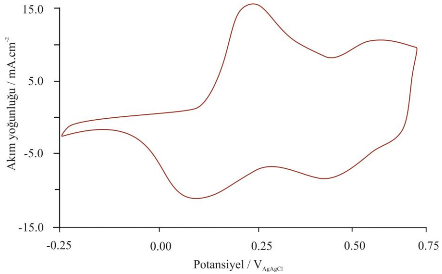
Şekil 3.8: PANi–kitosan /Pt kompozit filminin 0,5 M \text{H}_2\text{SO}_4 içerisinde kaydedilen temel diyagramı ( v=50\text{mV.s}^{-1} ).
