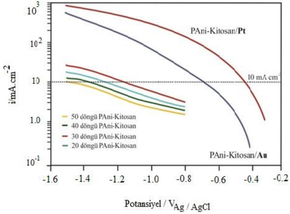
Şekil 4.14: Farklı döngü sayılarında PANi–kitosan, 30 döngü PANi–kitosan /Pt ve PANi–kitosan/Au kompozit yapılarının 0,5 M H 2 SO 4 çözeltisinde Tafel polarizasyon eğrileri ( v=1\text{mV.s}^{-1} ).
