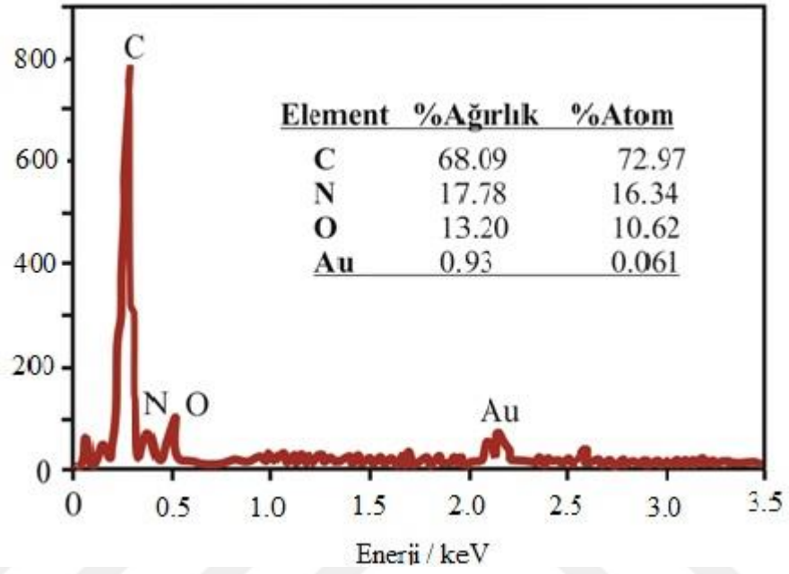
Şekil 4.4: Grafit/PANi–kitosan/Au yapısının enerji dağılım spektrumu (EDS).
