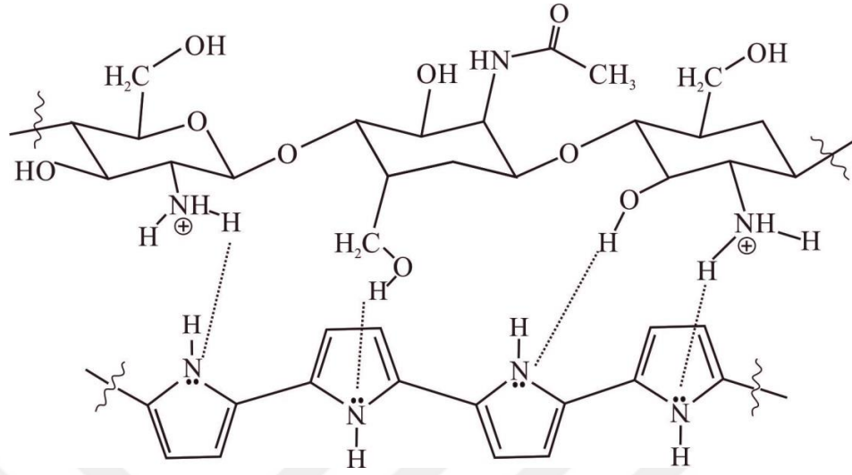
Şekil 3.11: PPy–kitosan kompozit yapısı.
