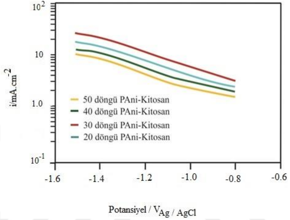
Şekil 4.13: Farklı döngü sayılarında PANi–kitosan kompozit yapılarının 0,5 M H_2SO_4 çözeltisinde Tafel polarizasyon eğrileri ( v=1mV.s^{-1} ).
