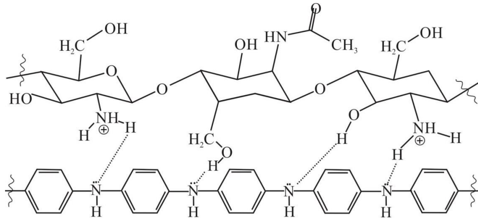
Şekil 3.4: PANi–kitosan kompozit yapısı.
