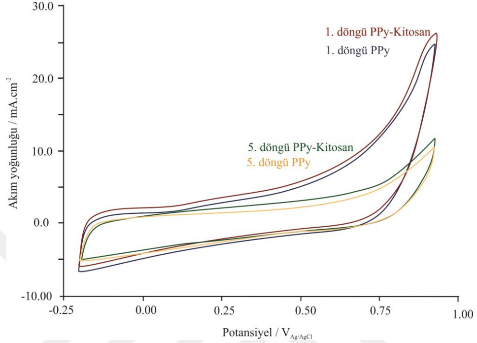
Şekil 3.10: PPy ve PPy–kitosan filmlerinin 0,3 M H 2 C 2 O 4 içerisinde kaydedilen temel diyagramları ( v=50\text{mV.s}^{-1} ).
