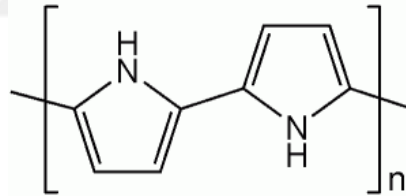
Şekil 2.5: Polipirolün kimyasal yapısı.
