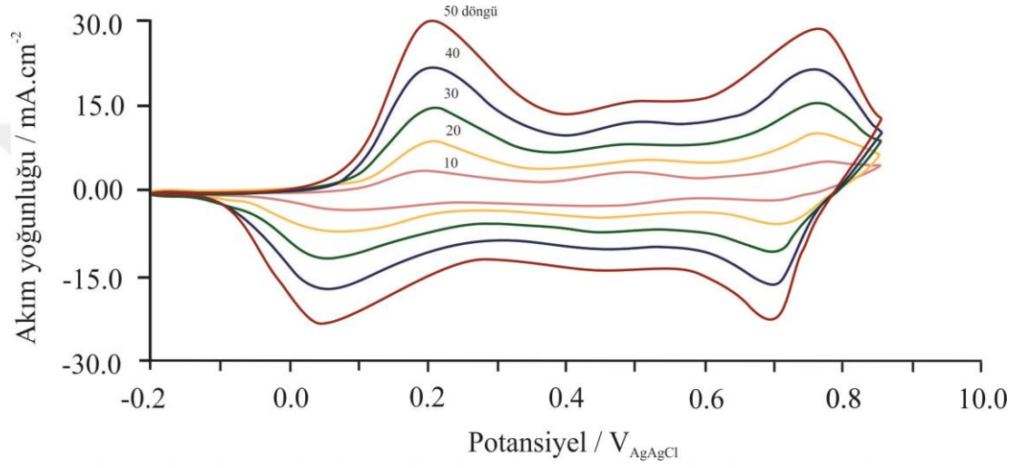
Şekil 3.2: PANi–kitosan kompozit yapısının kalem grafit elektrot üzerine 0,5 \text{ M H}_2\text{SO}_4 içerisinde elektropolimerizasyonu ( v=50\text{mV.s}^{-1} ).
