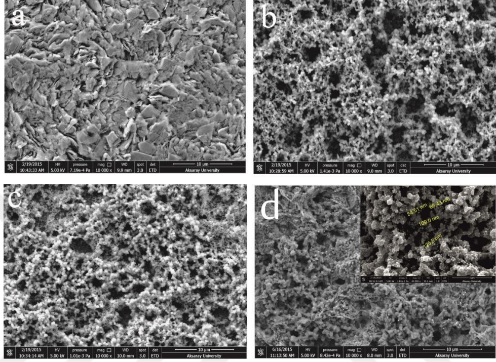
Şekil 4.3: a) Çıplak grafit b) Grafit/PANi c) Grafit/PANi–kitosan d) Grafit/PANi–kitosan/Au yapılarının taramalı elektron mikroskobu (SEM) görüntüleri.
