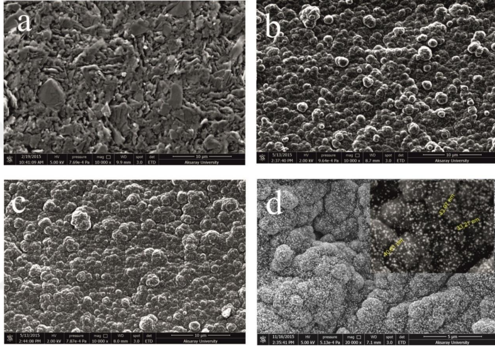
Şekil 4.6: a) Çıplak grafit b) Grafit/PPy c) Grafit/PPy–kitosan d) Grafit/PPy–kitosan/Pt yapılarının taramalı elektron mikroskobu (SEM) görüntüleri.
