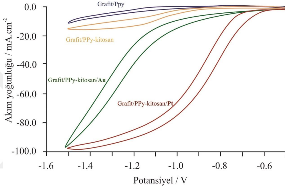
Şekil 4.21: Beş döngü sonucunda hazırlanan PPy–kitosan, PPy–kitosan/Au ve PPy–kitosan/Pt kompozit yapılarının 0,5 M H 2 SO 4 elektrolit ortamında kaydedilen dönüşümlü voltamogramları ( v=20 \text{ mV.s}^{-1} ).
