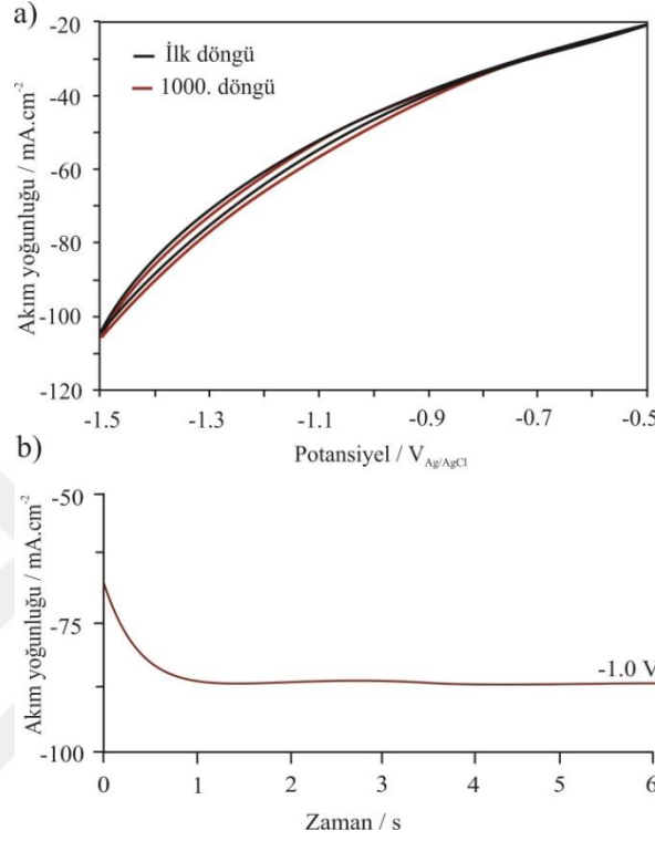
Şekil 4.19: Grafit elektrot üzerine kaplanmış PAni–kitosan/Pt kompozit filminin 0,5M H 2 SO 4 elektrolit ortamında kaydedilen a) İlk ve 1000 döngü sonucundaki dönüşümlü voltamogramları b) -1,0V sabit potansiyelde elde edilen kronoamperogramı.
