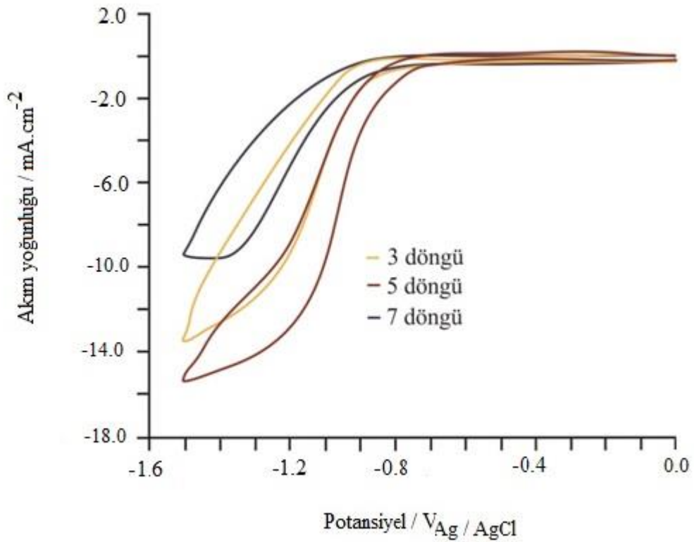
Şekil 4.20: Farklı döngü sayılarında hazırlanan PPY–kitosan kompozit yapılarının 0,5 M H 2 SO 4 elektrolit ortamında kaydedilen dönüşümlü voltamogramları ( v=20\text{mV.s}^{-1} ).
