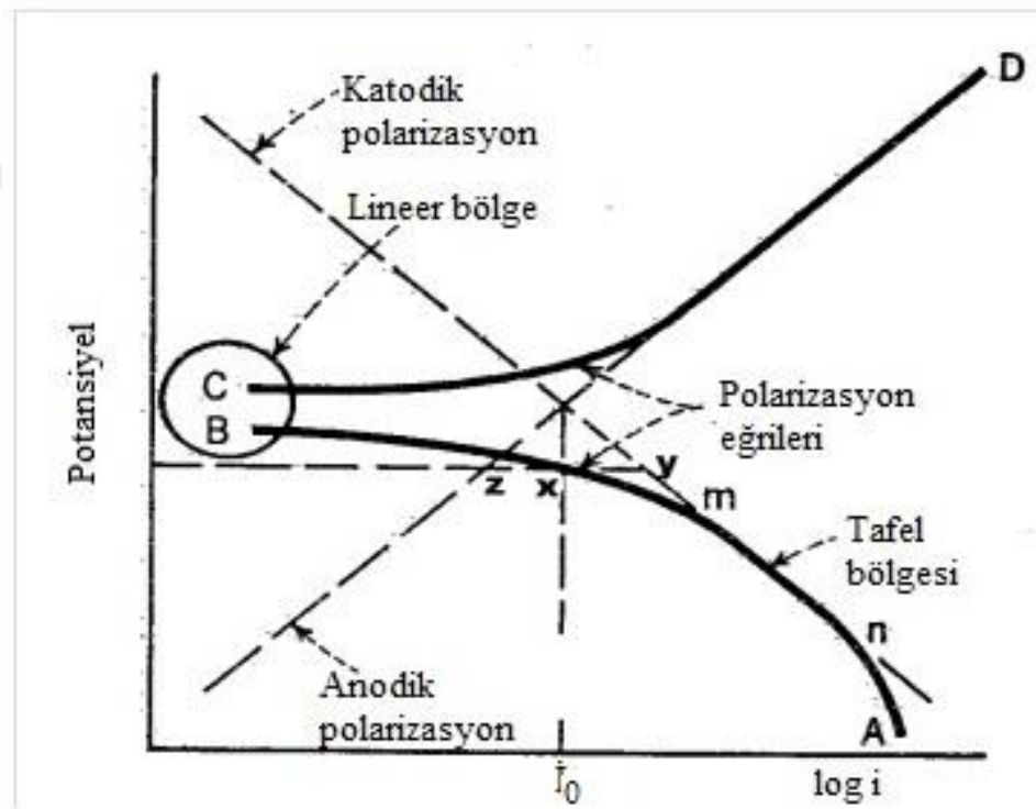
Şekil 2.9: Anodik ve katodik polarizasyon eğrileri.
