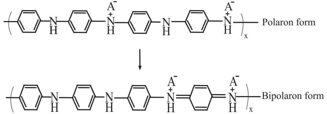
Şekil 2.4: Polianilinin kararlı rezonans sınır formülleri
