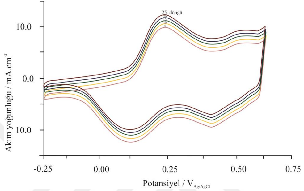
Şekil 3.7: PANi–kitosan filmi üzerine Pt nanopartiküllerinin 0,5 M \text{H}_2\text{SO}_4 içerisinde elektrodpozisyonu ( v=50\text{mV.s}^{-1} ).
