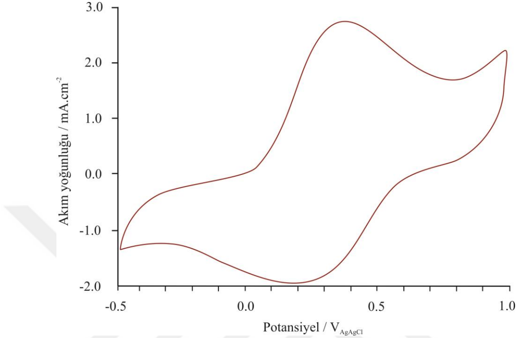
Şekil 3.13: PPy–kitosan/Au kompozit filmin 0,5 M H 2 SO 4 içerisinde kaydedilen temel diyagramı ( v=50\text{mV.s}^{-1} ).
