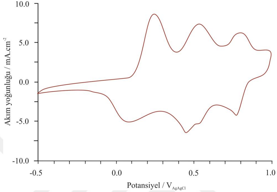
Şekil 3.6: PANi–kitosan/Au kompozit filmin 0,5 M H 2 SO 4 içerisinde kaydedilen temel diyagramı ( v=50\text{mV.s}^{-1} ).
