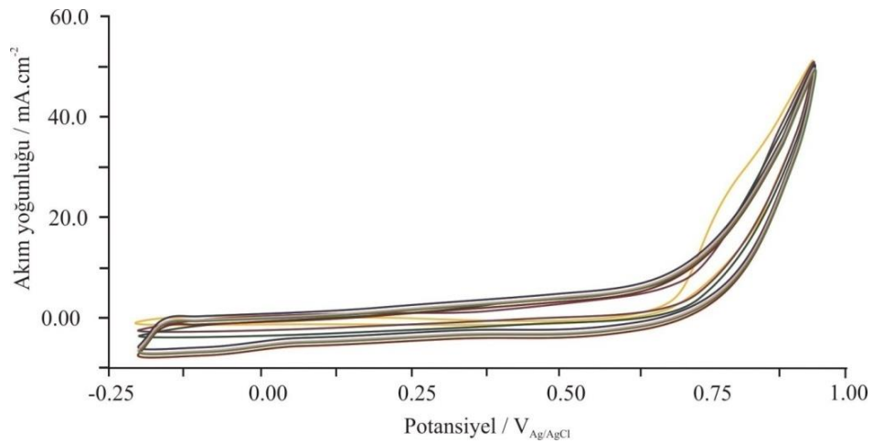
Şekil 3.9: PPy–kitosan kompozit yapısının kalem grafit elektrot üzerine elektropolimerizasyonu ( v=50\text{mV.s}^{-1} ).
