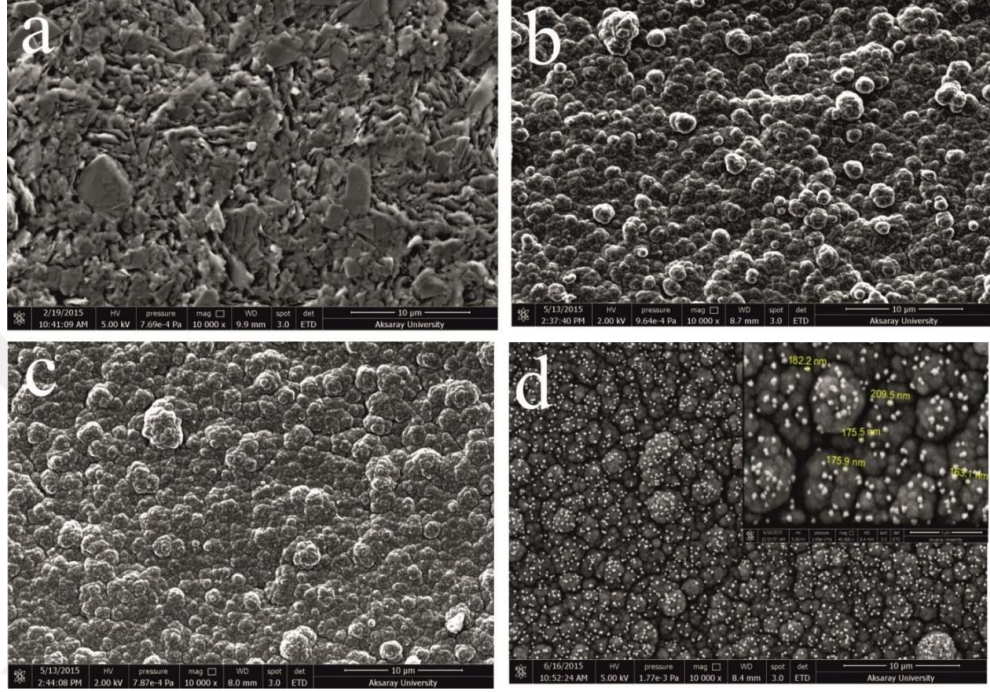
Şekil 4.8: a) Çıplak grafit b) Grafit/PPy c) Grafit/PPy–kitosan d) Grafit/PPy–kitosan/Au yapılarının taramalı elektron mikroskobu (SEM) görüntüleri.
