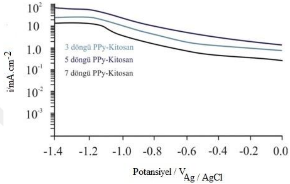
Şekil 4.22: Farklı döngü sayılarında PPy–kitosan kompozit yapılarının 0,5 M \text{H}_2\text{SO}_4 çözeltisinde Tafel polarizasyon eğrileri ( v=1\text{mV} \cdot \text{s}^{-1} ).
