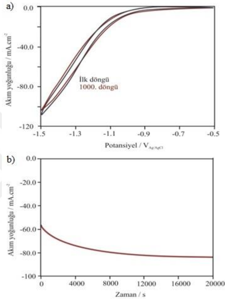
řekil 4.27: Grafit elektrot  zerine kaplanmıř PPy–kitosan/Au kompozit filminin 0,5M H 2 SO 4 elektrolit ortamında kaydedilen a)  lk ve 1000 d ng  sonucundaki d n ř ml  voltamogramları b) -1,0V sabit potansiyelde elde edilen kronoamperomogramı.
