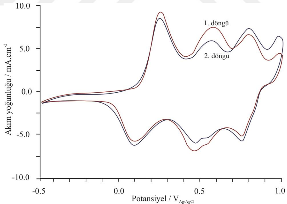
Şekil 3.5: Altın nanopartiküllerinin PANi–kitosan filmi üzerine 0,5 M \text{H}_2\text{SO}_4 içerisinde elektrodpozisyonu ( v=50 \text{ mV.s}^{-1} ).
