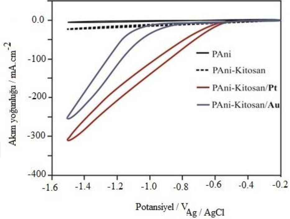
Şekil 4.12: PANi–kitosan/Pt kompozit yapısının 0,5M H 2 SO 4 çözeltisinde kaydedilen dönüşümlü voltamogramları ( v=20\text{mV.s}^{-1} ).
