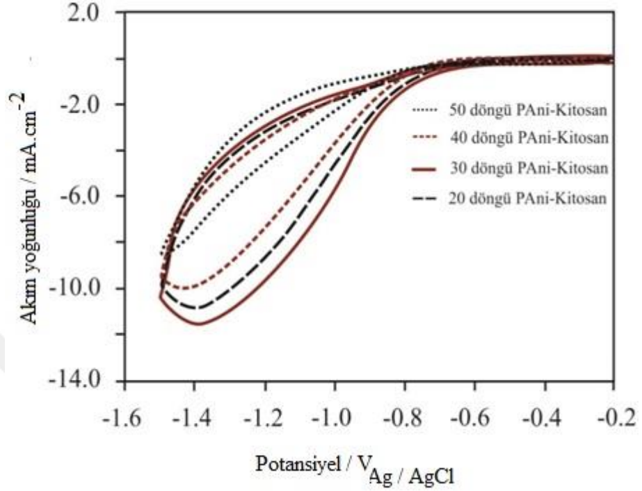
Şekil 4.11: film kalınlıklarında elde edilen PANi–kitosan kompozit yapısının 0,5 M H 2 SO 4 çözeltisinde kaydedilen dönüşümlü voltamogramları (v=20mV.s -1 ).
