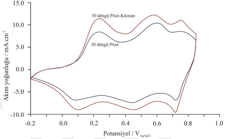
Şekil 3.3: PANi ve PANi–kitosan filmlerinin 0,5 M HCl içerisinde kaydedilen temel diyagramları ( v=50\text{mV.s}^{-1} ).
