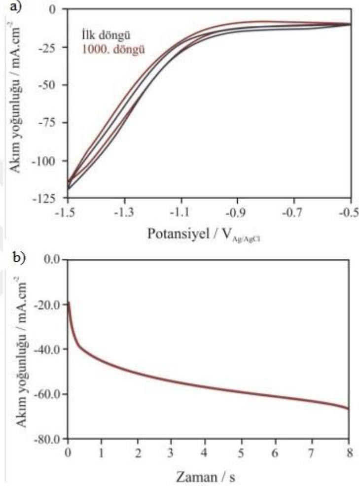
Şekil 4.28: Grafit elektrot üzerine kaplanmış PPy–kitosan/Pt kompozit filminin 0,5 M H 2 SO 4 elektrolit ortamında kaydedilen a) İlk ve 1000 döngü sonucundaki dönüşümlü voltamogramları b) -1,0V sabit potansiyelde elde edilen kronoamperomogramı.
