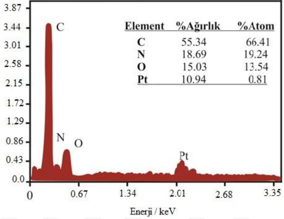
Şekil 4.7: Grafit/PPy–kitosan/Pt yapısının enerji dağılım spektrumu (EDS).
