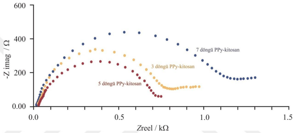
Şekil 4.24: Farklı döngü sayılarında hazırlanan kompozit yapıların 0,5 M H 2 SO 4 elektrolit ortamında 0,1-100000 Hz frekans aralığında -1,0V'ta kaydedilen elektrokimyasal impedans spektrumları.
