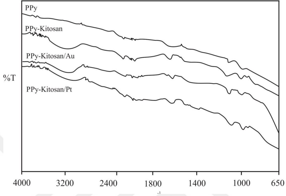
Şekil 4.10: Grafit elektrot yüzeyinde PPy, PPy–kitosan, PPy–kitosan/Au ve PPy–kitosan/Pt yapılarının FT–ATR spektrumları.
