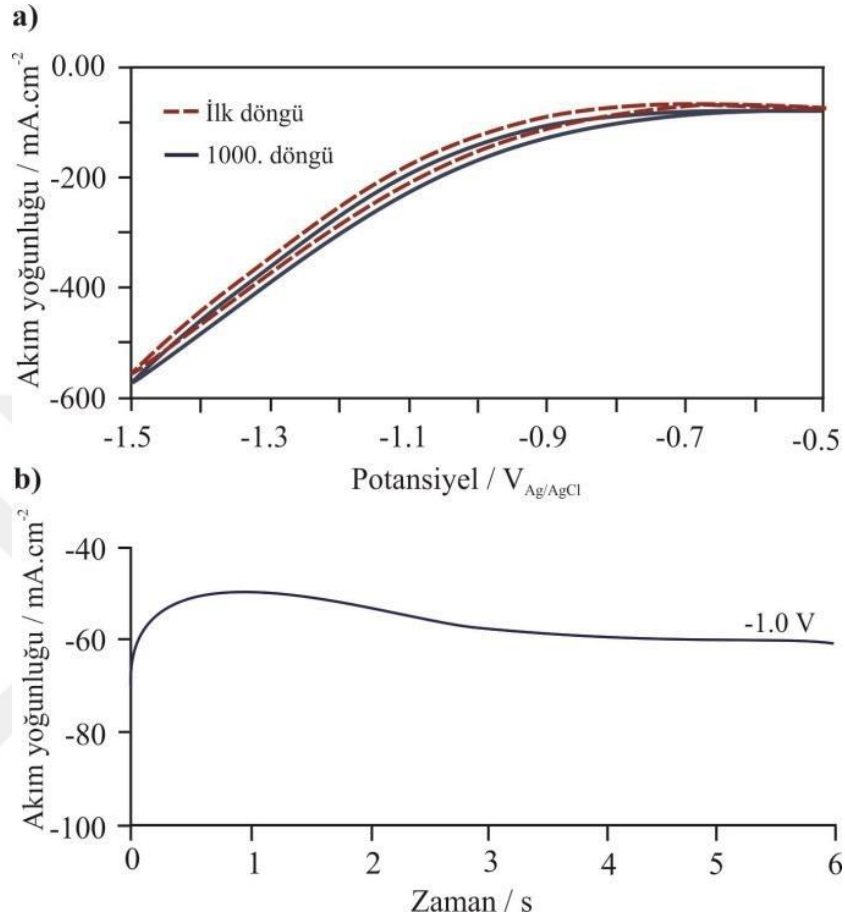
Şekil 4.18: Grafit elektrot üzerine kaplanmış PANi–kitosan/Au kompozit filminin 0,5 M H 2 SO 4 elektrolit ortamında kaydedilen a) İlk ve 1000 döngü sonucundaki dönüşümlü voltamogramları b) -1,0V sabit potansiyelde elde edilen konoamperomogram.
