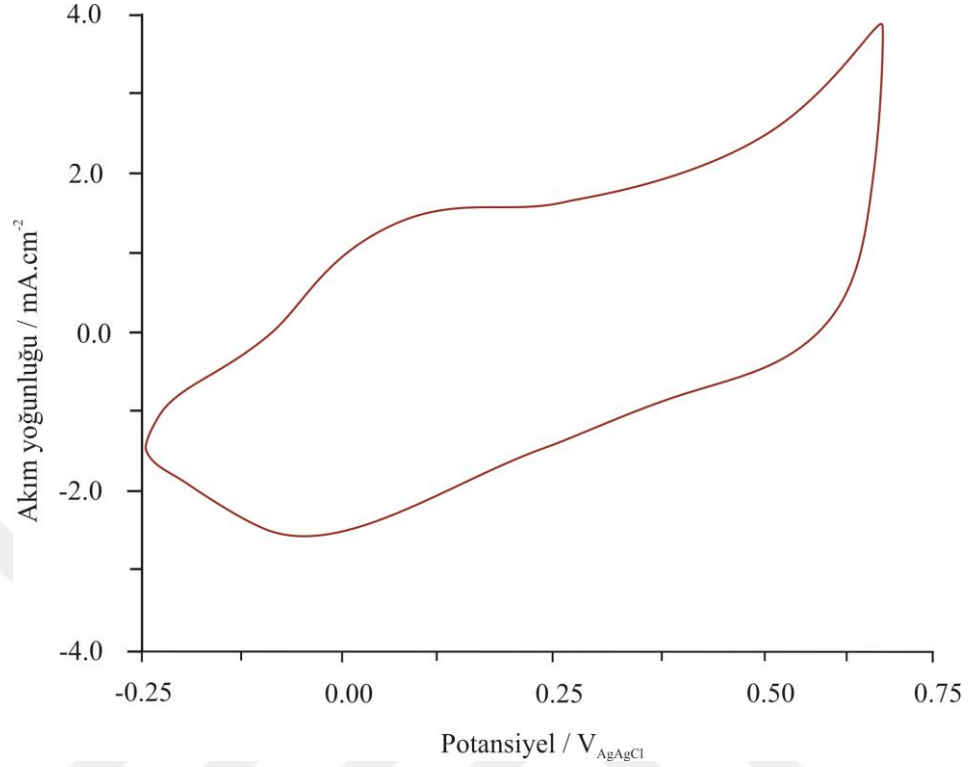
Şekil 3.15: PPy–kitosan/Pt kompozit yapısına ait 0,5 M H 2 SO 4 içerisinde kaydedilen temel diyagram (v=50mV.s -1 ).
