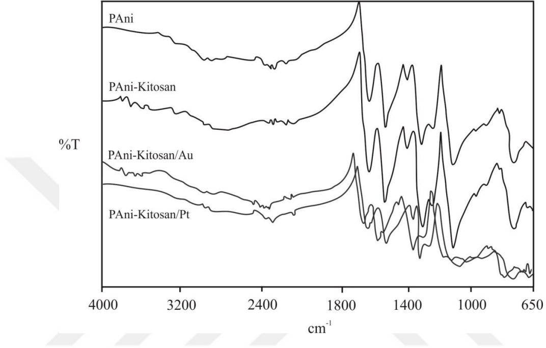
Şekil 4.5: PAni, PAni–kitosan, PAni–kitosan/Au ve PAni–kitosan/Pt yapılarının FT–ATR spektrumları.
