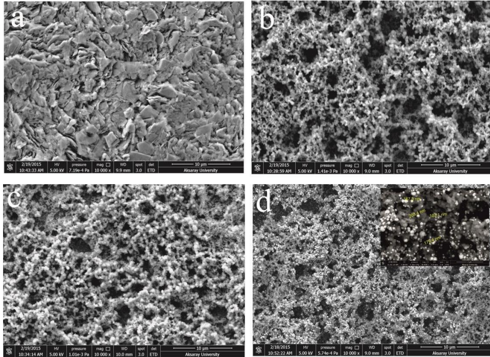
Şekil 4.1: a) Çıplak grafit b) Grafit/PAni c) Grafit/PAni–kitosan d) Grafit/PAni–kitosan/Pt yapılarının taramalı elektron mikroskobu (SEM) görüntüleri.
