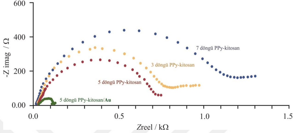
Şekil 4.25: Farklı döngü sayılarında hazırlanan kompozit yapıların ve 5 döngülük PPy–kitosan kompozit yapı üzerine Au nanopartiküllerinin elektrodpozisyonuyla elde edilen kompozit yapının 0,5 M H 2 SO 4 elektrolit ortamında 0,1–100000 Hz frekans aralığında -1,0V'ta kaydedilen Nyquist diyagramları.
