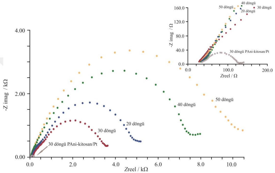
Şekil 4.17: Farklı film kalınlıklarında elde edilen PANi–kitosan kompozit yapıların ve 30 döngülük PANi–kitosan kompozit yapı üzerine Pt nanopartiküllerinin elektrodepozisyonu ile elde edilen kompozit yapının 0,5 M H 2 SO 4 çözeltisinde kaydedilen Nyquist diyagramları (inset diyagram).
