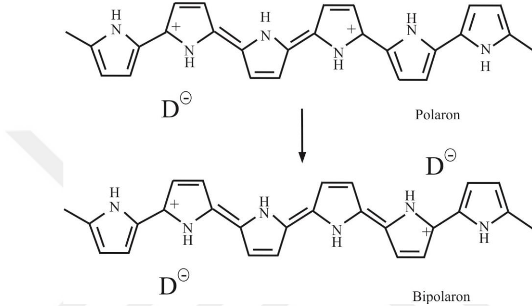
Şekil 2.6: Polipirolün kararlı rezonans formülleri.
