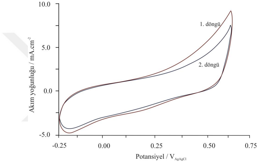
Şekil 3.14: PPy–kitosan filmi üzerine Pt nanopartiküllerinin 0,5 M H_2SO_4 içerisinde elektrodpozisyonu ( v=50 \text{ mV.s}^{-1} ).
