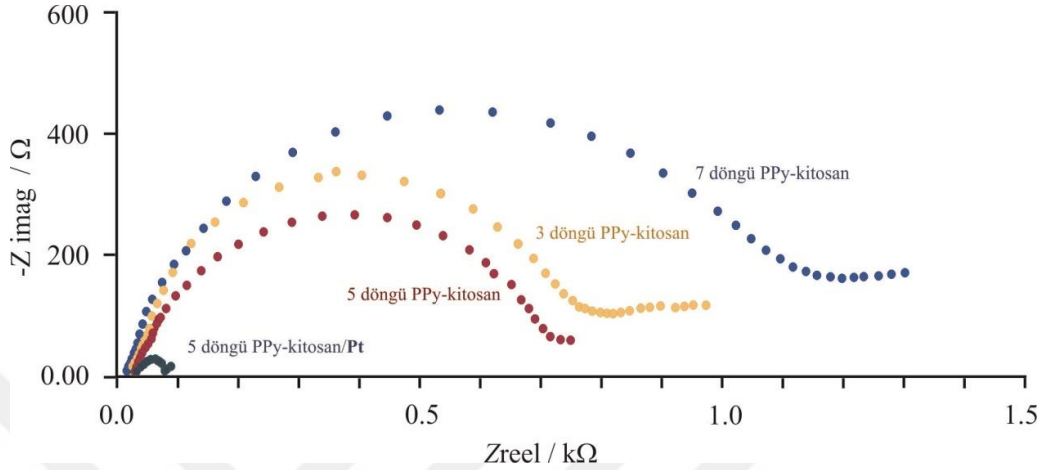
Şekil 4.26: Farklı döngü sayılarında hazırlanan kompozit yapıların ve 5 döngülük PPY–kitosan kompozit yapı üzerine Pt nanopartiküllerinin elektrodpozisyonuyla elde edilen kompozit yapının 0,5 M H 2 SO 4 elektrolit ortamında 0,1 – 100000 Hz frekans aralığında -1,0V'ta kaydedilen Nyquist diyagramları.
