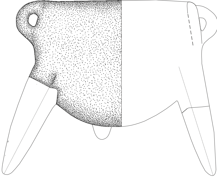
Çizim 89: B1a Tipi, Poliochne İTÇ IIIa Kaynak: Brea 1976: Tav. CCXIX.c
