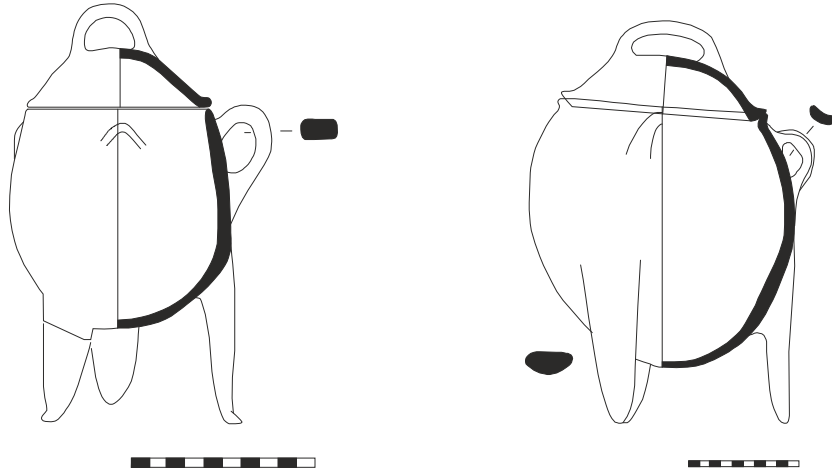
Çizim 13-14: Üç Ayaklı Mutfak Kabı ve Kapak, Küllioba
