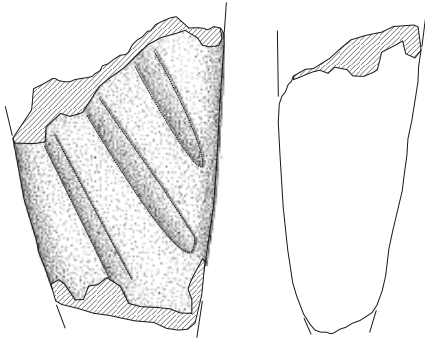
Çizim 198: B Tipi, Kanlıtaş İTÇ III
