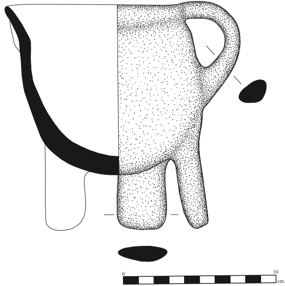
Çizim 27: A2 Tipi, Menye Köyü İTÇII Kaynak: Bostancı vd. 2006: 233: Lev. V. 5
