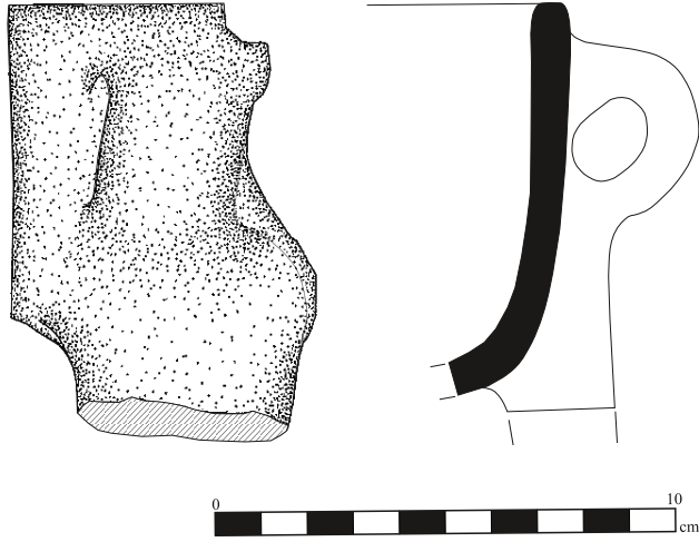
Çizim 60: B1 Tipi, Troya İTÇ IIIa Kaynak: Blegen vd. 1950:fig. 412.39
