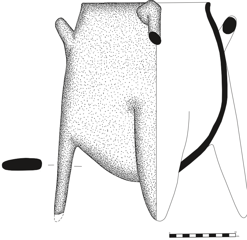
Çizim 114: C2 Tipi, Küllioba İTÇ IIIa Kaynak: Türkteki 2004: 66: Lev.7/1
