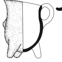
Çizim 21: A1 Tipi, Beycesultan İTÇ II Kaynak: Lloyd ve Mellaart 1962: 179: fig. 39/10
