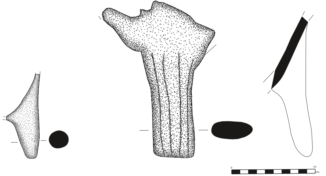
Çizim 144: A Tipi, Karataş-Semayük İTÇ II Kaynak: Eslick 2009: 207: KT464
