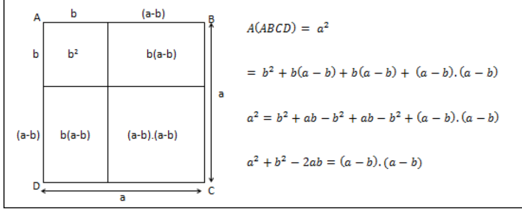
Şekil 3. (a-b).(a-b) ifadesi
