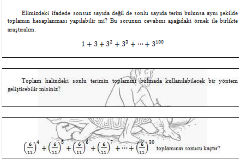
Şekil 10. Sonlu toplamlar
