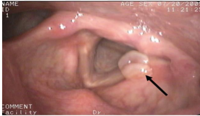
Şekil 7: Kontak Ülseri/Granülomu (49).
