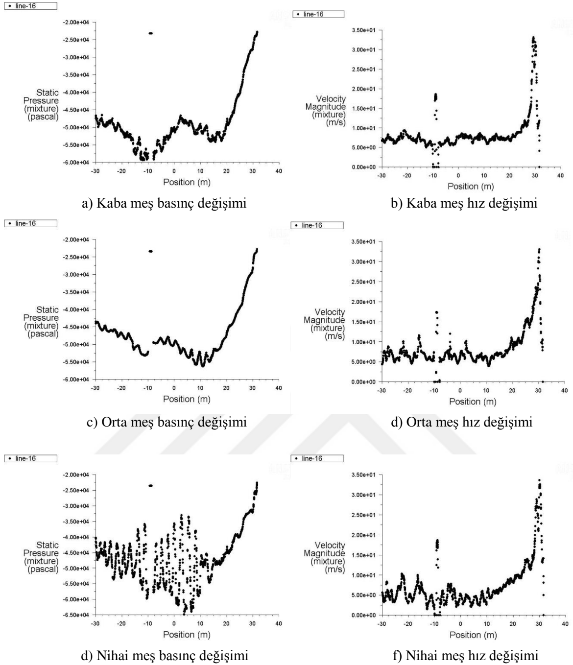
Şekil 4.12. Ilısu Barajı 1982 tasarımı dolusavak havalandırıcısı kaba-orta-ince (nihai) meş yapılarında H=2 m ve V=20 m/s durumu için ana hava kanalı boyunca basınç ile hava hızı değişimleri
