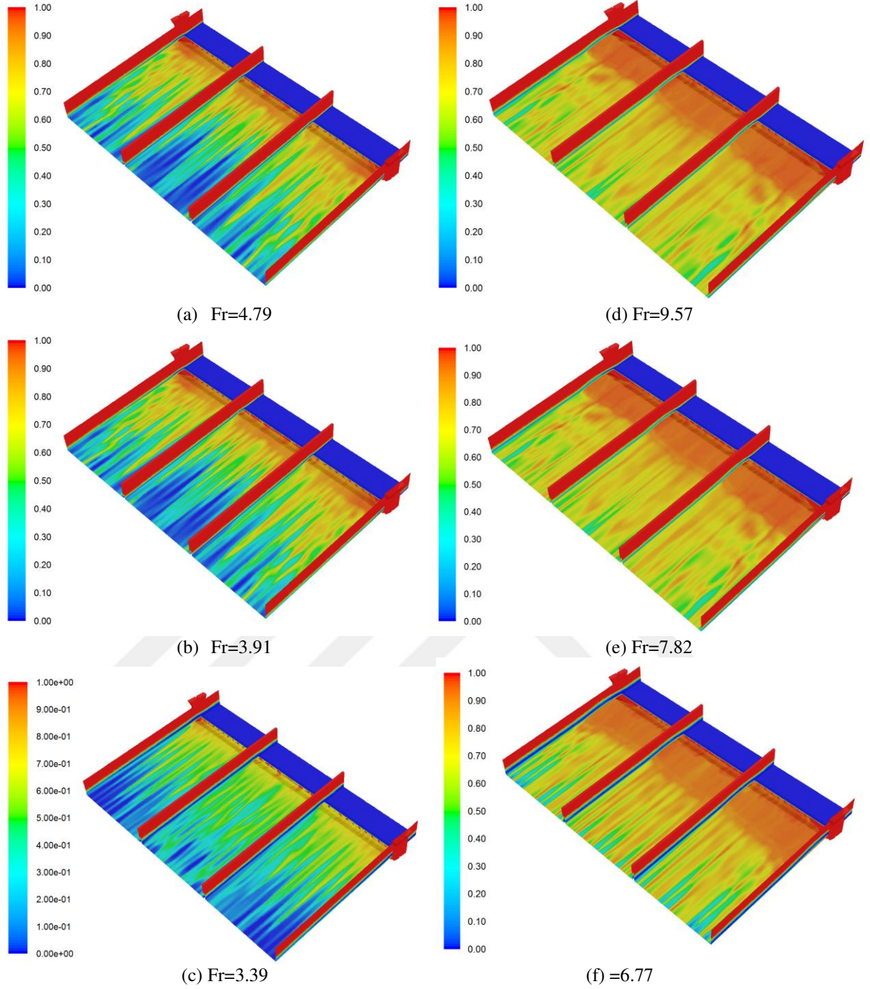
Şekil 4.16. Ilısu Barajı 2010 tasarım tabandaki hava-su faz oranları: (a) h=1.0\text{m} , v=15\text{m/s} , Fr=4.79 , (b) h=1.5\text{m} , v=15\text{m/s} , Fr=3.91 , (c) h=2.0\text{m} , v=15\text{m/s} , Fr=3.39 , (d) h=1.0\text{m} , v=30\text{m/s} , Fr=9.57 , (e) h=1.5\text{m} , v=30\text{m/s} , Fr=7.82 , (f) h=2.0\text{m} , v=30\text{m/s} , Fr=6.77
