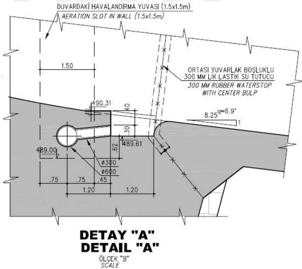
Şekil 3.5. Ilısu Barajı eşik yapısındaki nihai durumda havalandırıcı detayları (DSİ, 2010)
