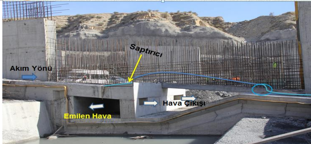
Şekil 3.7. Dolusavak şüt kanalı havalandırıcısı inşaatından görüntüler
