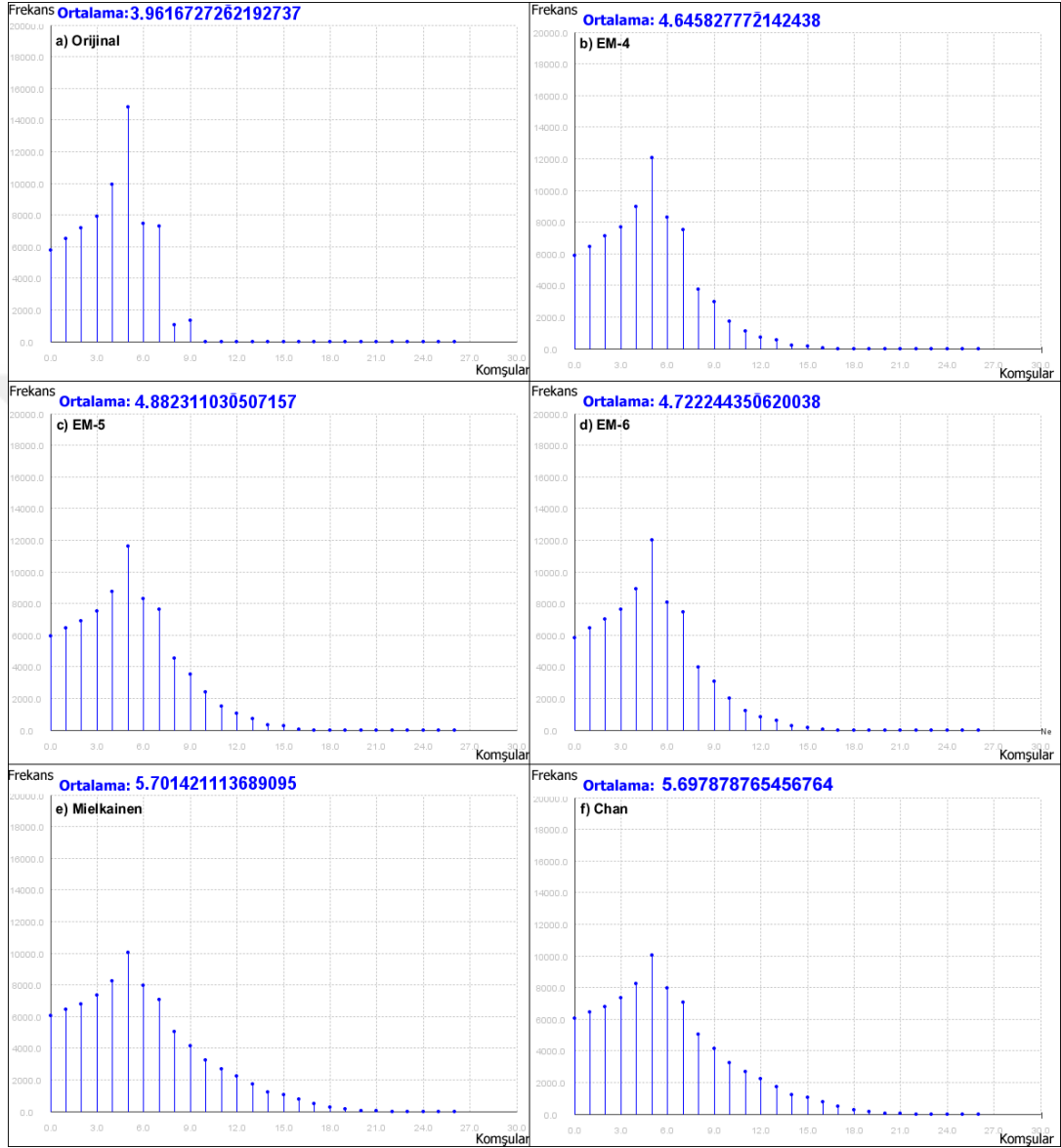
Şekil 4.6. 640x480 Lena imgesine önerilen yöntemler ve literatür çalışmalarıyla 1bpp veri gizlemeleriyle oluşan sırlı imgelerin komşuluk (neighbourhood) histogramı sıraçma sonuçları a) Orjinal imge b) EM-4 ile veri gizlenmiş sırlı imge c) EM-5 d) EM-6 e) Mielkainen
