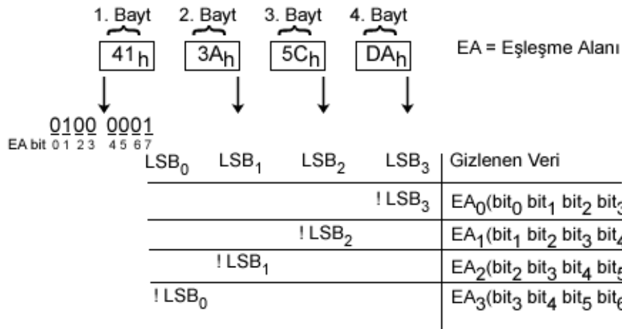
Şekil 3.1. EM-1 yönteminde eşleştirme alanlarının oluşturulması
