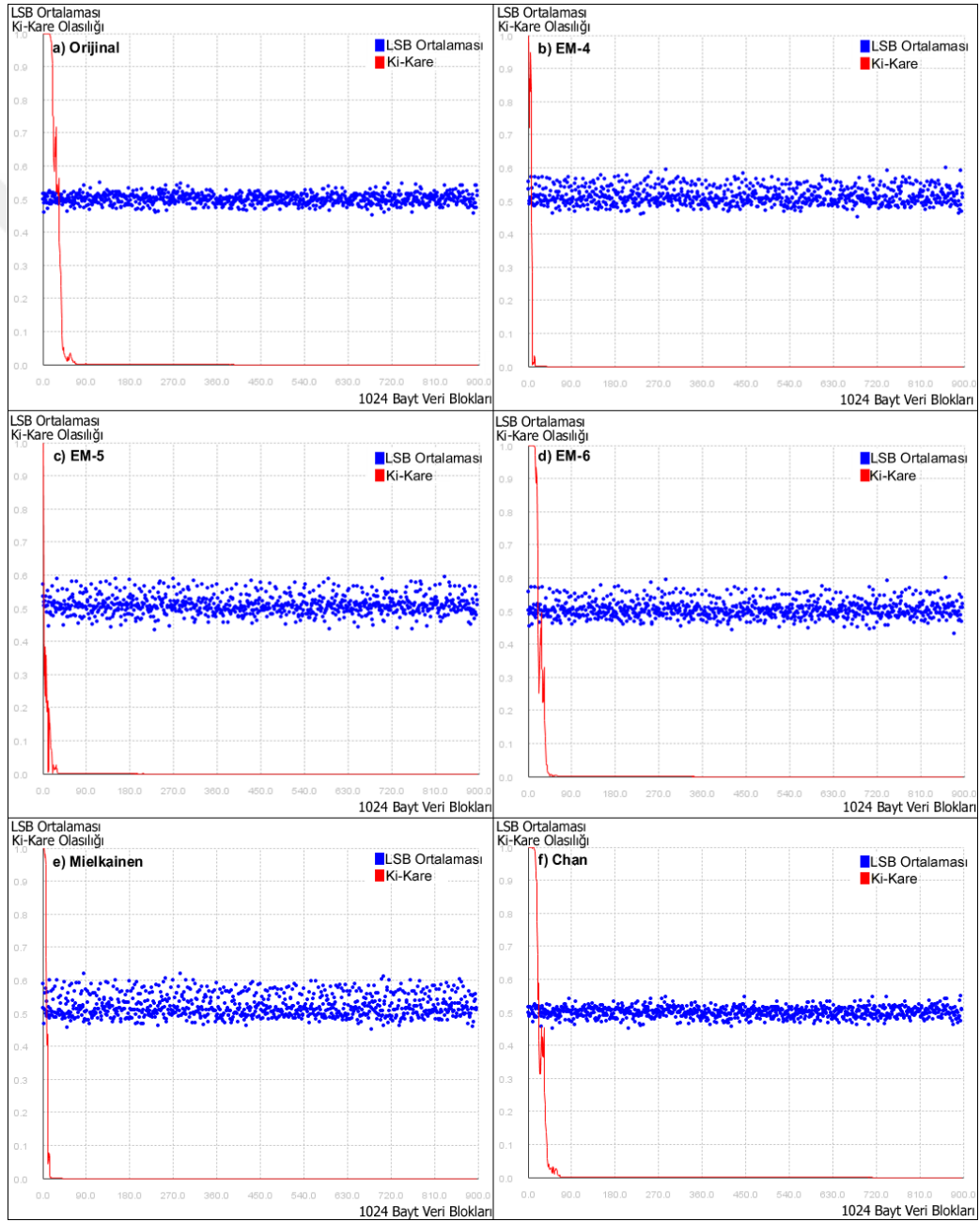
Şekil 4.8. 640x480 Lena imgesine önerilen yöntemler ve literatür çalışmalarıyla 1bpp veri gizlemeleriyle oluşan sırlı imgelerin ki-kare sırama sonuçları a) orijinal imgenin ki-kare sonucu b) EM-4 ile veri gizlenmiş sırlı imgenin ki-kare sonucu c) EM-5 d) EM-6 e) Mielkainen [2] f) Chan [3]
