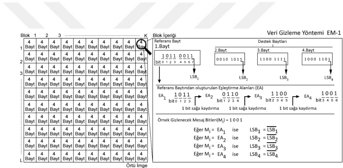
Şekil 3.2. EM-1 yönteminin çalışma prensibi
