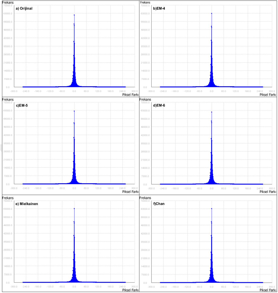
Şekil 4.7. 640x480 Lena imgesine önerilen yöntemler ve literatür çalışmalarıyla 1bpp veri gizlemeleriyle oluşan sırlı imgelerin piksel farkı histogram sıracma sonuçları a) Orjinal image b) EM-4 ile veri gizlenmiş sırlı image c) EM-5 d) EM-6 e) Mielkainen [2] f) Chan[3]
