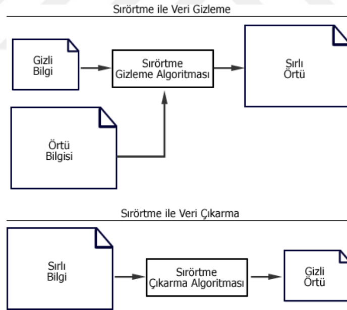
Şekil 2.1. Sırtörtme ile veri gizleme ve veri çıkarma işleminin genel diyagramı
