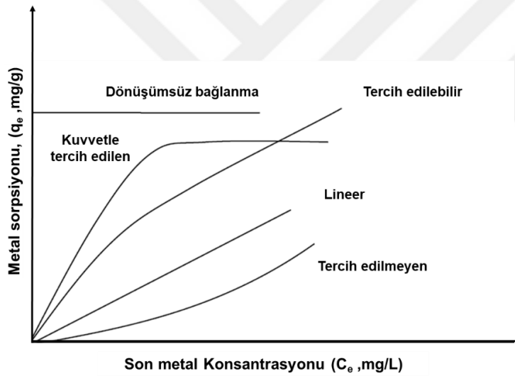
Şekil 2.8. Adsorpsiyon izotermi [1]
