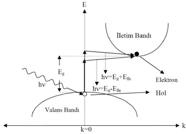
Şekil 6.3. Bir yarıiletkeninde indirekt bant geçişi.
