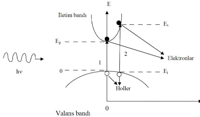
Şekil 6.2. Bir yarıiletkende direk bant geçişi.
