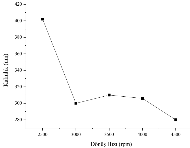
Şekil 3.8. Deney 1 için ölçülen kalınlıklar
