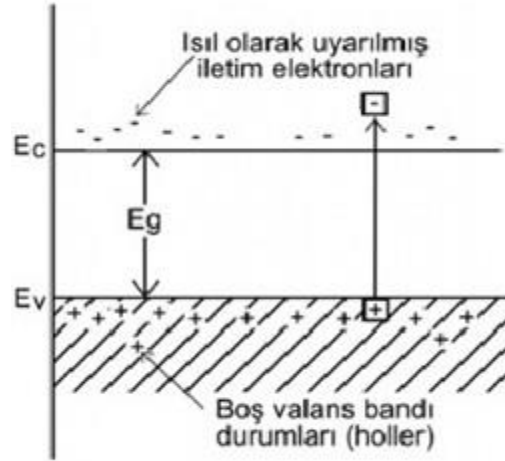
Şekil 2.3. Oda sıcaklığında iletim ve valans bantları; ısı uyarma sonucu oluşan elektron-hol çifti [36].
