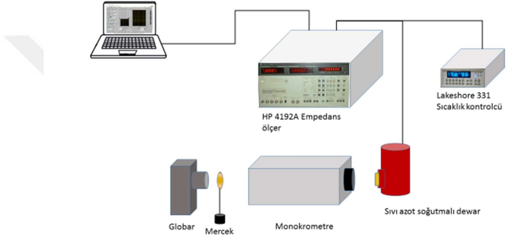
Şekil 3.8. Örneklerin fotokapasitans ölçümü için kullanılan düzeneğin şematik olarak gösterimi.
