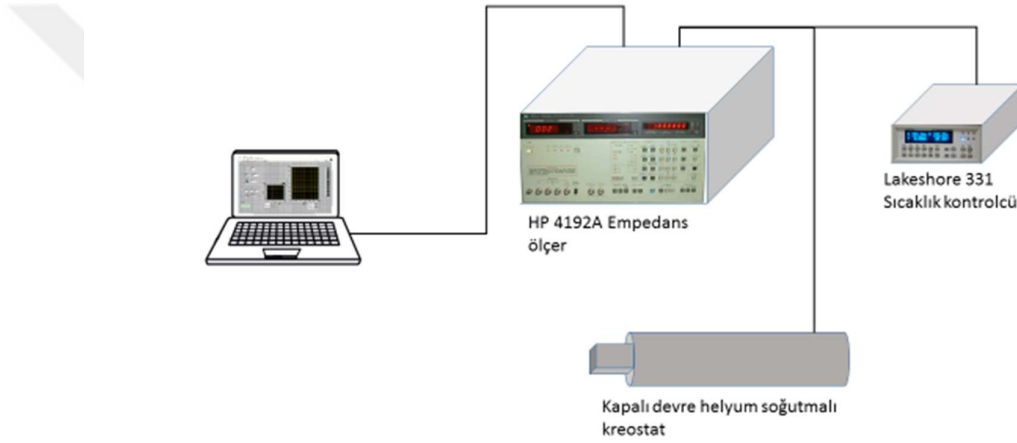
Şekil 3.7. Empedans ölçer, sıcaklık kontrolcüsü ve kreyostattan oluşan kapasitans-voltaj ölçüm düzeneği.
