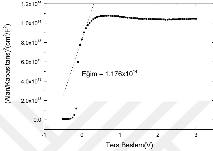
Şekil 4.5. (Alan/kapasitans)'ın karesi, ters beslem grafiği.
