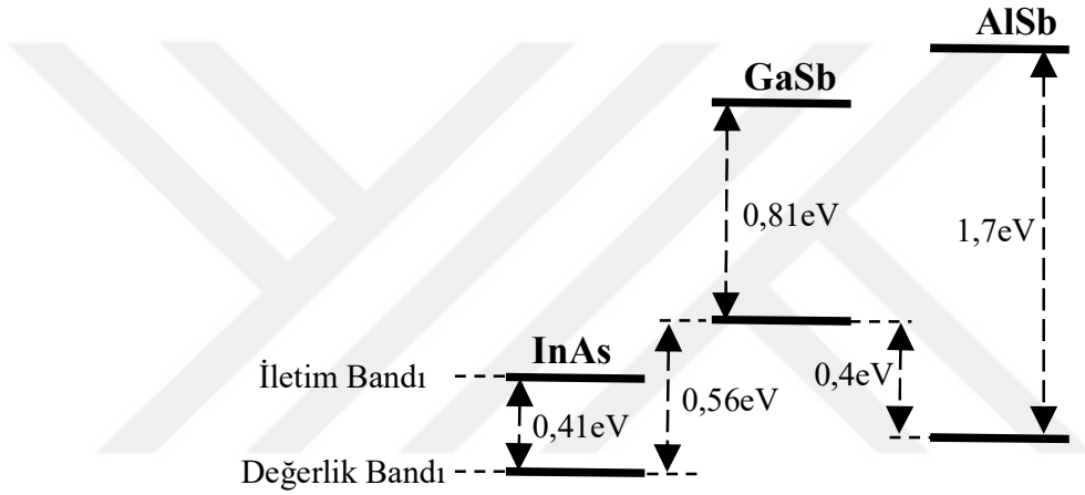
Şekil 2.2. InAs, GaSb ve AlSb'nin yasak bant aralıkları ve birbirlerine göre hizalanması.
