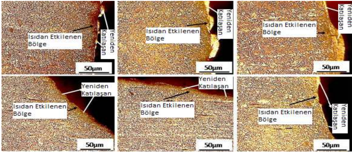
Resim 2.6. Farklı parametreler ile işlenmiş parçada meydana gelen yüzey kusurları [13]
