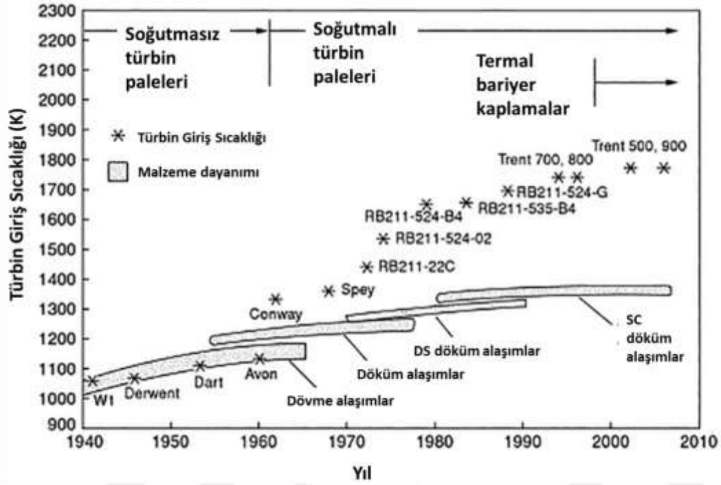
Şekil 1.1. Türbin giriş sıcaklığı ve malzemelerin gelişimi [2]
