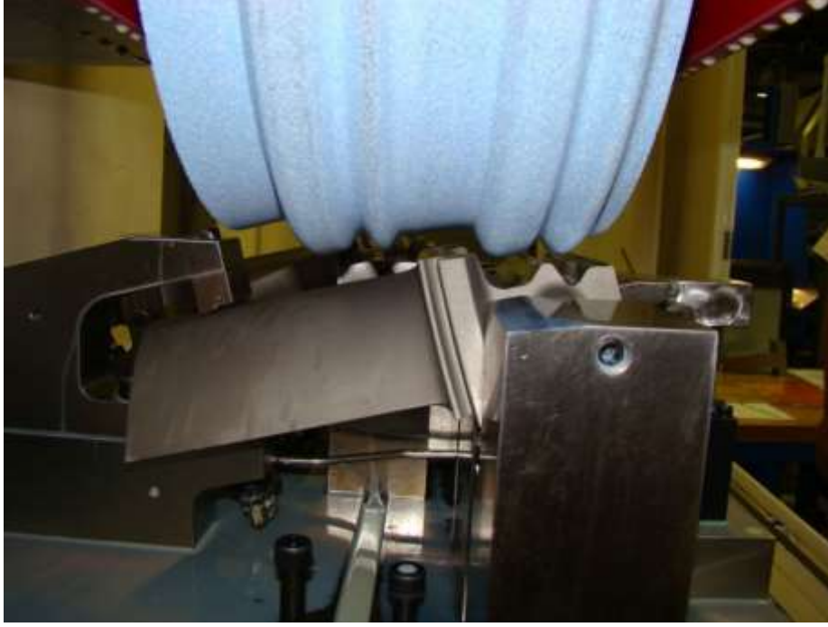
Resim 2.14. Türbin kökünün sürünme ilerlemeli taşlama prosesi ile işlenmesi [29]
