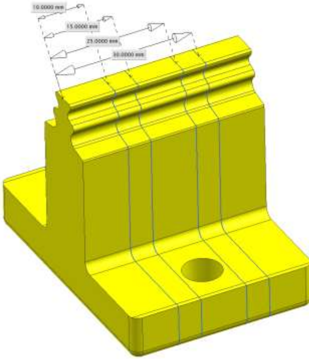
Resim 3.17. Numunelerin yeniden katılaşılan bölge ve HAZ ölçümleri için tel erozyon tezgahı ile parçalara bölünmesi için ölçüler
