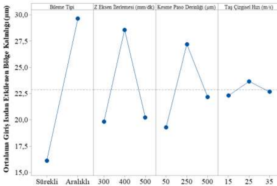
Şekil 4.6. Deney seti 1 giriş HAZ kalınlığı ölçümleri
