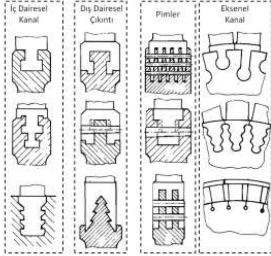
Resim 2.2. Türbin palesi kök bağlantı tipleri [5]
