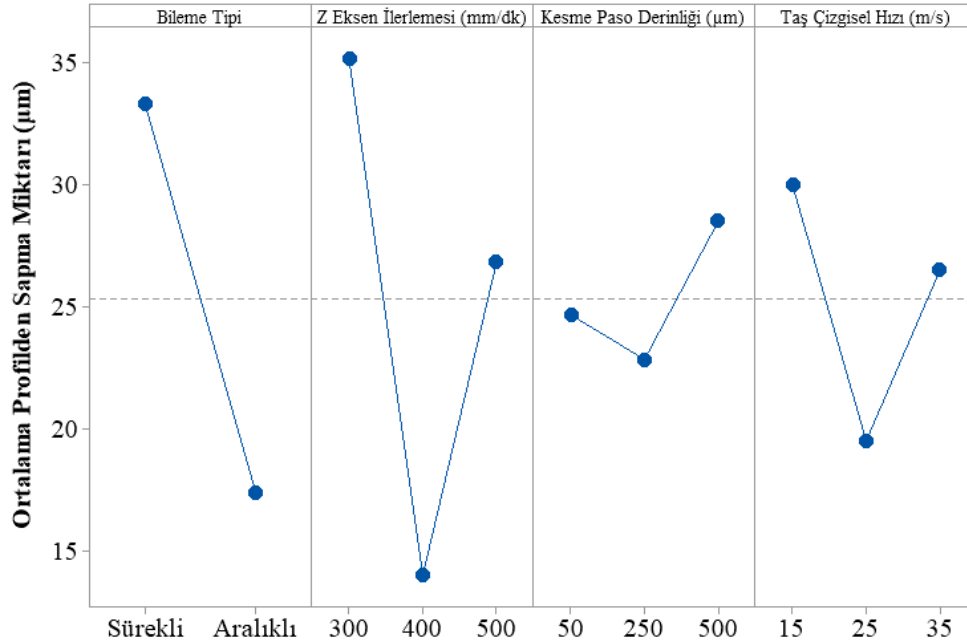
Şekil 4.1. Deney seti 1 profilden sapma miktarları
