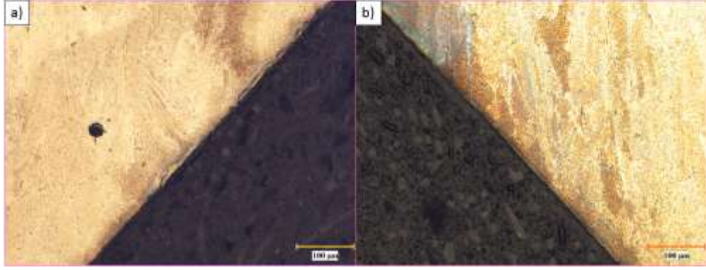
Resim 4.17. Örnek devamlı yeniden katılaşan bölge ve HAZ
