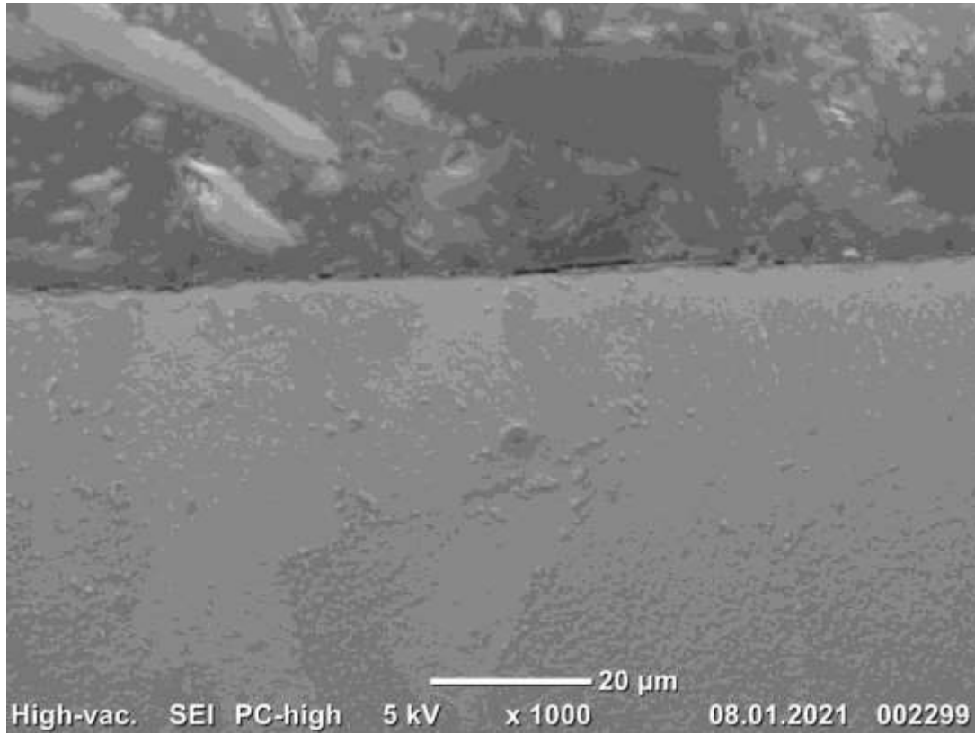
Resim 4.14. Yeniden katılaşan ve ısıdan etkilenen bölge için SEM görüntüsü
