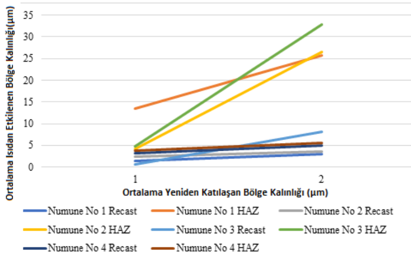
Şekil 4.8. Deney seti 1 ilk 4 numune giriş ve çıkış bölgeleri yeniden katılaştan bölge ve HAZ kalınlıkları
