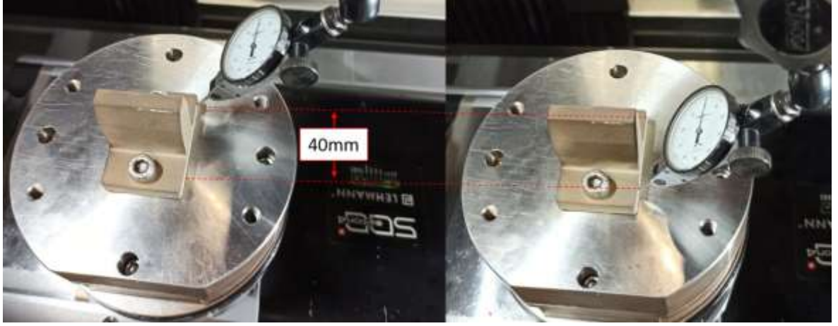
Resim 3.9. İndikatör yardımı ile açısız dönüklüğün giderilmesi
