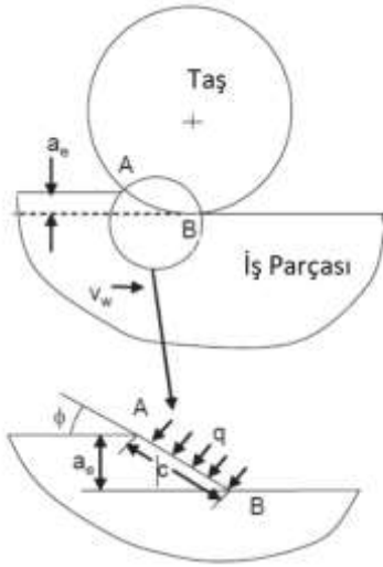
Resim 2.15. Taşlama sistemlerinde parça ve taş arasındaki açı [26]
