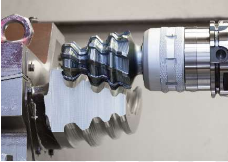
Resim 2.10. Örnek Fir-Tree freze takımı ve operasyonu [24]
