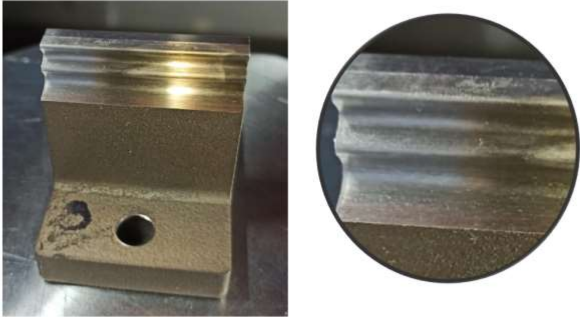
Resim 4.1. Deney seti 1 - 9 numaralı parametre yanık izi
