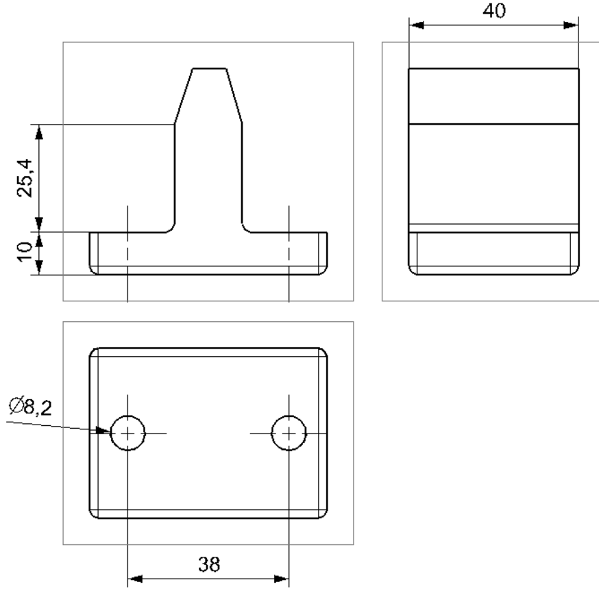
Resim 3.3. Numunelerin ölçüleri
