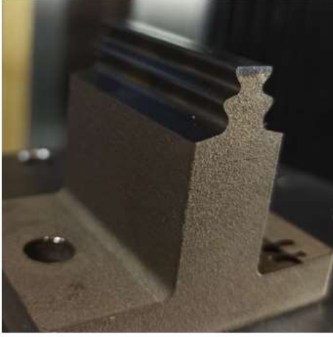
Resim 4.3. Parametre seti 12 numune görseli
