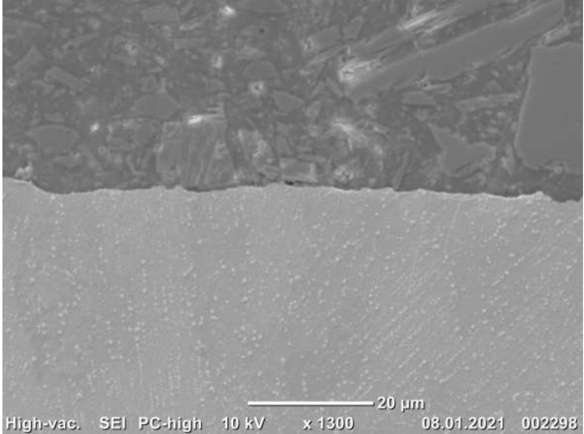
Resim 4.13. Yeniden katılaşan bölge için SEM görüntüsü
