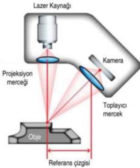
Resim 2.21. Lazer ile ölçüm sisteminin çalışma sistemi [35]
