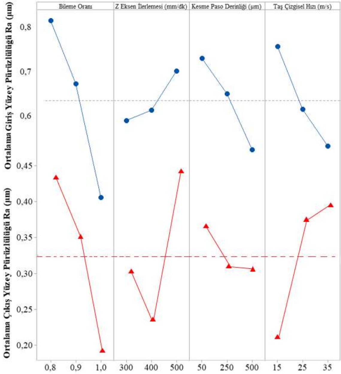
Şekil 4.4. Deney seti 2 giriş ve çıkış yüzey pürüzlülüğü
