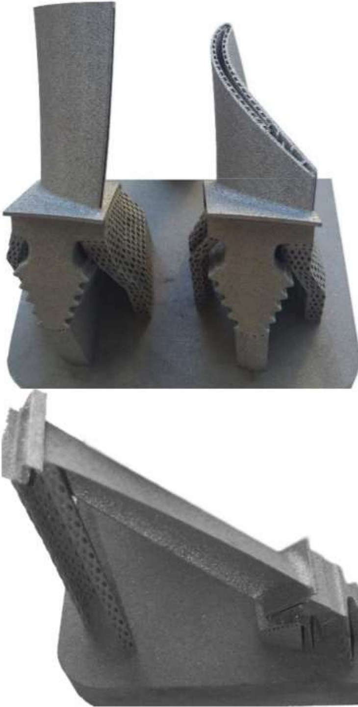
Resim 2.23. Katmanlı imalat ile üretilmiş türbin paleleri [42]
