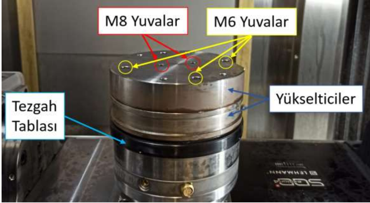
Resim 3.2. Denemelerde kullanılan fikstür
