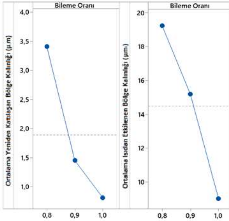
Şekil 4.9. Deney seti 2 bileme oranlarının yeniden katılaştıran bölge ve HAZ kalınlıklarına etkileri
