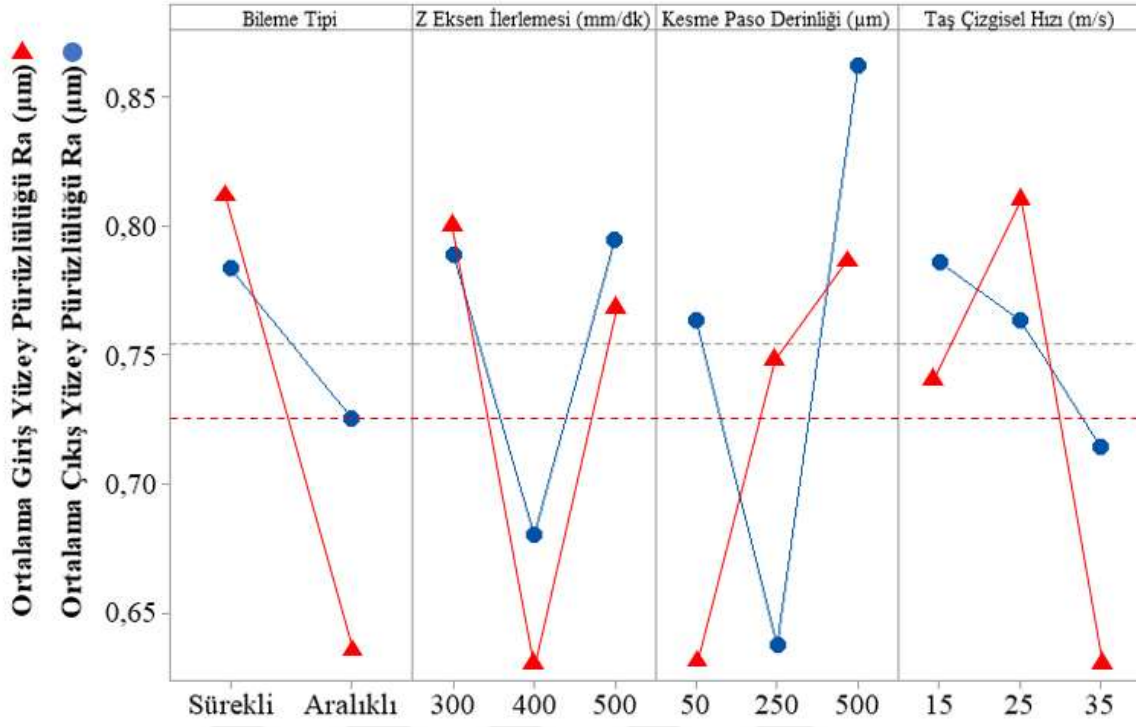
Şekil 4.2. Deney seti 1 giriş ve çıkış bölgesi yüzey pürüzlülüğü
