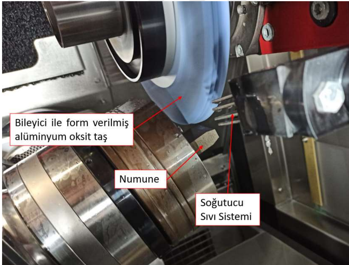
Resim 3.8. Parça işlemesi için tezgah görseli
