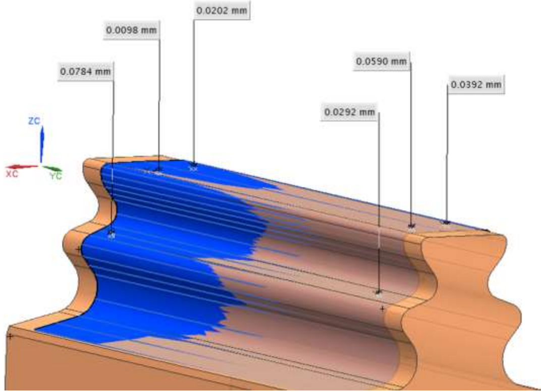
Resim 4.9. CMM ölçümlerinin normalleştirilmesi
