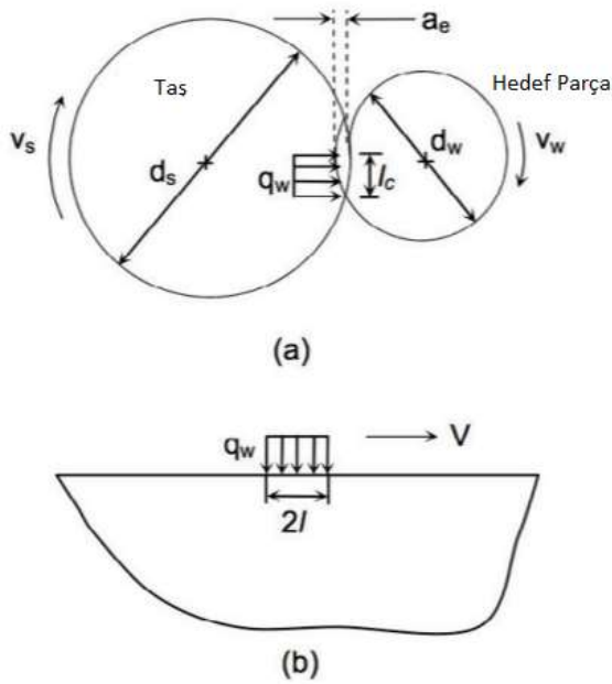
Resim 4.10. Konvansiyonel taşlama benzetmesi
