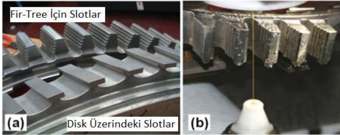
Resim 2.5. a) Tel erozyon tezgahı ile açılmış örnek kök slotları b) Tel erozyon tezgahı metodu ile açılmakta olan disk slotu [12]
