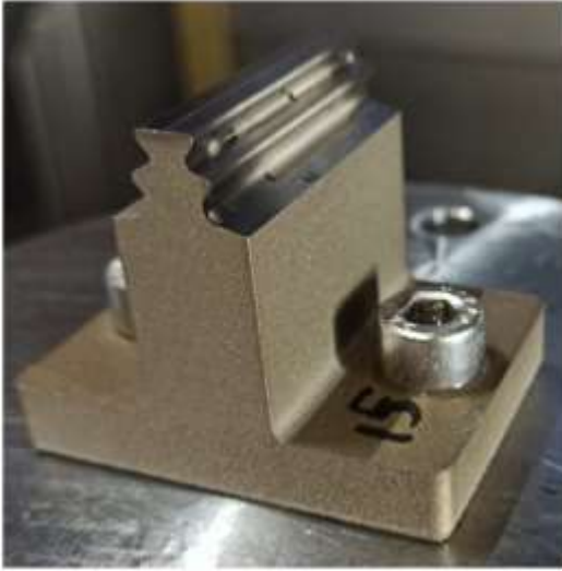
Resim 4.6. Parametre seti 15 numune görseli
