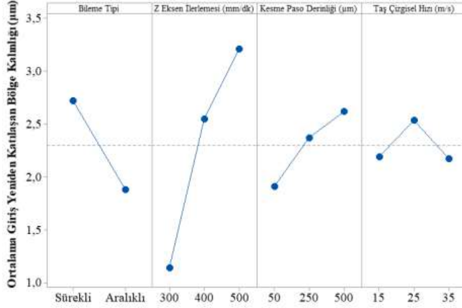
Şekil 4.5. Deney seti 1 giriş yeniden katılaştıran bölge kalınlığı ölçümleri
