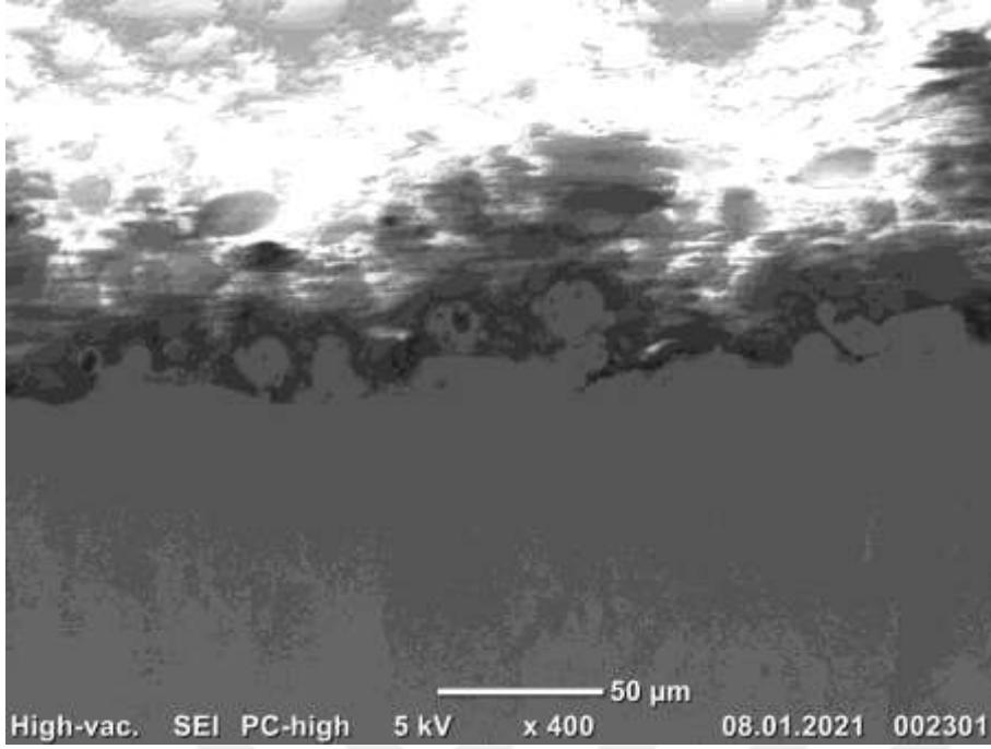
Resim 4.15. Yeniden katılaşan bölgenin parlatma sonrası sıvanma biçiminde gözlemlenmesi
