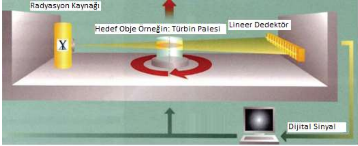
Resim 2.17. Tomografi cihazı çalışma mantığı [36]
