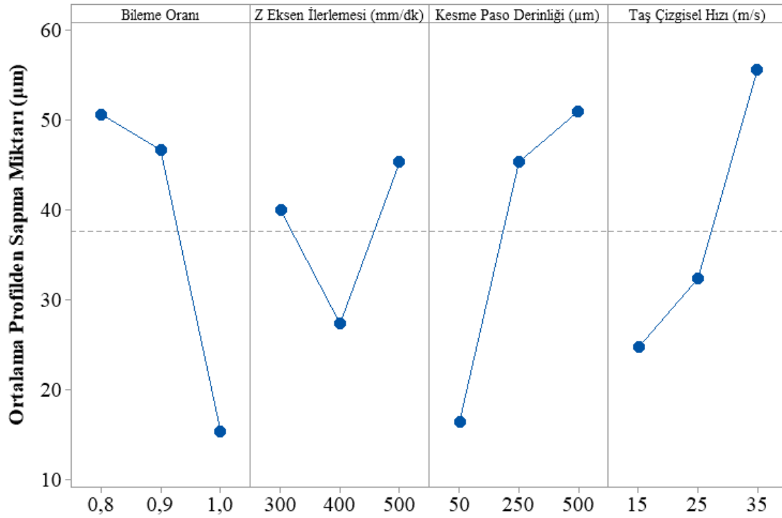
Şekil 4.3. Deney seti 2 profilden sapma
