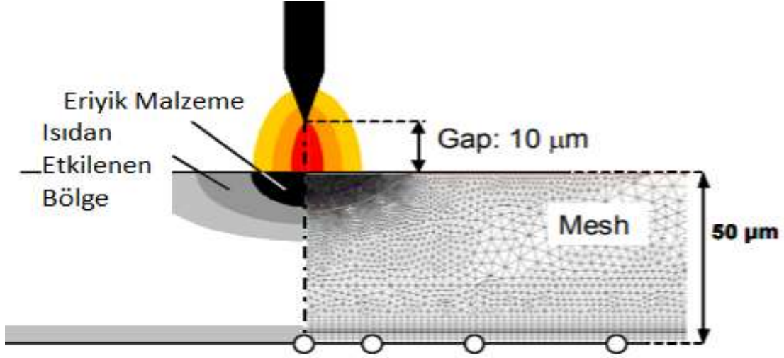
Resim 2.7. Erozyon sistemlerinde sıcaklığın etkisinin şematik görüntüsü [18]
