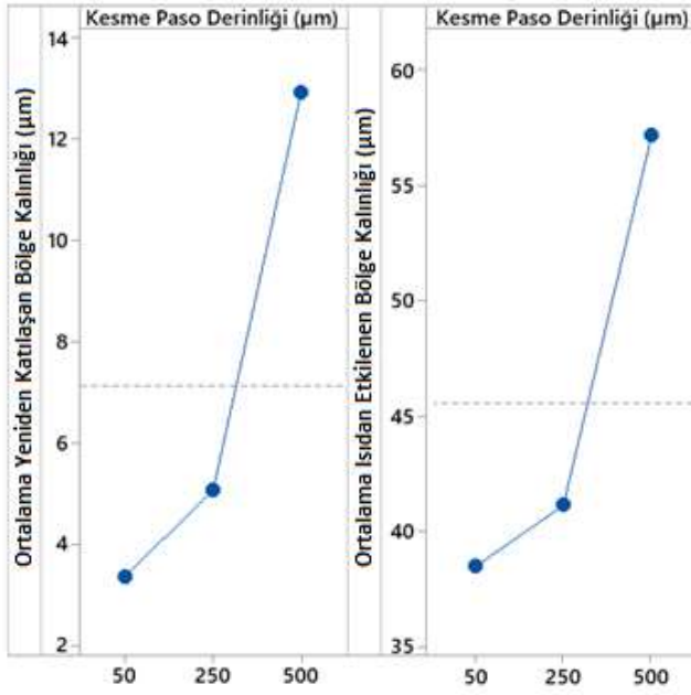
Şekil 4.7. Deney seti 1 çıkış yeniden katılaştıran bölge ve HAZ kalınlığı ölçümlerine paso miktarının etkisi
