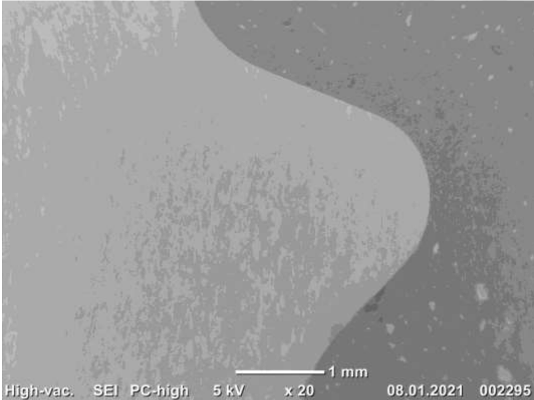
Resim 4.12. Taşlama yapılmış numuneler için SEM görüntüsü
