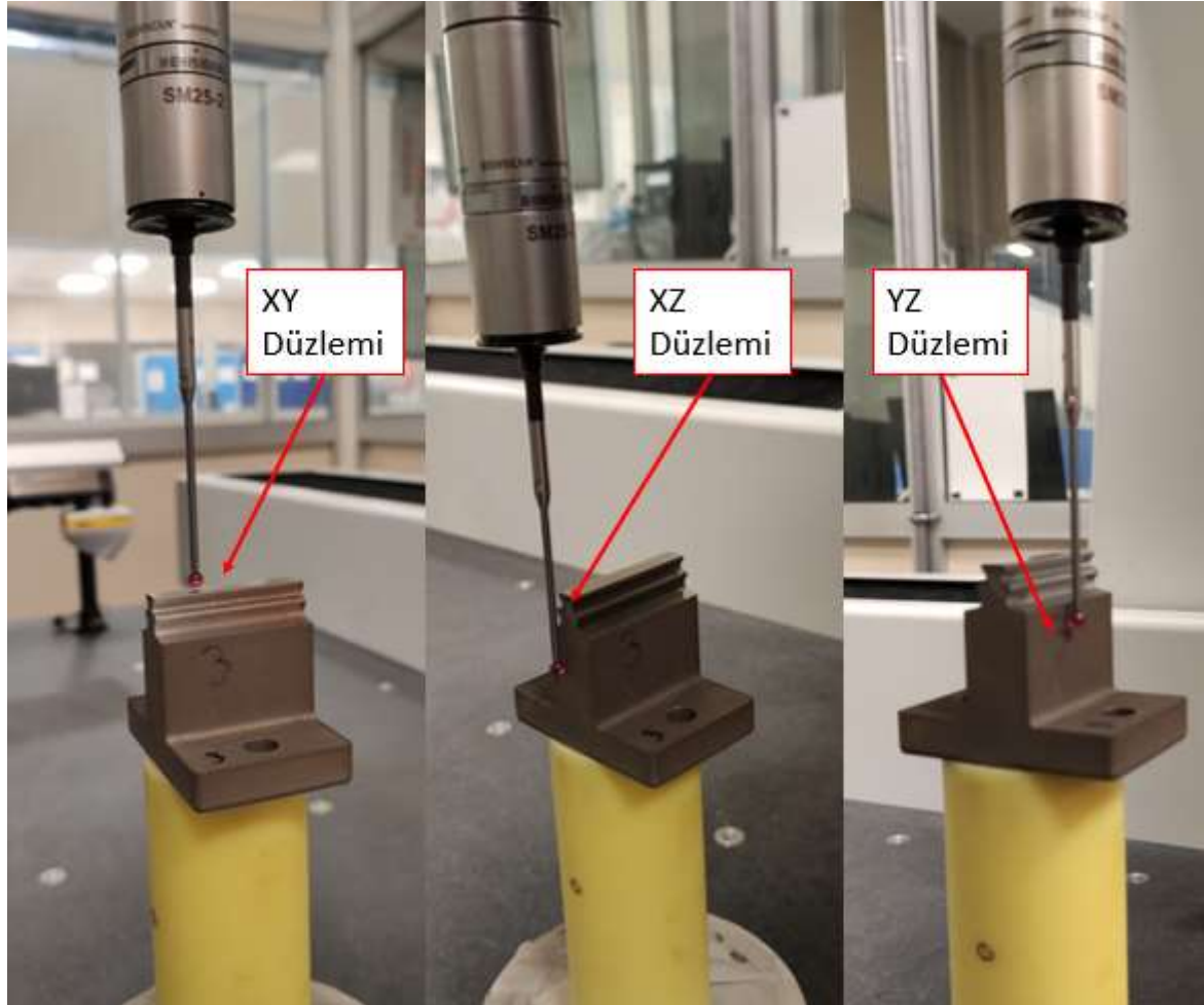
Resim 3.12. Numuneler için CMM ölçümü
