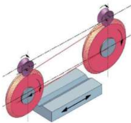
Resim 2.11. Sürekli bilemeli sürünme ilerlemeli taşlama prosesi [28]
