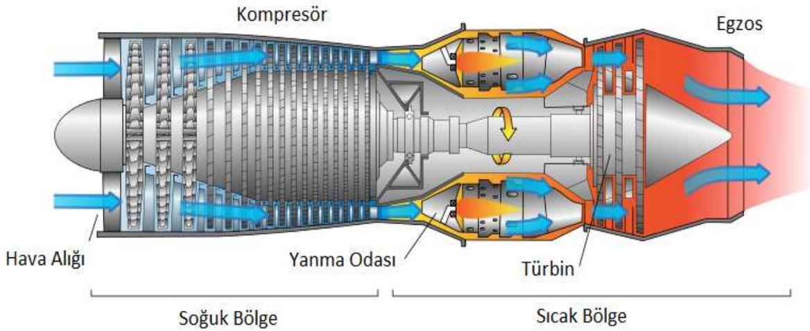
Resim 1.1. Gaz türbin bölgeleri [1]
