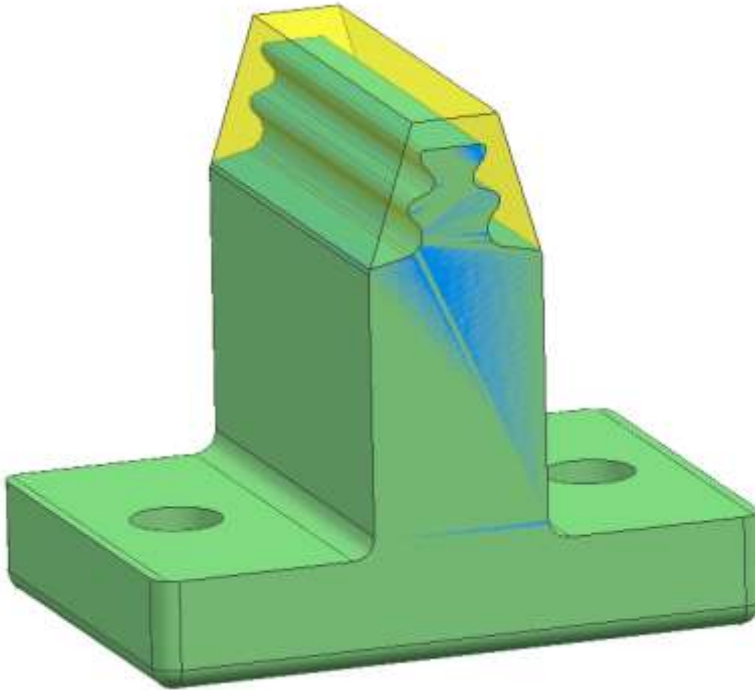
Resim 3.4. Üretilen numune ve hedef parça
