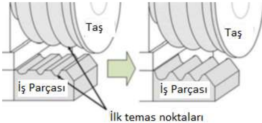
Resim 2.16. Taş ve Fir-Tree profilini ilk teması [30]
