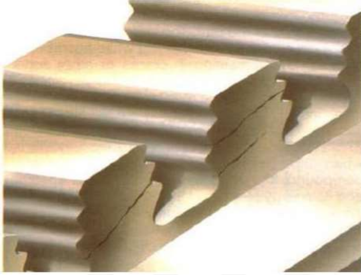
Resim 2.4. Yorulma kaynaklı disk üzerindeki kök geometrisindeki çatlaklar [8]
