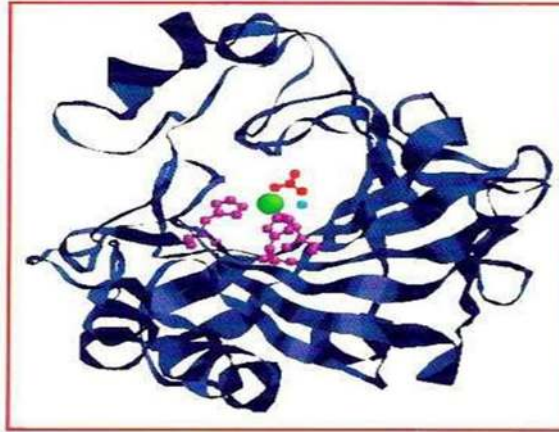
Şekil 2.2. CA-II'in polipeptit yapısı
