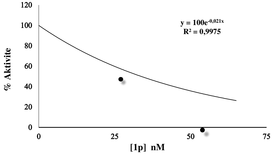
Şekil 4.5. 1 p bileşiğinin hCA- II için çizilen IC 50 grafiği
