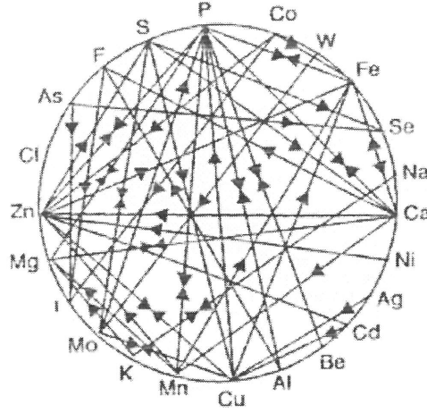
Şekil 1.11. Sindirim kanalı ve metabolizmada mineraller arasındaki potansiyel etkileşimler (Vieira 2008)
