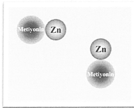
Şekil 1.6. Metal-spesifik amino asit kompleksi (Anonim 2004)
