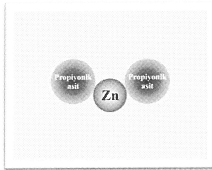
Şekil 1.10. Metal-propiyonik asit (Anonim 2004)
