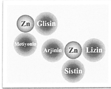
Şekil 1.8. Metal-amino asit şelatı (Anonim 2004)
