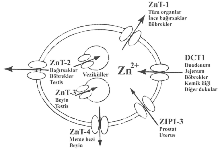
Şekil 1.2. Çinko taşıyıcı ZnT 1-4 ailesinin öngörülen konumları ve doku özgünlükleri. Her bir taşıyıcı, çinko iyonlarını sitosoldan veziküllere veya hücre dışı alana uzaklaştırmak için vektörel olarak konumlanmıştır. ZIP ve DCT1 çinkonun hücre içi taşıyıcıları olarak gösterilmiştir (McMahon ve Cousins 1998).
