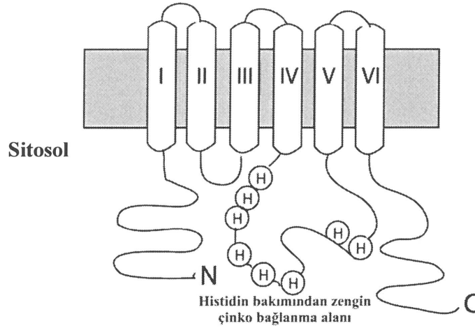
Şekil 1.1. ZnT çinko taşıyıcısının temel yapısı.
