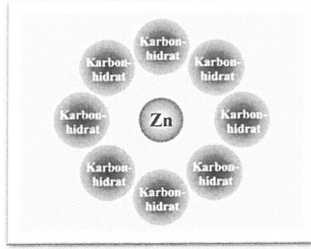
Şekil 1.9. Metal-polisakkarit kompleksi (Anonim 2004)
