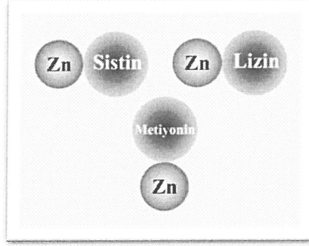
Şekil 1.5. Metal-amino asit kompleksi (Anonim 2004)
