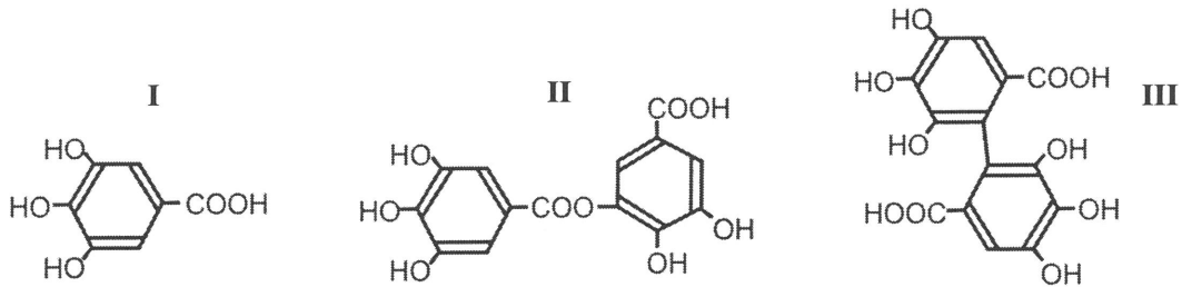
Şekil 1.12. Gallotanenler (I-gallik asit ve II-m-digallik asit) ile ellajiktanenlerin (III-hekzahidroksidifenik asit) molekül yapıları (Mangan 1988)
