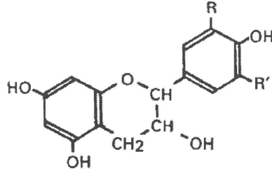
Şekil 1.13. Kondanse tanenlerin (flavan-3-ol) molekül yapısı (Mangan 1988)
