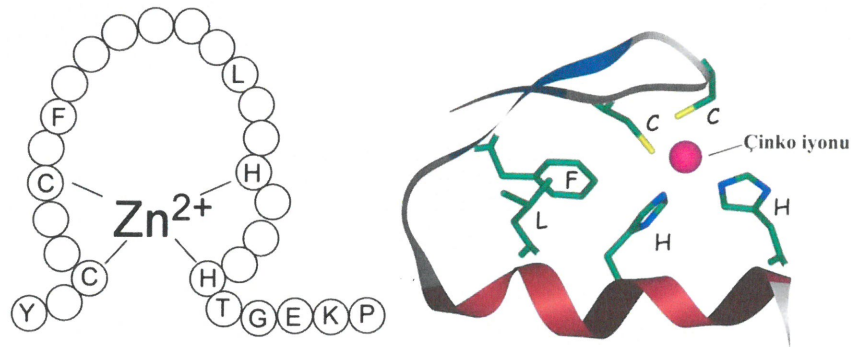
Şekil 1.3. C2H2 çinko parmağın yapısı (C, sistein; H, histidin) (Anonim 2014b)
