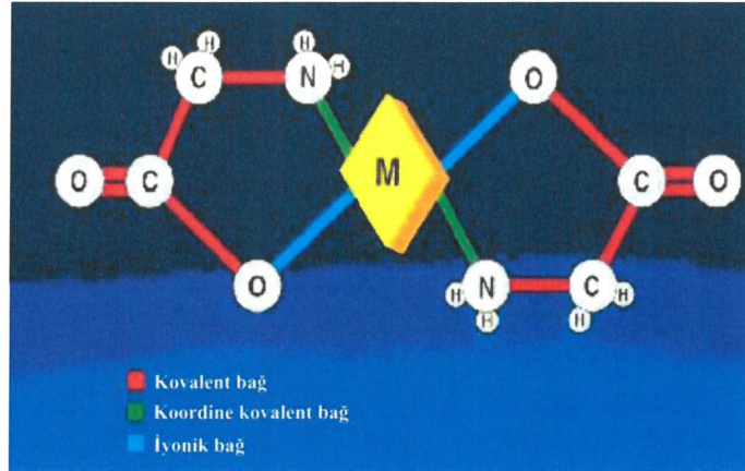
Şekil 1.4. Organik iz mineralin yapısı (Hardy 2003)
