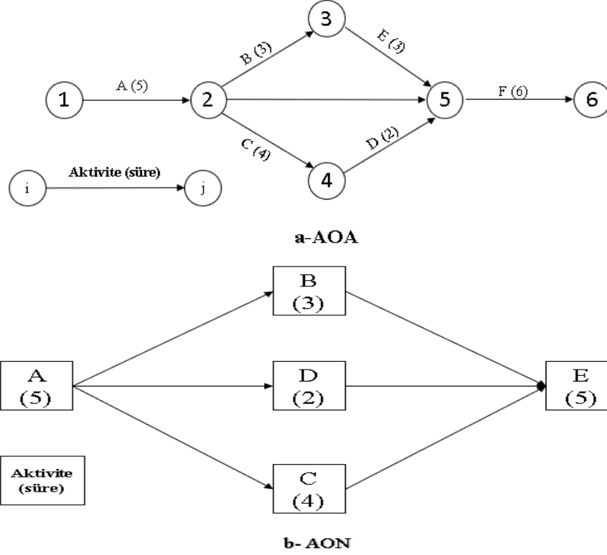
Şekil 2.4. AOA ve AON diyagramları (Değirmenci 2008)
