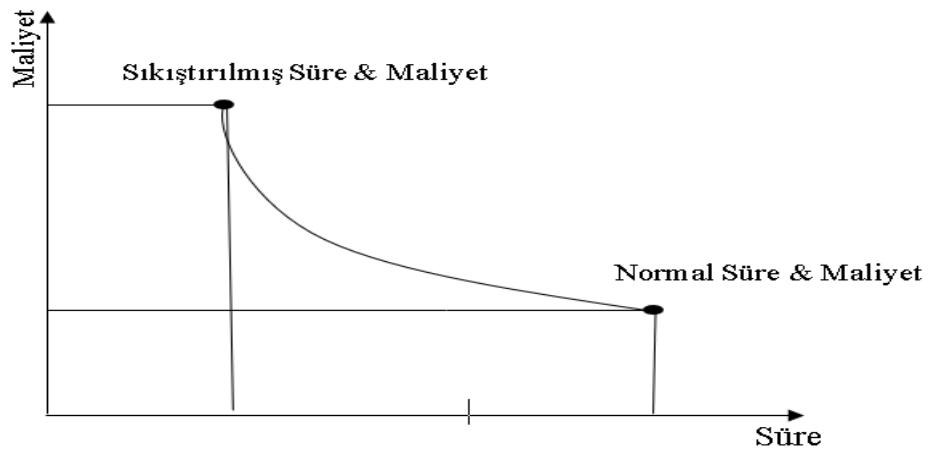
Şekil 2.9. Aktivite için lineer olmayan süre-maliyet ödünleşimin örneği
