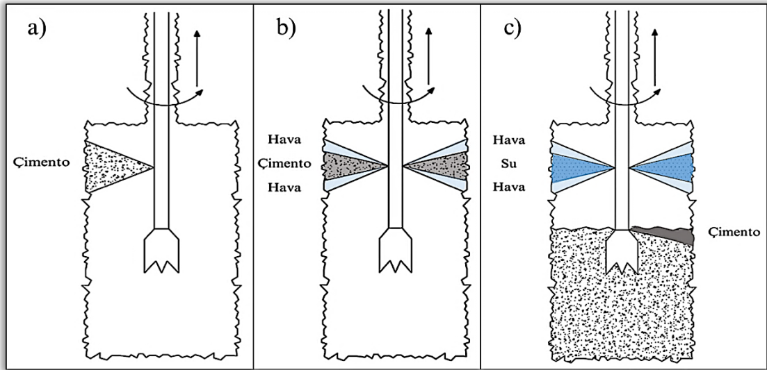
Şekil 2.10. Jet grout zemin iyileştirmede yöntemleri (a) Tek Akışkanlı Sistem, (b) İki Akışkanlı Sistem, (c) Üç Akışkanlı Sistem
