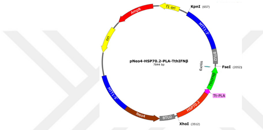
Şekil 6.6. pNeo4-HSP70.2-PLA-Tt-hIFN \beta -6XHis Vektör Yapısı. Genom entegrasyonu için oluşturulan orijinsiz vektörde gösterildiği üzere MTT1 gen lokusunun MTT1-5’ ile MTT1-3’ uç dizi bölgeleriyle homoloji kolları oluşturulmuş, bu iki kol arasına yerleştirilen kaset, böylelikle organizmanın genomunda MTT1 gen lokusuna homolog rekombinasyon ile entegre edilebilecektir. MTT1-5’ ile MTT1-3’ uç bölgeleri arasında ayrıca CdCl 2 (ağır metal) ile indüklenebilen MTT1 promotörü ve bu promotörün kontrolünde antibiyotik seçilimine olanak sağlayacak olan Neomisin direnç geni, BTU2 transkripsiyon sonlandırma bölgesi bulunmaktadır. Devamında ısı-şoku ile indüklenen T.thermophila ’nın HSP70-2 promotörü ve dışarı salgılatma dizisi PLA ve T.thermophila ’ya kodon uyumlu interferon beta geni ve 6XHis takısı yer almaktadır.
