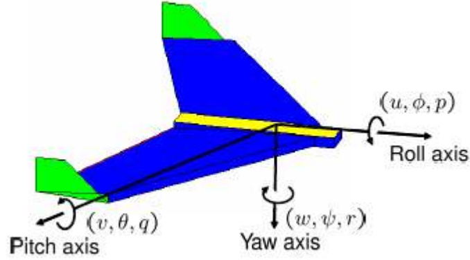
Şekil 4.5 Eksen tanımları
