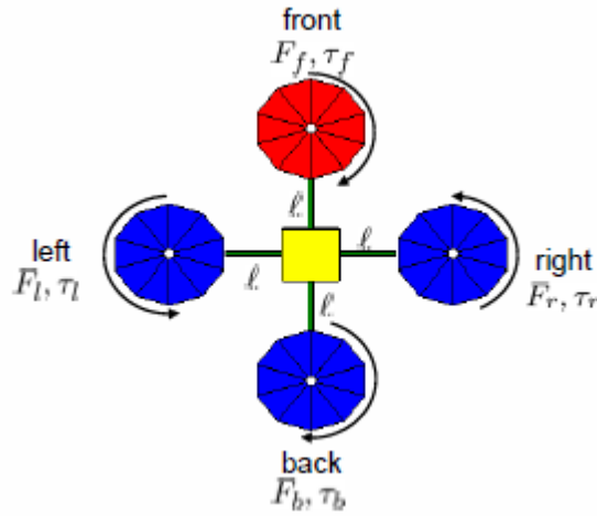
Şekil 4.6 İHA'ya yukardan bakış, tork ve kuvvetler
