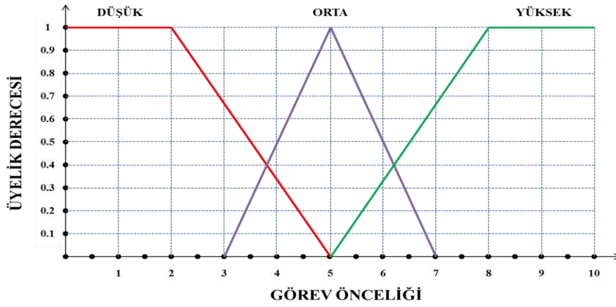
Şekil 5.9. Görev Önceliği Üyelik Fonksiyonu
