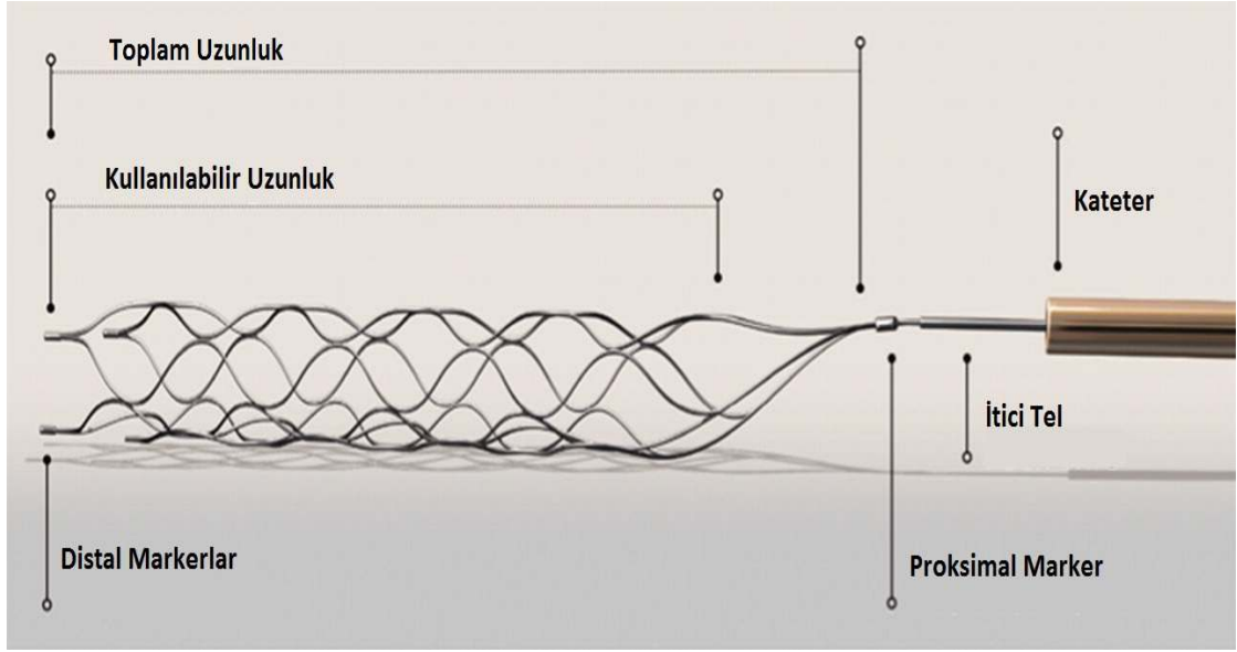
Şekil 10. Solitaire stent 114
