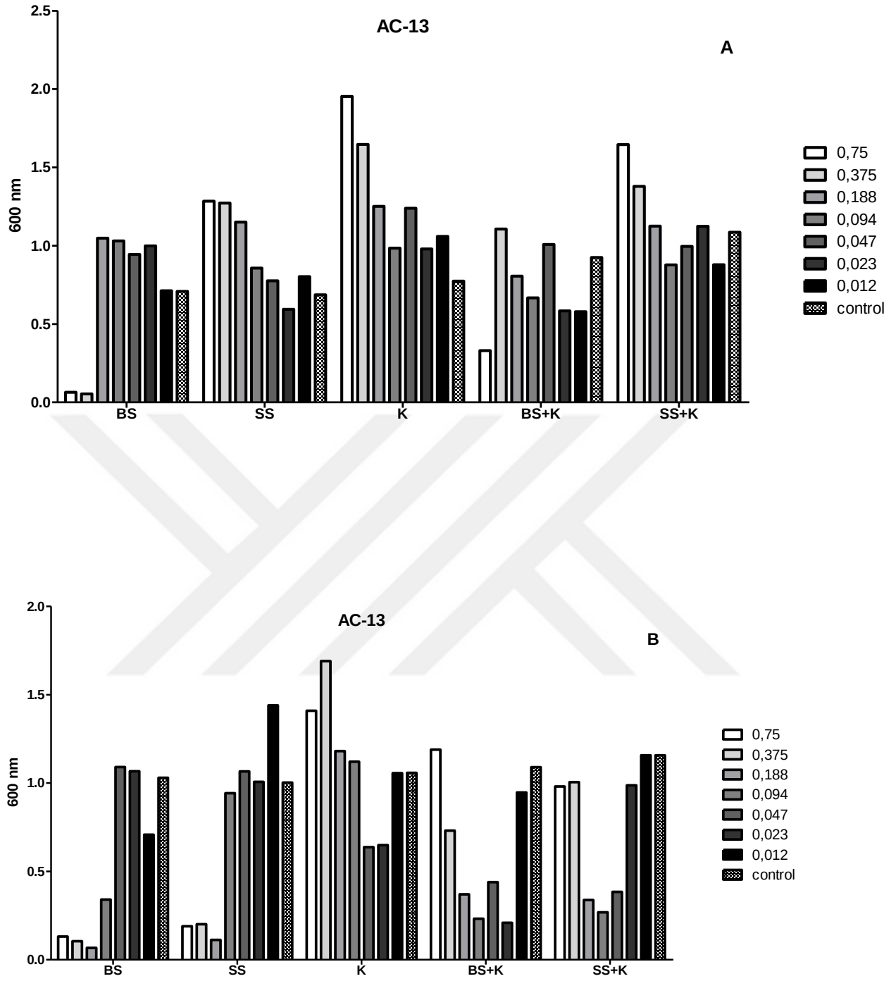
Şekil 4.19. A. A. baumannii -13 izolatın su ekstratı MIC grafiği B. A. baumannii -13 izolatın etil alkol ekstratı MIC grafiği
