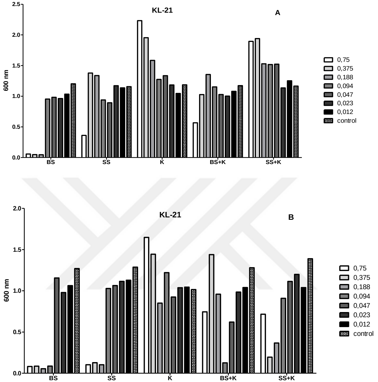
Şekil 4.11. A. K. pneumoniae -21 izolatın su ekstratı MIC grafiği B. K. pneumoniae -21 izolatın etil alkol ekstratı MIC grafiği
