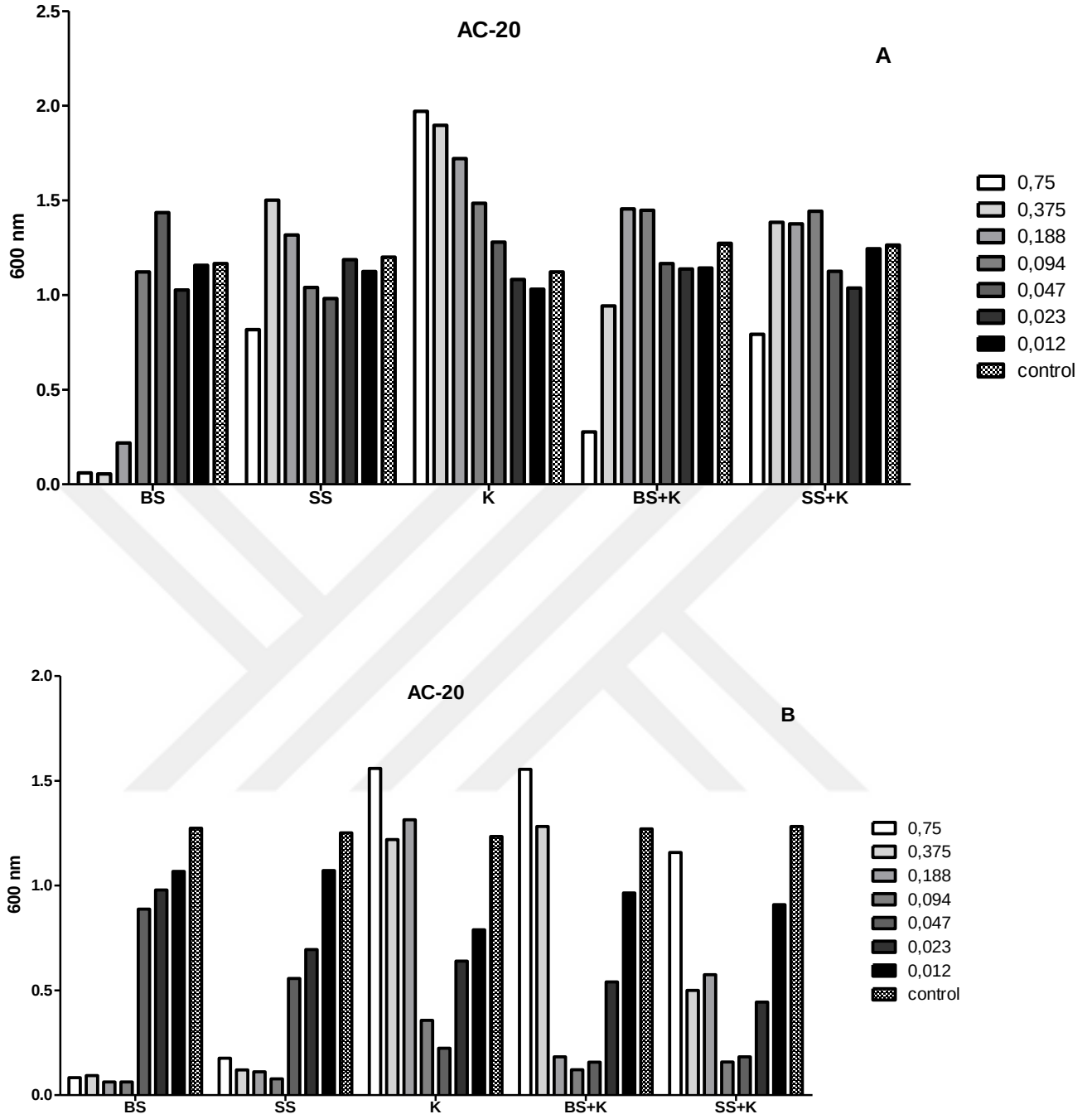
Şekil 4.20. A. A. baumannii -20 izolatın su ekstratı MIC grafiği B. A. baumannii -20 izolatın etil alkol ekstratı MIC grafiği
