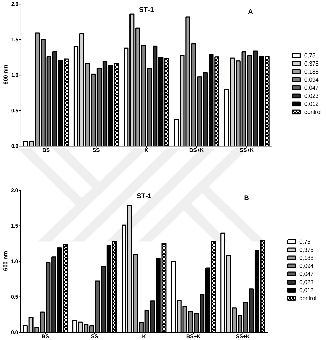
Şekil 4.12. A. Staphylococcus aureus -1 izolatın su ekstratı MIC grafiği B. Staphylococcus aureus -1 izolatın etil alkol ekstratı MIC grafiği
