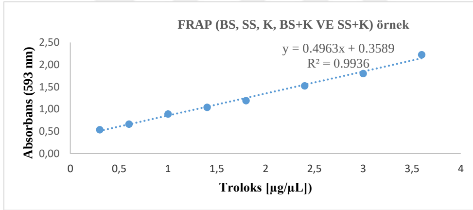
Şekil 4.26. Örnekler için Trolox standart grafiği
