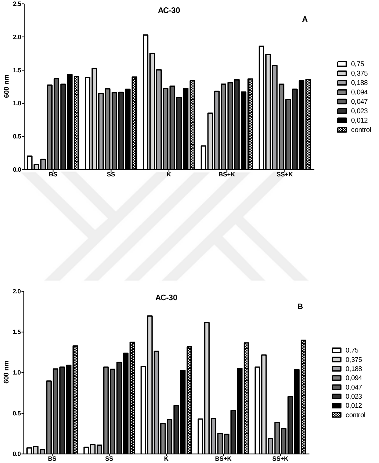
Şekil 4.21. A. A. baumannii -30 izolatın su ekstratı MIC grafiği B. A. baumannii -30 izolatın etil alkol ekstratı MIC grafiği
