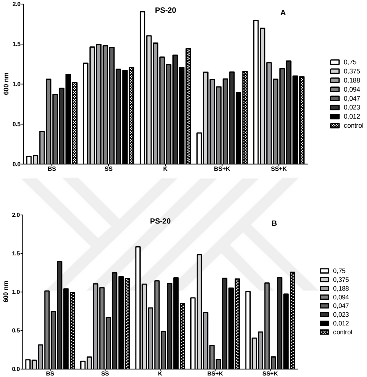
Şekil 4.5. A. P. aeruginosa -20 izolatın su ekstratı MIC grafiği B. P. aeruginosa -20 izolatın etil alkol ekstratı MIC grafiği
