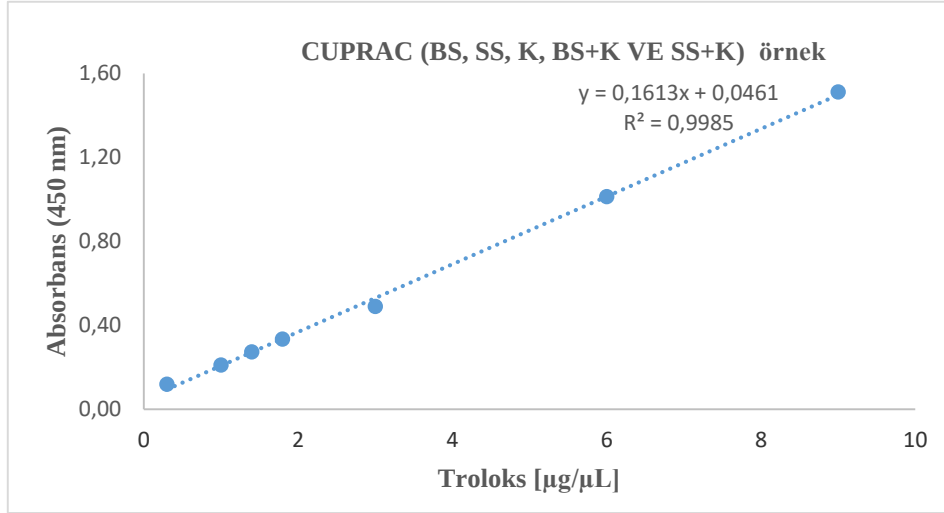
Şekil 4.25. Örnekler için Trolox standart grafiği
