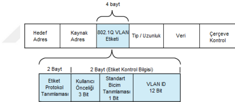
Şekil 2.8. 802.1q protokolü etiket yapısı
