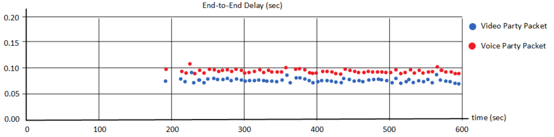
Şekil 4.9. SRC ağından DST1 ağına giden ses ve video paketleri için gecikme değerleri (a) önceliklendirme algoritması uygulanmadan önce (b) önceliklendirme algoritması uygulandıktan sonra
