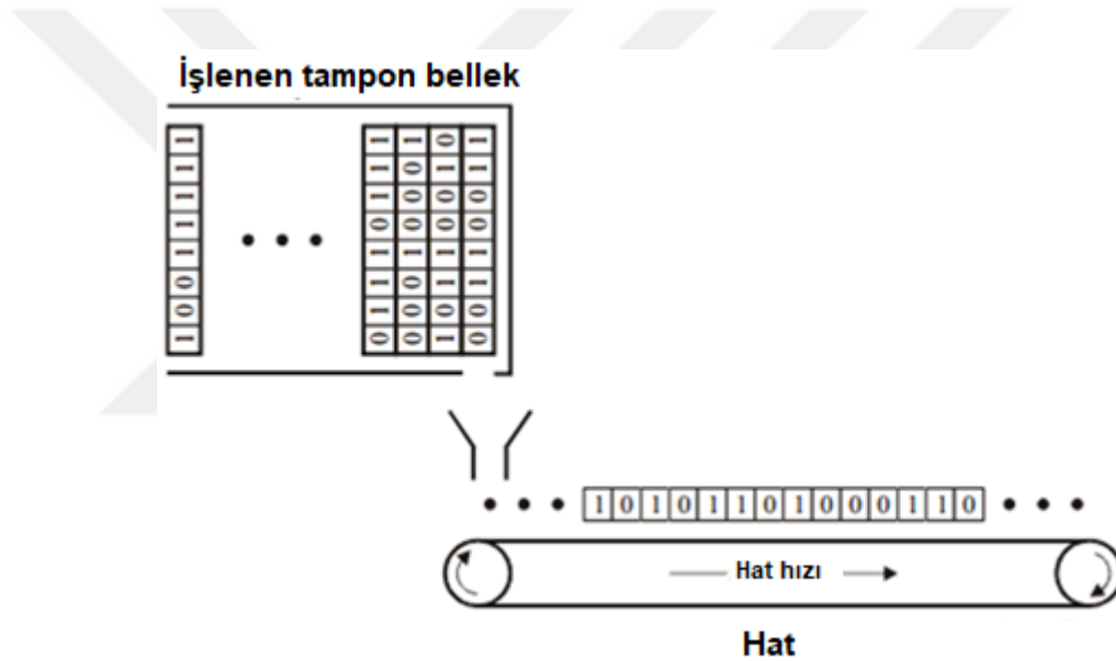
Şekil 2.4. Sıralama gecikmesi gösterimi
