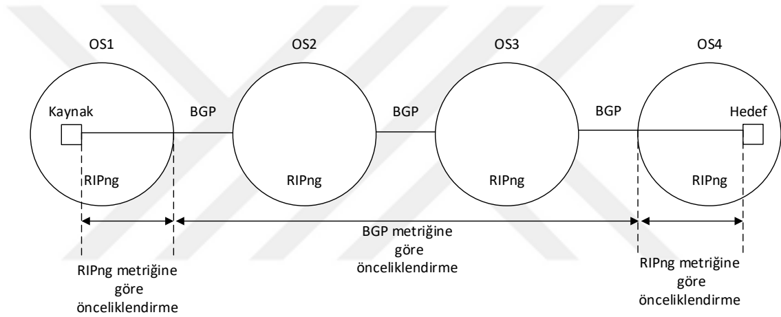
Şekil 4.14. BGP protokol metrik değerine göre yapılan önceliklendirmeye ait blok yapı
