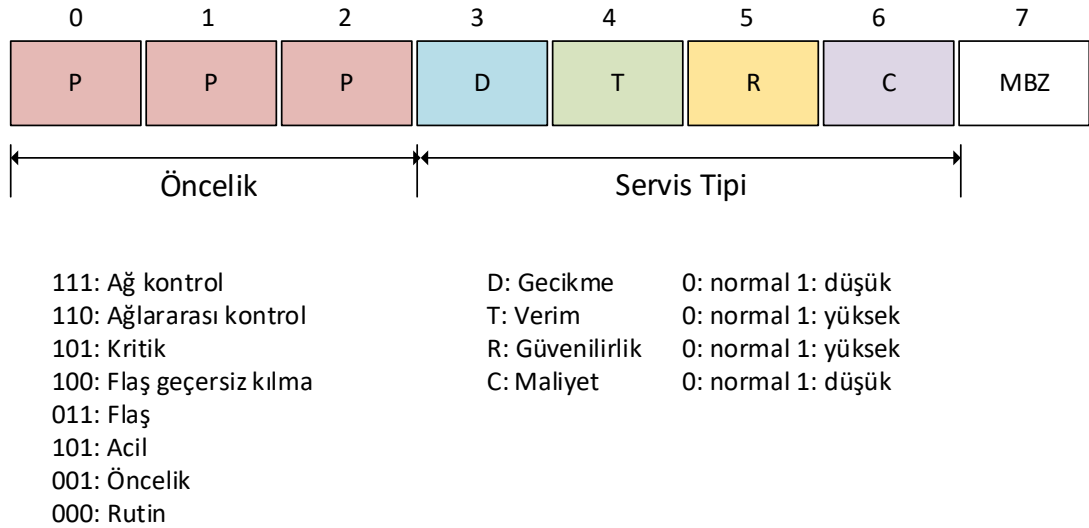
Şekil 2.10. IP başlığı içerisindeki önceliklendirme ve servis bitleri
