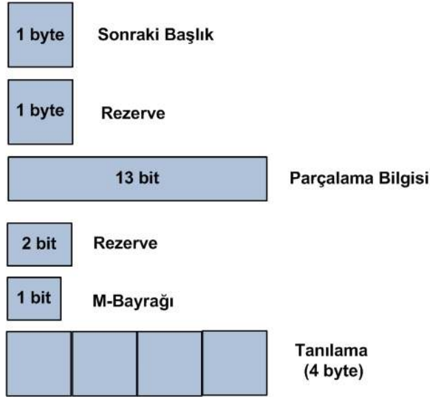
Şekil 6. IPv6 parçalama başlığı
