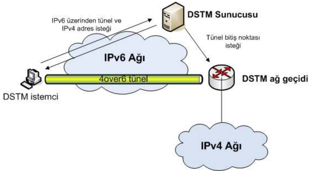
Şekil 24. DSTM mimarisi
