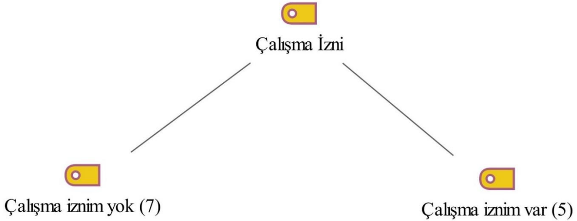
Şekil 3.9. Çalışma İzni
