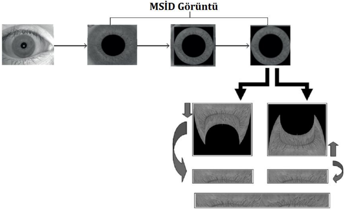
Şekil 2.11. İris görüntüsünün normalizasyon süreci [72].
