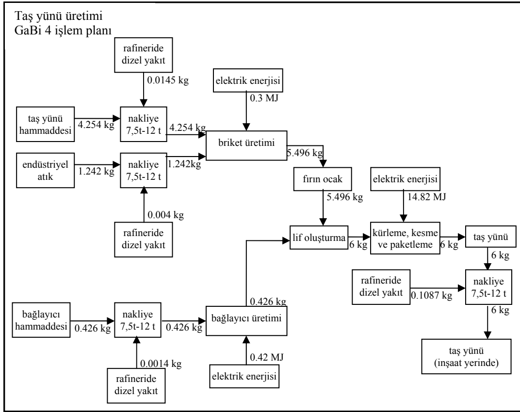
Şekil 3.7. Taş yünü üretimi işlem planı
