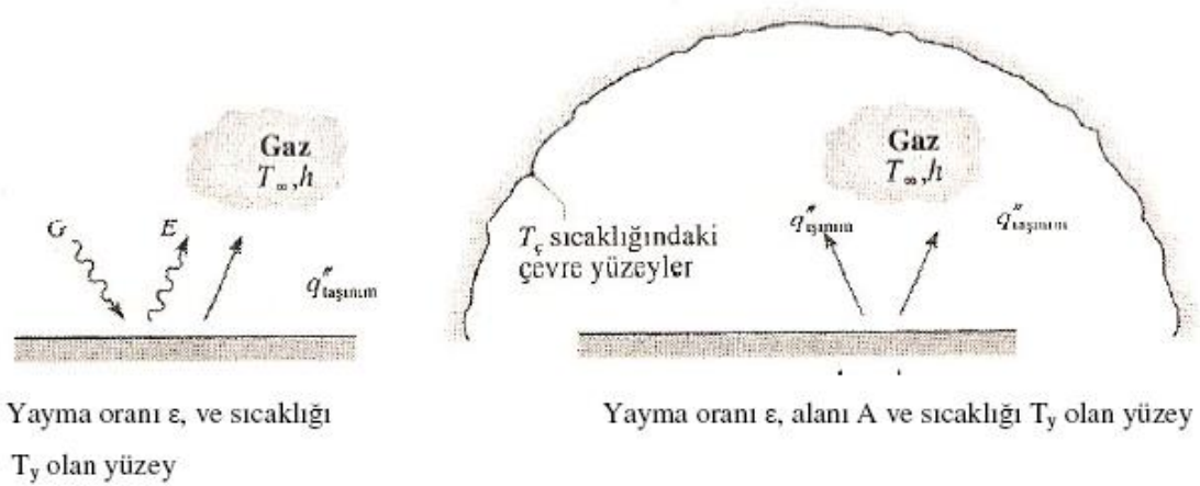
Şekil 1.3. Isınım ile ısı alışverişi (a) bir düzeyde (b) bir yüzey ile daha büyük çevre yüzeyler arasında [26].
