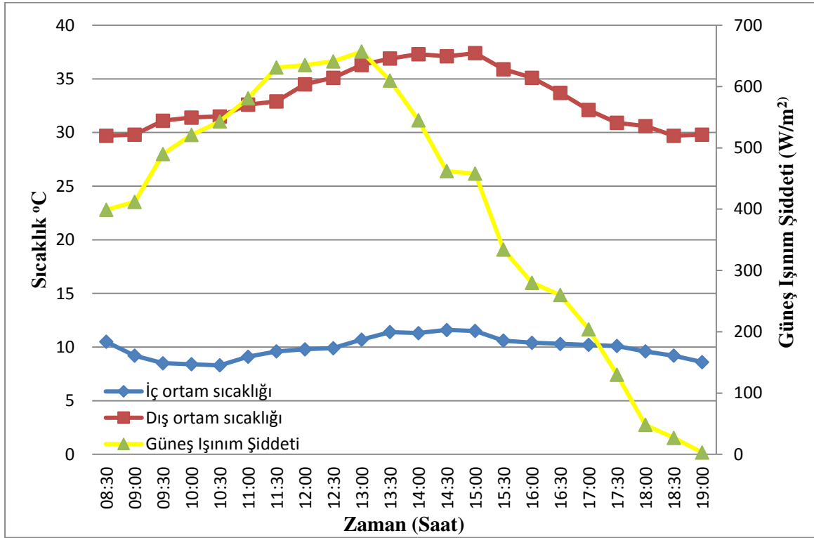
Şekil 3.13. Taşyünü kaplı deney odası için iç ve dış ortam sıcaklığın ve güneş ışıınım şiddetinin zamana bağılı değışimi
