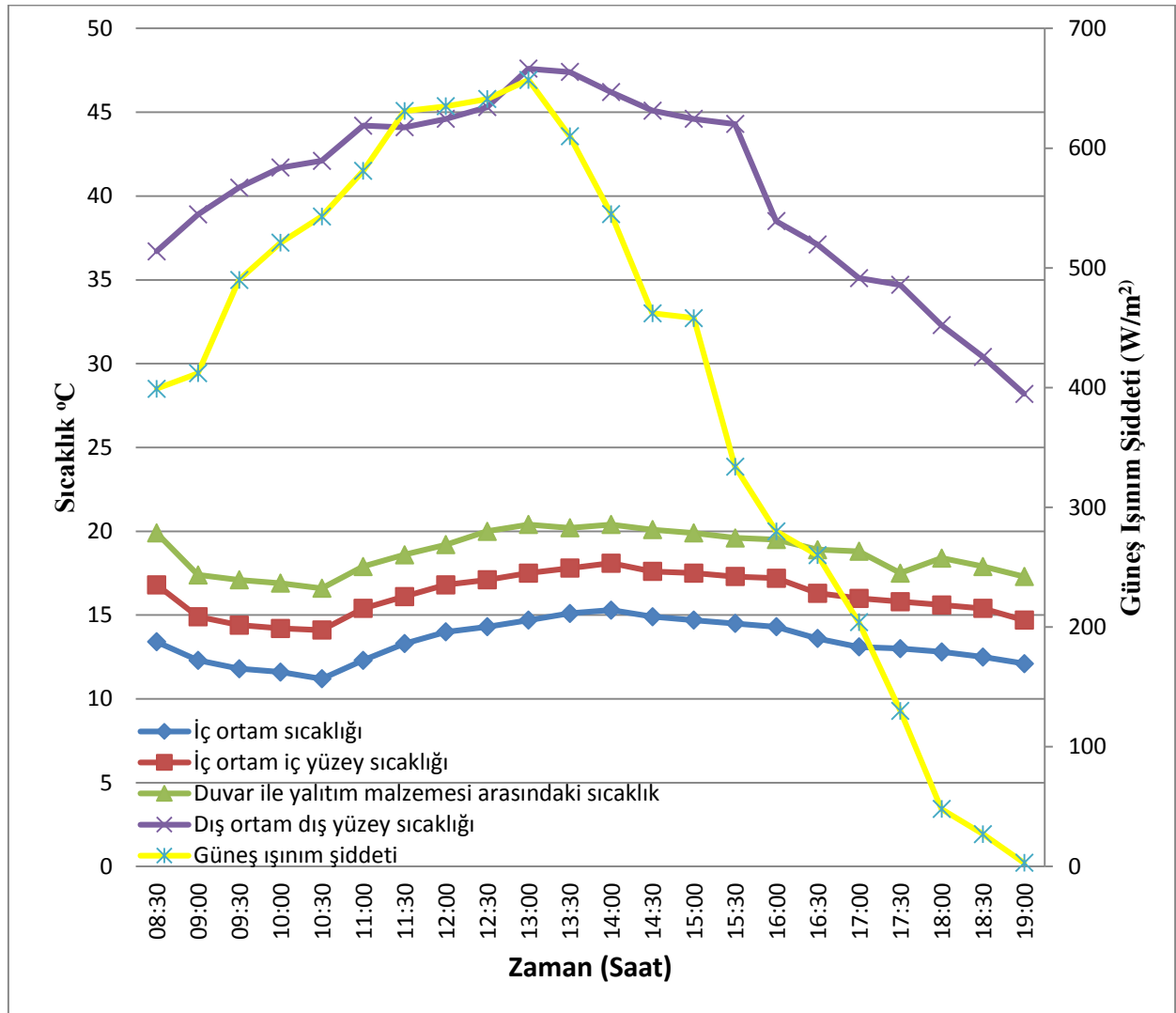
Şekil 3. 8. XPS Kaplı deney odası için zamana bağlı sıcaklık ve güneş ışıınım şiddeti ölçümler
