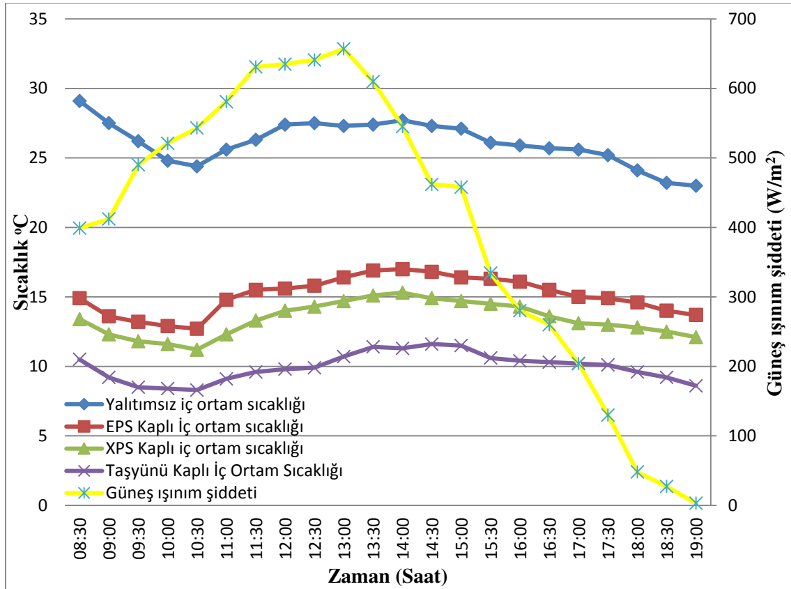
Şekil 3.14. Yalıtımsız ve Yalıtımlı durumlar için iç ortam sıcaklığının ve güneş ışınlam şiddetinin zamana bağlı değişimi
