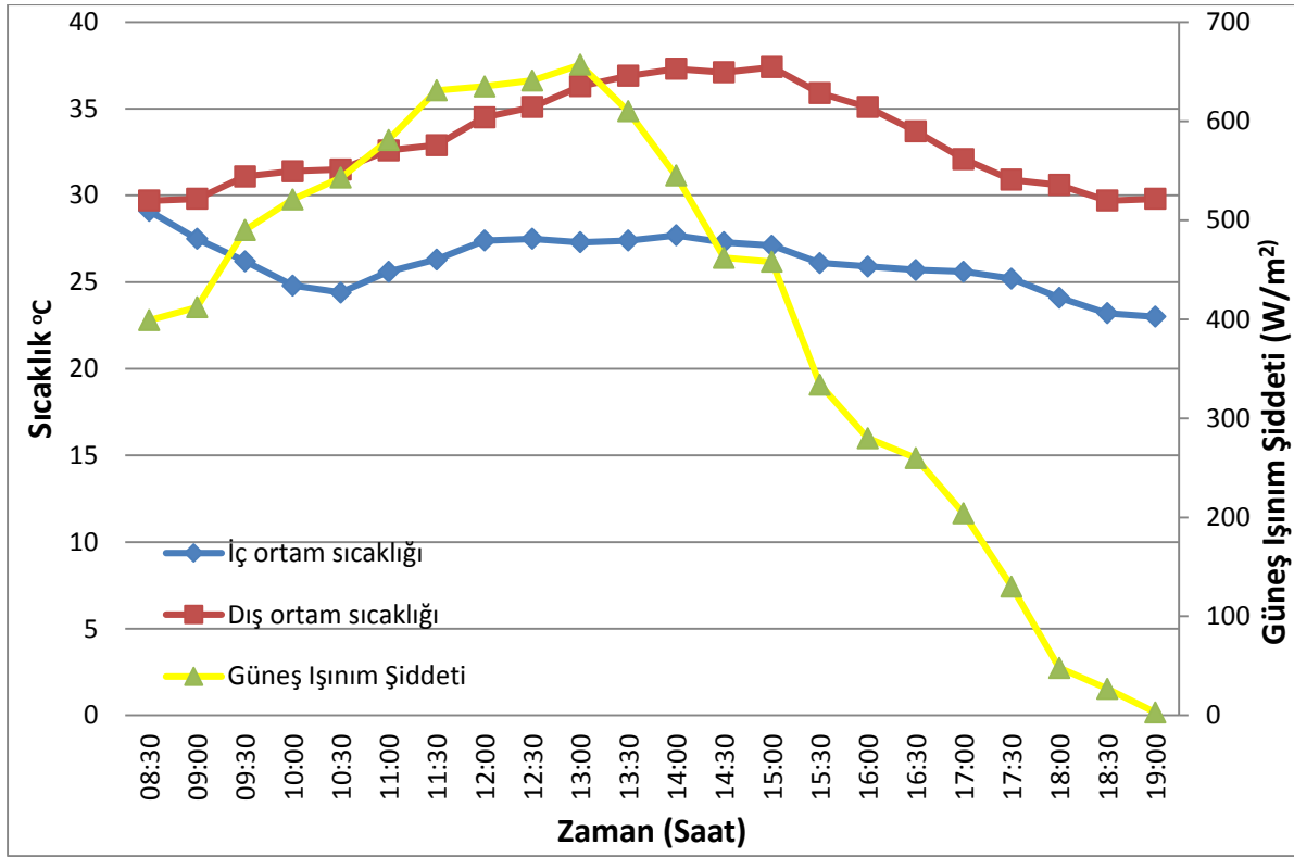
Şekil 3.10. Yalıtımsız iç ve dış ortam sıcaklığının ve güneş ışınım şiddetinin zamana bağlı değişimi
