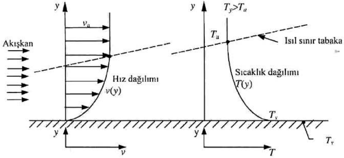
Şekil 1.2. Levha üzerindeki akışta hız ve sıcaklık dağılımları [25].
