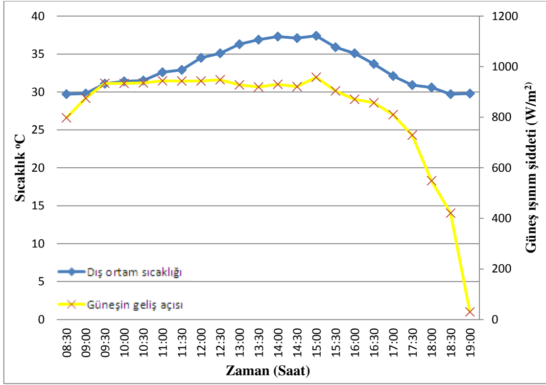
Şekil 3. 17. Dış ortam sıcaklığının ve güneş ışıınım şiddetinin zamana bağlı değişimi
