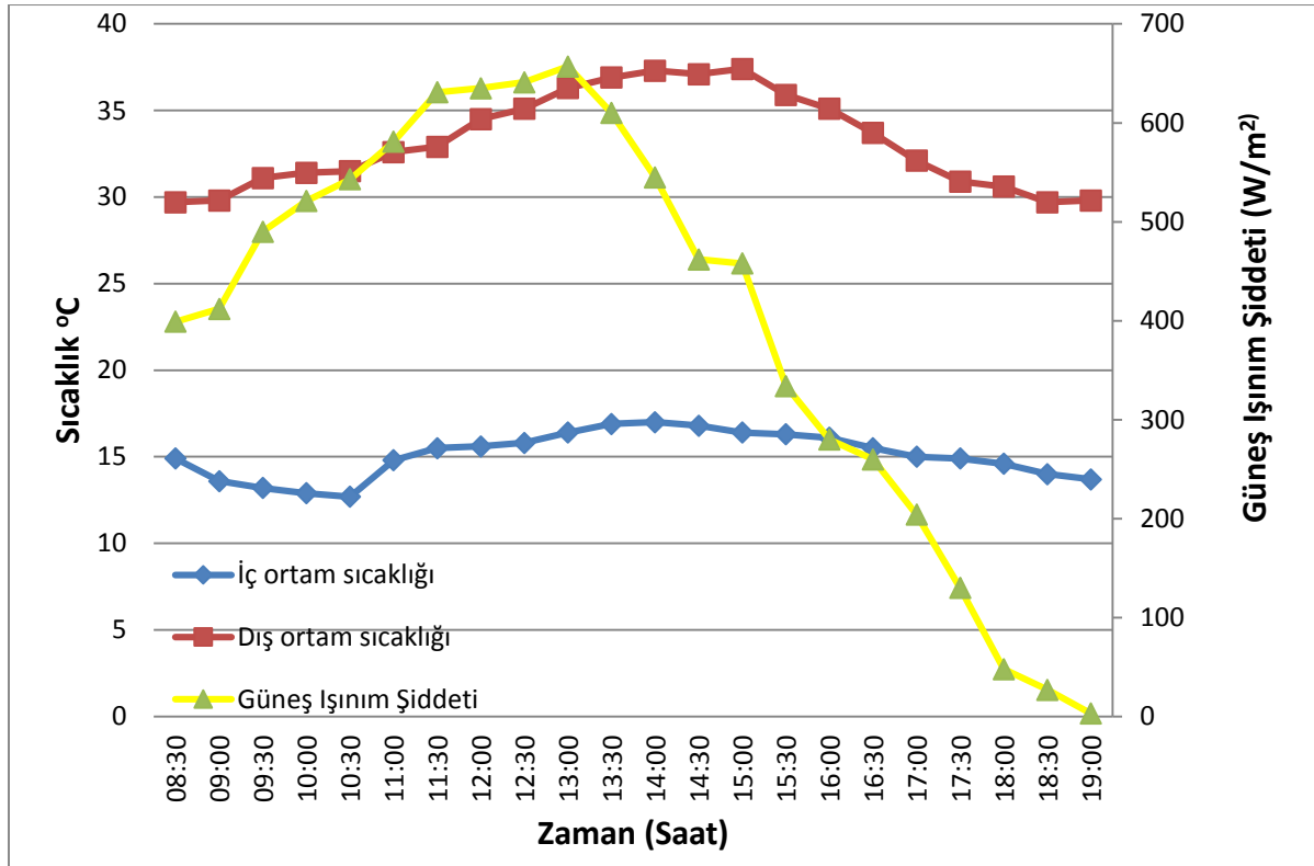
Şekil 3.11. EPS kaplı deney odası için iç ve dış ortam sıcaklığının ve güneş ışınım şiddetinin zamana bağlı değişimi
