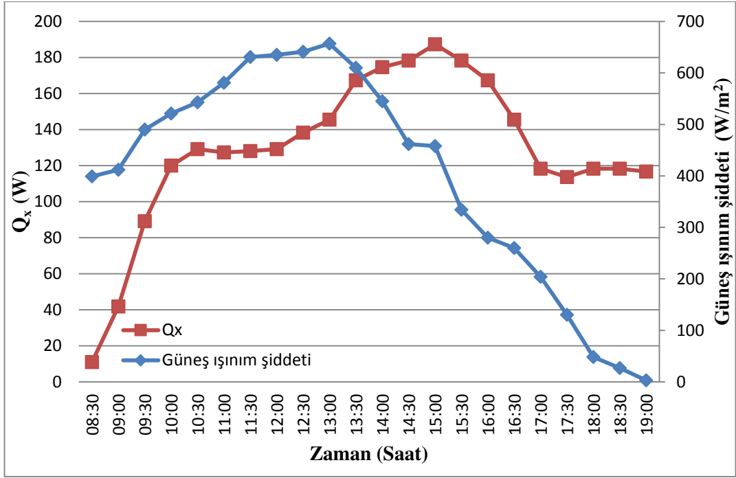
Şekil 3.2. Yalıtımsız deney odası için soğutma yükü ve güneş ışınlm şiddetinin zamana bağlı grafiğı
