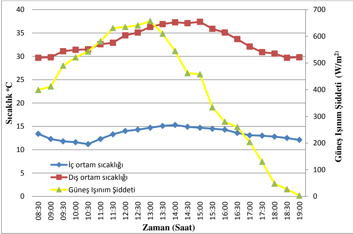
Şekil 3. 12. XPS kaplı deney odası için iç ve dış ortam sıcaklığın ve güneş ışıınım şiddetinin zamana bağılı değışimi
