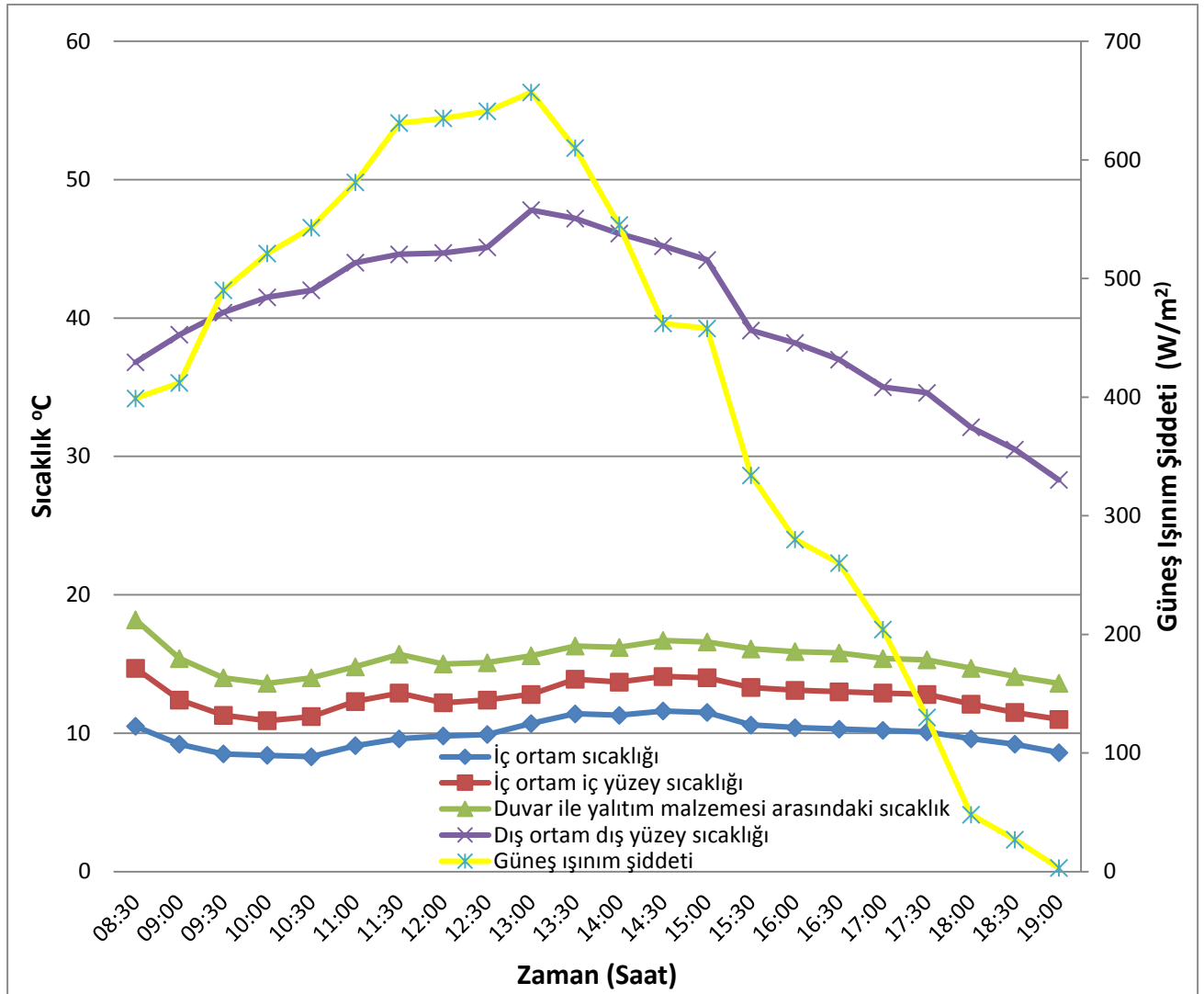
Şekil 3.9. Taşyünü Kaplı deney odası için zamana bağlı sıcaklık ve güneş ışıınım şiddeti ölçümler
