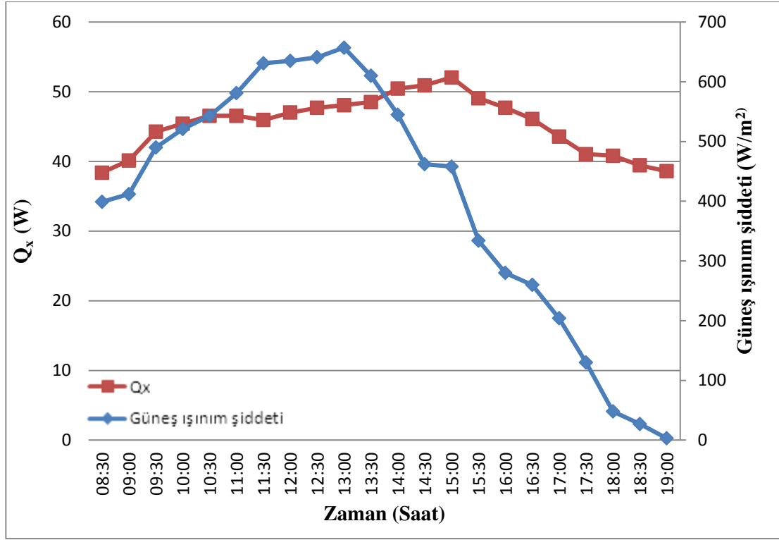
Şekil 3. 4. XPS kaplı deney odası için soğutma yükü ve güneş ışınlm şiddetinin zamana bağlı grafiğı
