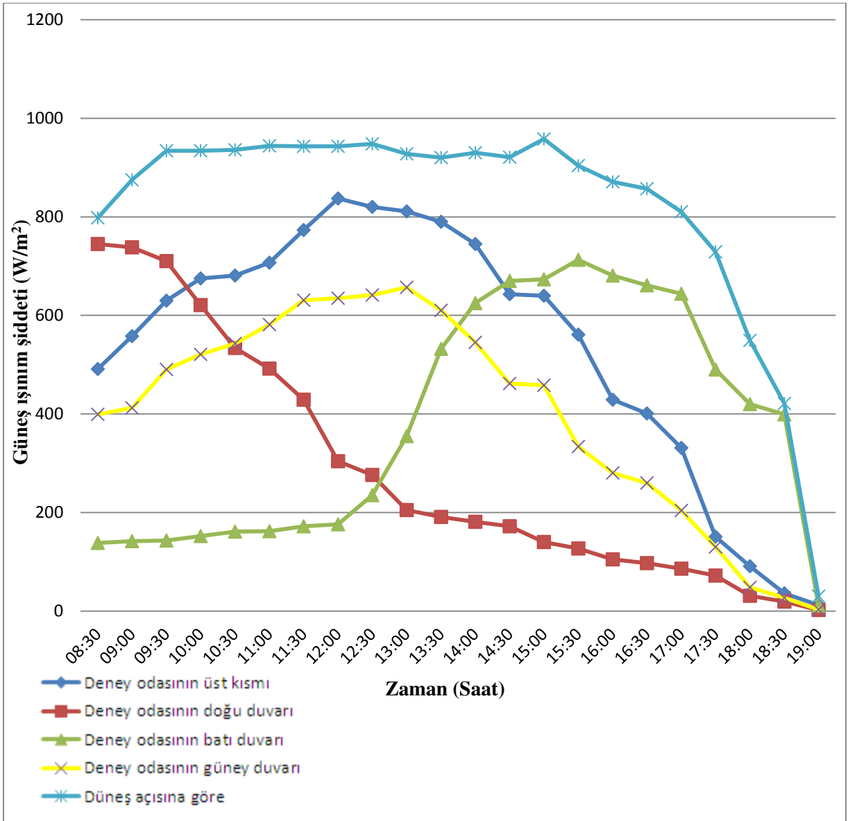
Şekil 3. 18. Güneş ışınlam şiddetinin gün içinde geliş yönlerinin zamana bağlı değişimi
