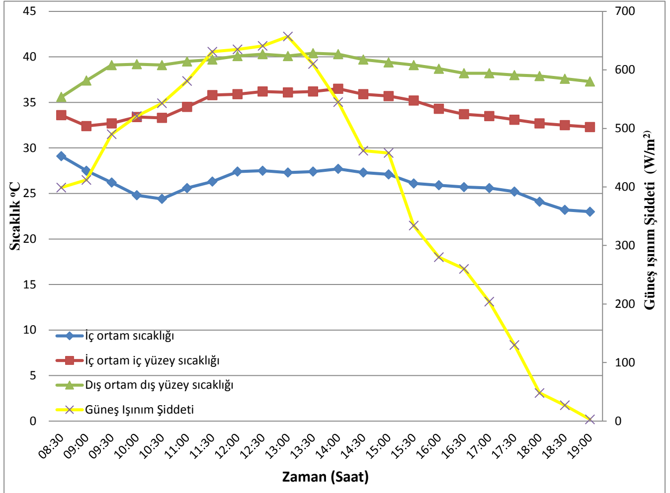
Şekil 3.6. Yalıtımsız deney odası için zamana bağlı sıcaklık ve güneş ışıınım şiddeti ölçümleri
