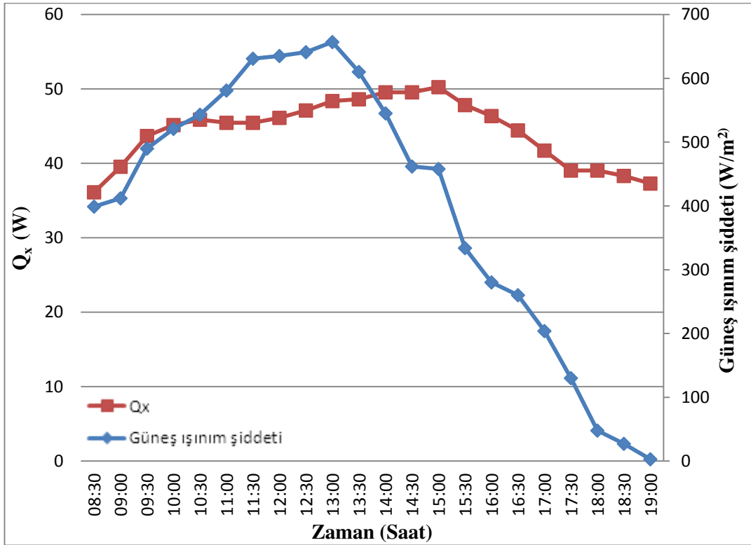
Şekil 3.2. Yalıtımsız deney odası için soğutma yükü ve güneş ışınlm şiddetinin zamana bağlı grafiğı
