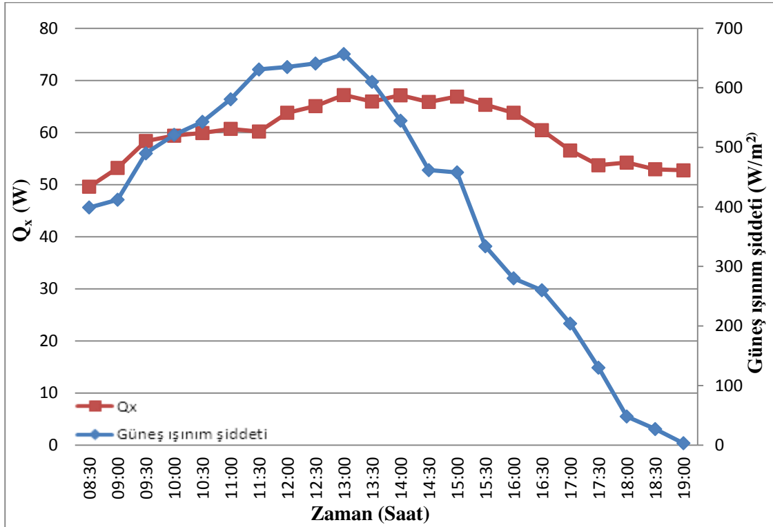
Şekil 3.5. Taşyünü kaplı deney odası için soğutma yükü ve güneş ışınlm şiddetinin zamana bağlı grafiğı
