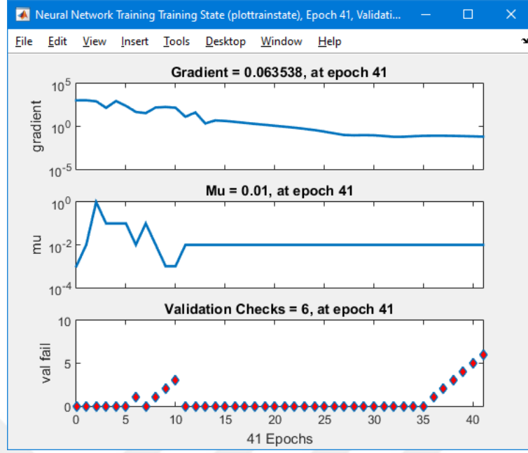
Şekil 4.11. Yapay sinir ağı modeli eğitim durumu grafiği
