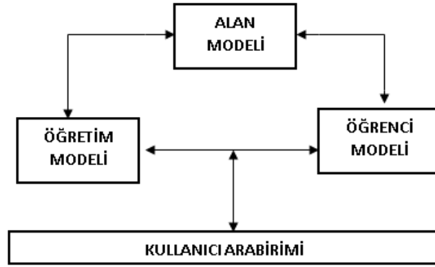
Şekil 3.7. Zeki öğretim sisteminin temel yapısı (Dağ ve Erkan, 2004)
