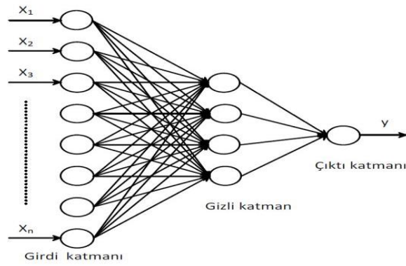
Şekil 4.5. Yapay sinir ağı hücresi
