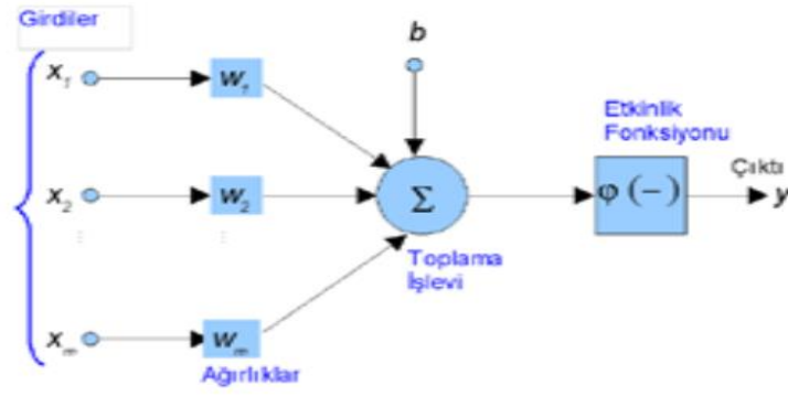
Şekil 3.3. Yapay sinir ağı hücresi
