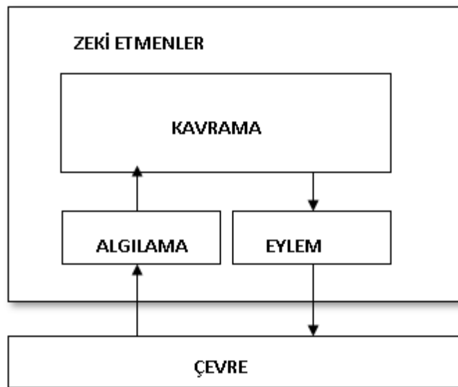
Şekil 3.6. Zeki etmen sisteminin yapısı (Aydın, 1997)
