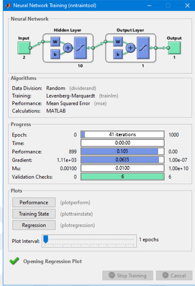
Şekil 4.9. Neural network eğitim ekranı
