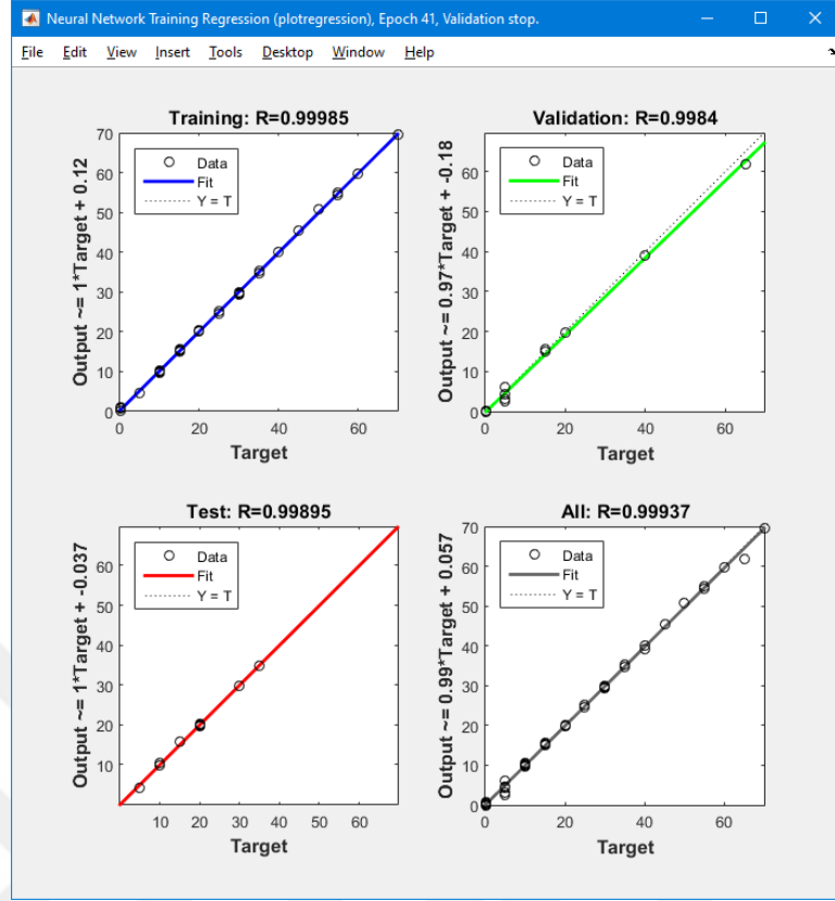
Şekil 4.10. Eğitimin regresyon ağ sonuçları
