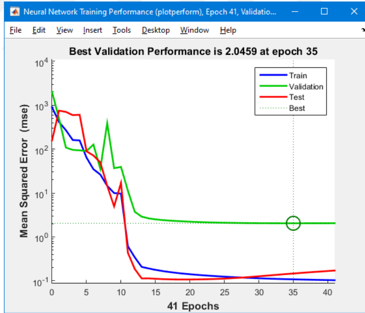
Şekil 4.12. Performans durum grafiği
