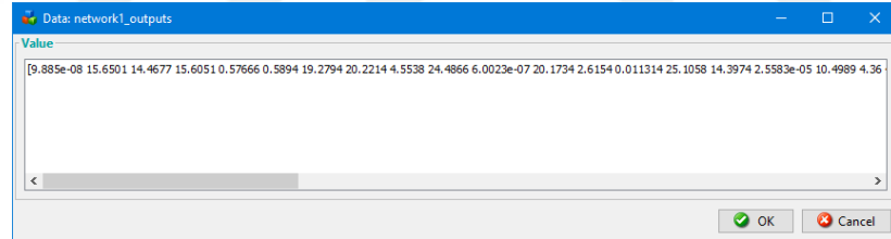
Şekil 4.14. Eğitilmiş veriler
