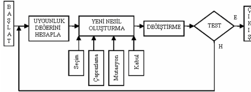
Şekil 3.4. Genetik algoritmaların akış şeması (Bolat vd., 2004)
