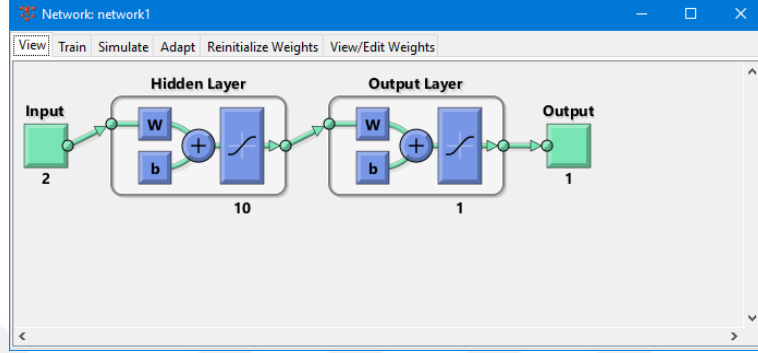
Şekil 4.8. Oluşturulan ağ sistemi
