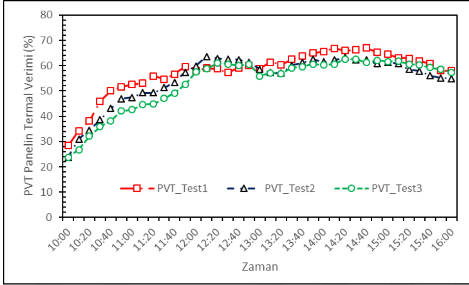
Şekil 7.23. PVT panelin termal verimi
