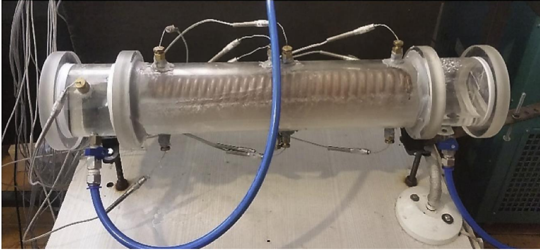
Resim 5.3. Rahimi ve diğerlerinin parafinli IED sistemi [92]
