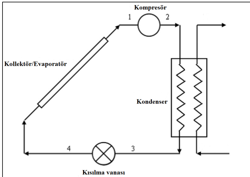
Şekil 3.3. Doğrudan genişlemeli güneş destekli ısı pompası sisteminin şeması [27]
