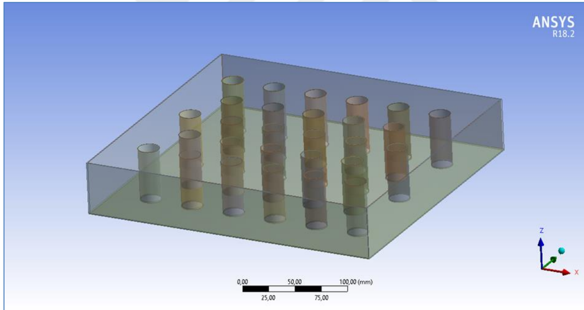
Şekil 6.1. Isıl enerji depolama ünitesinin nümerik modeli
