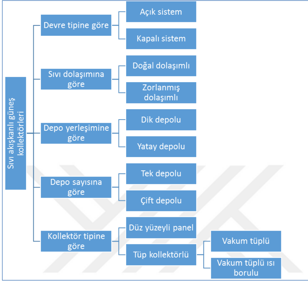
Şekil 2.2. Sıvı akışkanlı güneş kolektörlerinin sınıflandırılması [14]
