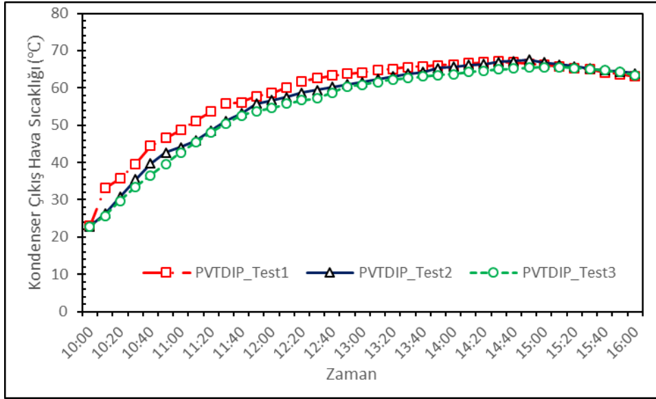
Şekil 7.25. PVTDIP sisteminin kondenser hava çıkış sıcaklığı
