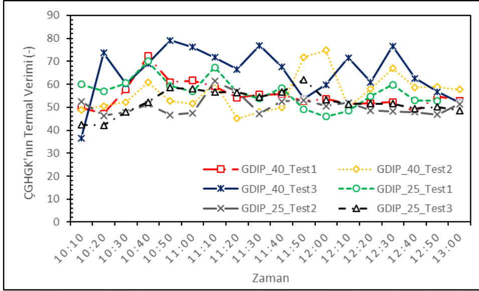
Şekil 7.18. Çift geçişli havalı güneş kollektörünün termal verimi
