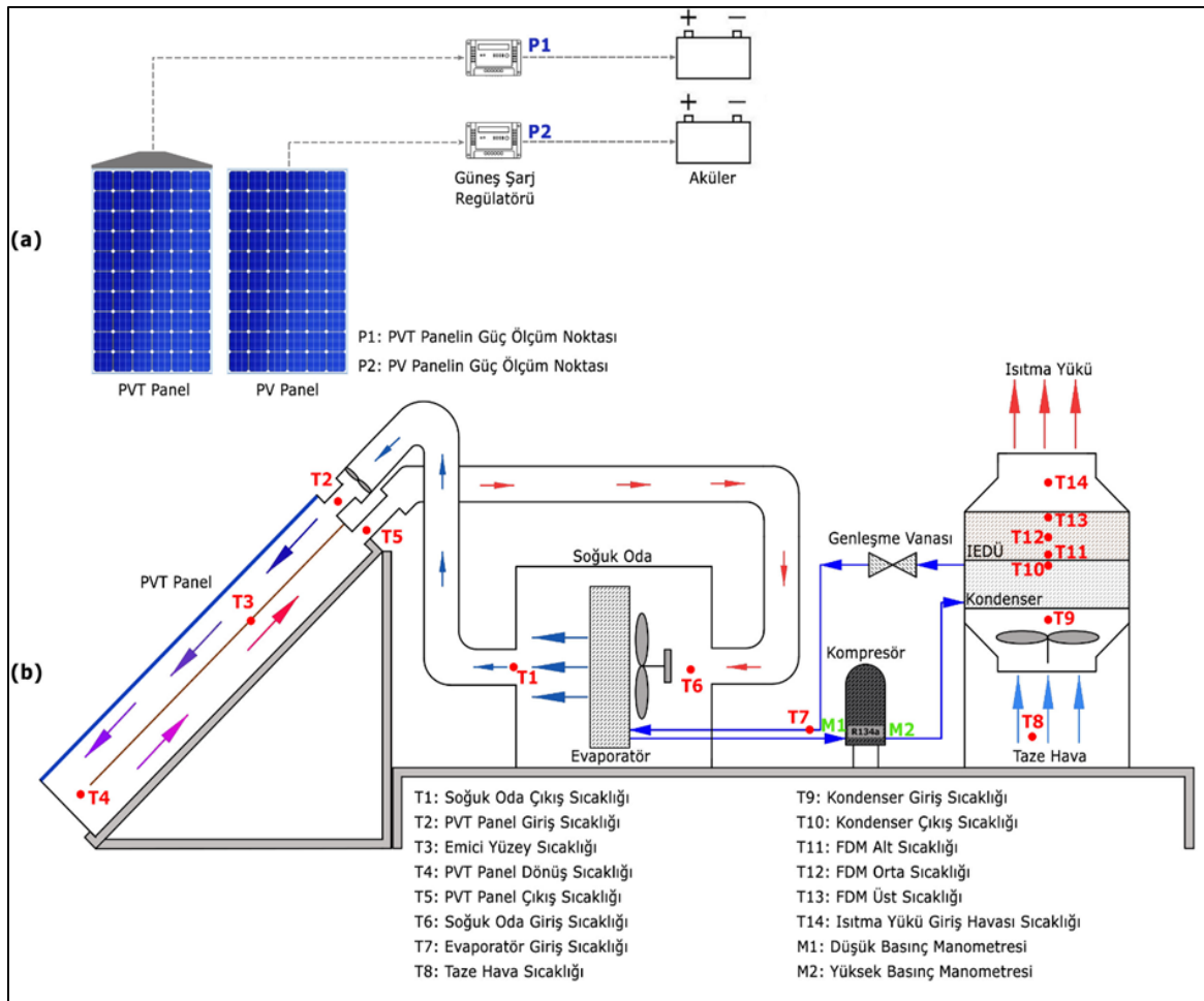
Şekil 6.8. Isıl enerji depolamalı PVT destekli ısı pompası sisteminin şematik gösterimi
