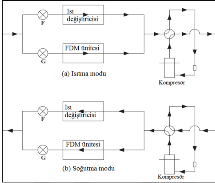
Şekil 5.3. Soğutma ve ısıtma enerjisi yükleme/boşaltma işlemine sahip hibrit bir ısı pompası [70]
