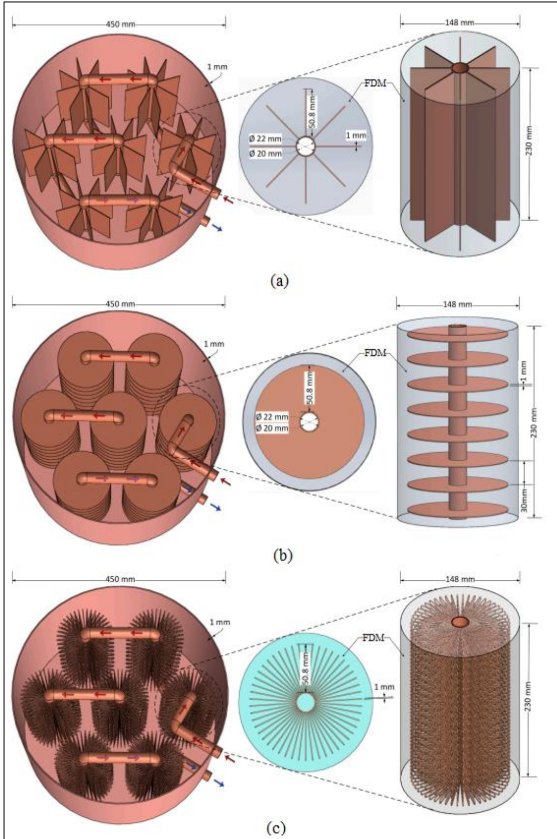
Şekil 5.9. Çok borulu geçişlere ve çeşitli uzatılmış yüzey yönlendirmelerine sahip gövde borulu ısı değiştiricisi: (a) uzunlamasına kanatçıklı, (b) dairesel kanatçıklı ve (c) tel sargılı kanatçıklı [95]
