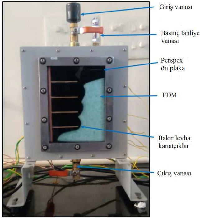
Resim 5.2. Kanatçıklı gizli ısı depolama ünitesi [89]
