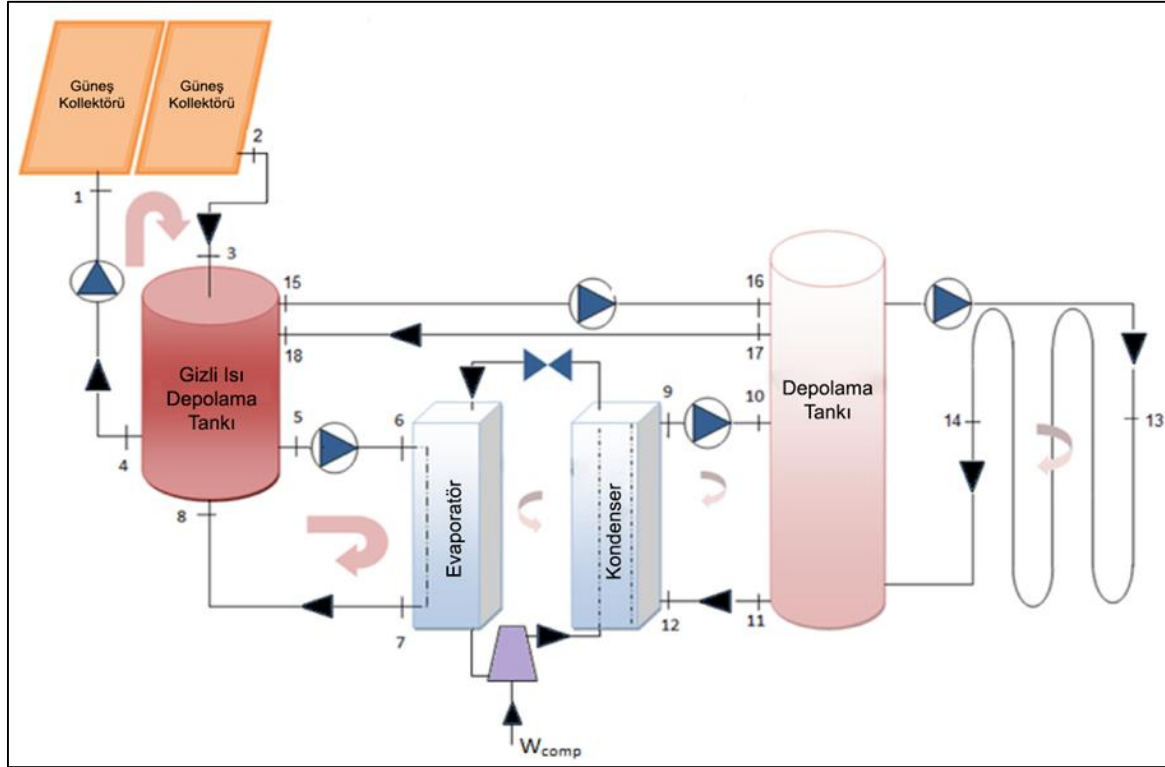
Şekil 5.4. Enerji depolamalı ısıtma sistemi diyagramı [73]
