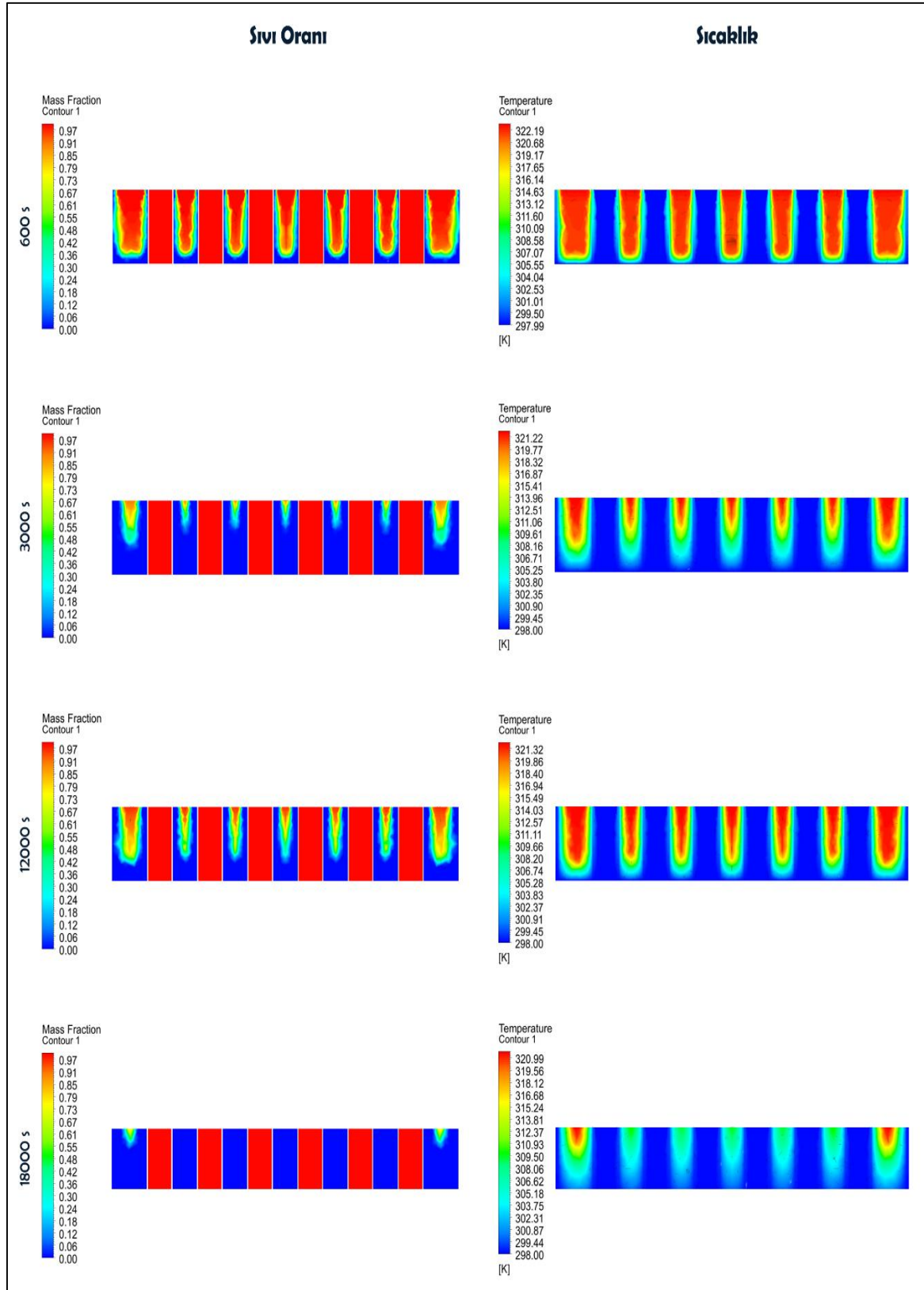
Şekil 7.4. Katılaştırma (deşarj) sırasında parafinin yarım kesit model sıvı oranı ve sıcaklık sınırları
