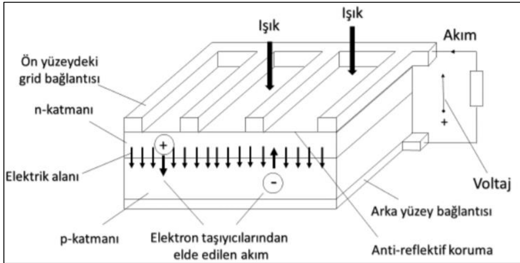
Şekil 2.5. Fotovoltaiik pilden elektrik üretimi [18]
