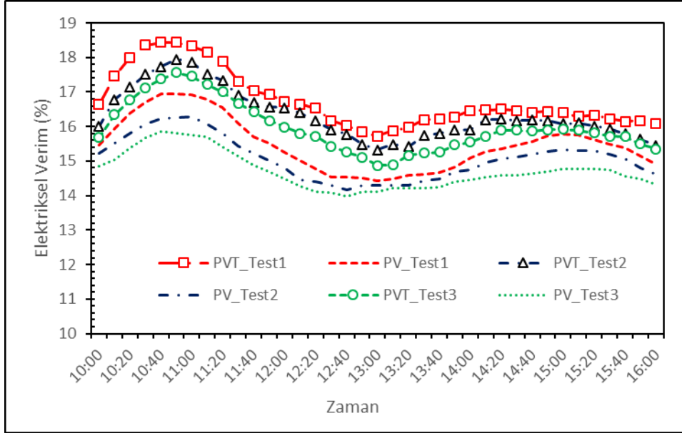
Şekil 7.22. PV ve PVT panellerin elektriksel verimleri
