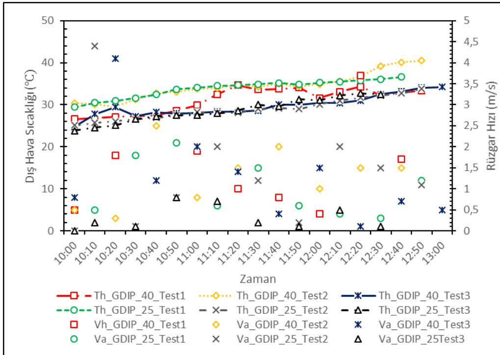
Şekil 7.14. GDIP deneylerinde zamana bağlı dış hava sıcaklığı ve rüzgâr hızı değişimi
