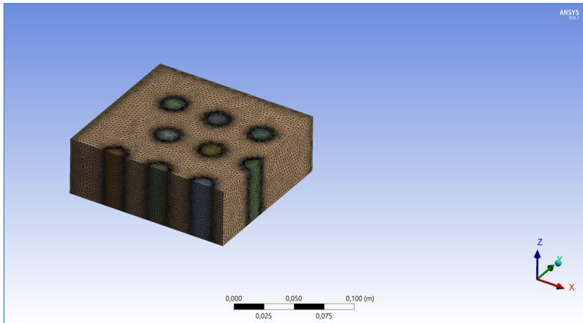
Şekil 6.2. Çeyrek simetrik modelin ağ yapısı
