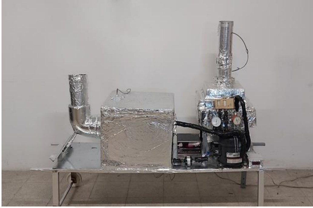
Ek-1. Isıl enerji depolamalı hava kaynaklı ısı pompası sisteminin fotoğrafi
