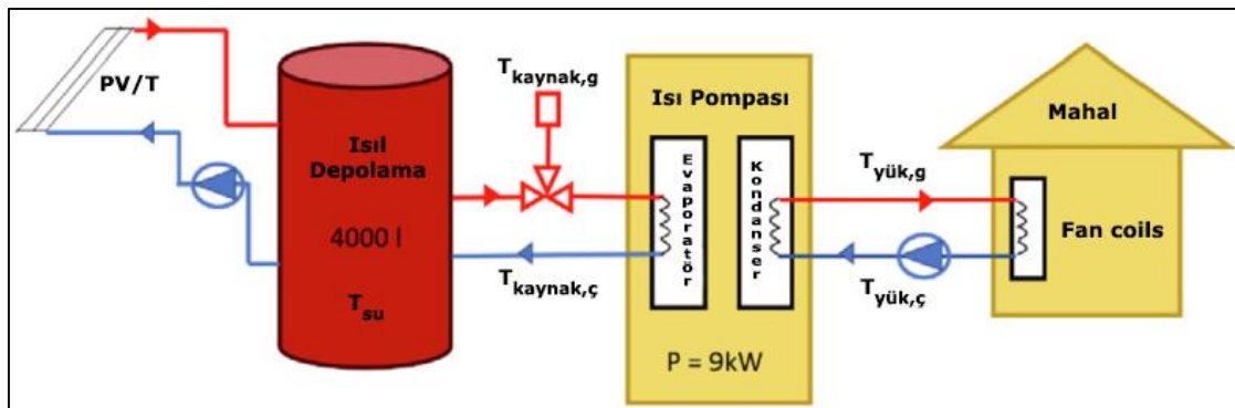
Şekil 5.7. Hibrit PVT ısı pompası sistemi [80]
