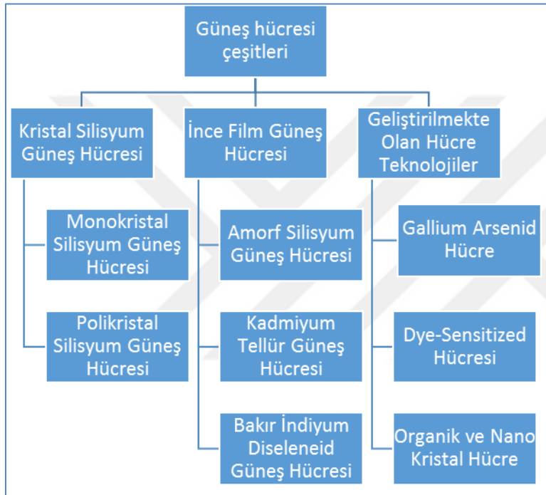
Şekil 2.6. Fotovoltaik panelde kullanılan güneş hücresi çeşitleri [19]
