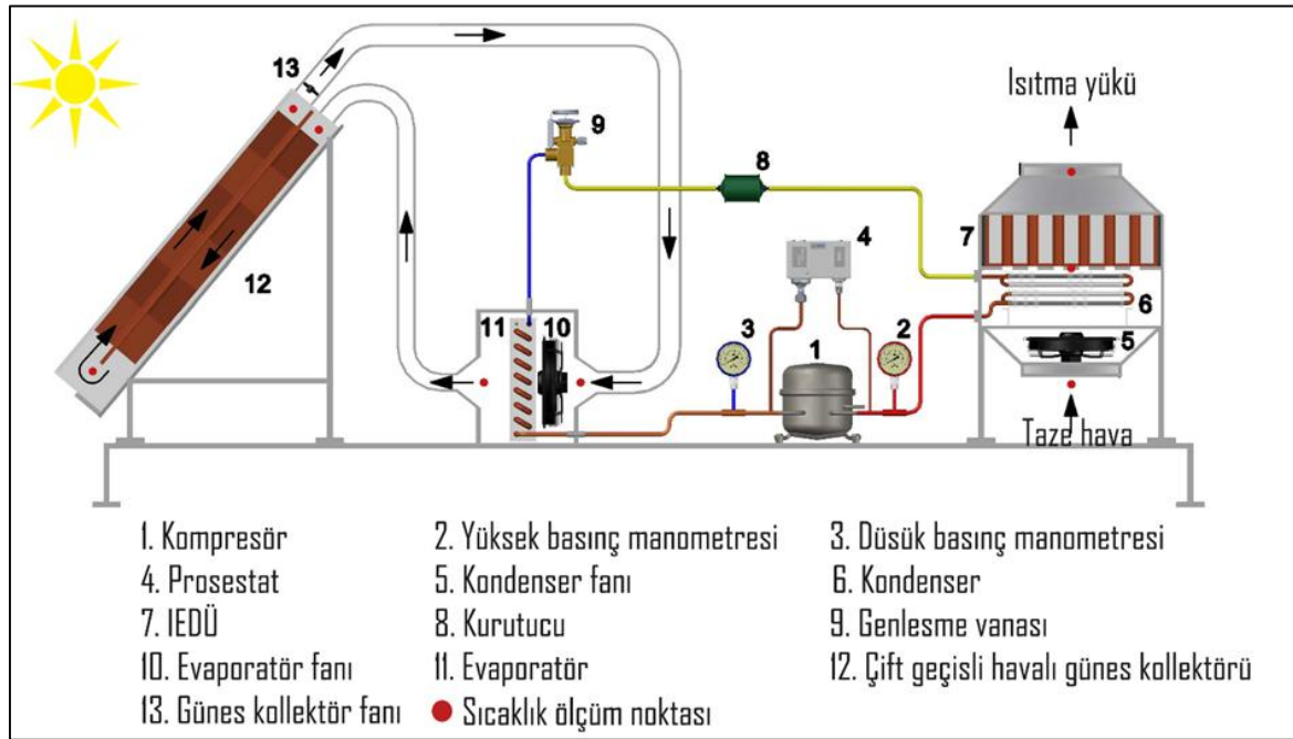
Şekil 6.7. Isıl enerji depolamalı hava kaynaklı ısı pompası sisteminin şematik gösterimi
