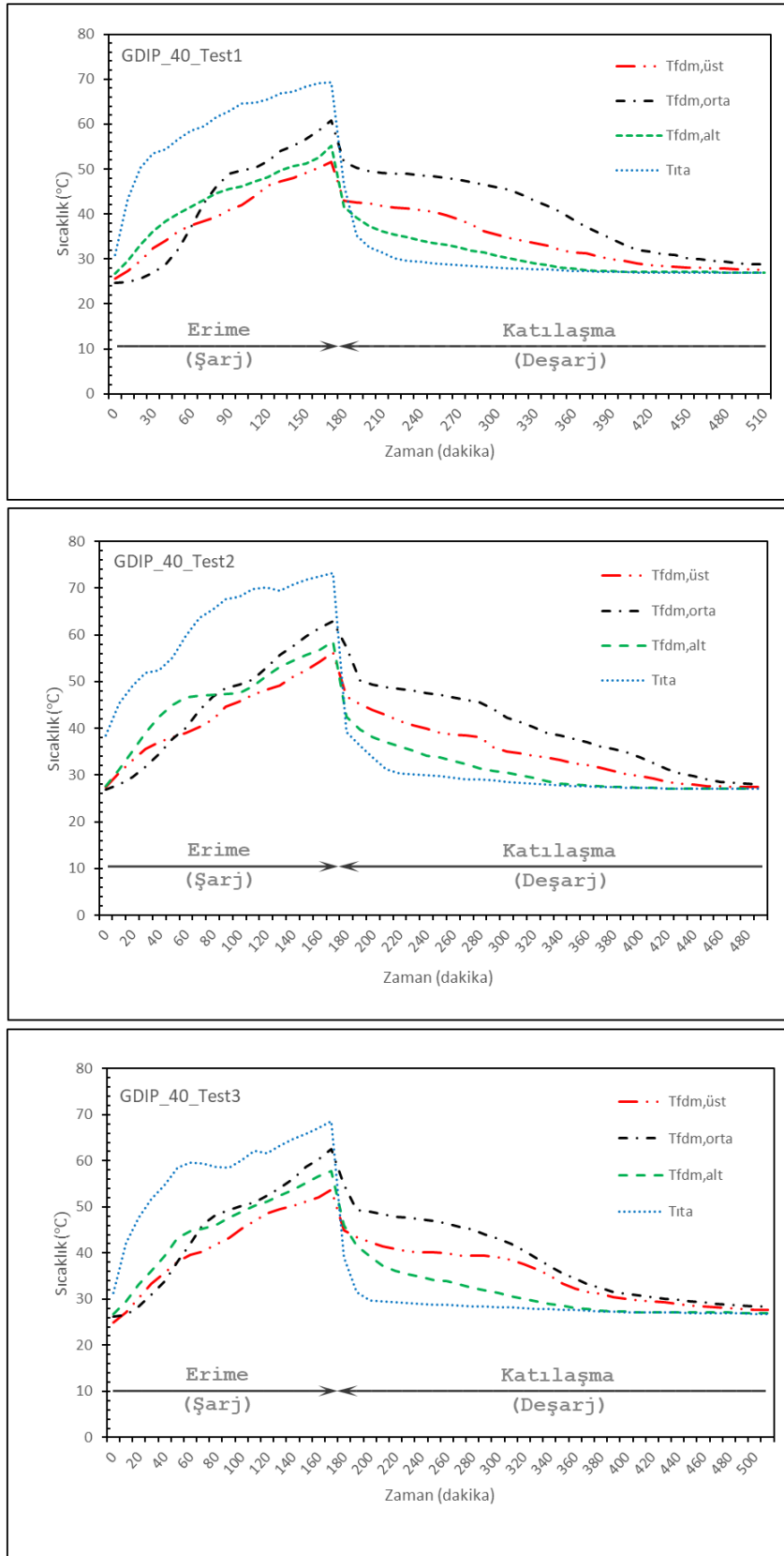
Şekil 7.19. GDIP sisteminde 40° açılı kolektör deneyinde erime ve katılaşma işlemi sırasında parafinin sıcaklığı
