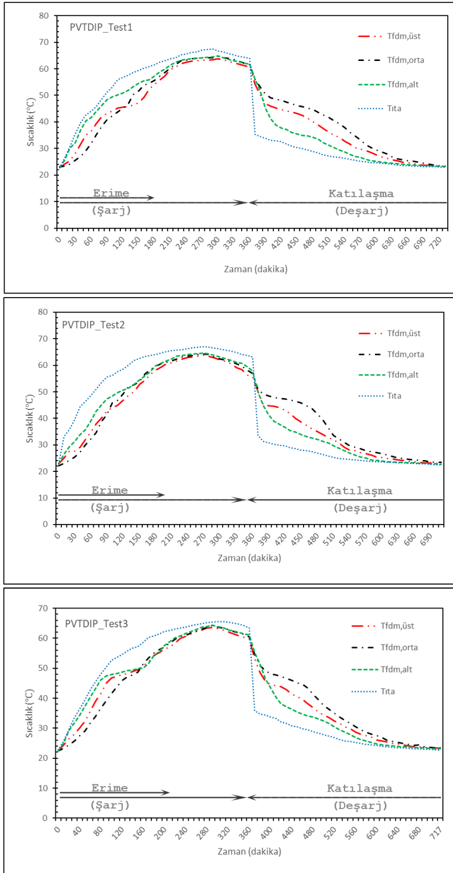
Şekil 7.27. PVT-DIP sisteminde erime ve katılaşma sırasında parafinin sıcaklığı
