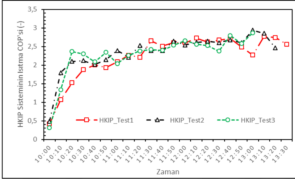
Şekil 7.7. HKIP sisteminin ısıtma COP değerleri
