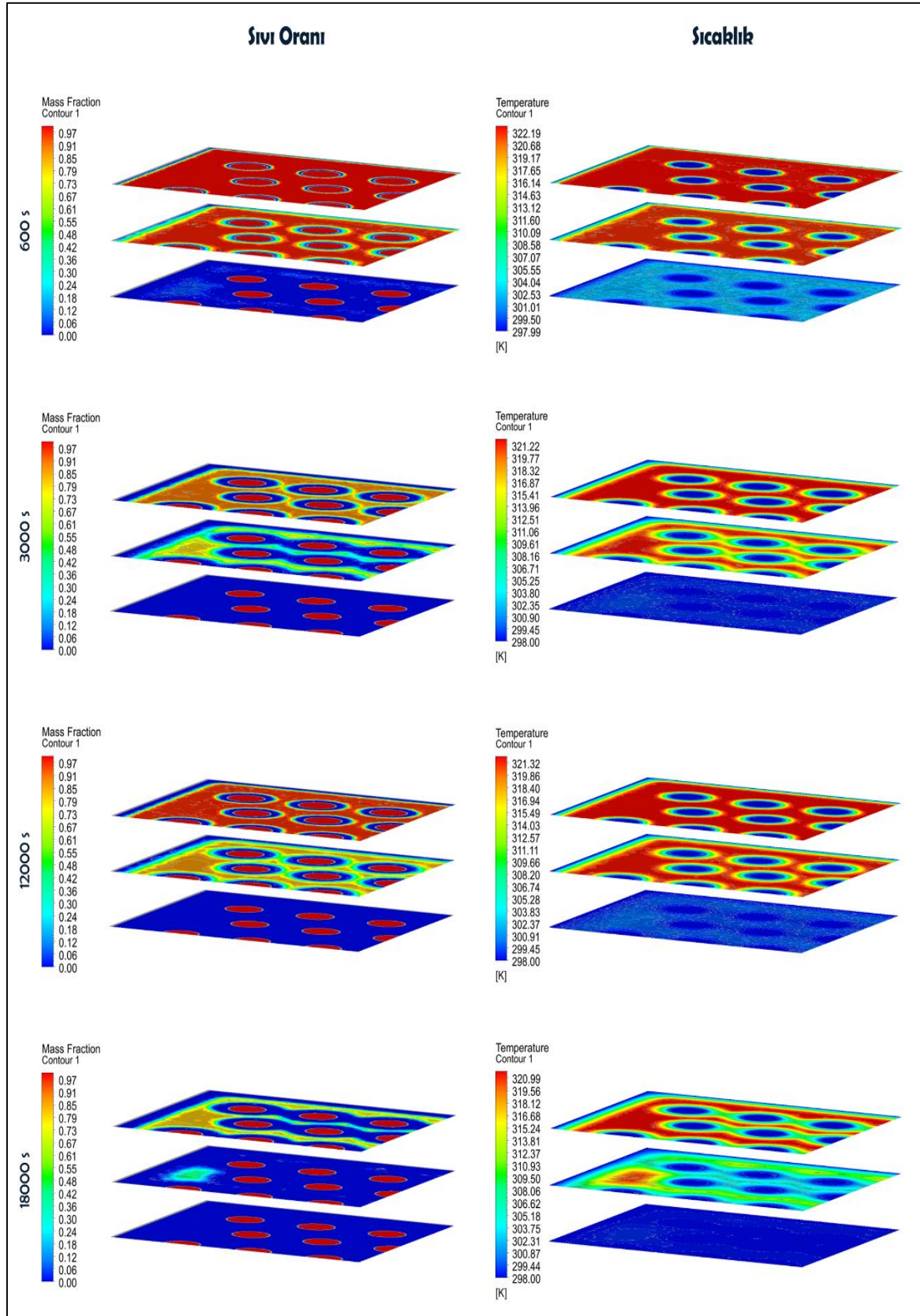
Şekil 7.3. Katılaştırma (deşarj) sırasında parafinin çeyrek simetrik model için sıvı oranı ve sıcaklık sınırları
