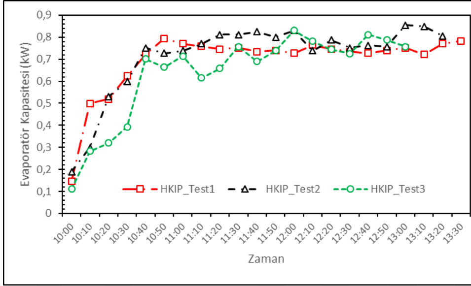
Şekil 7.10. HKIP sisteminin evaporator kapasitesi
