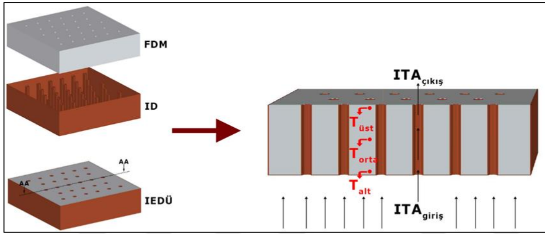
Şekil 6.4. Isıl enerji depolama ünitesinin şematik gösterimi ve yerleştirilen ısıl çiftlerin pozisyonları
