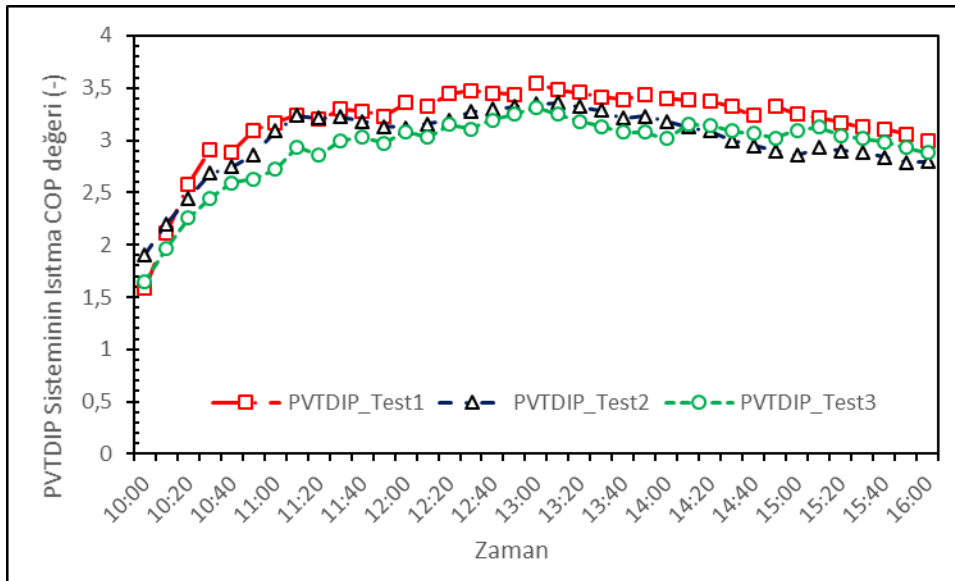
Şekil 7.24. PVTDIP sisteminin ısıtma performans katsayısı
