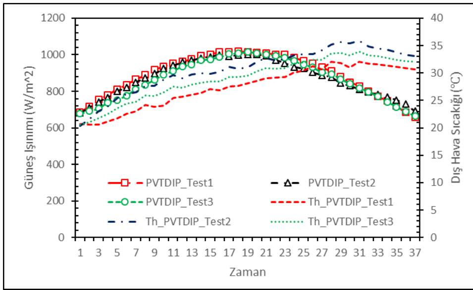
Şekil 7.21. PVTDIP deneylerinde zaman bağlı güneş ışınlamı ve dış hava sıcaklığı
