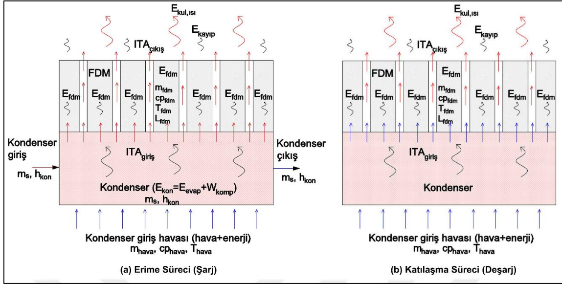
Şekil 6.10. Isıl enerji depolama ünitesindeki enerji dengesi
