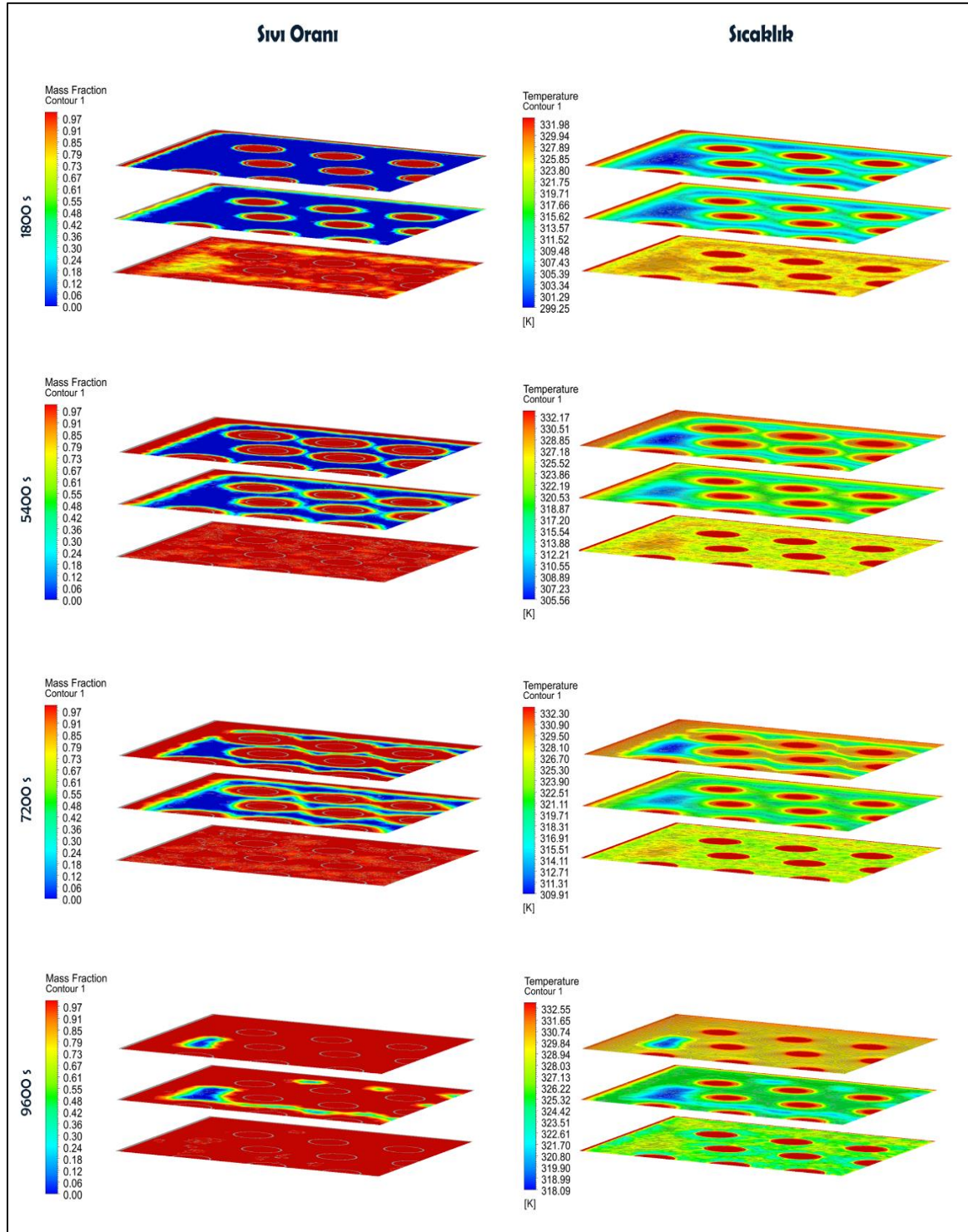
Şekil 7.1. Erime (şarj) sırasında parafinin çeyrek simetrik model için sıvı oranı ve sıcaklık konturları
