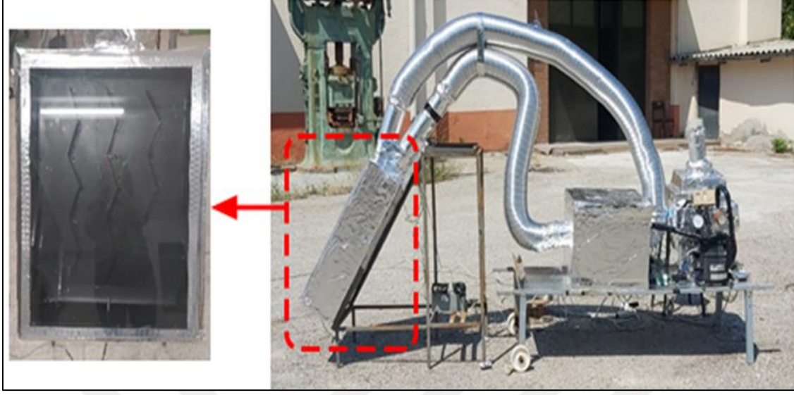
Ek-2. Isıl enerji depolamalı güneş destekli ısı pompası sisteminin fotoğrafı
