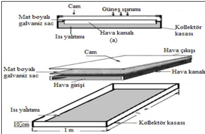
Şekil 2.4. Havalı güneş kollektörünün şematik gösterimi [15]
