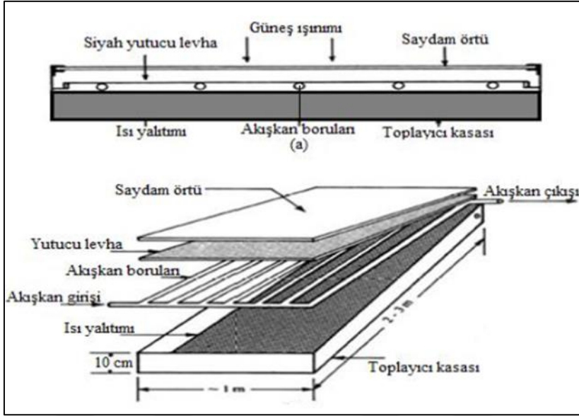
Şekil 2.3. Sıvı akışkanlı güneş kollektörünün şematik gösterimi [15]
