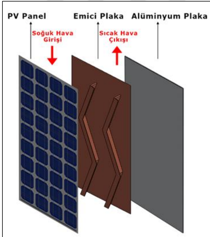
Şekil 6.9. PVT panelin ana parçaları
