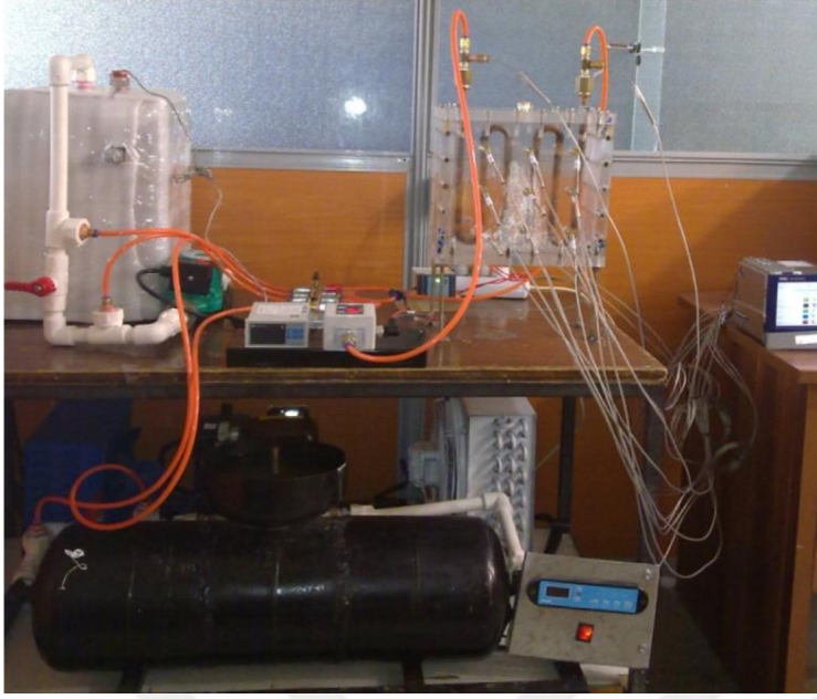
Resim 5.4. Rahimi ve diğerlerinin deney düzeneği [99]
