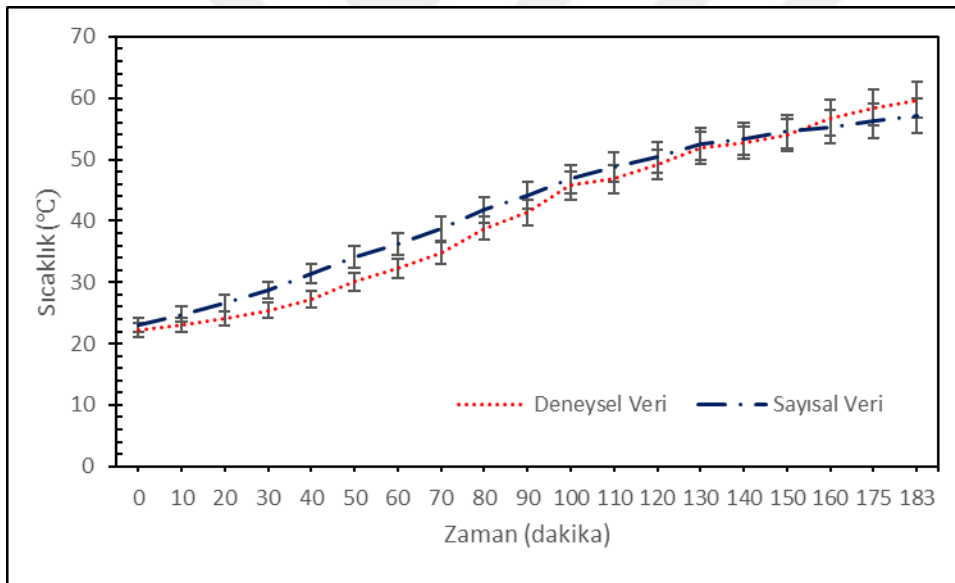
Şekil 7.30. Sayısal analiz sonucunun deneysel analiz sonucu ile doğrulanması
