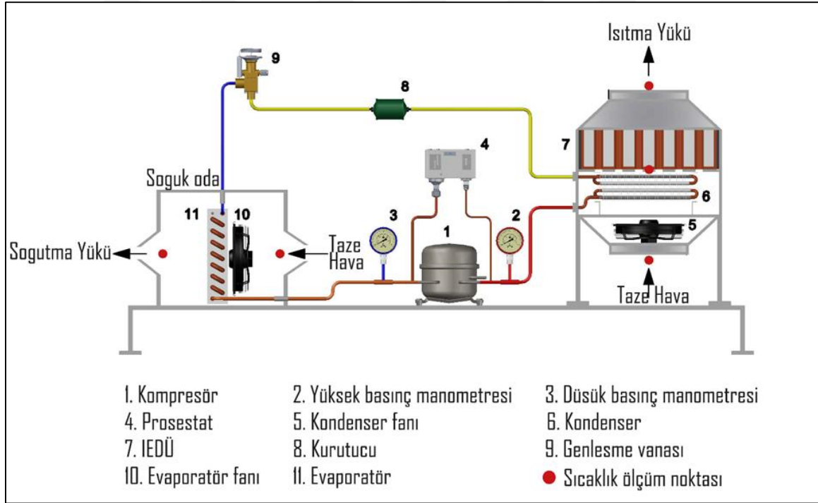
Şekil 6.6. Isıl enerji depolamalı hava kaynaklı ısı pompası sisteminin şematik gösterimi
