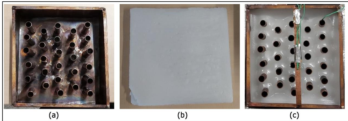
Şekil 6.3. (a) İmal edilen ısı değiştiricisi, (b) Parafin, (c) ısıl enerji depolama ünitesi
