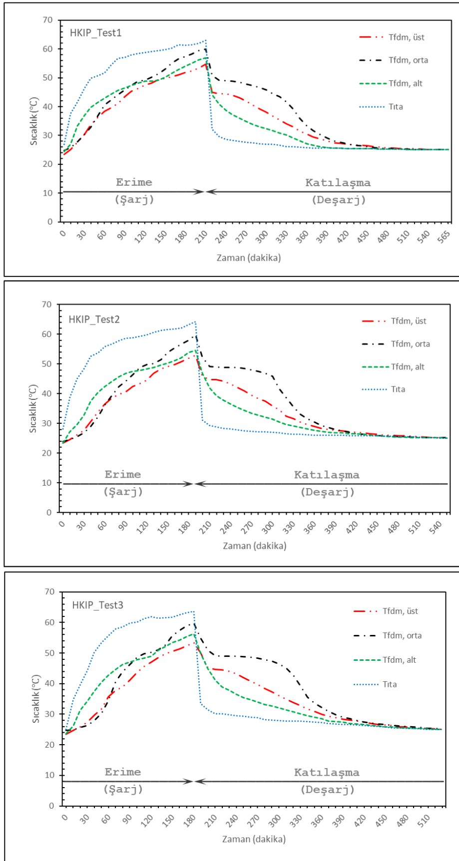
Şekil 7.11. HKIP sisteminde erime ve katılaşma sırasında parafinin zamana bağlı sıcaklığı
