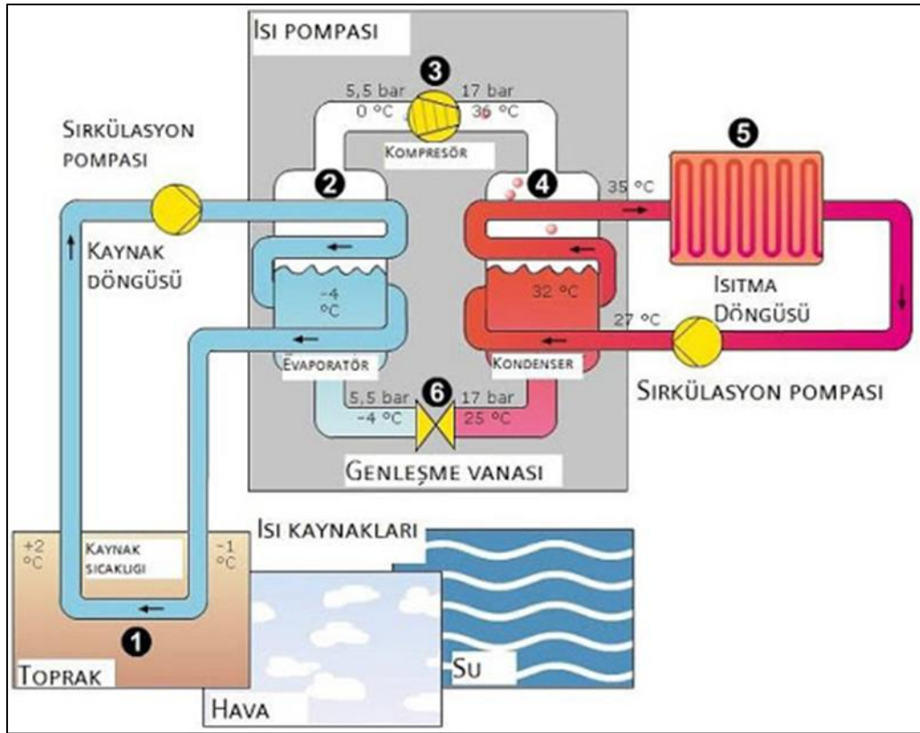
Şekil 3.2. Isı kaynaklarına göre ısı pompası sistemi örneği [25]
