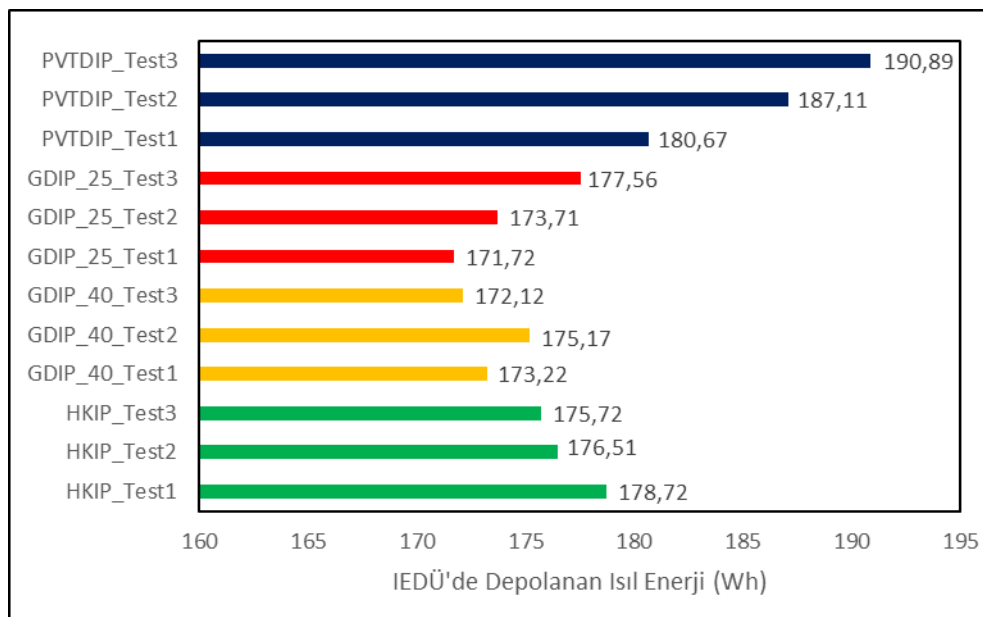
Şekil 7.29. IEDÜ'deki parafinde depolanılan ısı enerjisi miktarı
