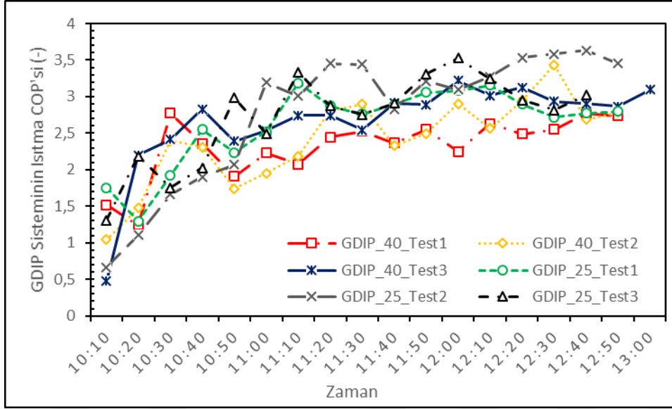
Şekil 7.17. GDIP sisteminin ısıtma performans katsayısı
