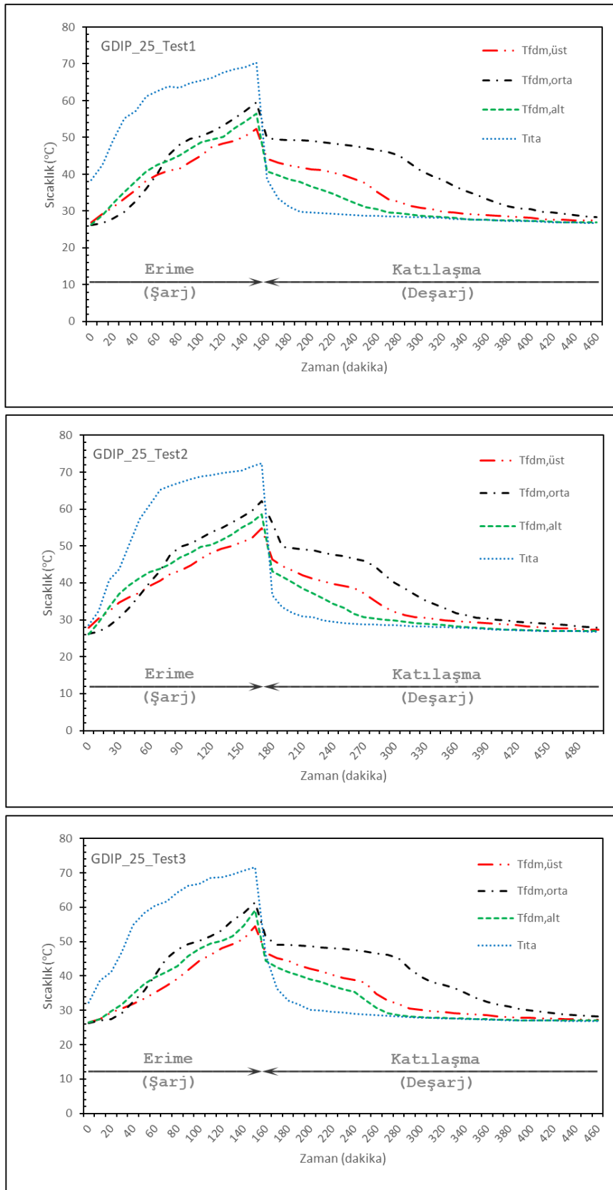
Şekil 7.20. GDIP sisteminde 25° açılı kolektör deneyinde erime ve katılaşma işlemi sırasında parafinin sıcaklığı
