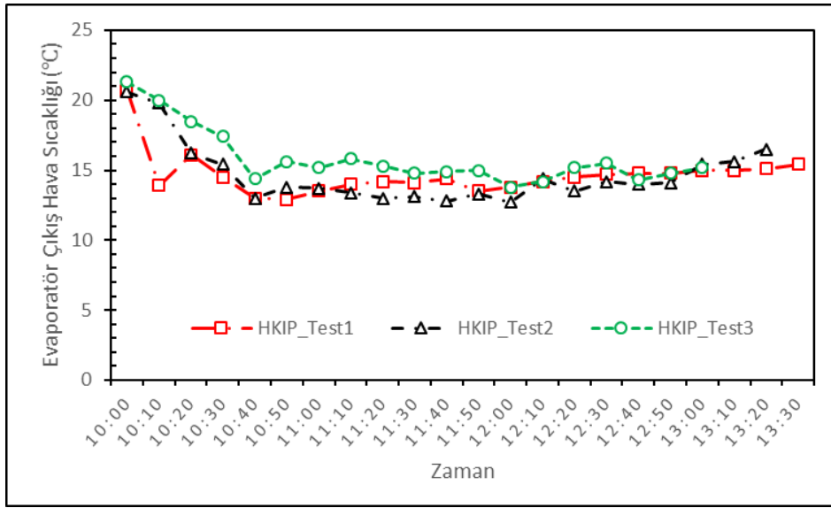
Şekil 7.6. HKIP sisteminin evaporatör hava çıkış sıcaklığı
