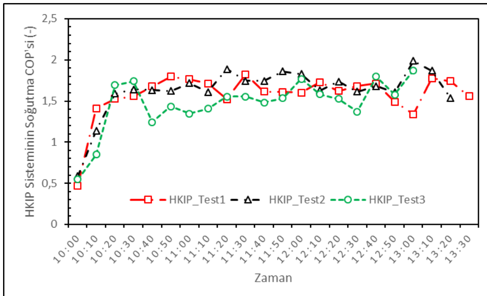
Şekil 7.8. HKIP sisteminin soğutma COP değerleri
