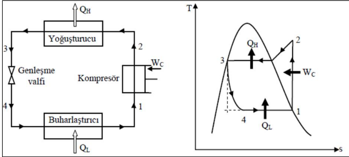
Şekil 3.1. İdeal buhar sıkıştırırmalı soğutma çevrimi [24]
