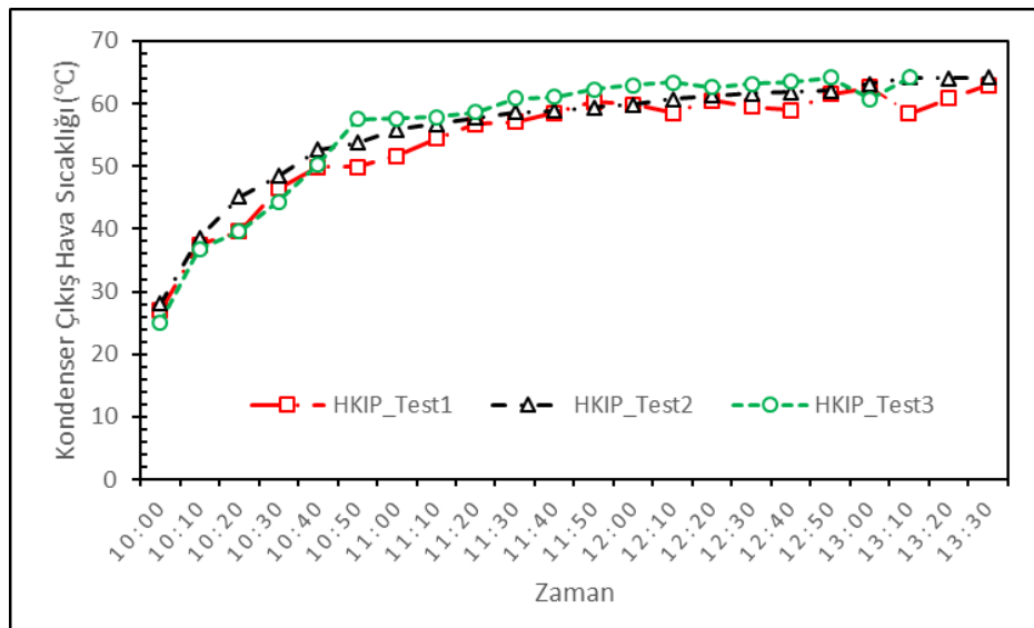
Şekil 7.5. HKIP sisteminin kondenser hava çıkış sıcaklığı
