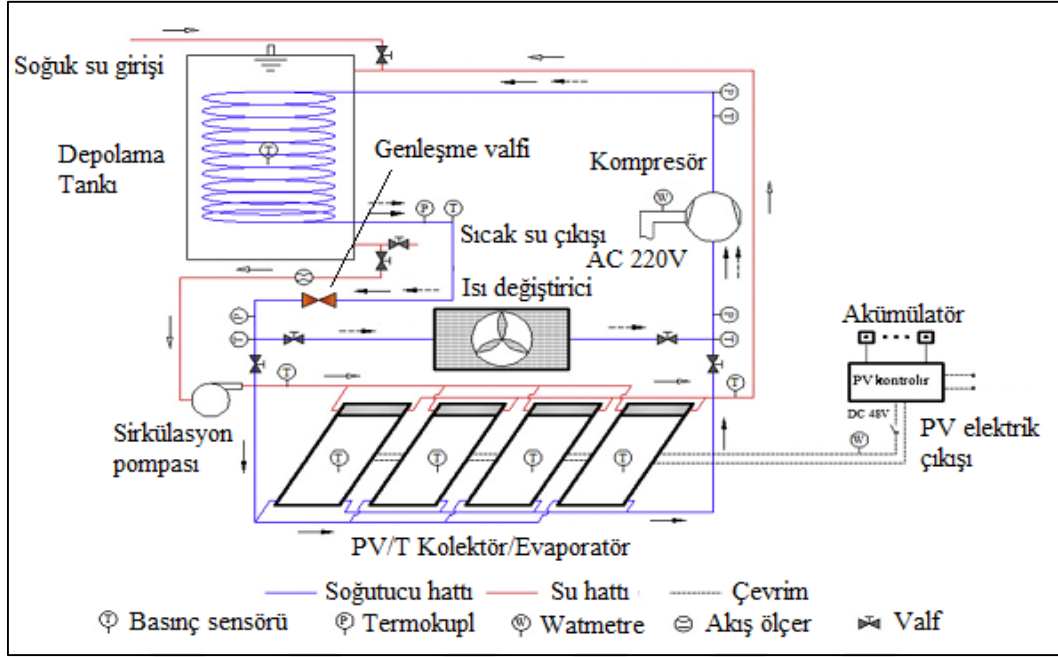
Şekil 5.6. PV-SAHP/HP test ekipmanının şematik diyagramı [79]
