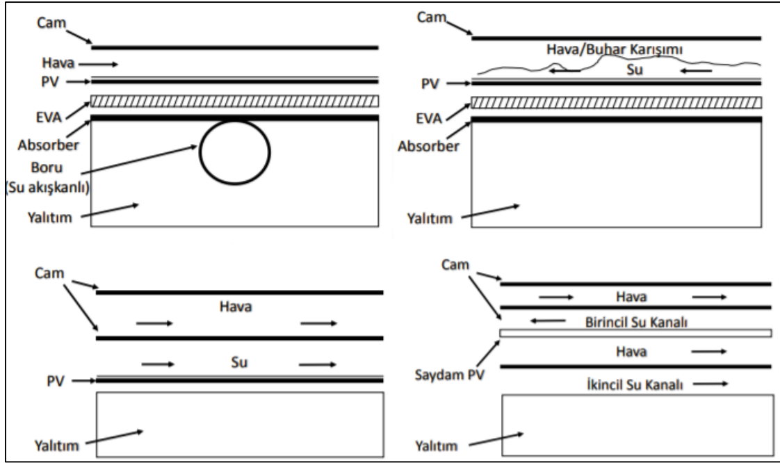
Şekil 2.7. Fotovoltaik-termal güneş panel çeşitleri [21]
