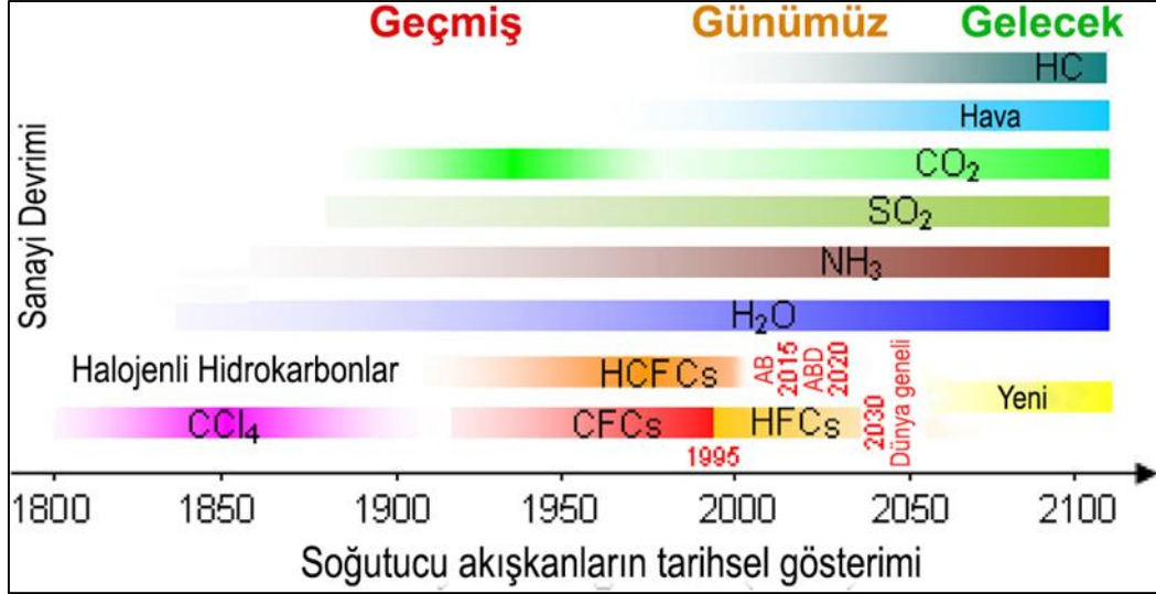
Şekil 3.5. Soğutucu akışkanların tarihsel gelişimi [35]
