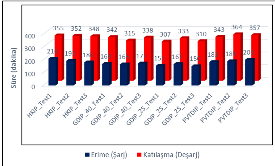
Şekil 7.28. IEDÜ'deki parafinin erime ve katılaşma süreleri
