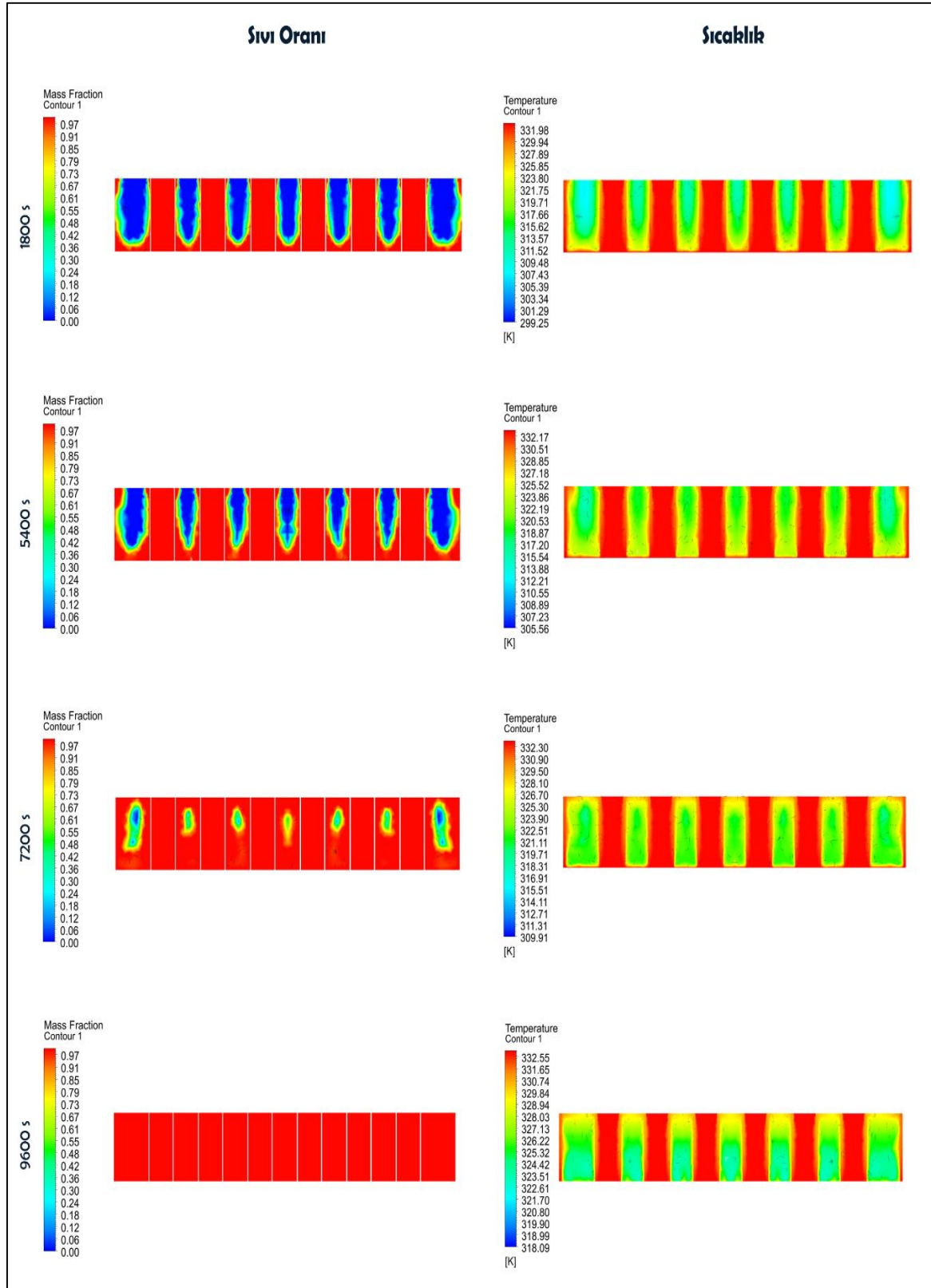
Şekil 7.2. Erime (şarj) sırasında parafinin yarım kesit model için sıvı oranı ve sıcaklık konturları
