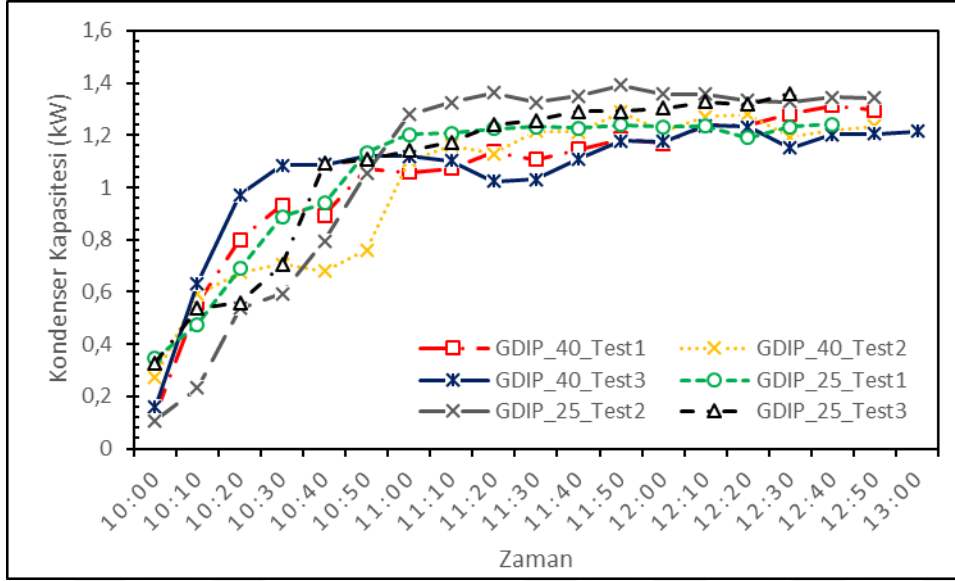
Şekil 7.16. GDIP deneylerinde kondenser kapasiteleri
