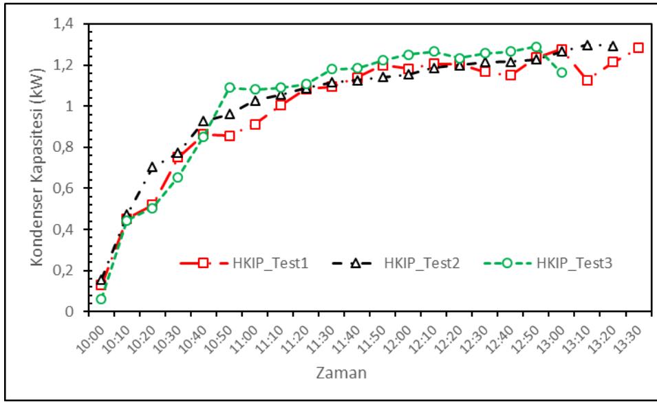
Şekil 7.9. HKIP sisteminin kondenser kapasitesi
