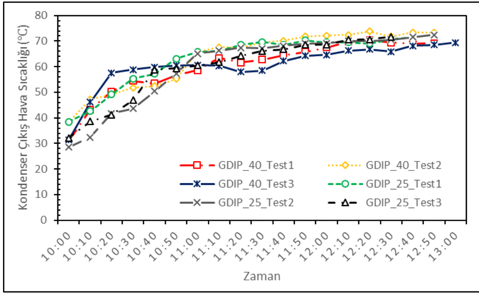
Şekil 7.15. GDIP sisteminin kondenser çıkış hava sıcaklığı grafiği
