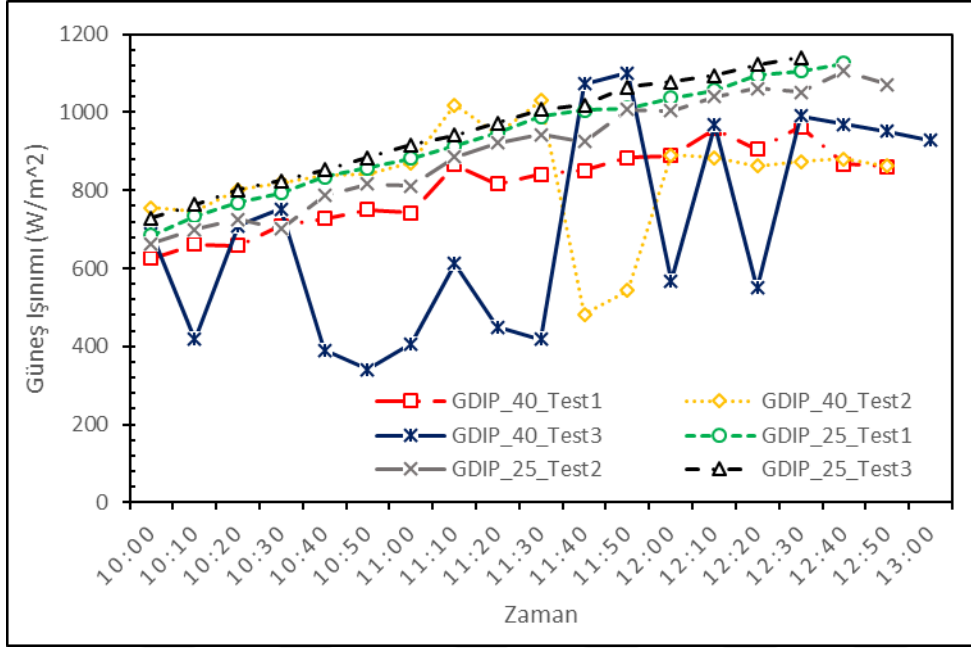
Şekil 7.13. GDIP deneylerinde zamana bağlı güneş ışınlamı değerleri
