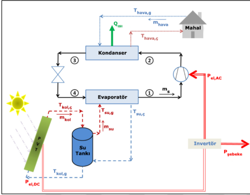
Şekil 5.5. PVT ısı pompası sistemi [78]
