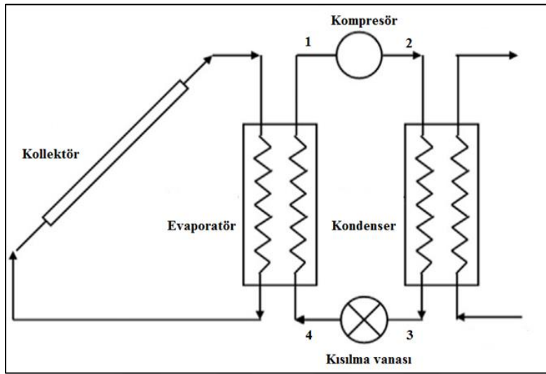
Şekil 3.4. Dolaylı genleşmeli güneş destekli ısı pompası sisteminin şeması [27]
