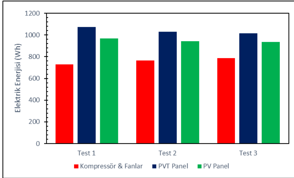
Şekil 7.26. PVTDIP sisteminde elektrik enerjisi dağılımı
