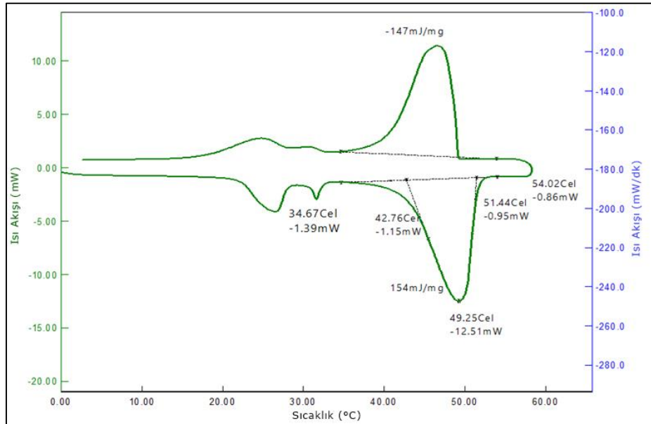
Şekil 6.5. Parafinin DSC eğrisi
